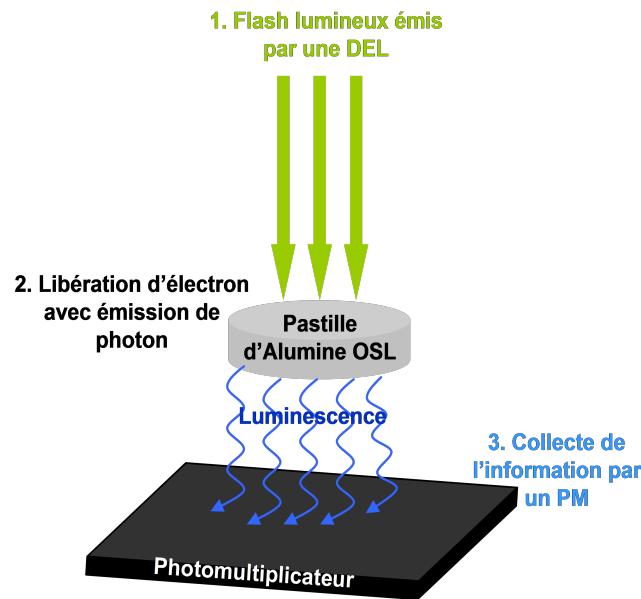
FIGURE 4.4 – Schéma de la procédure globale de lecture de l'OSL.
