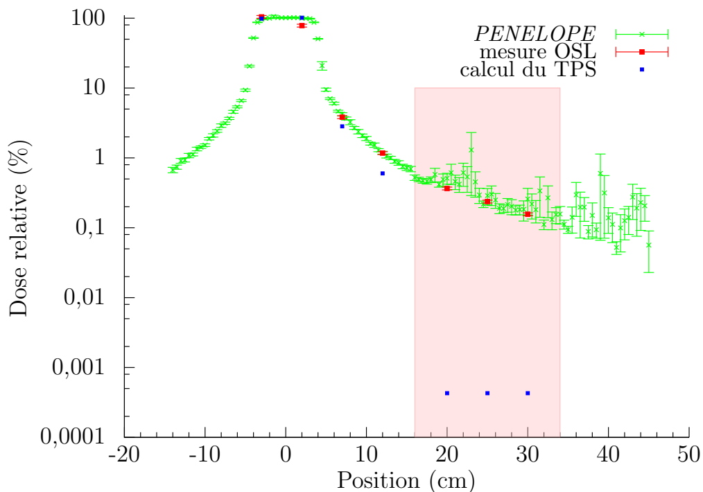
FIGURE 5.19 – Comparaison des doses calculées par PENELOPE et le TPS et mesurées par l’OSL selon l’axe du poumon droit. La zone pulmonaire est signalée en rose.
