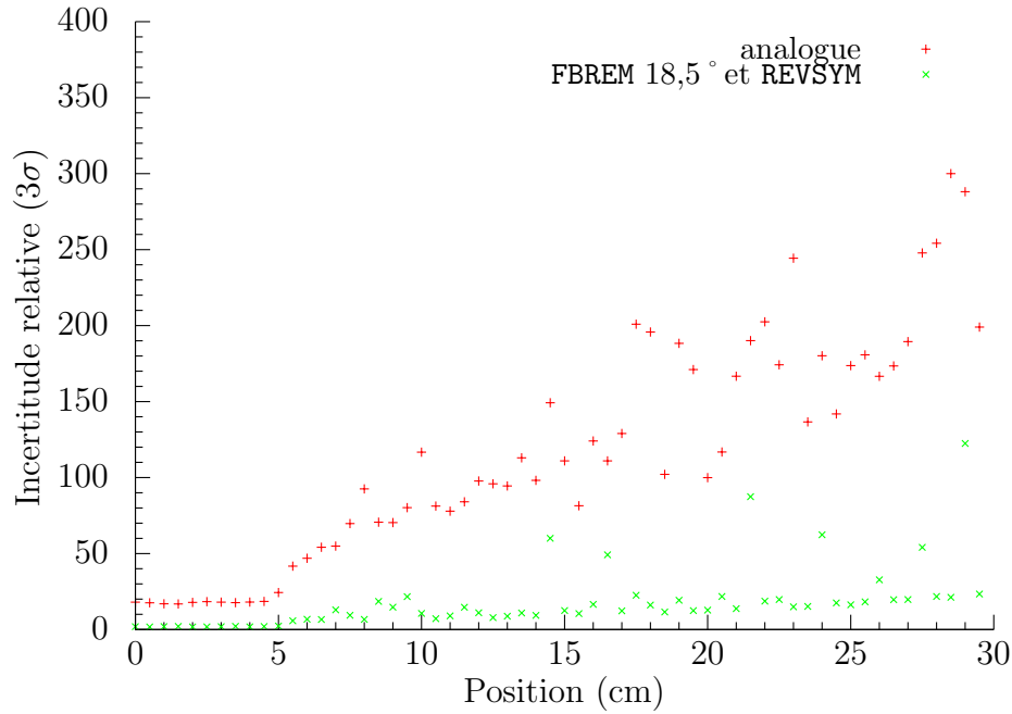
FIGURE 2.12 – Impact des deux techniques de réduction de variance sur l'incertitude statistique relative comparativement à la simulation analogue. L'irradiation est faite à 12 MV avec un champ de 10 \times 10 \text{ cm}^2 et avec 10^8 et 10^9 histoires simulées, respectivement, pour la simulation non-analogue et analogue.
