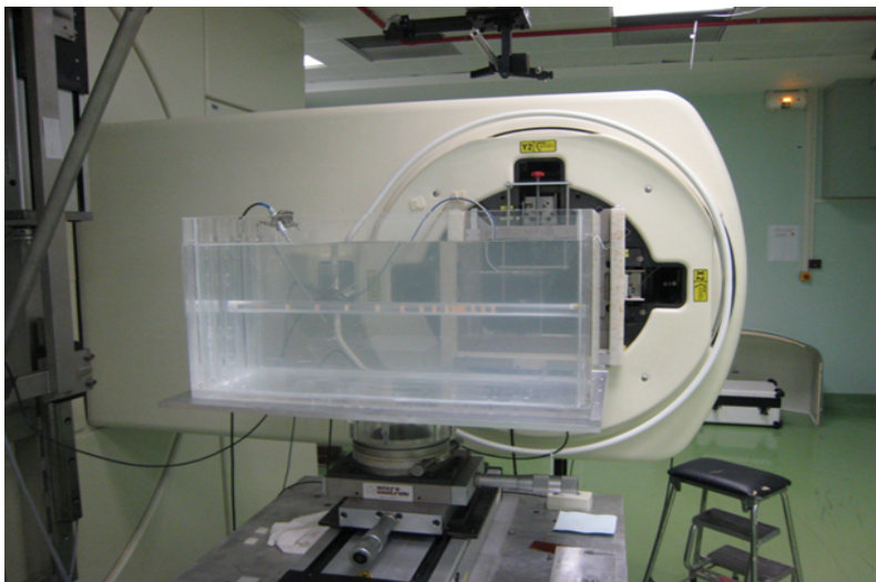
FIGURE 5.3 – Photographie de la cuve à eau positionnée dans l'axe du faisceau de l'accélérateur GE SATURNE 43 .
