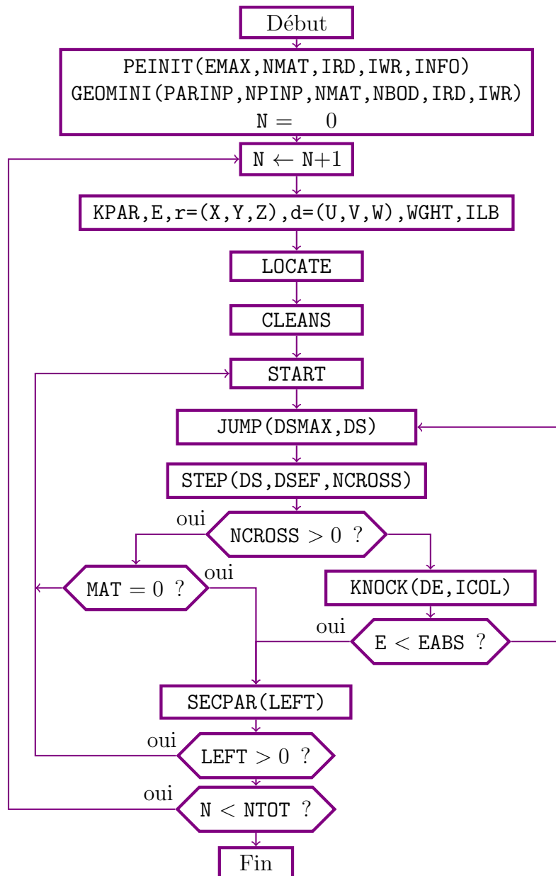
FIGURE 2.1 – Diagramme de flux du programme principal penmain.f de PENELOPE .
