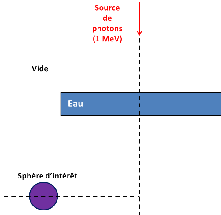
FIGURE 3.13 – Schéma de la configuration simple de test de l'implémentation du processus pseudo-déterministe avec penmain_simple.f .
