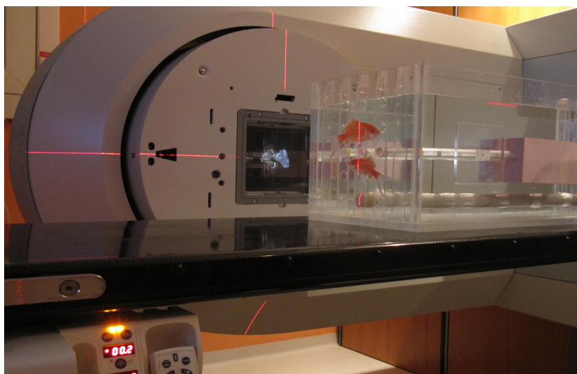
FIGURE 5.15 – Photographie de la cuve placée sous le faisceau latéral droit défini par le MLC de l'Artiste.
