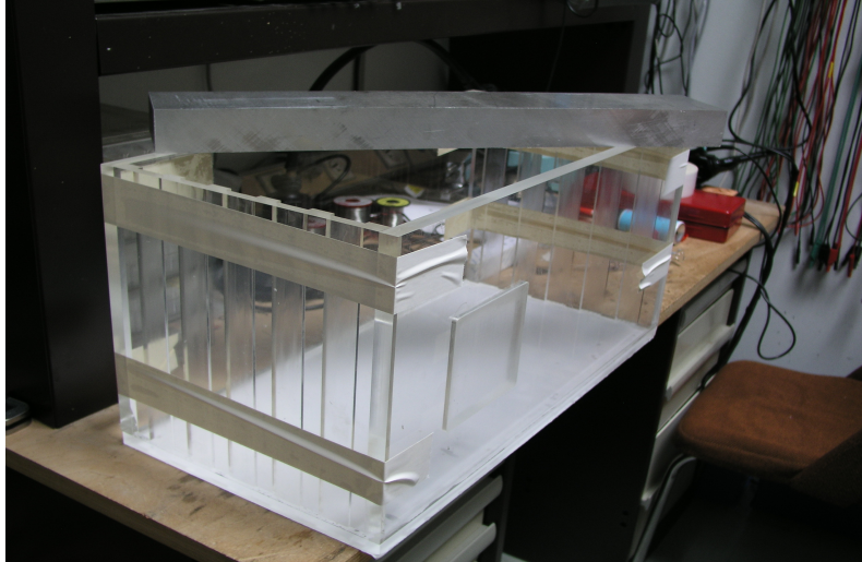
FIGURE 5.2 – Photographie de la cuve à eau spécifique lors de son assemblage.
