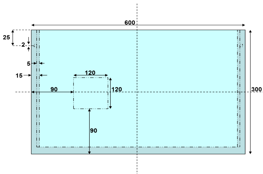
FIGURE 5.1 – Schéma de la cuve vue depuis le faisceau avec la fenêtre d’entrée traversée par le faisceau (les dimensions sont données en mm).
