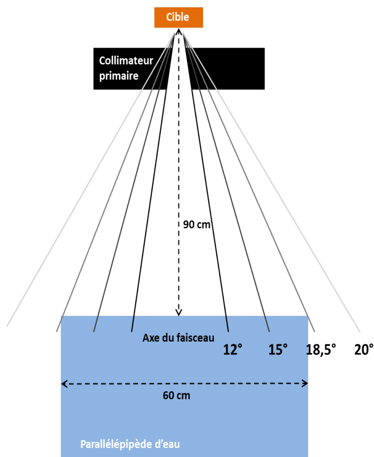
FIGURE 2.8 – Définition des ouvertures testées pour l'optimisation des paramètres du splitting du bremsstrahlung .
