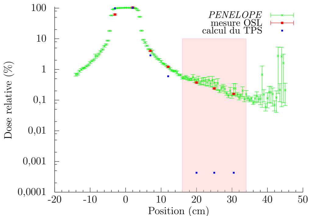
FIGURE 5.18 – Comparaison des doses calculées par PENELOPE et le TPS et mesurées par l’OSL selon l’axe du poumon gauche. La zone pulmonaire est signalée en rose.
