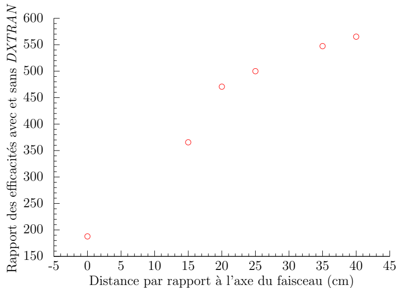
FIGURE 3.5 – Rapport de l'efficacité du calcul de dose avec et sans DXTRAN selon l'éloignement de la sphère de l'axe principal du faisceau.
