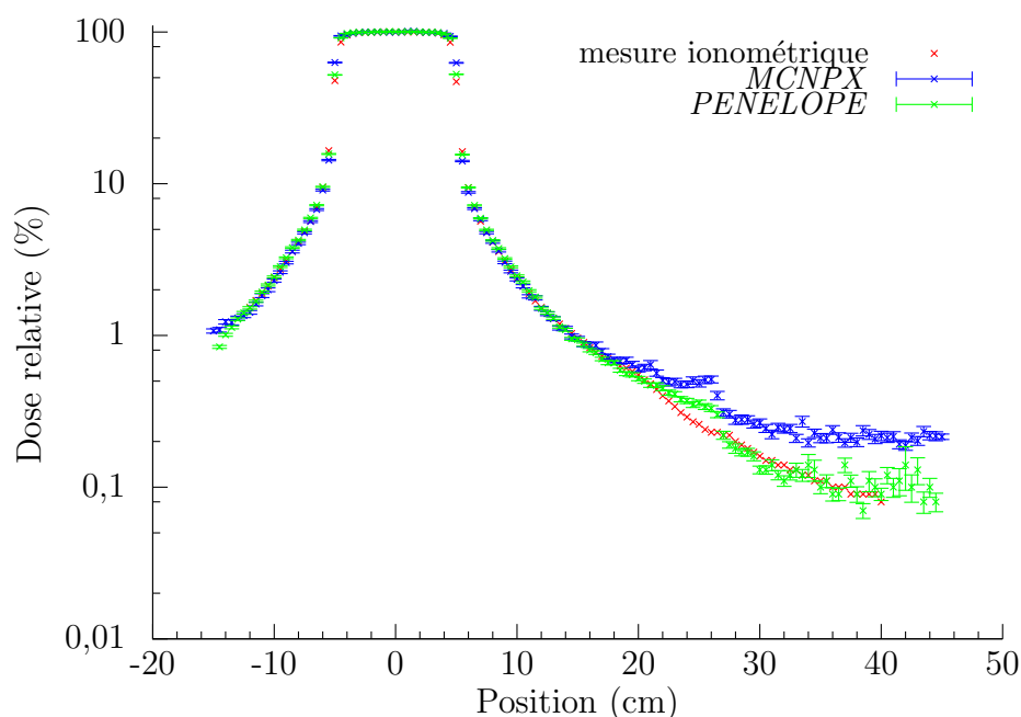
FIGURE D.1 – Profils de dose relative calculés avec PENELOPE , MCNPX et mesuré avec une chambre d'ionisation à 10 cm de profondeur dans un parallélépipède d'eau, à une distance de 100 cm de la source. L'irradiation est faite à une qualité de faisceau correspondant à 12 MV avec une taille de champ de 10 \times 10 \text{ cm}^2 .
