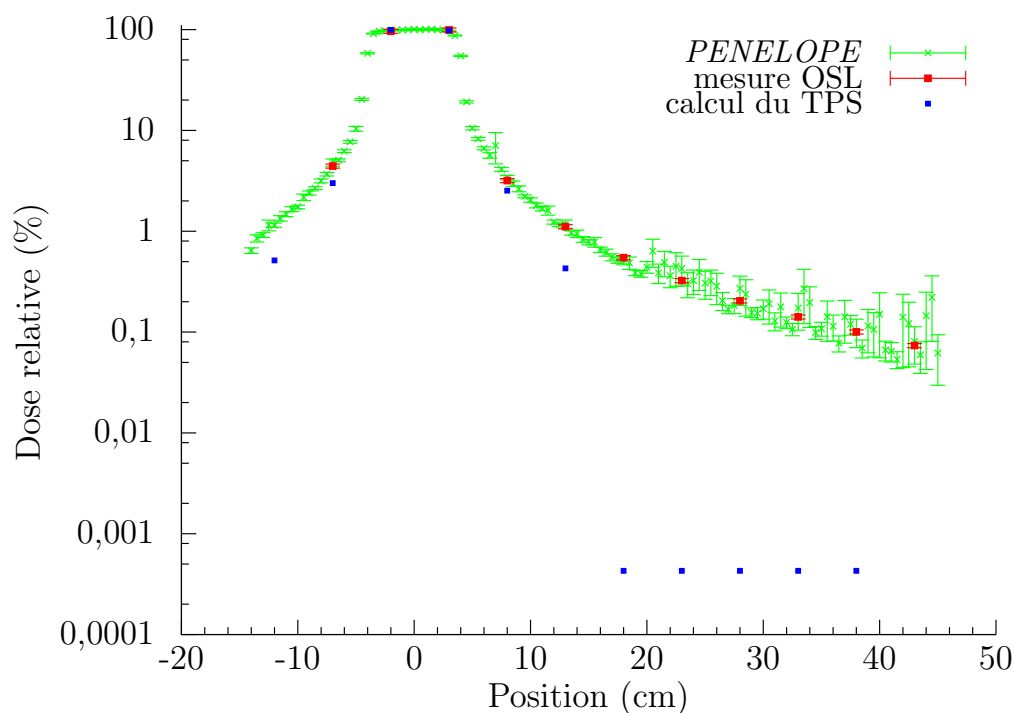
FIGURE 5.17 – Comparaison des doses calculées par PENELOPE et le TPS et mesurées par l'OSL selon l'axe de la prostate.
