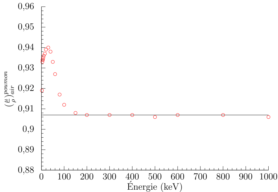
FIGURE 5.16 – Rapport des coefficients d’absorption massiques entre un matériau équivalent poumon et l’air (données du NIST).
