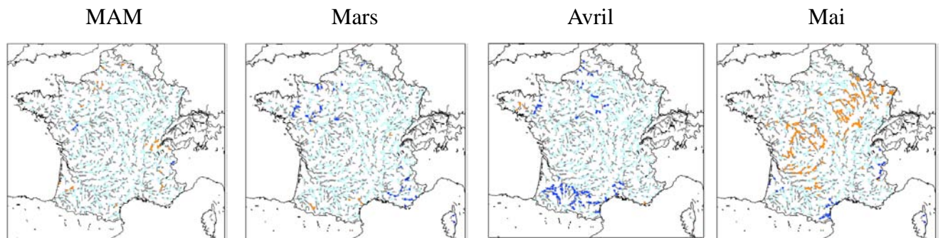
FIG. 6.16. Régions où : l'expérience avec la descente d'échelle DSCLIM est meilleure que celle avec la descente d'échelle simple (en orange) ; l'expérience avec la descente d'échelle simple est meilleure qu'avec DSCLIM (en bleu foncé) ; les deux expériences sont équivalentes (bleu clair) ; les calculs sont réalisés pour les 100 \Delta R pour les débits moyens trimestriels et mensuels (cf. détails sect. 4.3).
