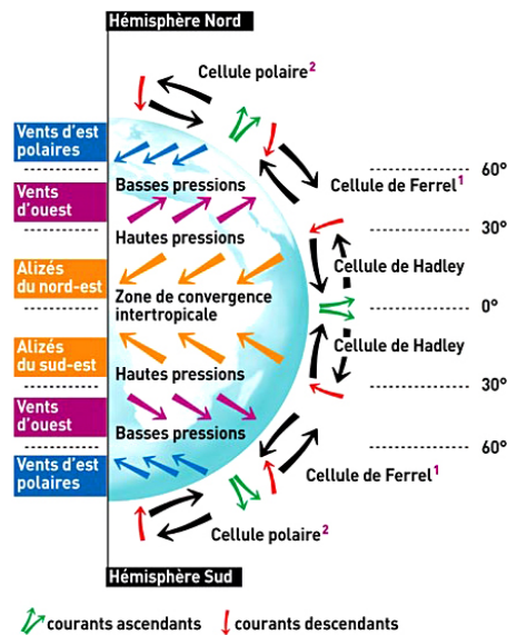
FIG. 1.3. Coupe schématisée de la circulation atmosphérique générale [CEA, source : http://www.cea.fr/jeunes/themes/le_climat/le_climat/complements_sur_le_climat/fonctionnement_de_la_circulation_atmospherique_m ]
