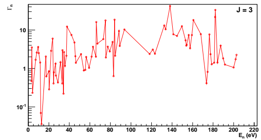
FIGURE 2.55 – Largeur neutronique des résonances de spin J = 3 en fonction de l'énergie neutron.
