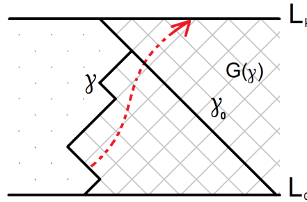
FIGURE 3.2 – En pointillés, l'évènement \{\gamma_{|[0,k]} \rightarrow ([\gamma_k, \infty[, k) \text{ dans } G(\gamma)\} .
