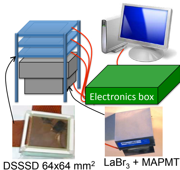
FIG. 5.1 – Schéma de principe du prototype de télescope Compton à rayons gamma développé à Orsay. Cet instrument associera un calorimètre-imageur en \text{LaBr}_3\text{:Ce} à trois couches minces de détecteurs silicium à pistes double-faces.
