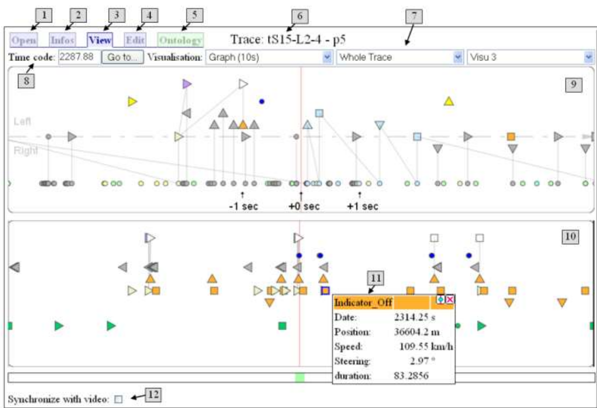
Figure 1-12 Visualisation in ABSTRACT ( http://liris.cnrs.fr/abstract )
