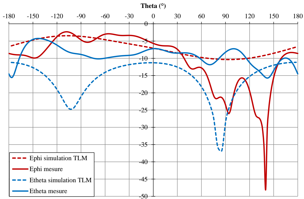
Figure III-42 : Diagramme de rayonnement de l'antenne adaptée dans le plan H
