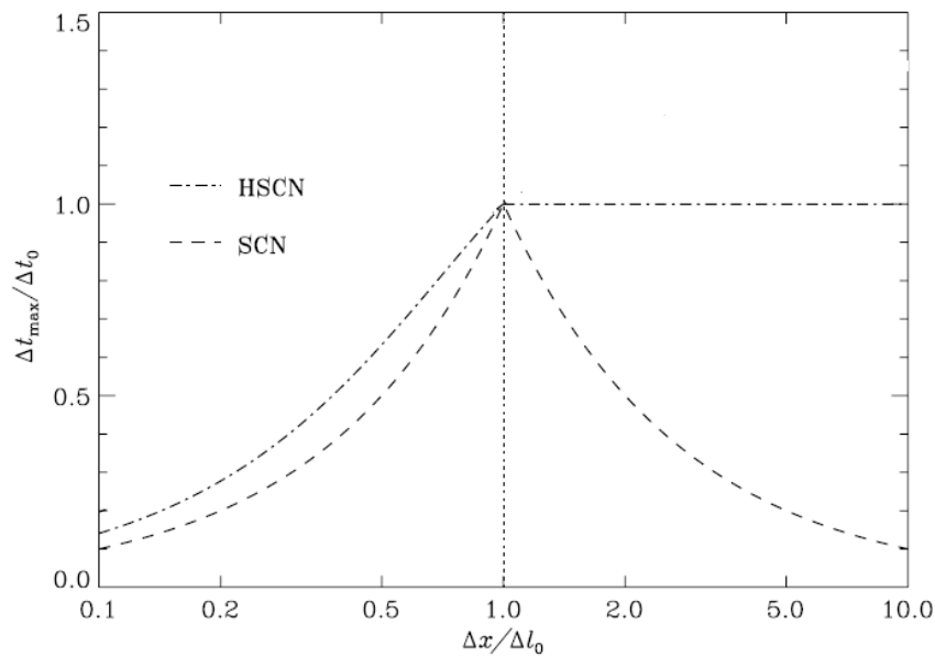
Figure I-13 : Evolution du pas temporel maximal dans le vide pour les nœuds SCN et HSCN lorsque la dimension de la cellule varie
