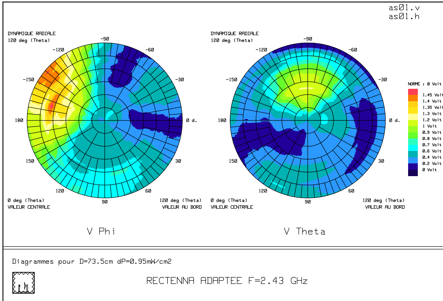
Figure III-60 : Diagrammes 3D de la tension continue récupérée par la rectenna adaptée pour une distance de 73.5cm
