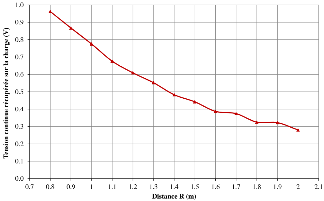
Figure III-67 : Tension continue récupérée par la rectenna optimisée en fonction de la distance
