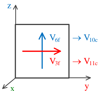
Figure II-5 : Impulsions sur les interfaces entre le maillage grossier et le maillage fin
