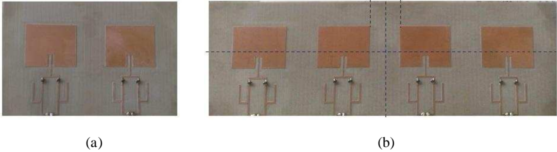
Figure III-13 : Réseaux de rectennas (a) à 2 éléments (b) à 4 éléments [Takhedmit10]
