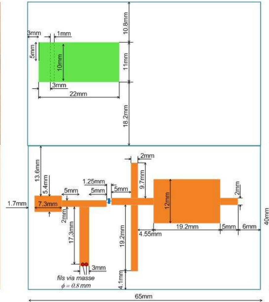
Figure III-65 : Dimensions de la rectenna optimisée ( 65 \times 40 \times 2 \text{mm}^3 )
