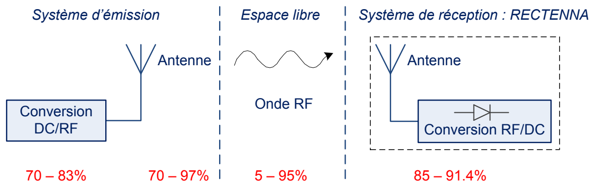
Figure III-5 : Principe de la TESH et les différents rendements d'un système de TESH
