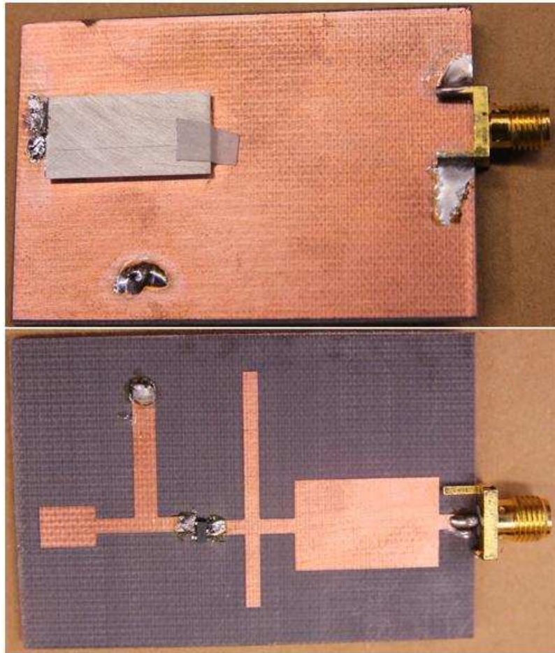
Figure III-65 : Dimensions de la rectenna optimisée ( 65 \times 40 \times 2 \text{mm}^3 )
