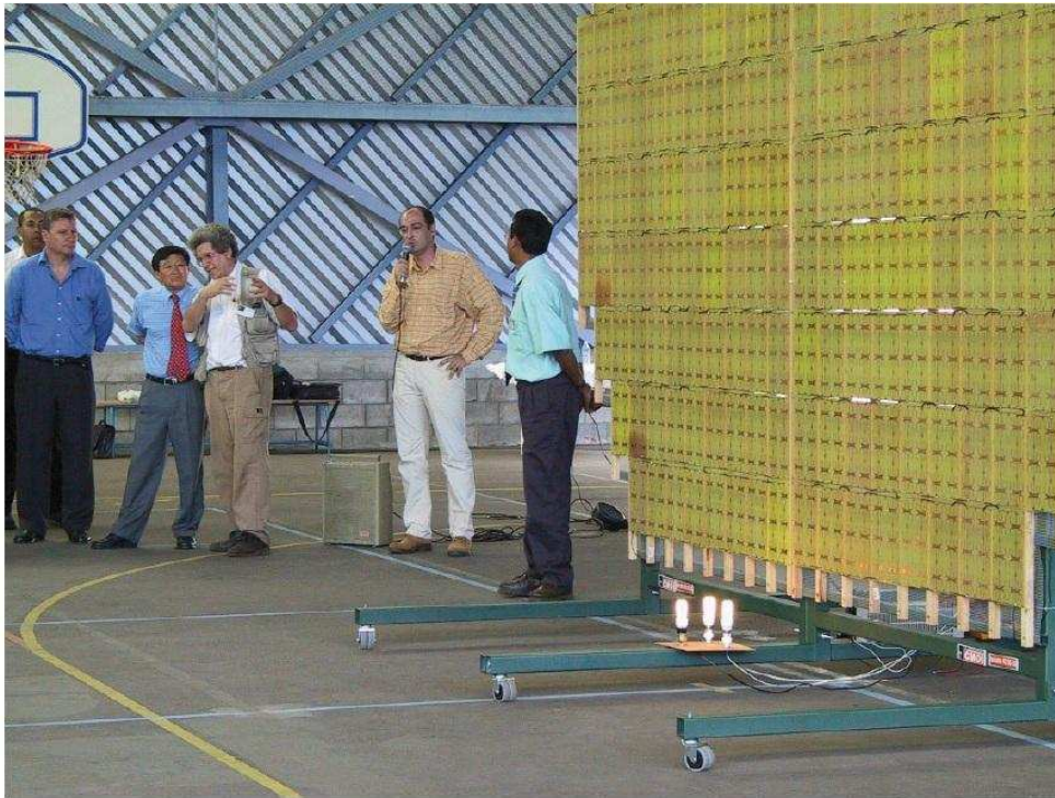
Figure III-4 : Panneau des rectennas alimentant les lampes
