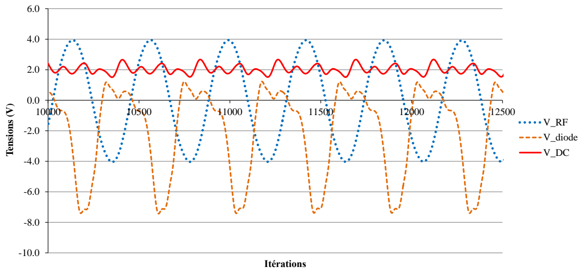
Figure III-29 : Tensions temporelles aux bornes du générateur, de la diode et de la charge quand l'amplitude du signal d'entrée est de 4\text{V}
