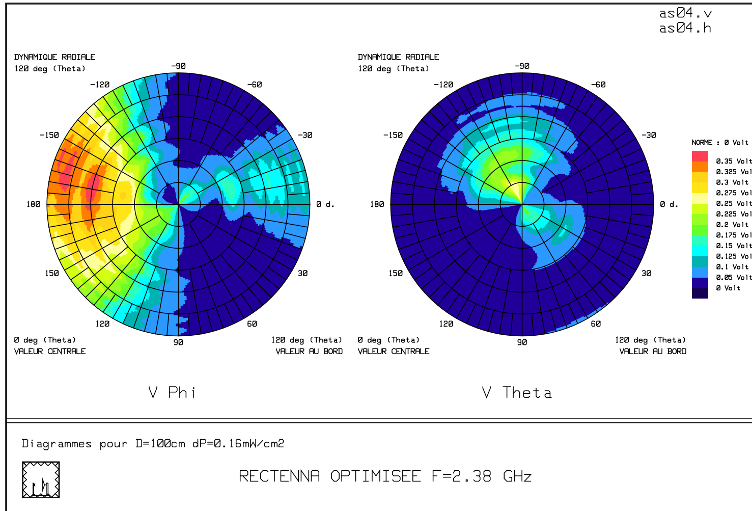
Figure III-71 : Diagrammes 3D de la tension continue récupérée par la rectenna optimisée pour une densité de puissance de 0.16mW/cm 2
