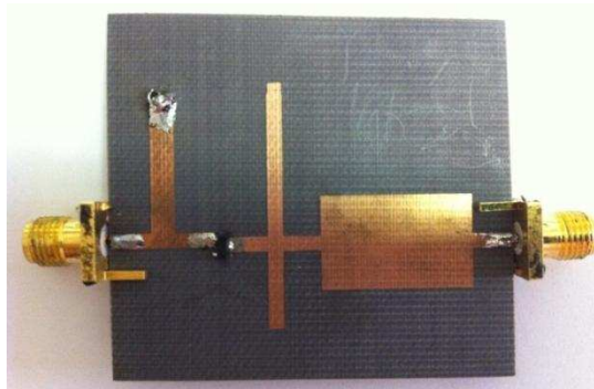
Figure III-63 : Circuit de redressement sans le module d'adaptation
