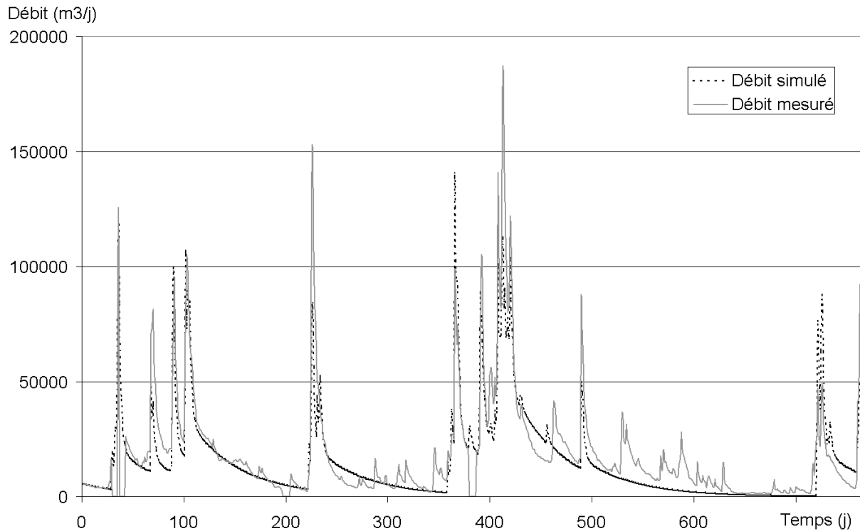
Figure 61. Résultats graphiques de la phase de validation sur la source du Rubicon (avec un décalage d'une journée dans la chronique de débit simulé).
