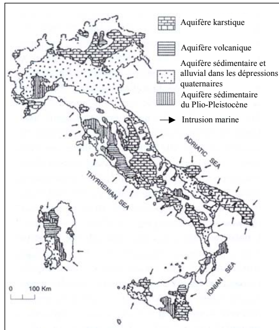
Figure 37. Salinisation des aquifères karstiques côtiers en Espagne (d'après Gomez, 2003) et en Italie (d'après Barrocu, 2003).
