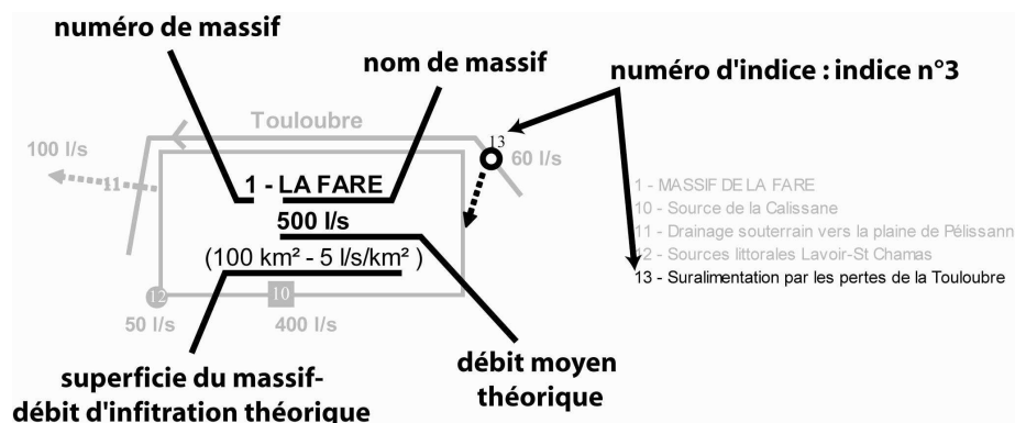
Figure 5-20 : Schéma explicatif pour la lecture du schéma de bilan hydrique global. Exemple du massif de la Fare
