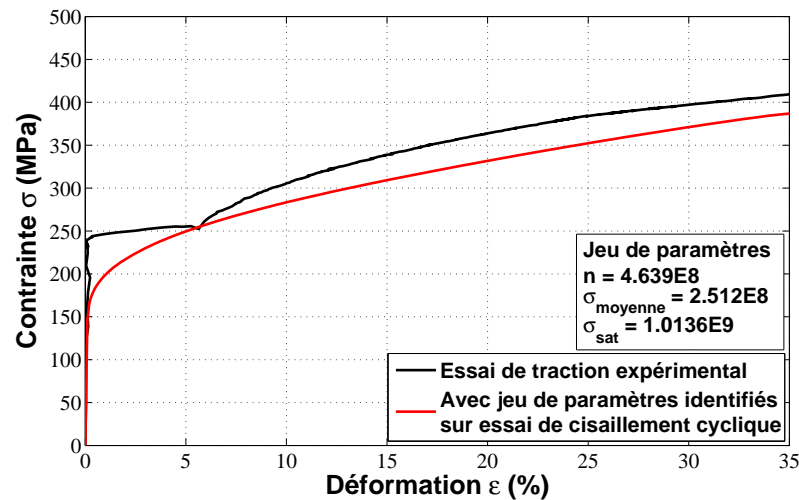
Fig. 4.3.13: Comparaison de la courbe contrainte en fonction de la déformation \sigma(\epsilon) provenant de l'essai de traction expérimental et numérique avec jeu de paramètres optimisé du comportement local issu de l'essai de cisaillement.
