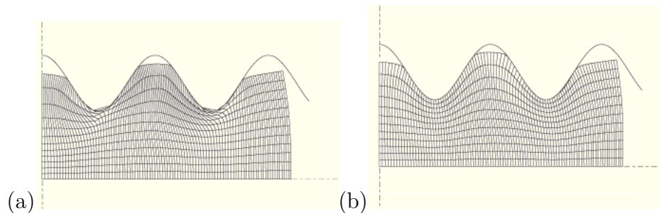
Fig. 1.5.1: Comparaison d'un maillage : (a) sans ALE et (b) avec ALE d'après [?].
