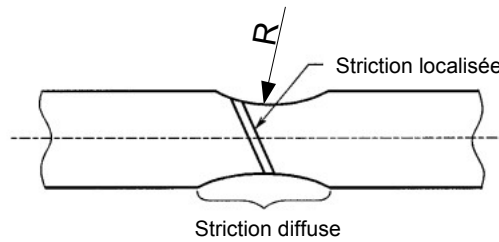
Fig. 2.2.1: Éprouvette de type cylindrique faisant apparaître deux types de striction : la striction diffuse et la striction localisée ainsi que le rayon de courbure R utilisé par la méthode de Bridgman.
