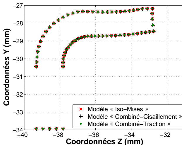
Fig. 4.2.7: Profils de pièce déformée issus de trois simulations effectuées avec trois modèles de comportement différents : « Iso-Mises », « Combiné-Cisaillement » et « Combiné-Traction ».
