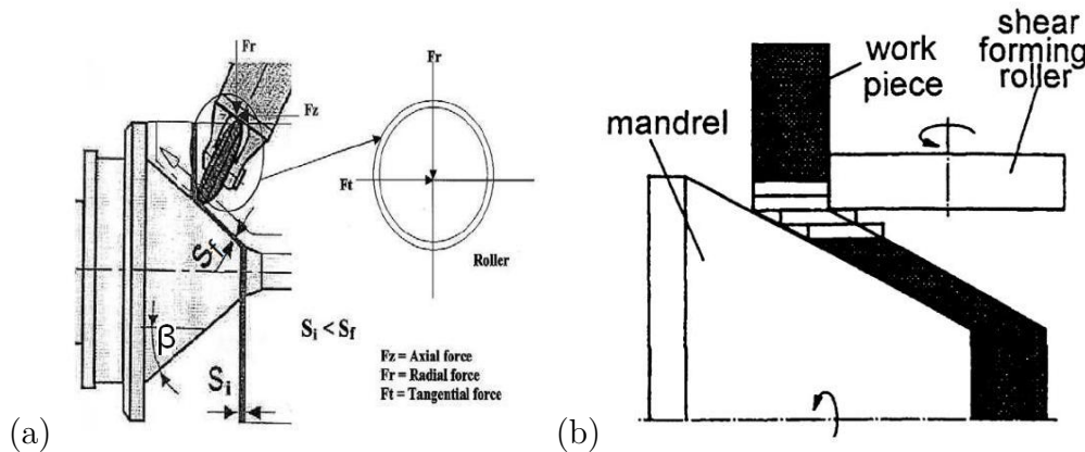
Fig. 1.2.3: Schéma du fluotournage conique montrant : (a) les outillages et l'épaisseur initiale et finale et (b) comment se déforme le flan d'après [Runge 97].
