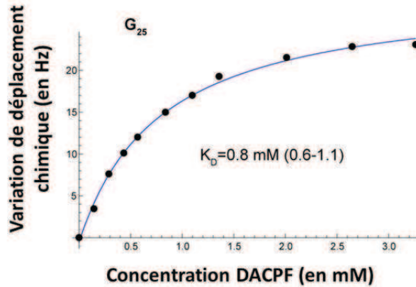
Figure S-161 Mesure de l'affinité du DACPF pour l'aptamère à la néomycine par RMN ^1\text{H} via la variation du déplacement chimique du proton imino de la bases \text{G}_{25} lors de l'augmentation de la concentration en DACPF.
