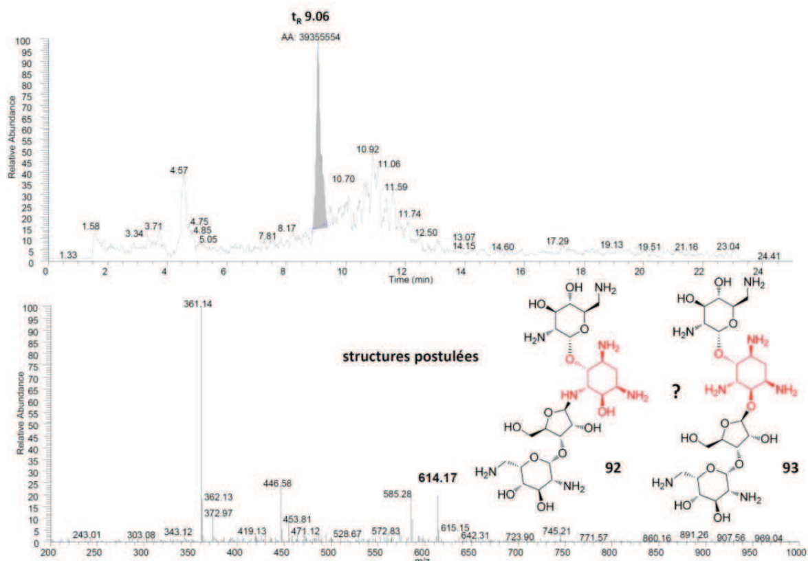
Figure III-108 Complémentation de \Delta neo6 avec le mutasython 90 (spectre de masse extrait à t_R = 9.06 min)
