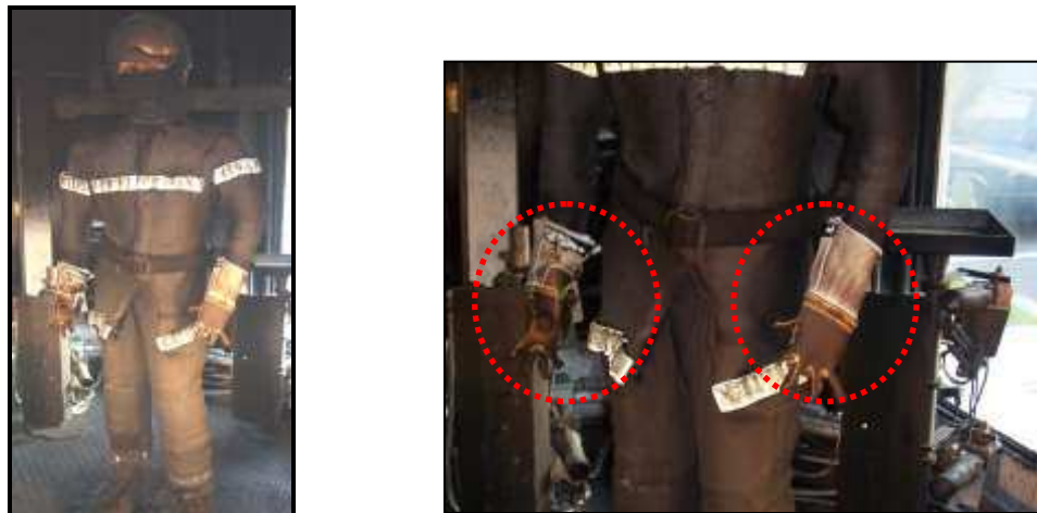
Figure 3.22 : Etat général de l'équipement E1 (Photo BSPP)
