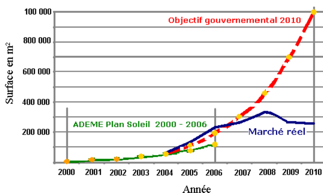
Figure I-16: Marché du capteur solaire en m 2 en France métropolitaine
