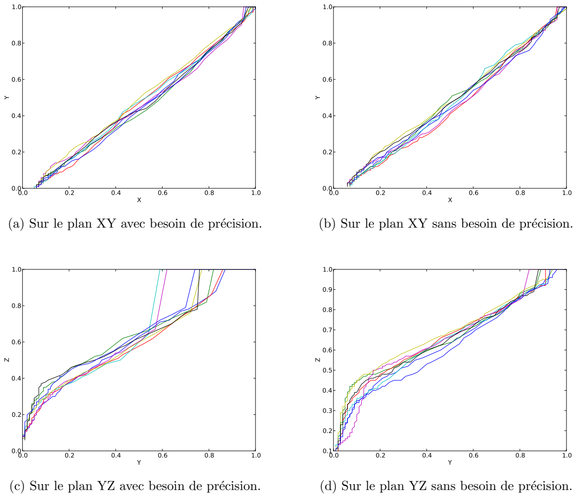
FIGURE 3.10 – Trajectoires 2-D des différents participants pour la technique Z-technique .
