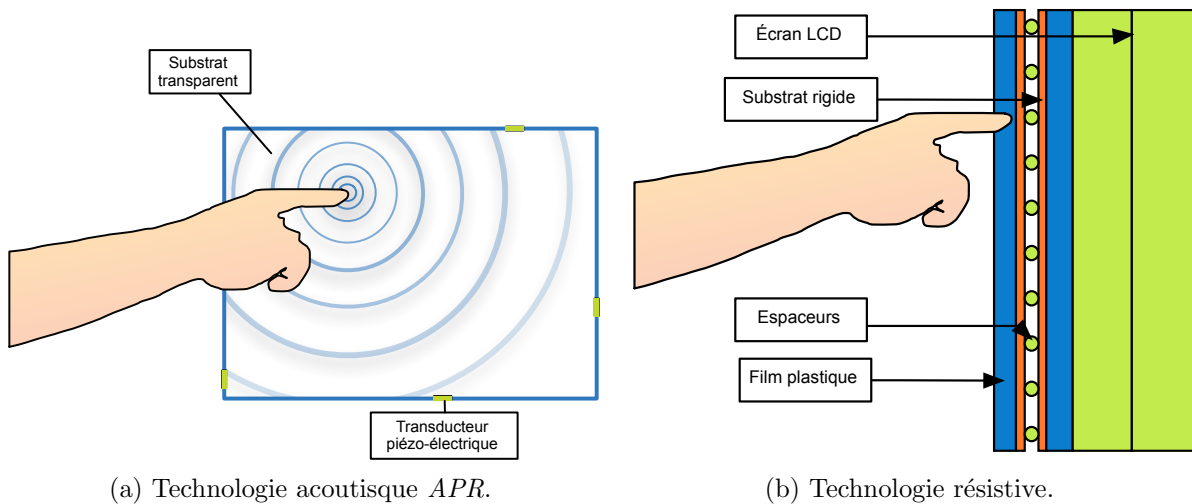
FIGURE 1.9 – Illustration de différentes technologies tactiles.
