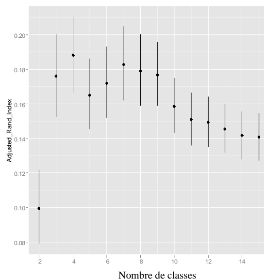
Figure 32. Moyenne de l'indice de Rand corrigé pour différents niveaux de coupure du dendrogramme
