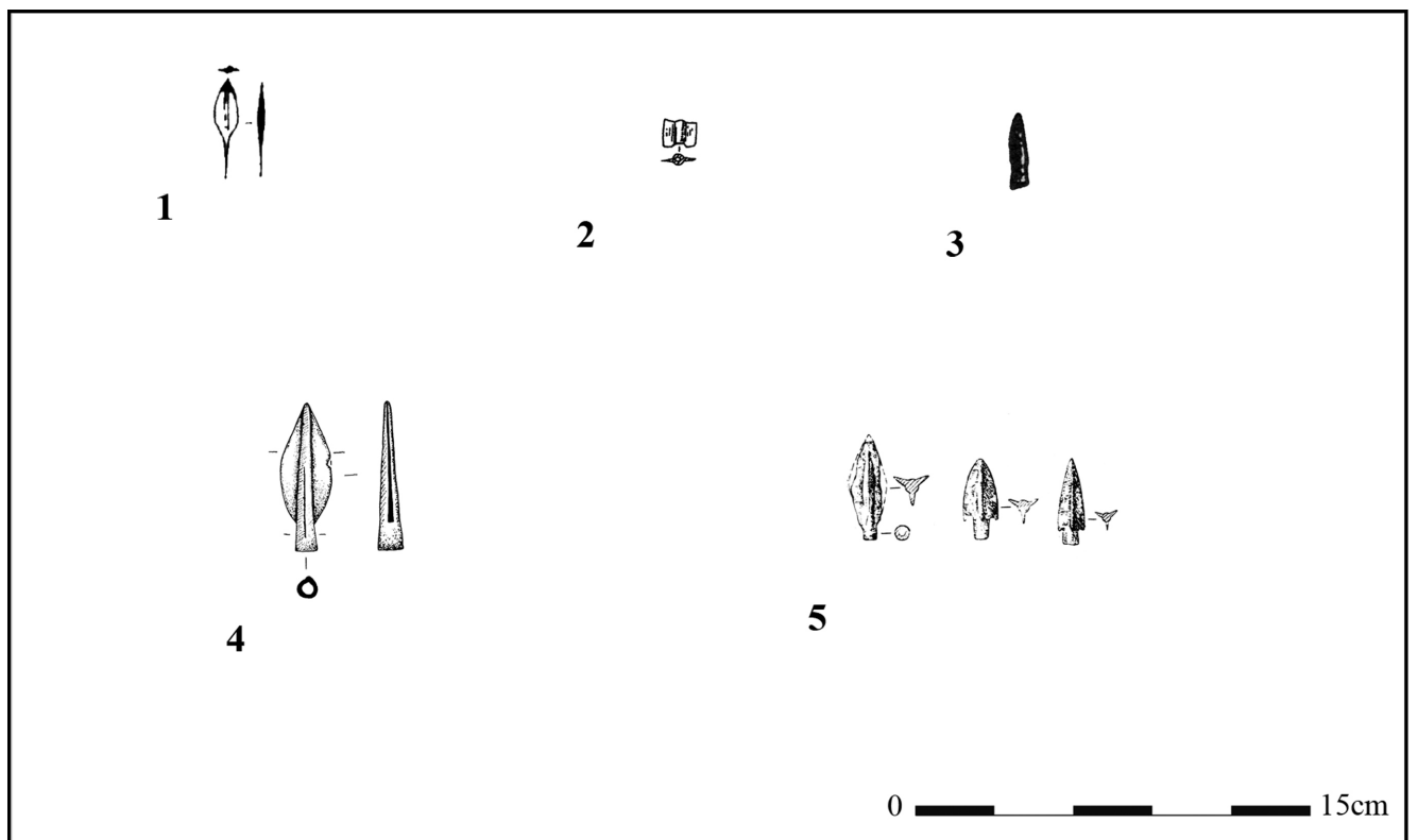
Figure 385 : Pointes de flèche. 1. Type 1. KANGURTTUT établissement : Vinogradova 2004a, p.145, fig.27, 14 ; 2. Type 2. RANNIJ-TULKHAR : s é p.n°45: Mandel'shtam 1968, p.149, fig.VIII, 7 ; 3. Type 3. DZHARKUTAN 4B : s é p.n°207 : Ionesov 1990d, p.264, fig.59, 18 ; 4. Type 4. DZHAM : Avanesova, Shajdullaev, Erkulov 2001, p.69, fig.4, 3; 5. Type 5. TAKHIRBAJ 3 (surface) : Sarianidi 1990, p.241, fig.XXVI, 14, 16-17.
