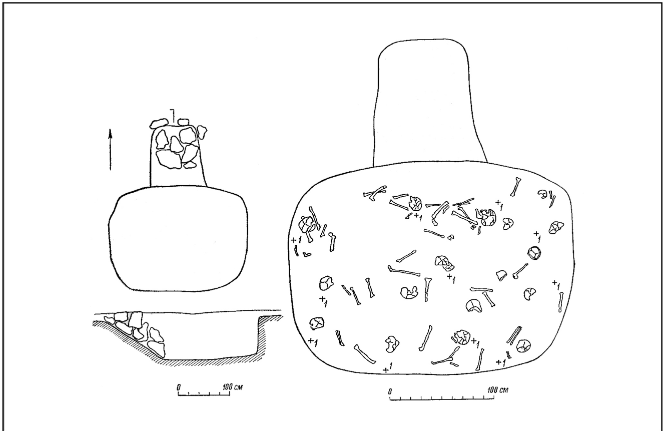
Figure 544 : Fosse avec rampe d'accès. RANNIJ-TULKHAR : sép.n°72 : Mandel'shtam 1968, p.46, fig.30. Légende: 1. fragments de coquilles d'oeufs.
