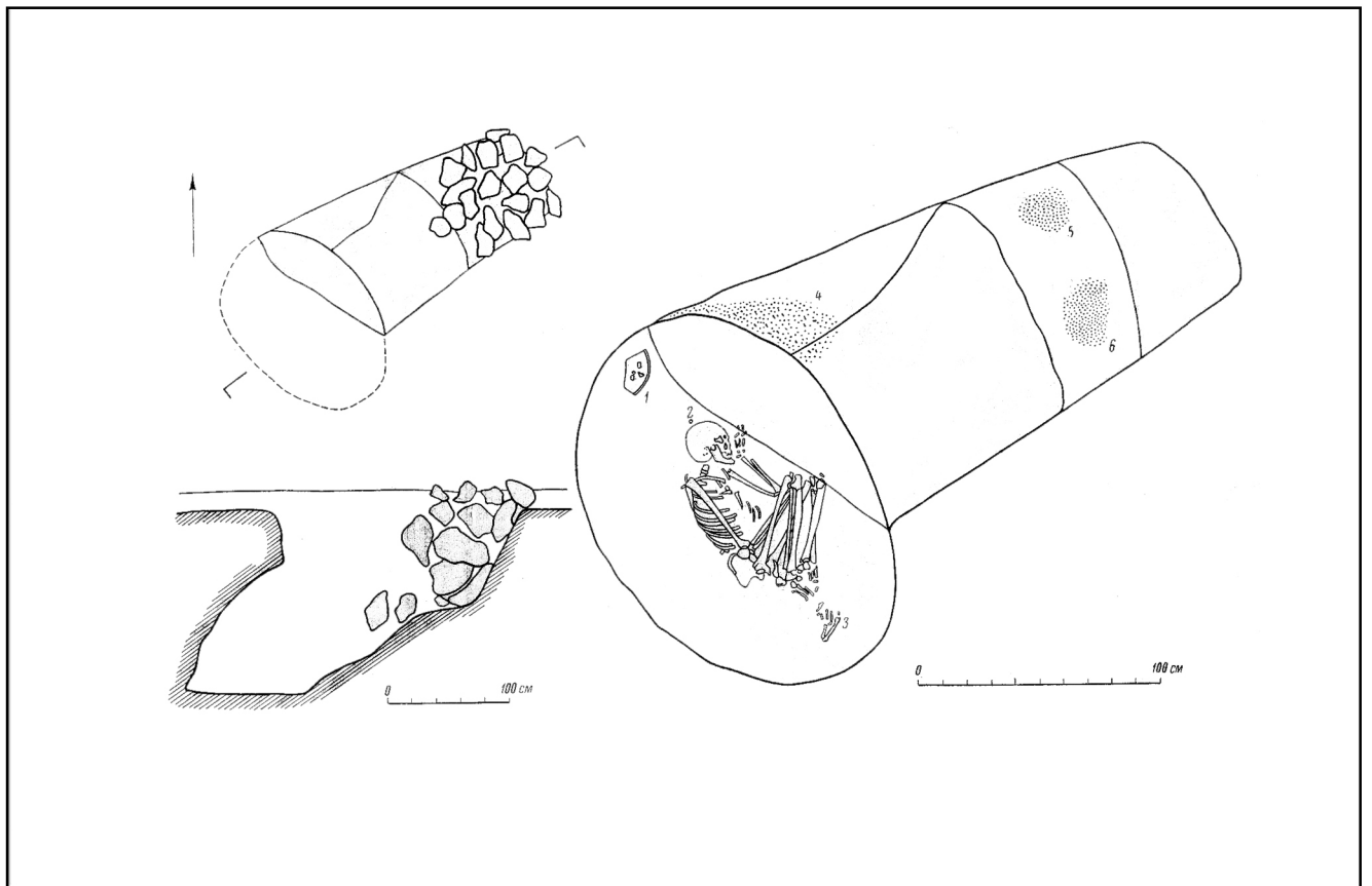
Figure 538 : Tombes à chambre funéraire. RANNIJ-TULKHAR : sép.n°1 : Mandel'shtam 1968, p.9, fig.1.
