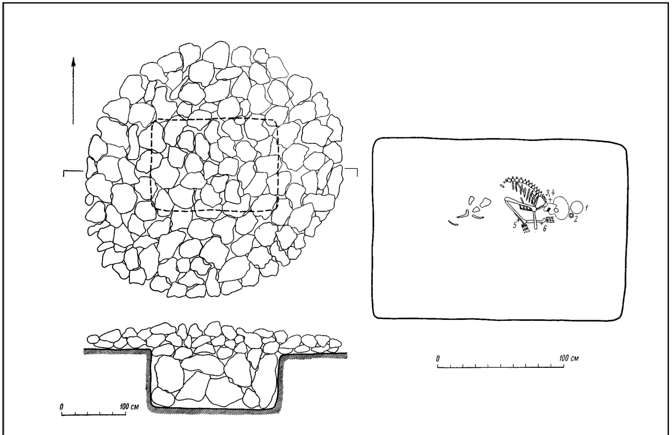
Figure 540 : Fosses. RANNIJ-ARUKTAU : sép.n°XIX, 1 : Mandel'shtam 1968, p.51, fig.34.
