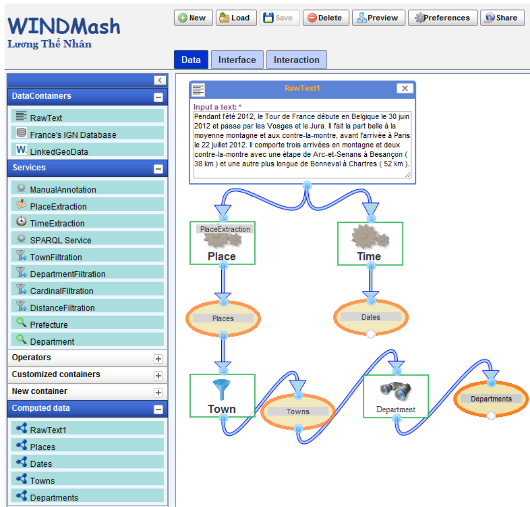
FIGURE 5.24 – Une solution envisageable de la phase Contenu lors de l'évaluation
