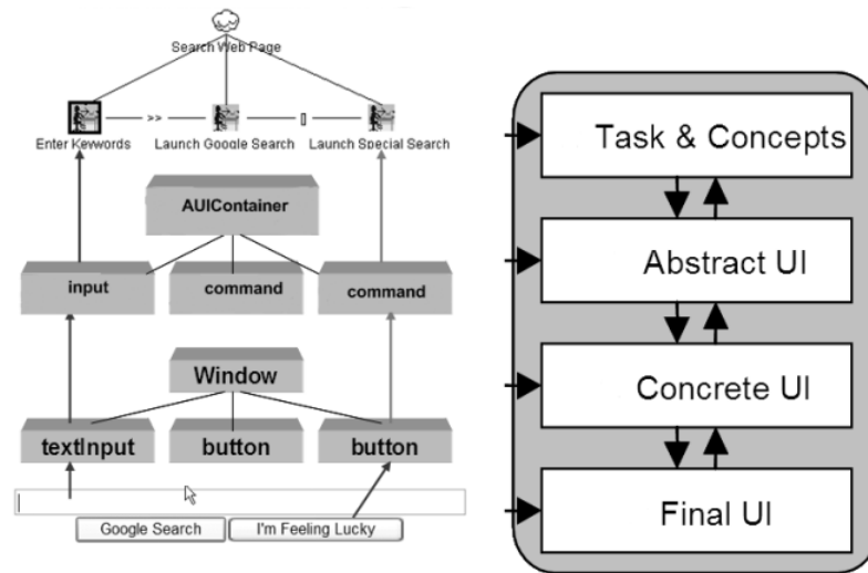
FIGURE 4.8 – Modélisation de l'interface utilisateur dans le projet Cameleon
