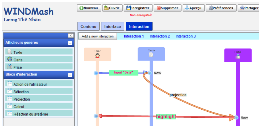
FIGURE 5.13 – Spécification du comportement 3 dans la phase Interaction pour le scénario
