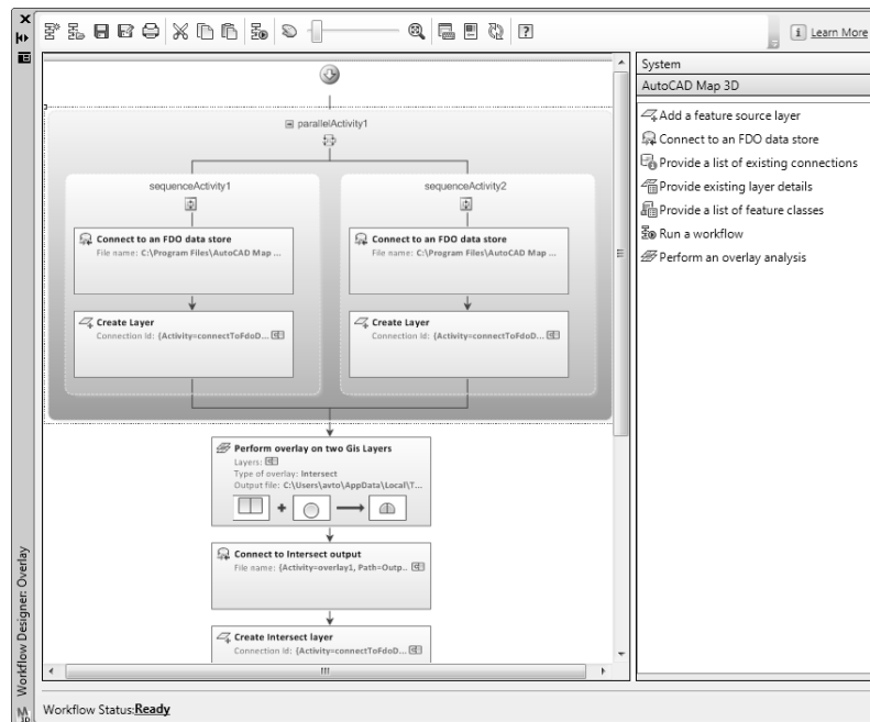
FIGURE 4.21 – Exemple de workflow élaboré sous AutoCAD Map 3D
