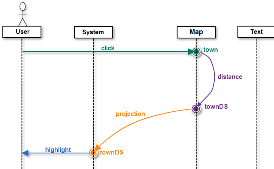
FIGURE 4.38 – Un autre exemple de spécification d’interaction multi-niveaux
