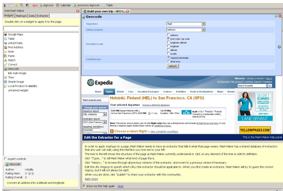
FIGURE 3.17 – MashMaker intégré dans le navigateur
