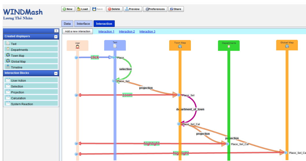
FIGURE 5.30 – Une solution envisageable de la phase Interaction lors de l'évaluation
