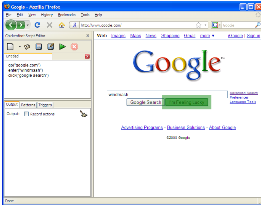
FIGURE 3.11 – Environnement de développement de Chickenfoot sous Firefox
