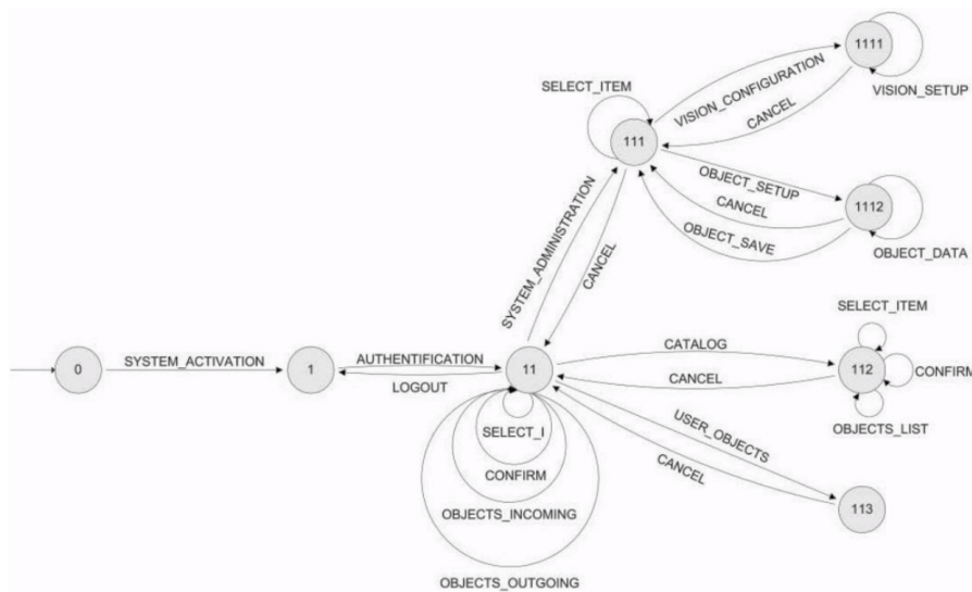
FIGURE 4.7 – Modélisation des dialogues d’une application avec HephaisTK [DLG+08]
