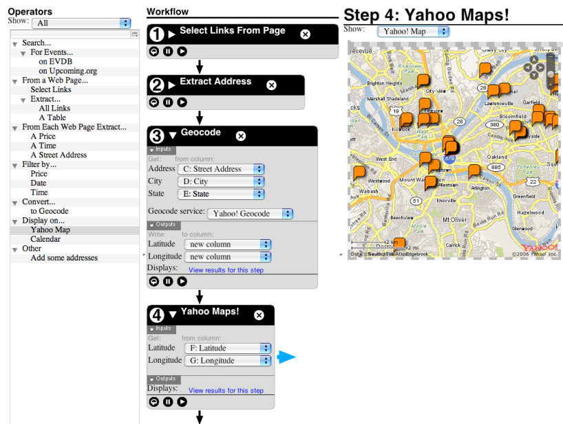
FIGURE 3.16 – Marmite, un outil de programmation de Mashups pour l'utilisateur final
