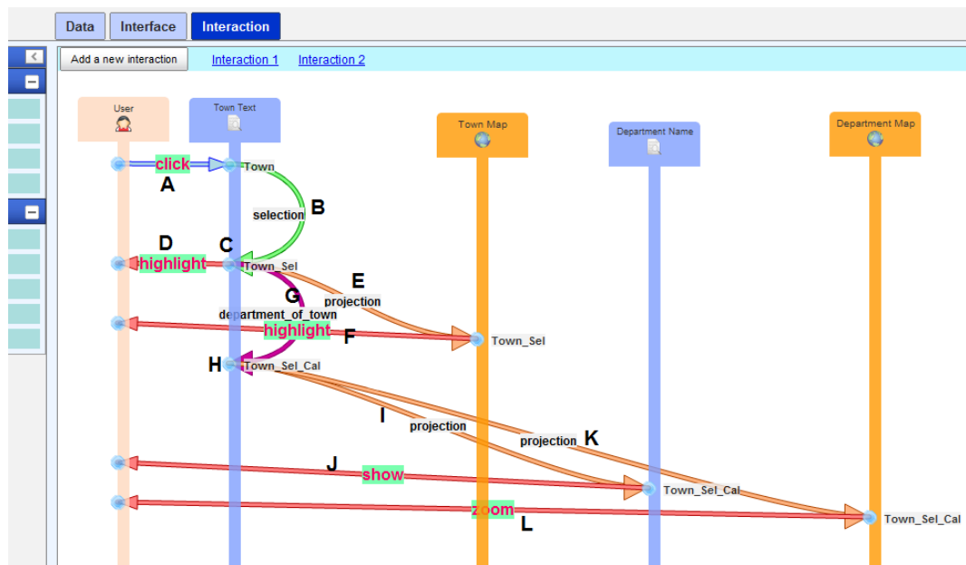
FIGURE 5.21 – Interaction conçue avec WINDMash
