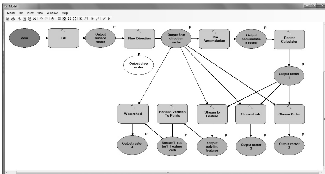
FIGURE 4.20 – Construction et affichage de données géographiques avec le Model Builder de ArcGIS
