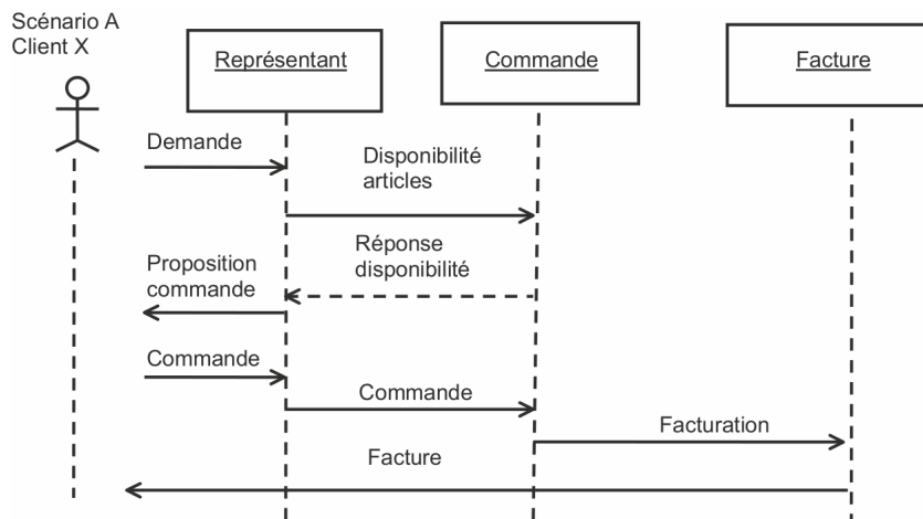
FIGURE 4.13 – Exemple de diagramme de séquence pour l'achat d'articles [GG08]
