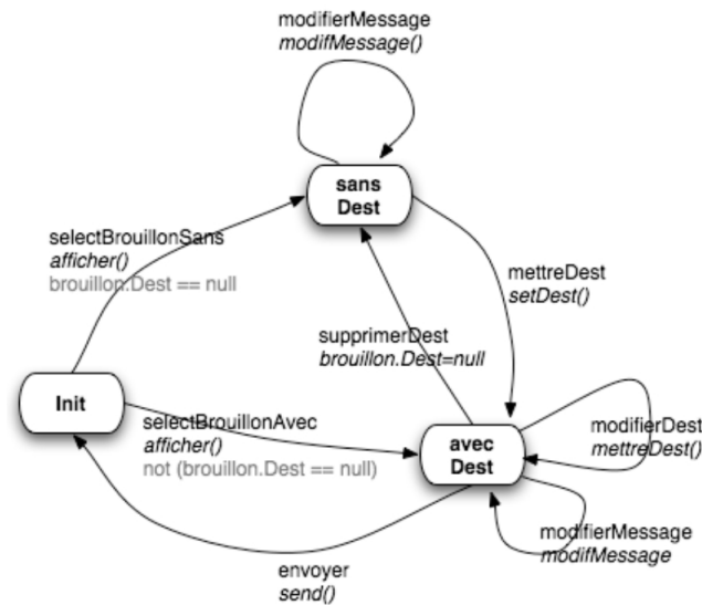
FIGURE 4.6 – Modélisation des dialogues avec un mailer via un automate [CGGS09]
