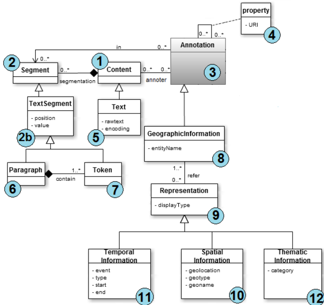
FIGURE 3.20 – Modèle conceptuel de la phase Contenu
