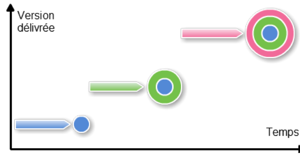
FIGURE C.2 – Modèle incrémental
