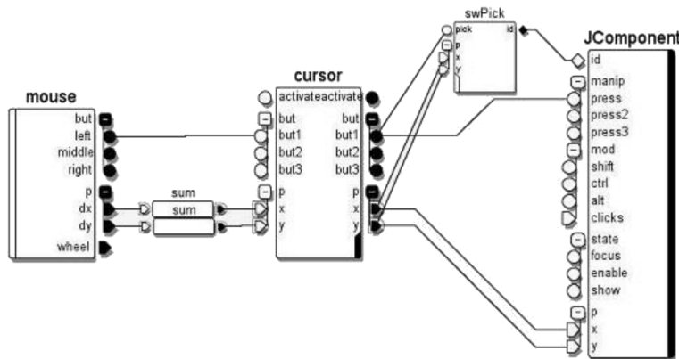
FIGURE 4.18 – Sélection d'un objet graphique modélisée via ICON [DF04]
