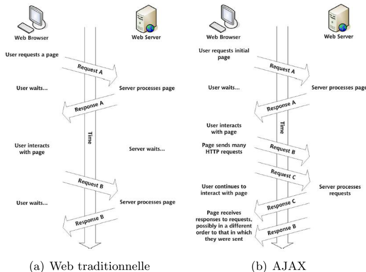
FIGURE D.1 – Comparaison entre une application Web traditionnelle (a) et AJAX (b)
