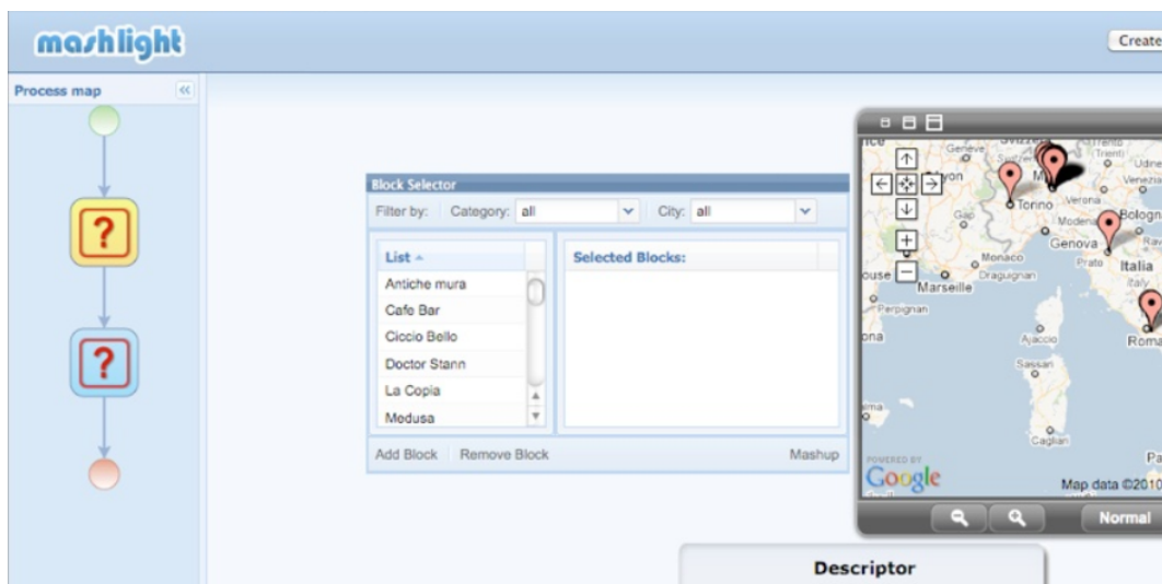
FIGURE 2.4 – Exemple de conception avec le mashup MashLight [BG10]
