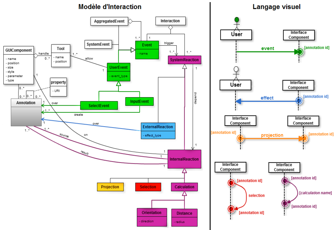
FIGURE 5.3 – Les cinq notions de base du langage de programmation visuel
