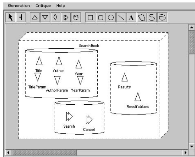
FIGURE 4.16 – Exemple de diagramme de présentation avec UML i [PdSP03]
