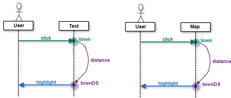
FIGURE 4.36 – Décomposition d’interactions définies à un niveau “système”
