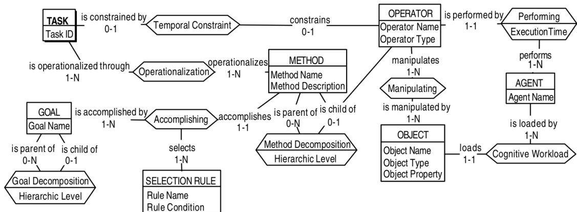
FIGURE 4.1 – Méta-modèle de GOMS [LPV01]
