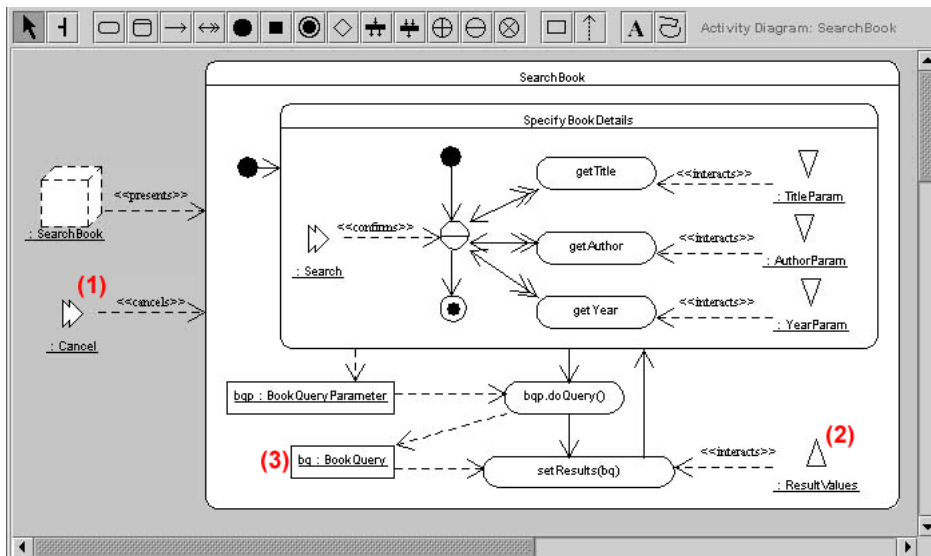
FIGURE 4.17 – Exemple de diagramme de dialogue avec UMLi [PdSP03]
