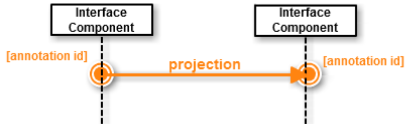
FIGURE 4.29 – Spécification de la projection (réaction interne du système)
