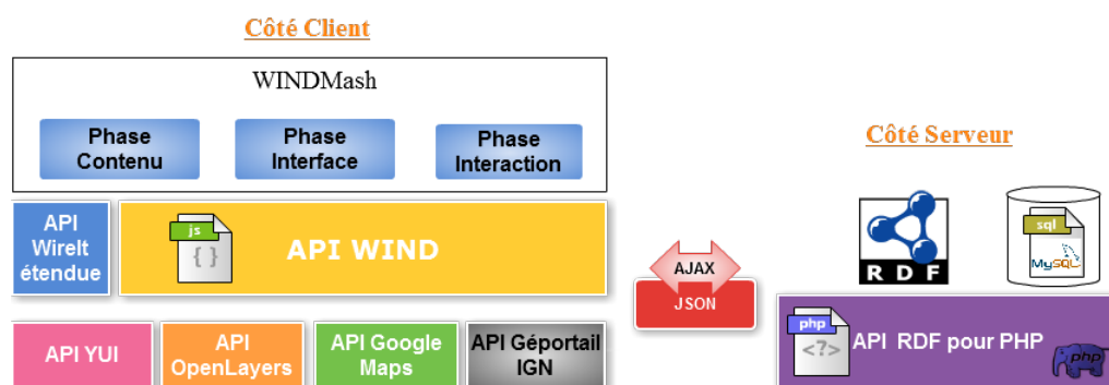
FIGURE F.2 – Technologies Web utilisées pour implémenter WINDMash
