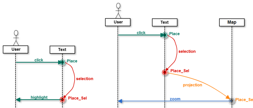
FIGURE 4.34 – Décomposition de l'interaction présentée sur la figure 4.33
