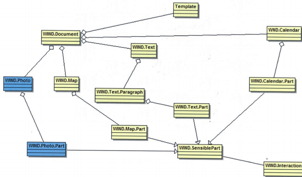
FIGURE 5.34 – Évolution de l'API WIND après le projet PIND
