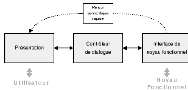
FIGURE 4.9 – Modèle de Seeheim [DF04]
