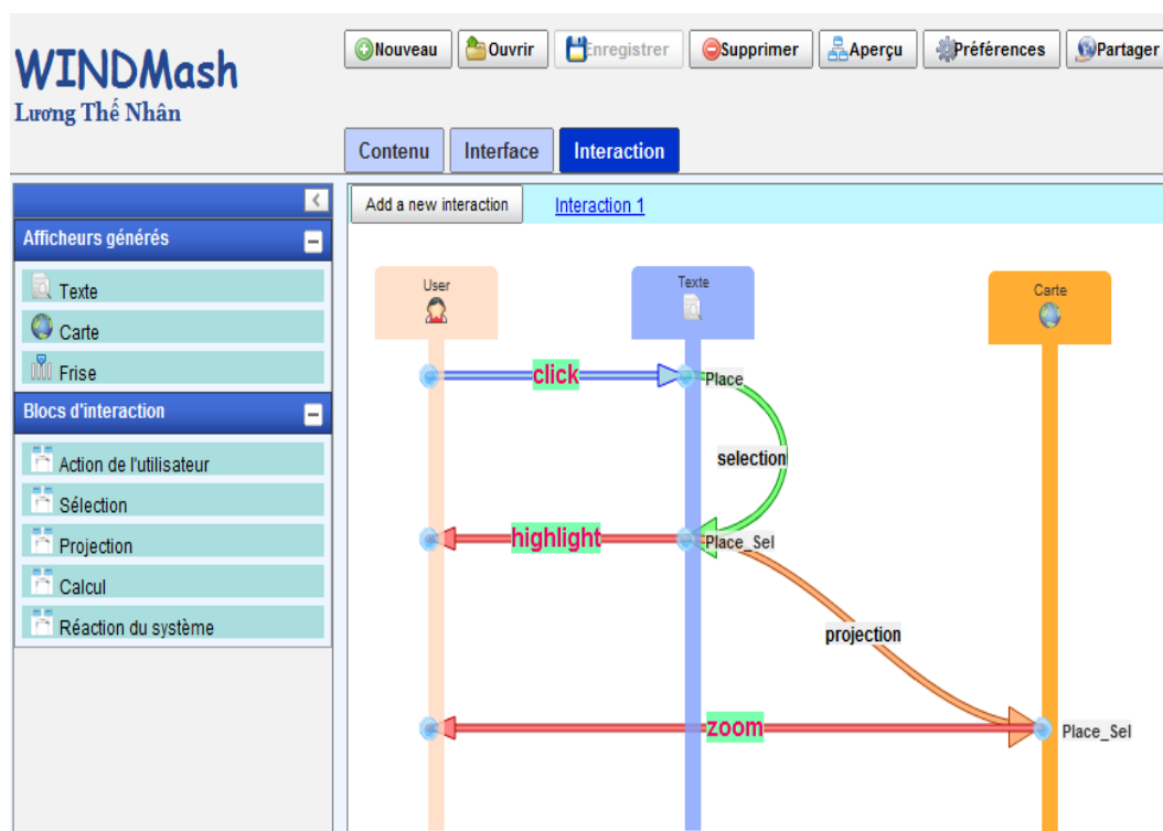
FIGURE 4.43 – Spécification graphique d’une interaction dans WINDMash
