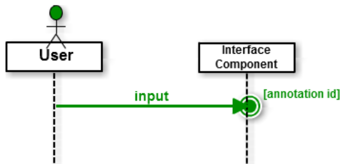
FIGURE 4.26 – Spécification d'une action de saisie de la part de l'utilisateur
