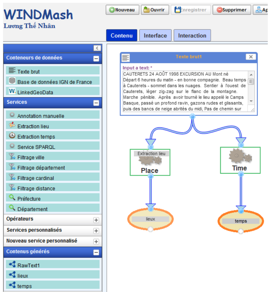
FIGURE 5.7 – Manipulation de la phase Contenu pour le scénario
