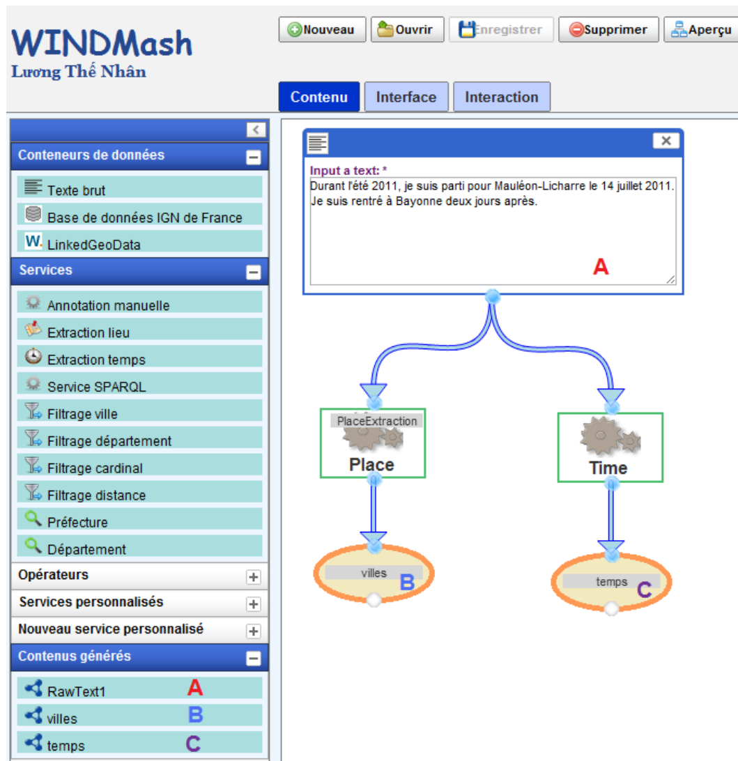
FIGURE 3.30 – Éditeur de flux de WINDMash (Phase Contenu )
