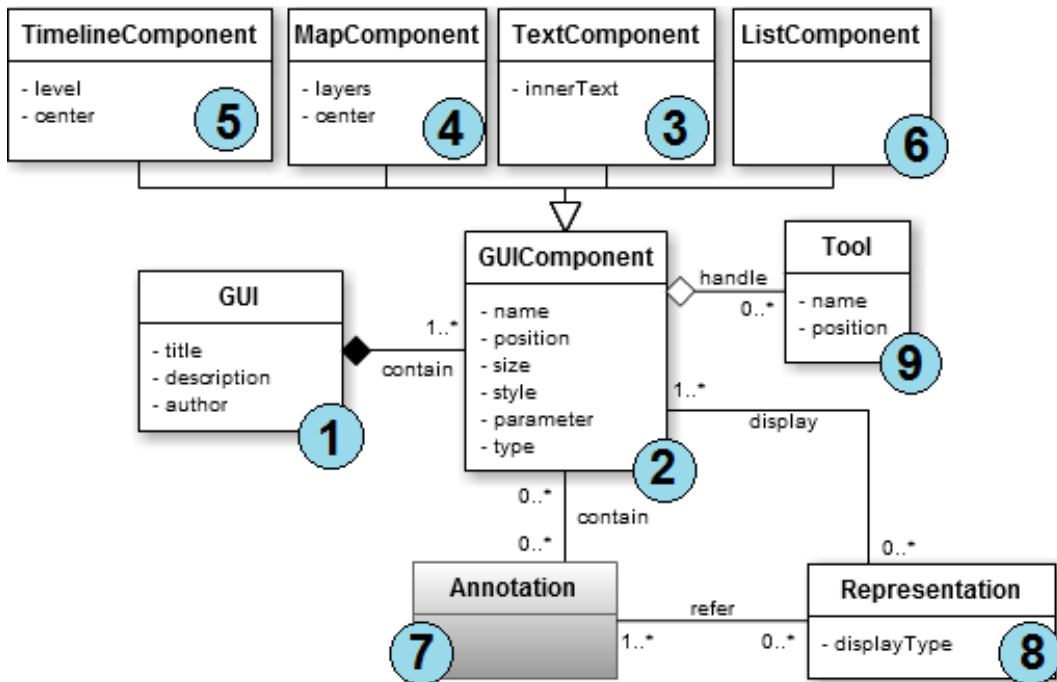
FIGURE 3.23 – Modèle conceptuel de la phase Interface
