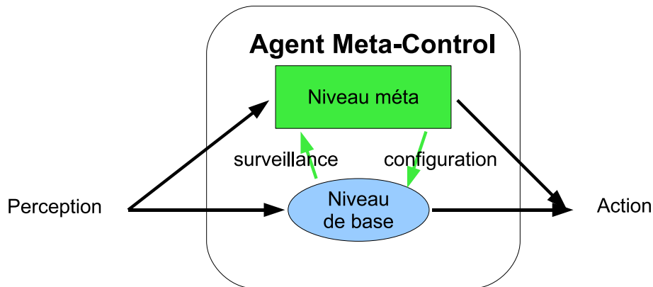
FIGURE 3.3 – Architecture META-CONTROL (vue simplifiée).
