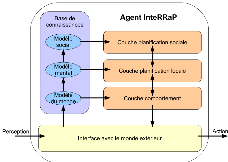
FIGURE 3.2 – Architecture hybride INTERRRAP (vue simplifiée).
