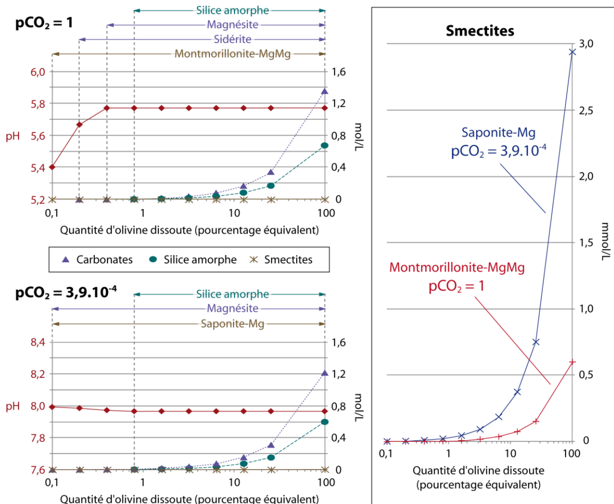
Figure 5-18 – Modélisation par le code CHESSE de l'évolution du pH et des minéraux secondaires précipités en fonction de la quantité d'olivine dissoute (exprimée en pourcentage de la quantité utilisée dans l'expérience) et en fonction de la pression partielle de dioxyde de carbone. Par souci de clarté, la magnésite et la sidérite sont regroupées au sein de la même courbe. L'axe des abscisses est en échelle logarithmique pour les trois diagrammes.
