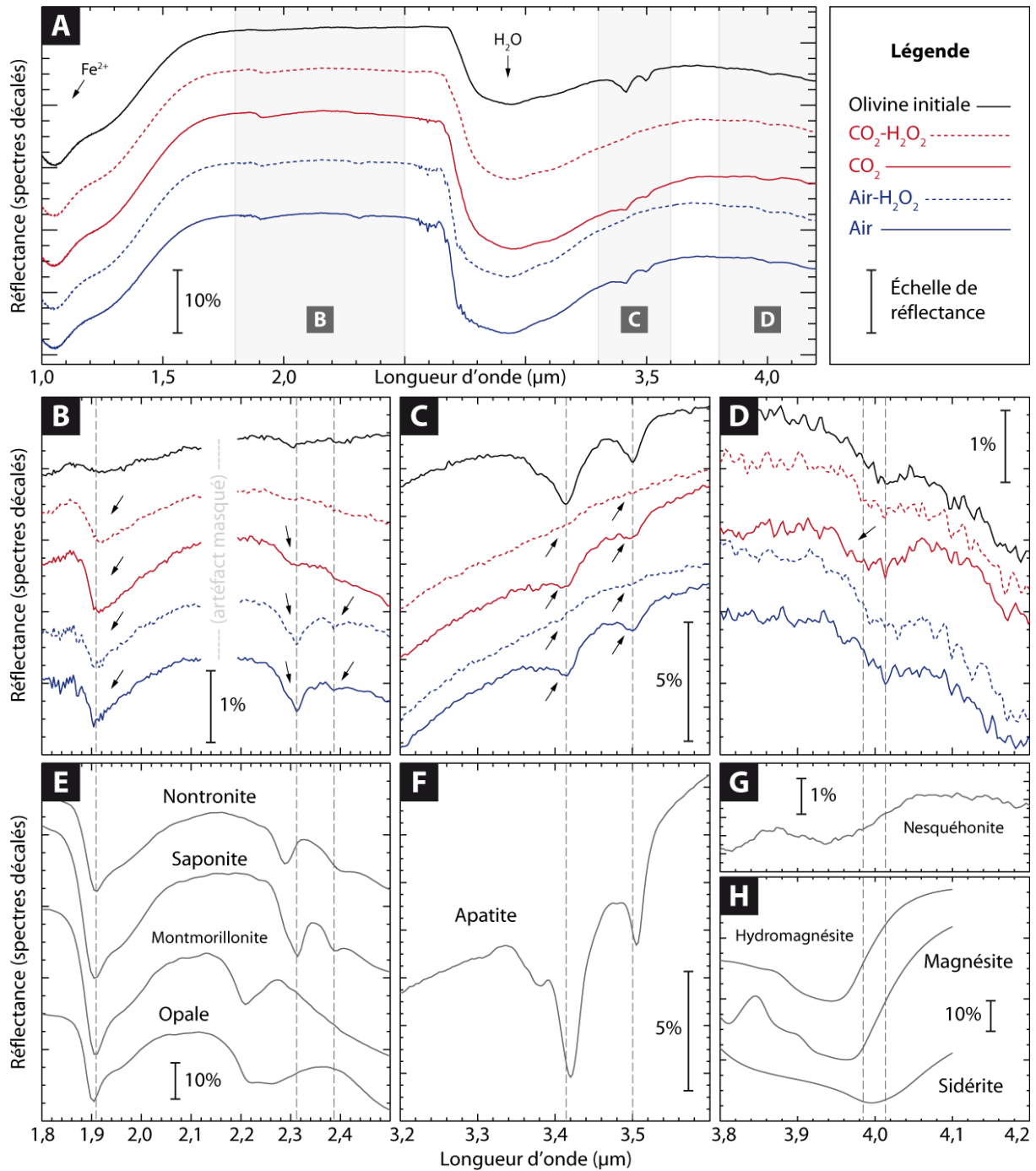
Figure 5-7 – Spectres FTIR de l’olivine initiale et des échantillons altérés, et comparaisons avec des spectres de référence. A : présentation générale des spectres sur la gamme 1,0-4,2 μm. B : zoom sur la gamme 1,8-2,5 μm. C : zoom sur la gamme 3,2-3,6 μm. D : zoom sur la gamme 3,8-4,2 μm. Les flèches en B, C et D indiquent des modifications entre l’olivine initiale et les échantillons altérés. E : spectres de minéraux argileux et d’opale extraits de la librairie USGS [Clark et al. , 2007] (nontronite NG-1a, saponite SapCa-1 et montmorillonite CM20 ; opale TM8896-hyalite). F : spectre d’apatite extrait de la librairie CRISM (échantillon LAAP03). G : spectre d’un échantillon naturel de carbonates de magnésium hydratés, à nesquehonite dominante [Dehouck et al. , 2012]. H : spectres de minéraux carbonatés extraits de la librairie USGS (hydromagnésite LACB28A, magnésite LACB03A et sidérite LACB08A).
