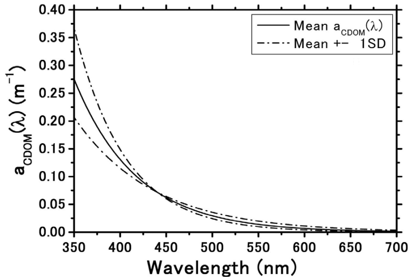
Figure I-4 : Spectre moyen d'absorption du CDOM ( a_{CDOM} ) mesuré dans l'Océan Arctique Ouest (d'après Matsuoka et al., 2011). Valeur moyenne (ligne continue), \pm écart type (ligne discontinue).
