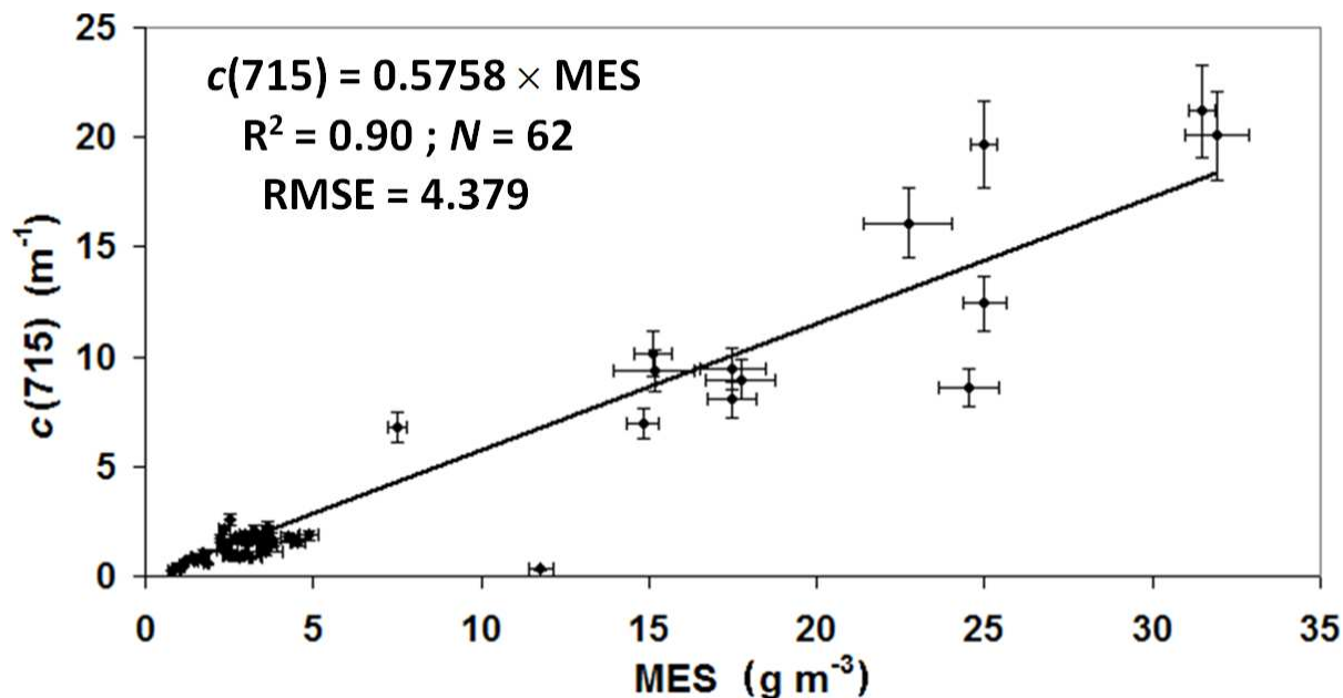
Figure III-28 : Relation entre c(715) en m^{-1} fonction de la concentration en MES en g\ m^{-3} . La régression linéaire entre ces deux paramètres est reportée sur le graphique. Les barres d'erreurs horizontales et verticales sont les déviations standard des concentrations en MES et de c(715) .
