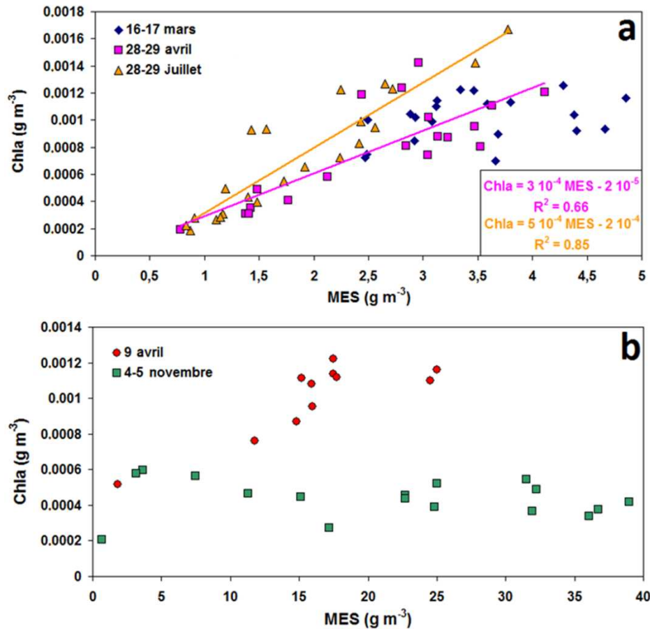
Figure III-8 : Concentration en Chla ( \text{g m}^{-3} ) en fonction de la concentration en MES ( \text{g m}^{-3} ) en 2010 durant a) les trois épisodes hors crue : 16-17 mars, 28-29 avril ( \text{Chla} = 3 \cdot 10^{-4} \text{MES} - 2 \cdot 10^{-5} ; R^2 = 0.66 ) et 28-29 juillet ( \text{Chla} = 5 \cdot 10^{-4} \text{MES} - 2 \cdot 10^{-4} ; R^2 = 0.85 ); b) les deux épisodes de crues : 9 avril et 4-5 novembre.
