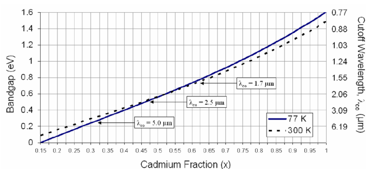
FIGURE 4.4 – Evolution de la longueur d'onde de coupure du détecteur \lambda_{co} avec le rapport de mélange x (fraction de cadmium par rapport au mercure). Tennant et al. (2008).
