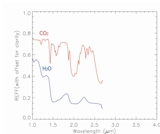
FIGURE 2.16 – Spectres de réflectance de glaces sur Mars d'après les données OMEGA (Mars Express). En rouge : spectre de la glace de CO_2 ; en bleu : spectre de la glace d' H_2O .
