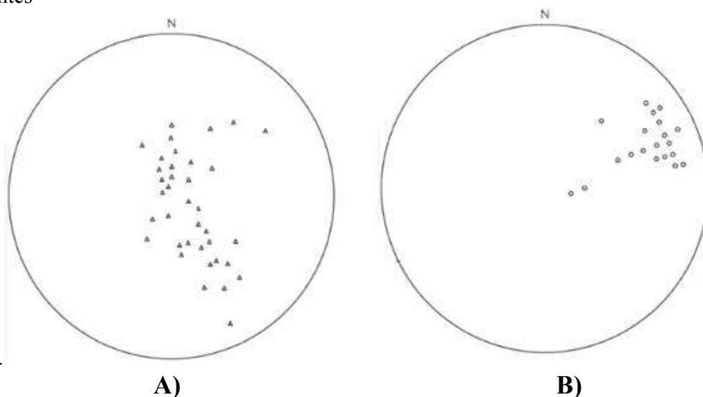
Figure II.8 : Projection dans un diagramme stéréographique (Wulf, hém. inf.) des mesures de foliations (A) et de linéations d'allongement (B) de l'unité orientale
