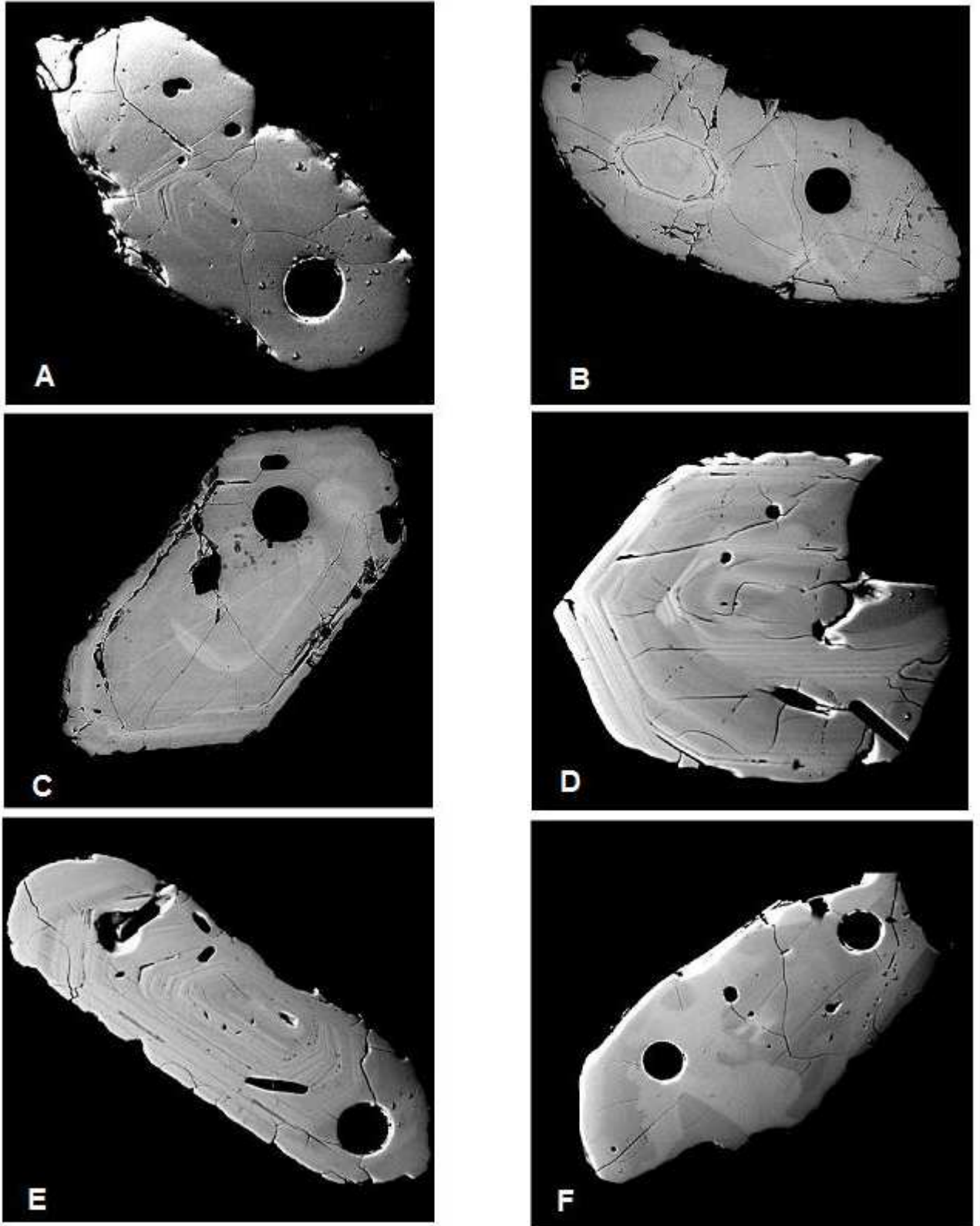
Figure V.3 : Images de microscopie électronique à balayage (MEB) des grains de zircon de deux échantillons de l'unité orientale : (A,B,C) orthogneiss 08PC07 et (D,E,F) granite 08PC11. La taille des cratères d'ablation est de 26 \mu m.
