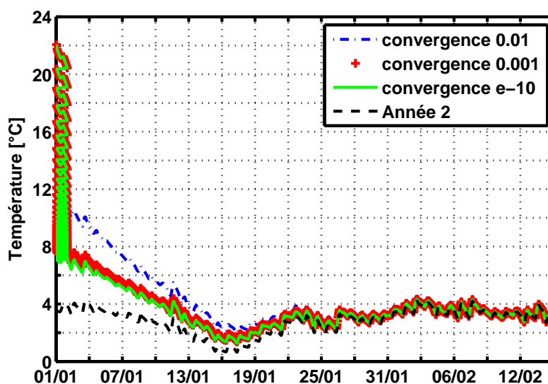
Figure 3.7 – Comparaison de résultats de température d’air du RDC avec différentes valeurs de convergences
