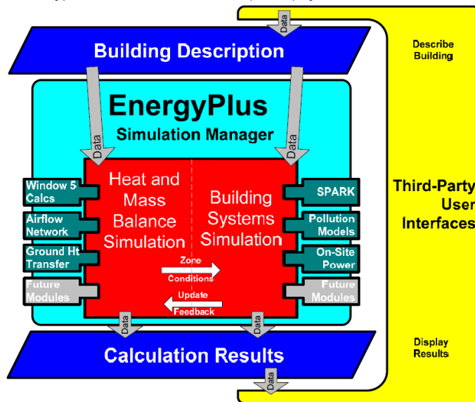
Figure 3.2 – EnergyPlus (extrait du manuel d'utilisateur d'EnergyPlus [4])
