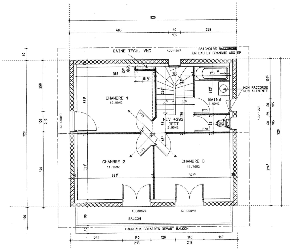
Figure 38 – Plan de l'étage de la maison I-BB
