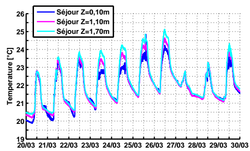
(b) Gradient du 20 au 30 mars 2011
