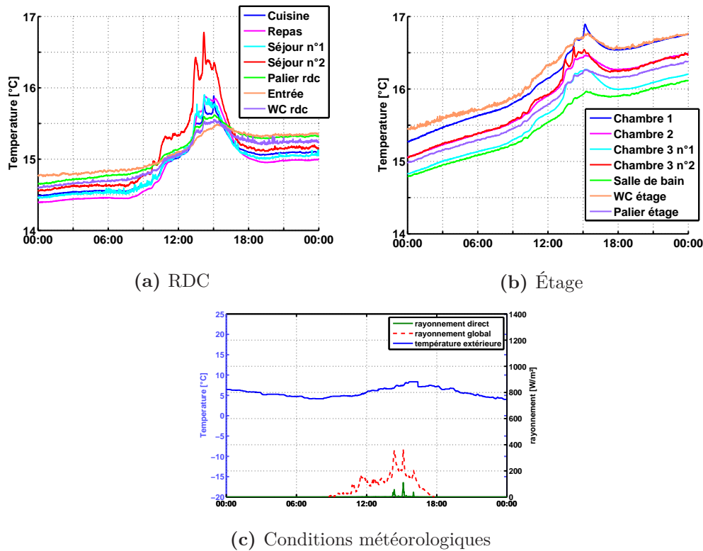
Figure 2.29 – Température d'air sèche dans la maison I-DM pour le 15 février 2011
