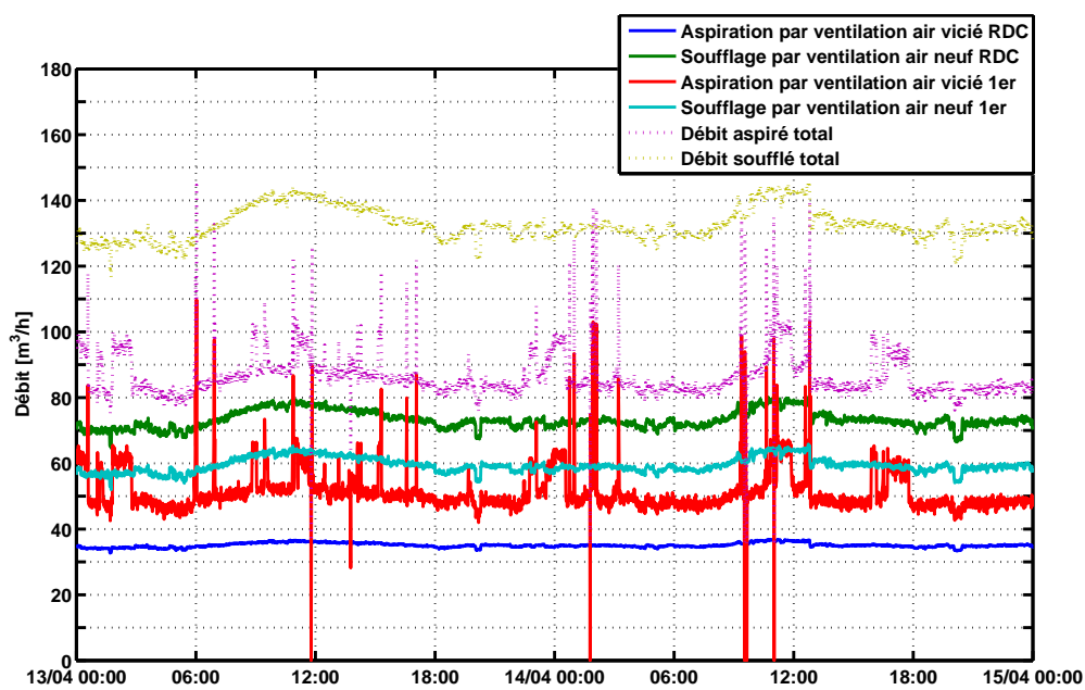
Figure 2.25 – Mesure du débit pour la maison I-DM le 13 et 14 avril
