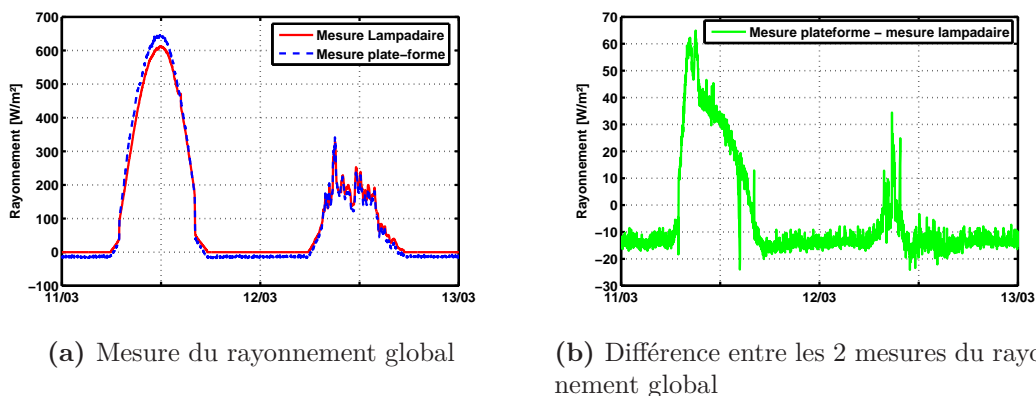
Figure 2.10 – Mesure du rayonnement global pour le 11 et 12 mars 2011 à l'INES
