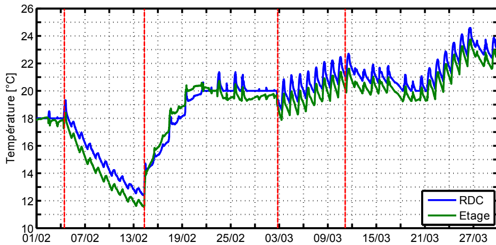
(a) Température d'air RDC et étage
