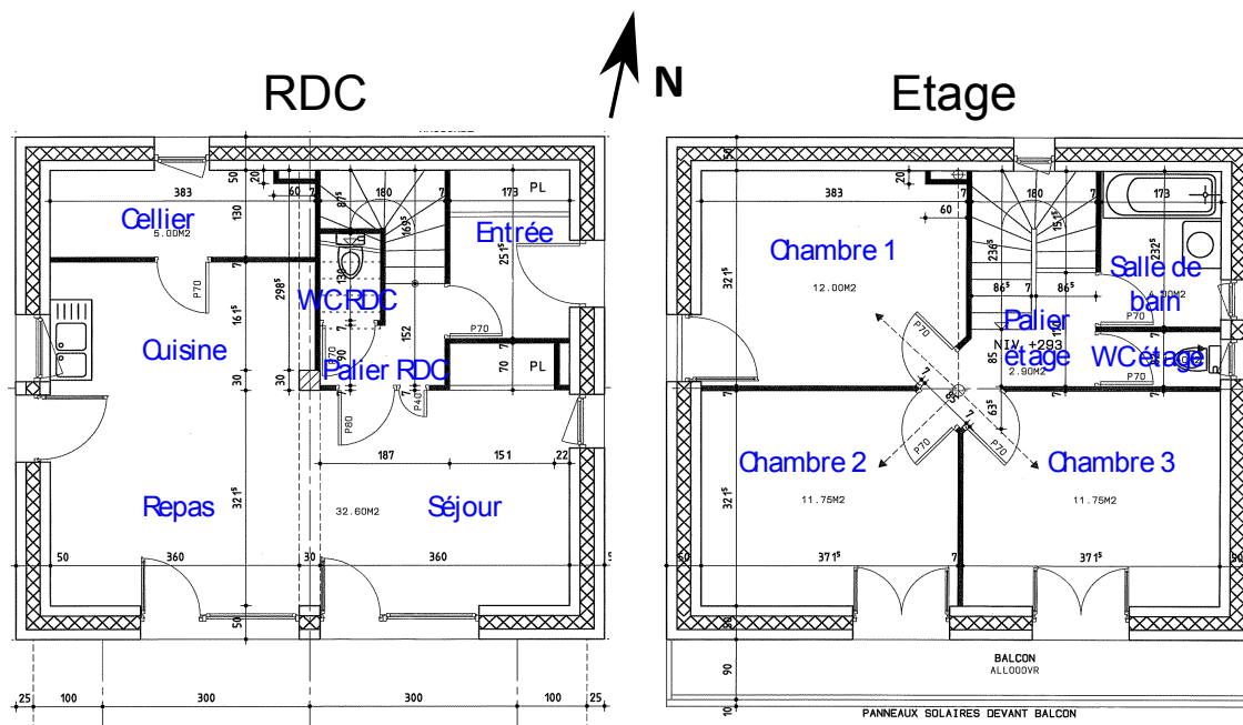
Figure 2.3 – Plan du RDC et de l'étage de la maison expérimentale I-DM
