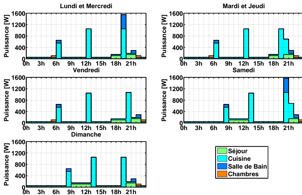
Figure 4.2 – Scénario de dégagement des charges internes dues à l'électroménager
