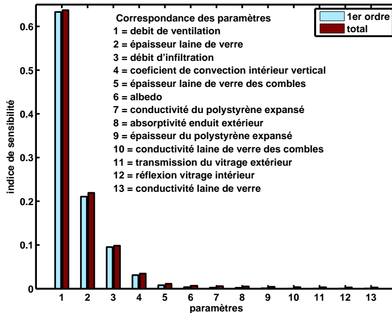
Figure 4.21 – Résultat de l’analyse de sensibilité globale pour le besoin de chauffage pour la maison RT 2005
