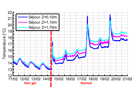
(a) Gradient du 11 au 21 février 2011
