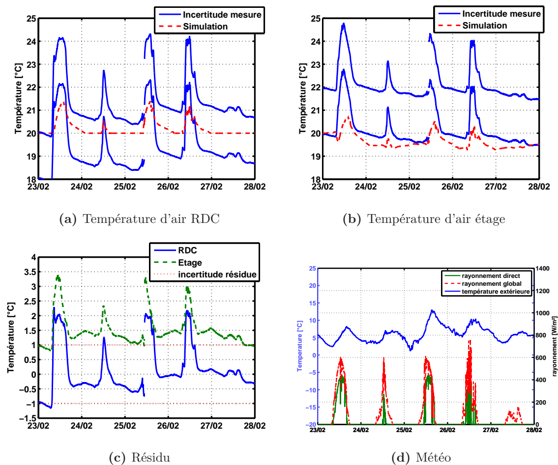
Figure 3.15 – Comparaison entre la simulation et une plage d'incertitude de la mesure de la température d'air du RDC et de l'étage, résidu du RDC et de l'étage et conditions météorologiques pour la maison I-DM du 23 au 28 février 2011
