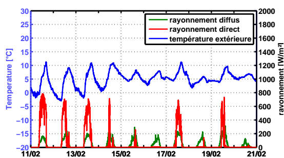
(c) Météo du 11 au 21 février 2011
