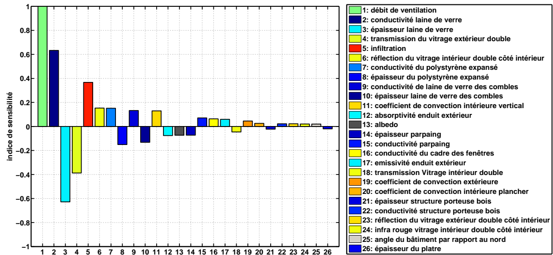
Figure 4.10 – Résultat de l'analyse de sensibilité locale pour le besoin de chauffage pour la maison RT2005
