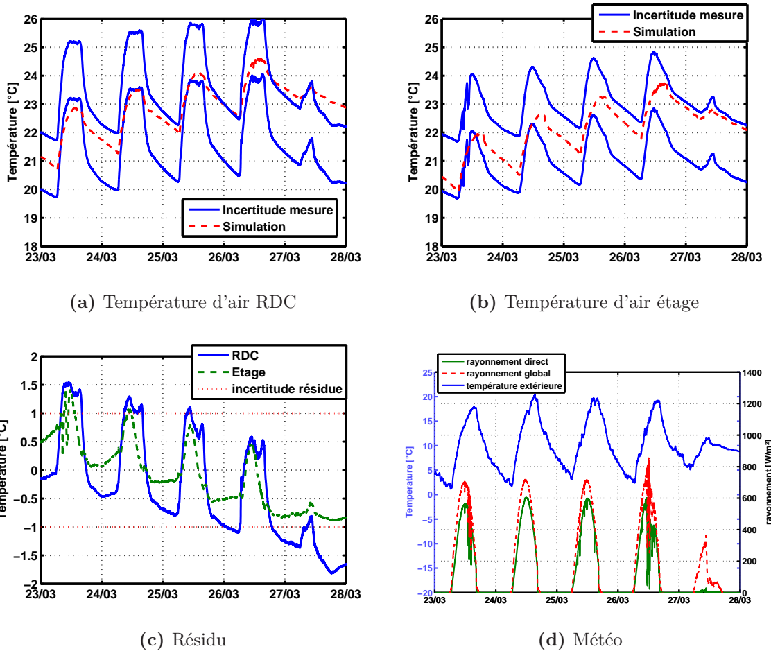
Figure 3.16 – Comparaison entre la simulation et une plage d’incertitude de la mesure de la température d’air du RDC et de l’étage, résidu du RDC et de l’étage et conditions météorologiques pour la maison I-DM du 23 au 28 mars 2011
