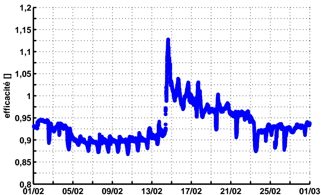
Figure 2.22 – Efficacité de l'échangeur
