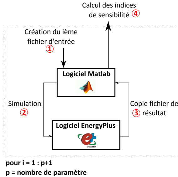
Figure 4.6 – Étape pour obtenir les résultats de l'analyse de sensibilité locale
