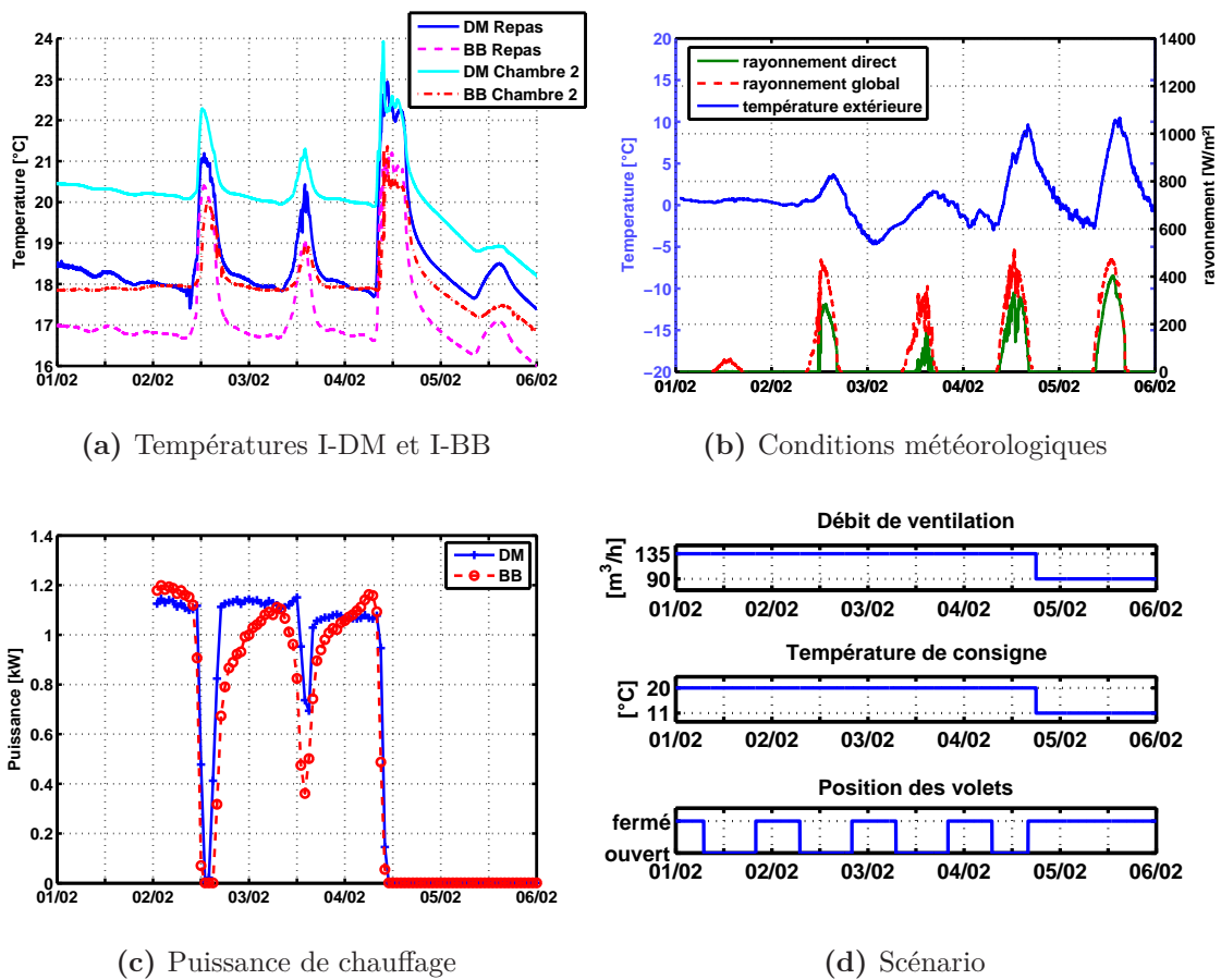
Figure 2.15 – Température d’air et puissance de chauffage dans les maisons I-DM et I-BB, météo et scénario du 1 er au 5 février
