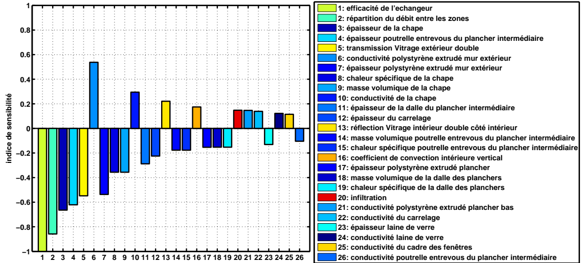
Figure 4.9 – Résultat de l'analyse de sensibilité locale pour le besoin de chauffage pour la maison I-BB
