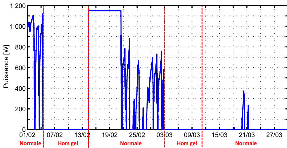
(b) Puissance de chauffage
