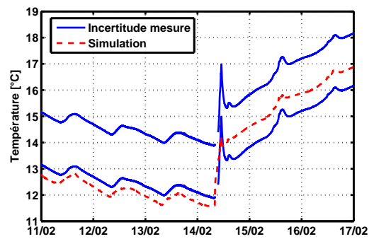
(b) Température d'air étage
