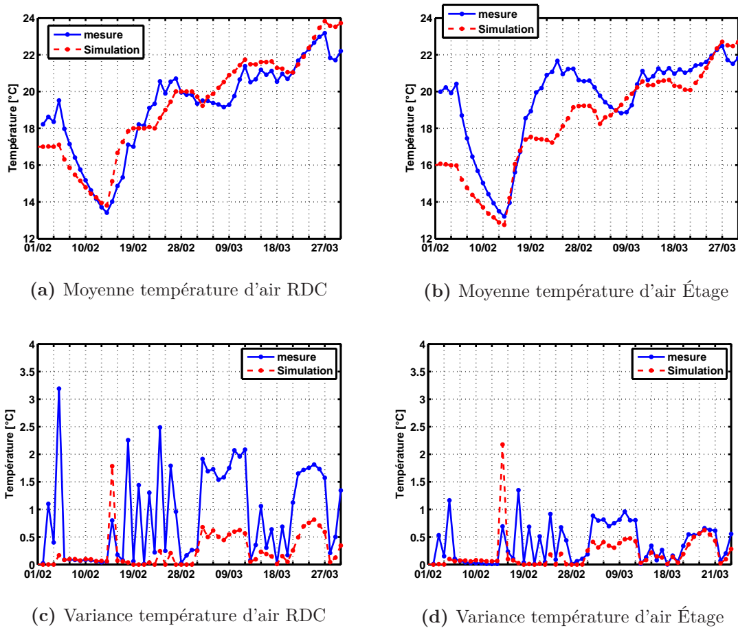
Figure 3.18 – Comparaison entre la simulation et la mesure pour la moyenne et la variance journalière des températures d'air du RDC et de l'étage pour la maison I-BB
