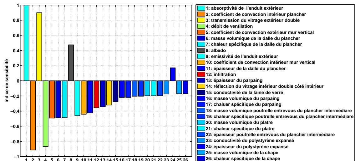
Figure 4.13 – Résultat de l’analyse de sensibilité locale pour le confort d’été pour le rez de chaussé pour la maison RT2005
