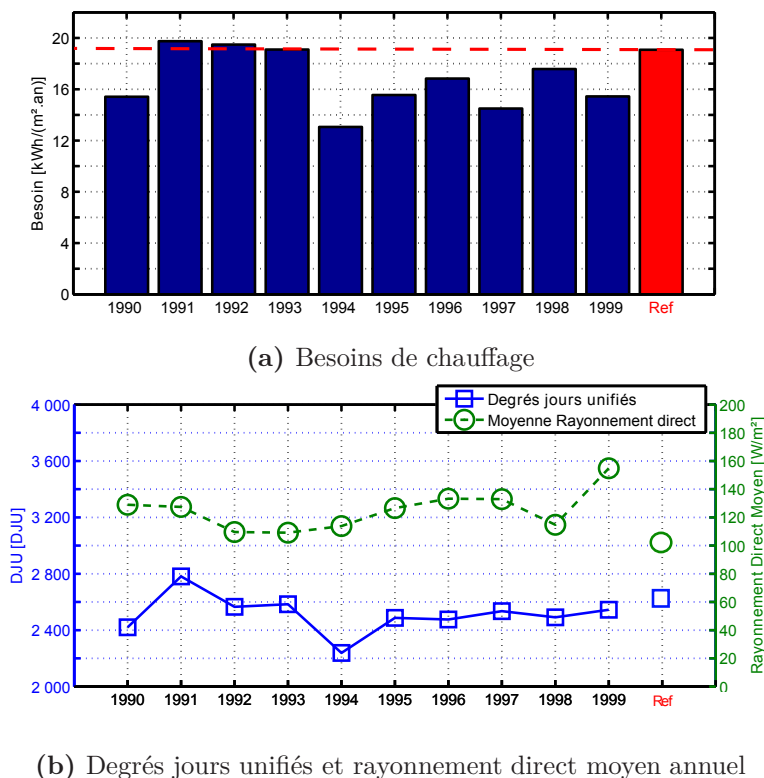
Figure 1.3 – Besoins de chauffage, degrés jours unifiés et rayonnement direct moyen annuel pour les années de 1990 à 1999 et pour la référence de la maison I-DM du climat de Genève
