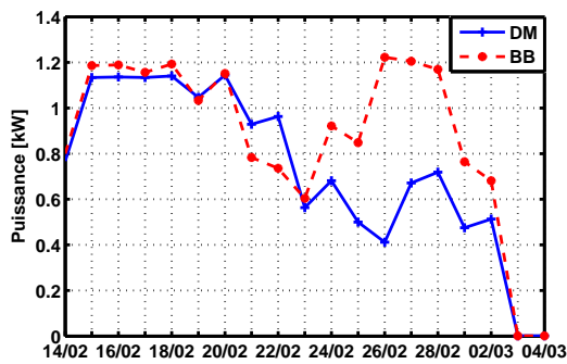
(c) Puissance de chauffage
