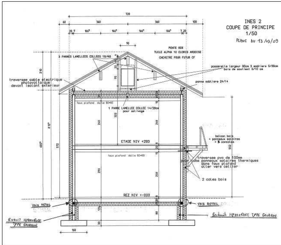
Figure 36 – Coupe de principe de la maison I-BB
