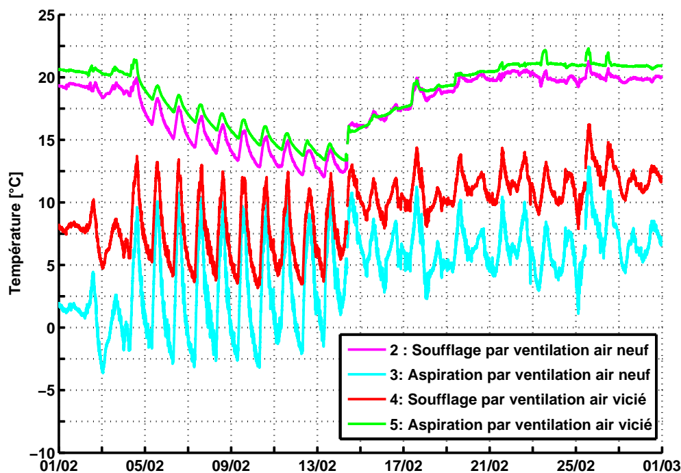
Figure 2.21 – Température d'air aux extrémités de l'échangeur pour le mois de février 2011
