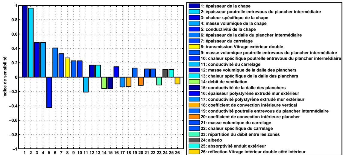
Figure 4.11 – Résultat de l’analyse de sensibilité locale pour le confort d’été pour le rez de chaussé pour la maison I-DM
