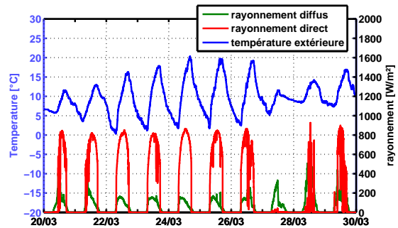
(d) Météo du 20 au 30 mars 2011
