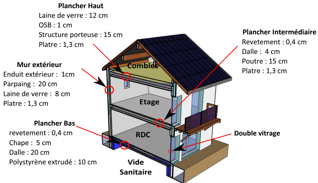
Figure 4.1 – Enveloppe de la maison RT 2005
