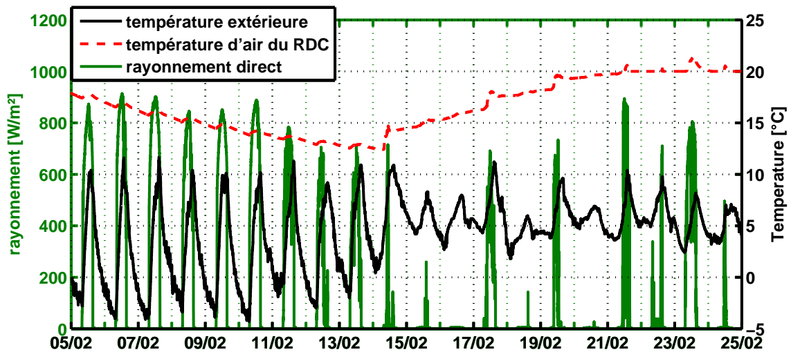
(a) Période 1 : du 5 au 25 février 2011
