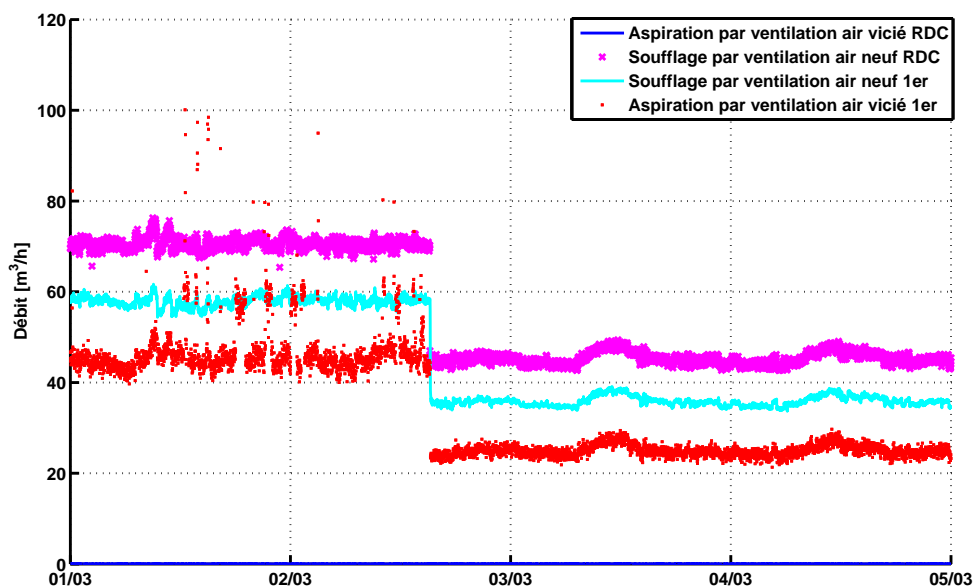
Figure 2.24 – Mesure du débit pour la maison I-DM du 1 er au 4 mars
