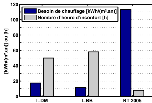
Figure 4.4 – Résultats de simulations pour les 3 maisons étudiées : besoin de chauffage et nombre d'heure d'inconfort
