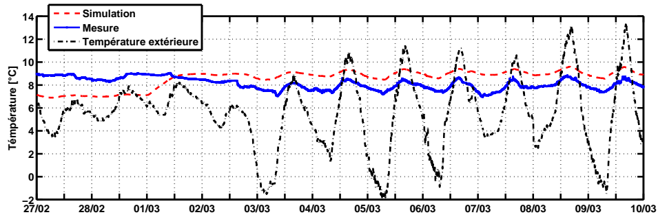
(a) Température vide sanitaire mesure et simulation
