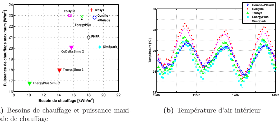
Figure 1.4 – Besoins de chauffage, puissance maximale de chauffage et température d'air intérieur pour trois jours en été avec six outils de simulation appliqués au cas de la maison I-DM (Source : A. Brun et al (2009) [9])
