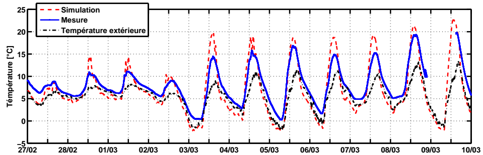
(a) Température des combles mesure et simulation
