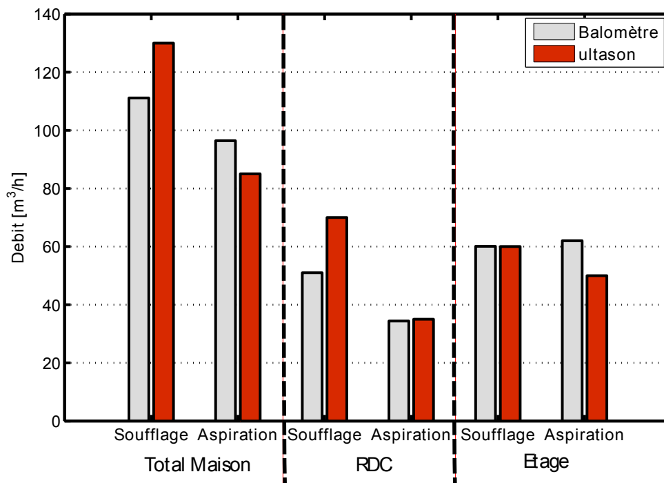
Figure 2.26 – Comparaison des mesures de débit par le balomètre et le débitmètre à ultrason
