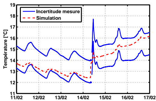
(a) Température d'air RDC
