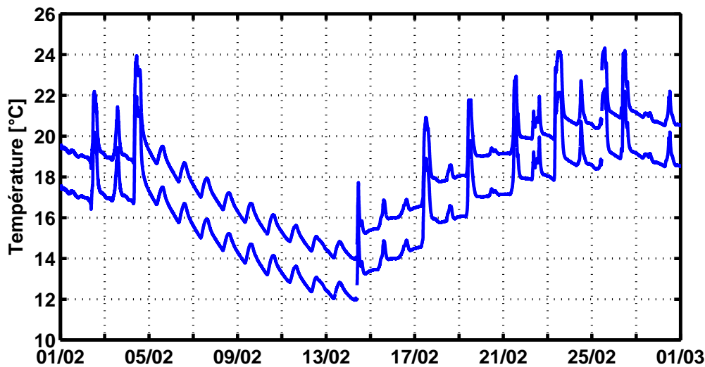
Figure 2.31 – Plage de température pour le niveau du RDC de la maison I-DM
