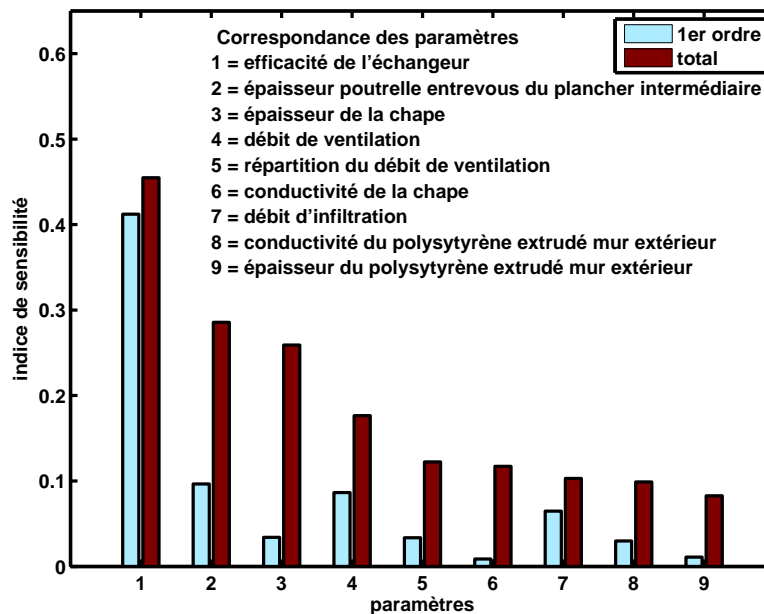
Figure 4.22 – Résultat de l'analyse de sensibilité globale pour le besoin de chauffage pour la maison I-BB en considérant neuf paramètres influents
