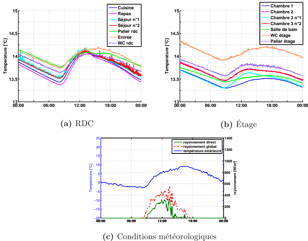
Figure 2.28 – Température d'air sèche dans la maison I-DM pour le 12 février 2011
