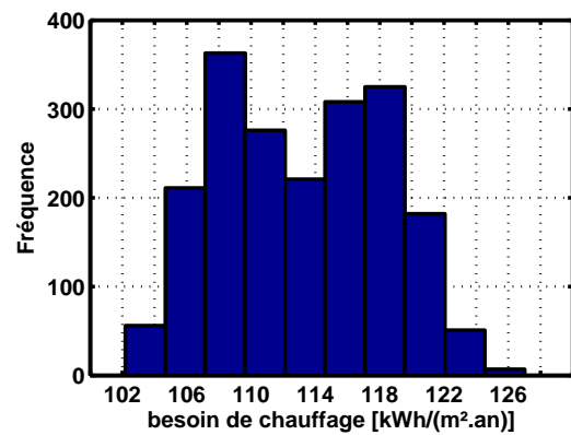
(c) Maison RT 2005
