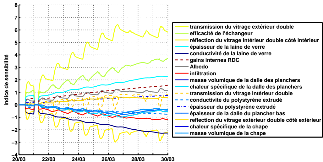
Figure 4.25 – Résultat de l'analyse de sensibilité locale pour la maison I-DM pour la température d'air du RDC du 20 au 30 mars 2011
