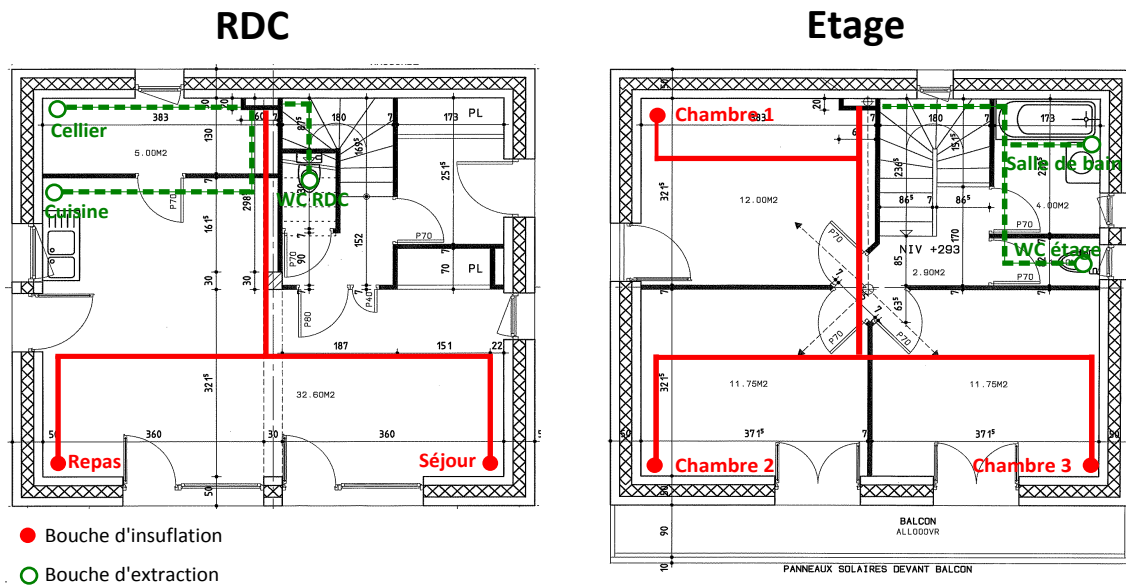
Figure 2.19 – Réseau de ventilation
