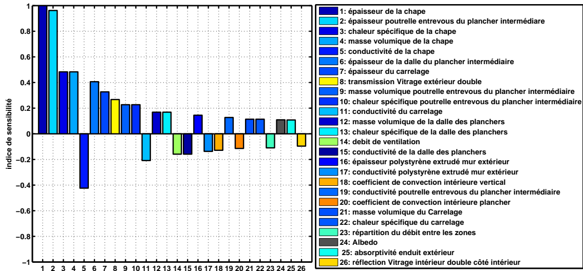
Figure 4.12 – Résultat de l’analyse de sensibilité locale pour le confort d’été pour le rez de chaussé pour la maison I-BB
