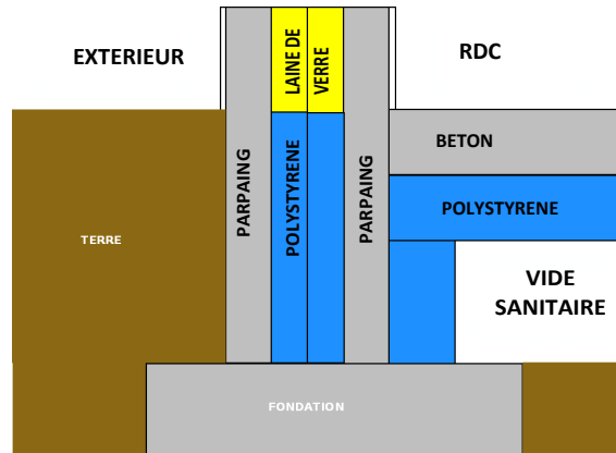
Figure 2.4 – Liaison plancher bas mur extérieur de la maison I-DM
