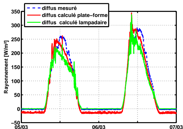
Figure 2.11 – Rayonnement diffus mesuré et calculé à l'aide des deux pyranomètres disponible sur le site pour le 5 et 6 mars 2011
