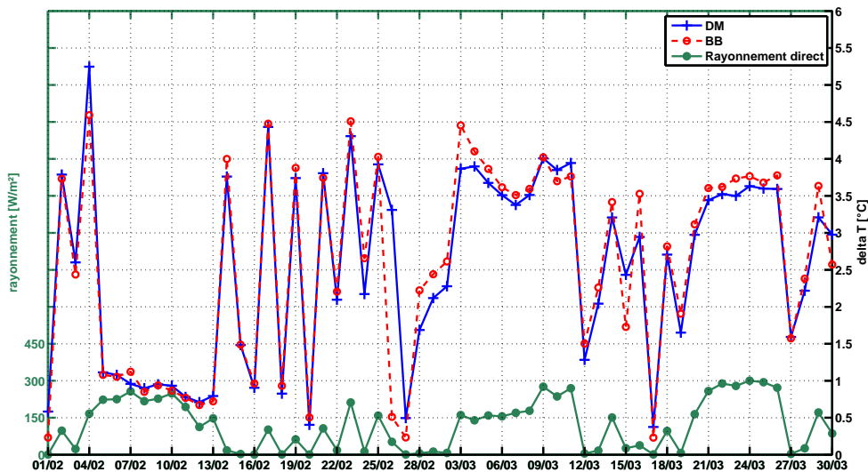
Figure 2.18 – Différence de température journalière des maisons I-DM et I-BB pour le RDC et rayonnement direct journalier du 1 er février au 30 mars
