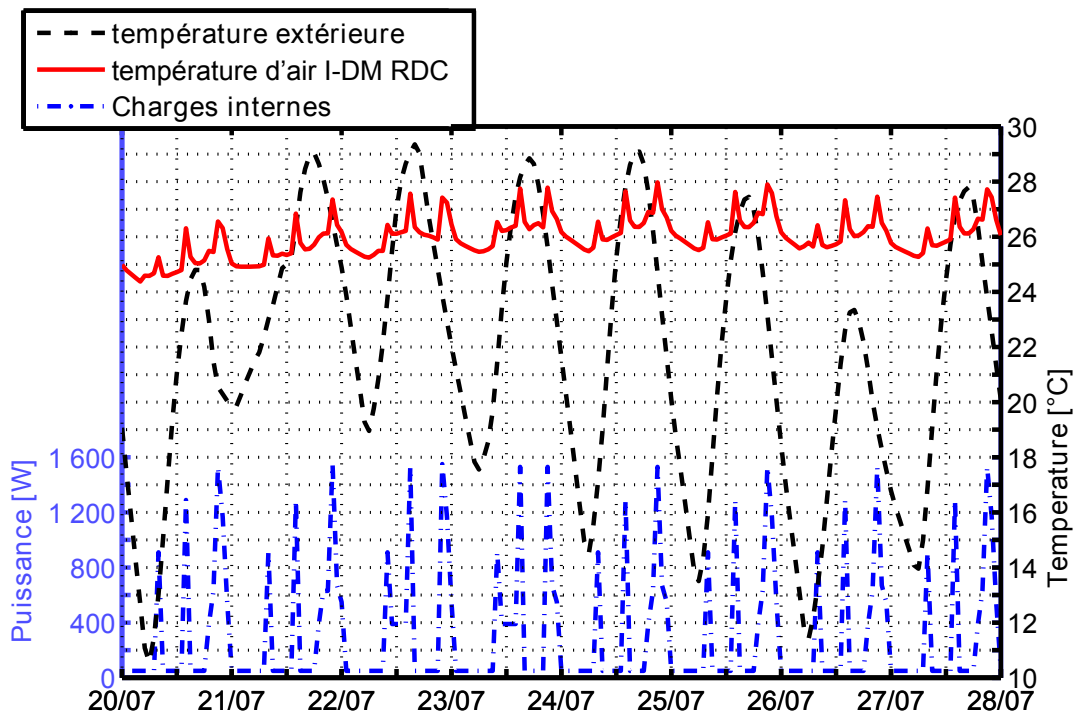
Figure 4.5 – Température intérieure au RDC de la maison I-DM, température extérieure et charges internes dégagées au RDC du 20 au 28 juillet
