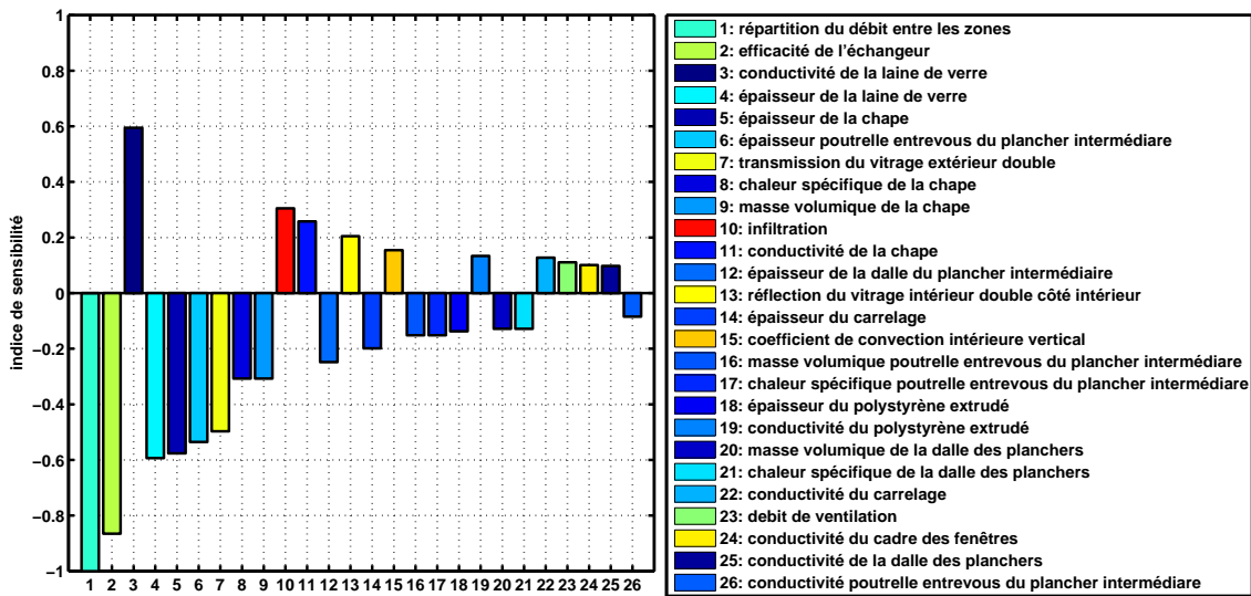
Figure 4.8 – Résultat de l’analyse de sensibilité locale pour le besoin de chauffage pour la maison I-DM
