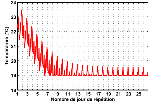
(b) Phase d'initialisation : répétition du 1 er jour de simulation : le 1 er janvier
