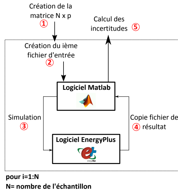
Figure 4.15 – Étape pour obtenir les résultats de l'analyse d'incertitude
