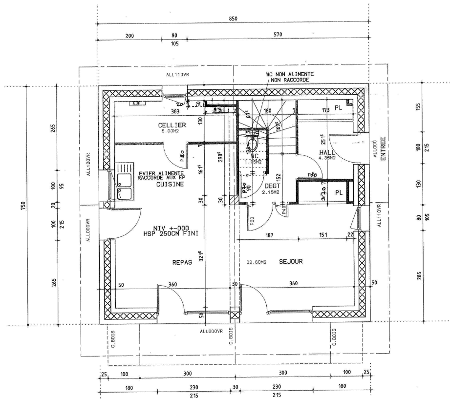
Figure 34 – Plan du RDC de la maison I-DM
