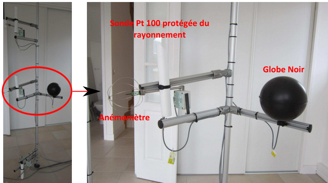
Figure 2.12 – Mât dans la maison I-DM à l'étage se composant de 3 hauteurs différentes 0,10m, 1,10m et 1,70m du sol avec la température d'air et la vitesse d'air ainsi que la température de rayonnement à 1,10m du sol
