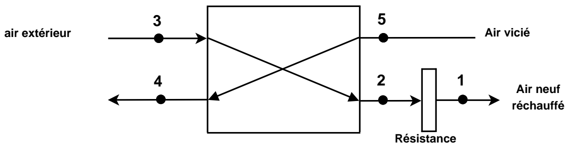
Figure 2.20 – Schéma de l'échangeur
