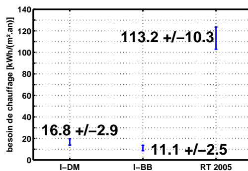
Figure 4.16 – Résultats des moyennes du besoin de chauffage et des incertitudes pour 2000 simulations pour les 3 maisons étudiées
