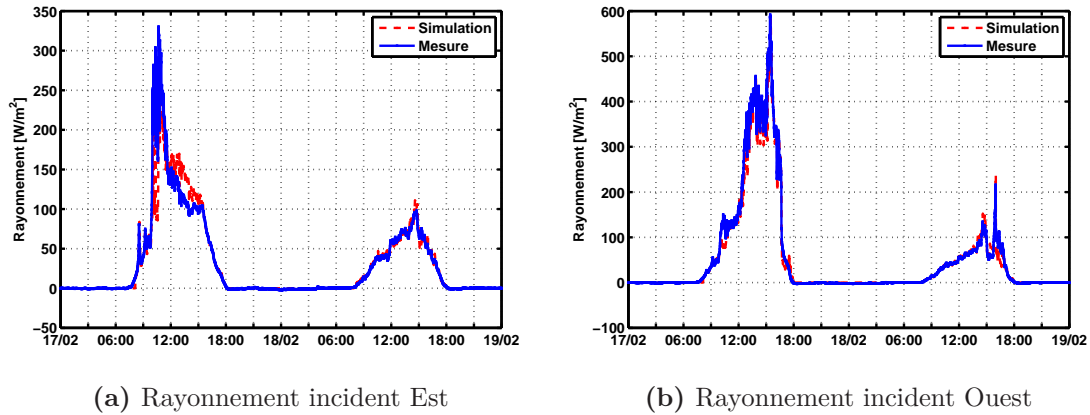
Figure 3.9 – Comparaison mesure simulation pour le rayonnement incident Est et Ouest pour le 17 et 18 février 2011
