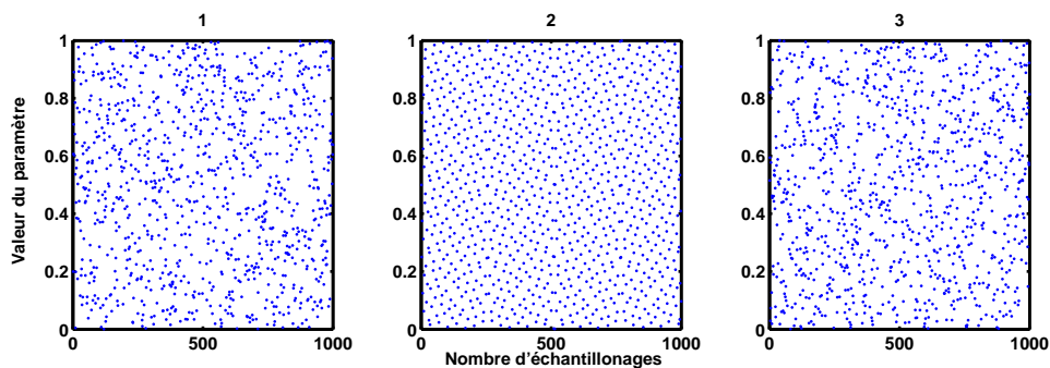
Figure 1.7 – Les trois techniques d'échantillonnage : 1 = la méthode de Monte Carlo, 2 = la méthode de Quasi-Monte Carlo et 3 = l'échantillonnage Latin Hypercube Sampling
