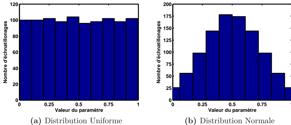
Figure 1.8 – Les deux distributions utilisées : la distribution uniforme et la distribution normale
