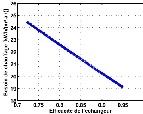
Figure 1.6 – Variation du besoin de chauffage en fonction de la valeur de l’efficacité de l’échangeur pour la maison I-DM
