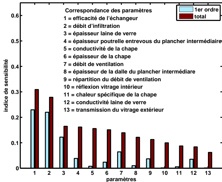
Figure 4.19 – Résultat de l'analyse de sensibilité globale pour le besoin de chauffage pour la maison I-DM
