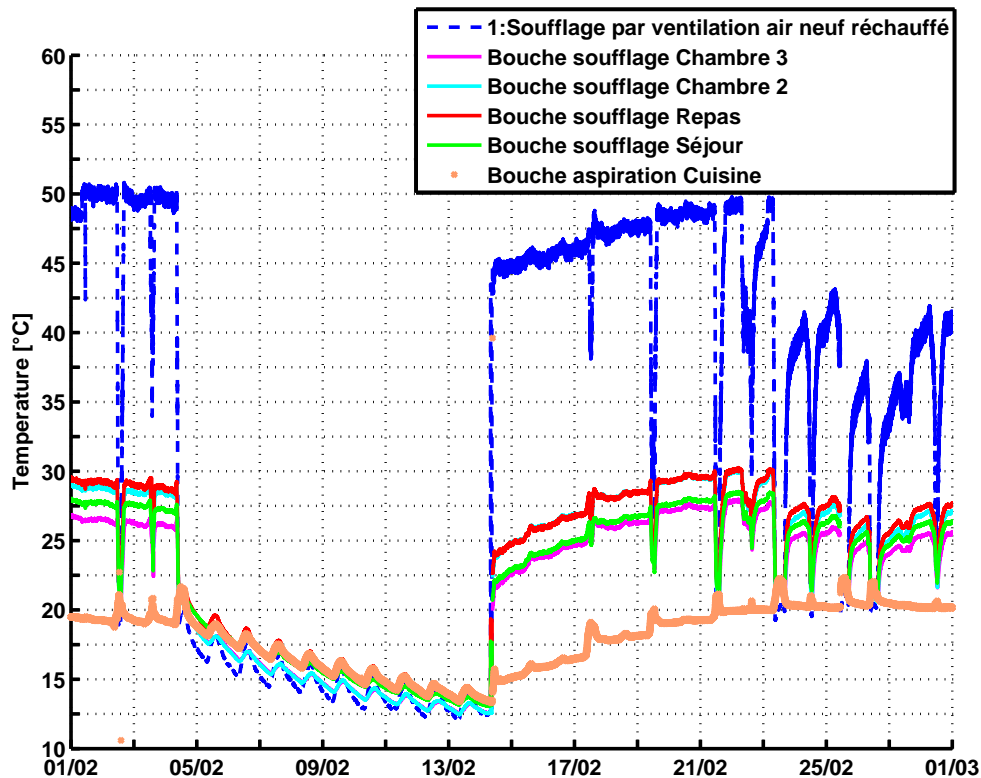
Figure 2.23 – Température d'air du réseau de ventilation pour le mois de février 2011
