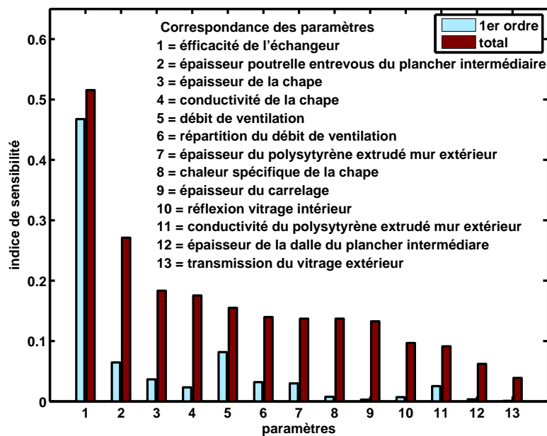
Figure 4.20 – Résultat de l'analyse de sensibilité globale pour le besoin de chauffage pour la maison I-BB
