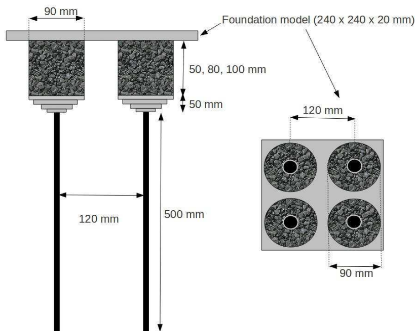
Figure 7.80: Les inclusions rigides (en partie inférieure) sont associées aux colonnes en gravier entourées par l'argile - LTCs (Load Transfer Columns)
