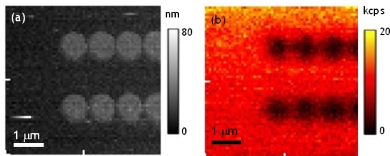
Figure 5.9 : Images ( 25 \mu\text{m}^2 , 64 \times 64 pixels) obtenues en SNOM avec une pointe active à base d'agrégats de YAG:Ce (0.2%). (a) Topographie. (b) Image optique en transmission, filtrée dans la bande d'émission du cérium (passe-bande 582 \pm 40 nm). La fluorescence des agrégats en bout de pointe est utilisée comme source de lumière. La puissance de l'excitation à 457 nm en bout de pointe vaut 1.4 \mu W. Le temps d'intégration par pixel est fixé à 20 ms. Tiré de (11).
