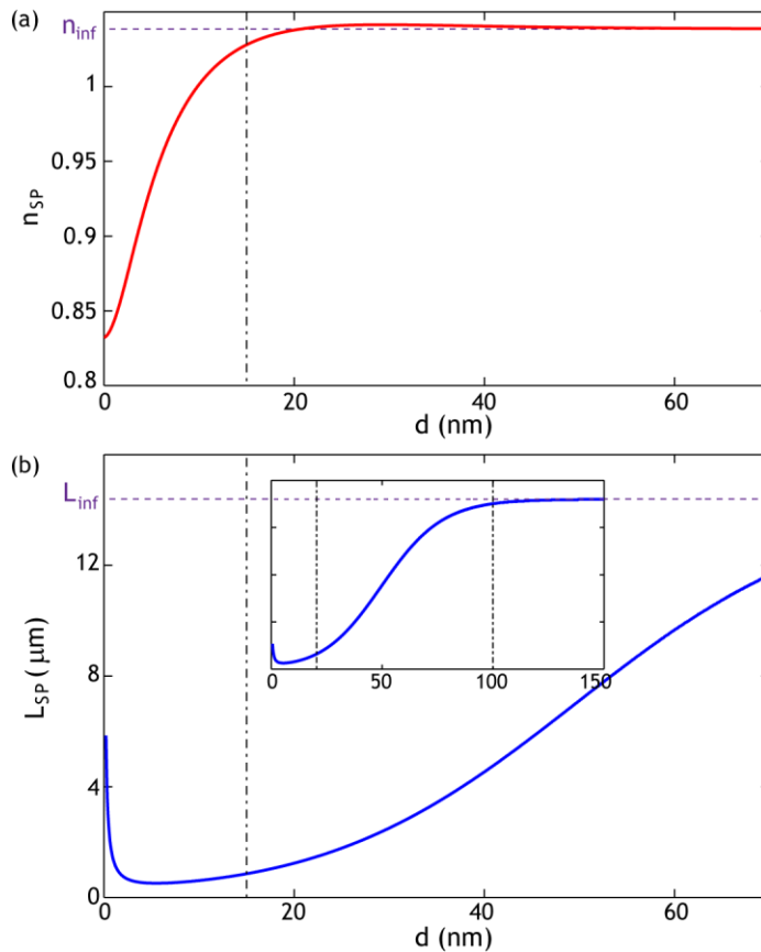
Figure 1.6 : Pour un système air/or/verre et un faisceau incident de longueur d'onde \lambda=661 nm (a) Évolution de l'indice du SP ( n_{SP} = k'_y/k_0 ) avec l'épaisseur d du film métallique. (b) Évolution de la longueur de propagation du SP pour d , entre 0 et 70 nm. (Encart : pour d entre 0 et 150 nm) Les droites n = n_{inf} (a) et L = L_{inf} (b) indiquent les valeurs limites de chaque grandeur dans le cas d'un film infiniment épais.
