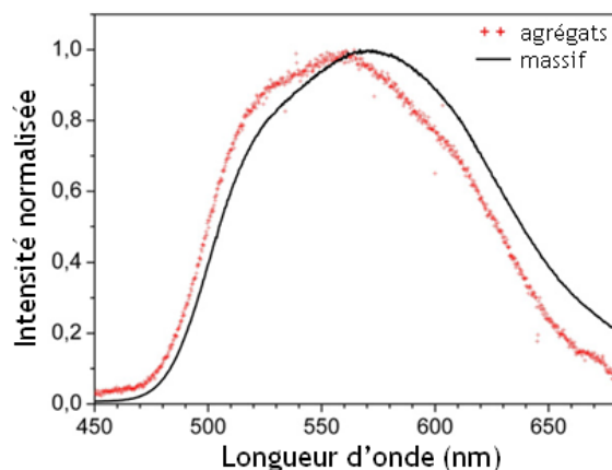
Figure 5.3 : Spectres obtenus en cathodoluminescence (énergie d'excitation 5 keV, courant 0.5 \mu A) pour le matériau massif (courbe noire) et pour les agrégats (marqueurs rouges). Tiré de (11).
