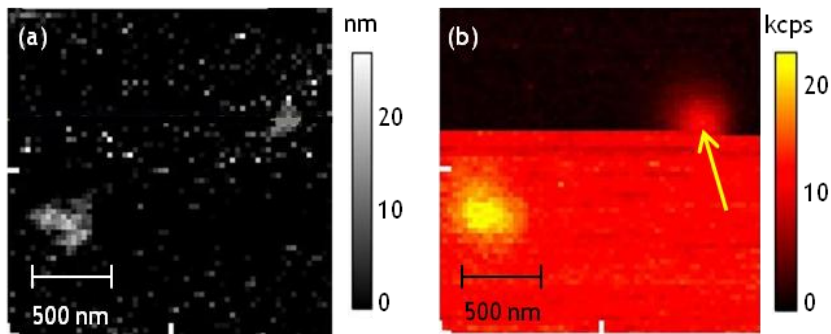
Figure 3.12 : Images ( 2 \mu\text{m}^2 , 64 \times 64 pixels) de l'accroche d'un nano-diamant contenant un centre NV unique en bout d'une pointe SNOM recouverte de poly-l-lysine. Le balayage est effectué de droite à gauche et de haut en bas. (a) Topographie. (b) Image optique en fluorescence. Excitation à 488 nm ( \mathcal{P}_{\text{inj}} = 120 \mu\text{W} ), filtrage dans la bande d'émission du centre \text{NV}^0 (passe-bande 607 \pm 35 \text{ nm} ). Le temps d'intégration par pixel est fixé à 80 ms et la vitesse de scan est de 1 \mu\text{m} \cdot \text{s}^{-1} . La flèche dans l'image (b) marque la position de la pointe lors de l'accroche. Tiré de (28).
