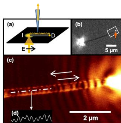
Figure 1.12 : (a) Configuration de la détection en PSTM. (b) Image de l'intensité diffusée : la structure est excitée au niveau du spot brillant, on remarque la lumière diffusée à l'autre extrémité du nano-fil (flèche). (c) Image PSTM au niveau du carré blanc en (b). Les SP invisibles en champ lointain sont maintenant observables. Comme indiqué par les flèches, les SP sont réfléchis au niveau de l'extrémité du fil. (d) Coupe au niveau des franges d'interférences (période \approx \lambda_{SP}/2 ). Tiré de (38).
