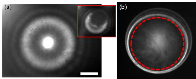
Figure 4.7 : Distribution d'intensité mesurée par LRM en fluorescence avec la sonde active de la Figure 4.6 dans le champ proche du film d'or. (a) Image dans le plan direct de la propagation des SP (barre d'échelle : 10 \mu\text{m} ). Encart : image similaire mais filtrée dans le plan de Fourier. Le signal plasmonique manquant en haut à droite est dû à un faible désalignement du cache dans le plan de Fourier. (b) Image dans le plan de Fourier de la distribution des vecteurs \vec{k} . Le cercle rouge délimite la lumière autorisée. Il illustre la taille du filtre de Fourier. Tiré de (5).
