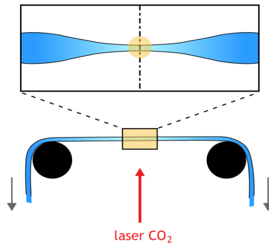
Figure 2.8 : Principe de fabrication des pointes par fusion-étirage. La partie haute de la figure est un zoom au niveau du point d'interaction entre le laser et la fibre. À cause de la chaleur amenée par le faisceau, la pointe fond et s'affine jusqu'à la rupture.
