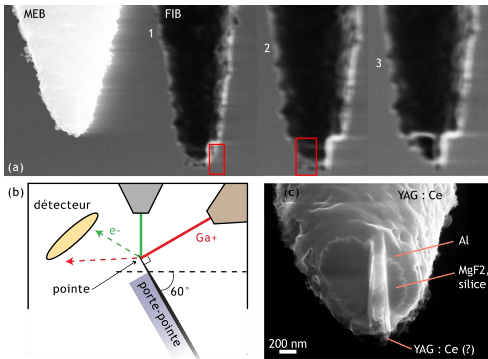
Figure 5.10 : (a) Gravure d'une pointe au FIB en trois étapes. Sur la première image, on observe les images prises simultanément en MEB et en FIB (le contraste n'est pas très bien réglé pour l'image MEB). Les carrés rouges correspondent aux zones gravées. (b) Disposition des différents éléments à l'intérieur du MEB/FIB. Le faisceau vert schématise les électrons, le rouge les ions gallium. Le détecteur est un détecteur d'électrons, il est utilisé pour détecter les électrons secondaires (représentés par les traits en pointillés) créés par l'impact des particules pour chacun des deux faisceaux. (c) Image MEB de la pointe présentée en (a) après gravure. Les différentes couches sont bien visibles. On suppose qu'on a encore quelques agrégats de YAG:Ce sur la crête. La largeur de la crête est d'environ 200 nm. Il n'est pas évident de se rendre compte des autres dimensions car l'angle entre la pointe et le faisceau d'électrons distord l'image.
