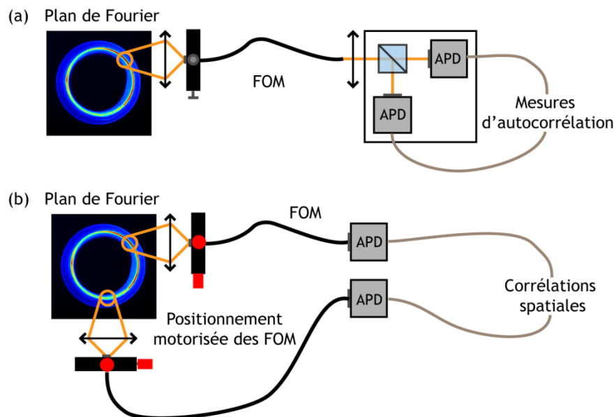
Figure 4.18 : Comparaison entre (a) le montage HBT existant, ici dans la configuration présentée en 4.3.4 et (b) le nouveau montage de corrélation développé en collaboration avec James Hulse stagiaire dans l'équipe Champ proche de novembre 2011 à juin 2012.
