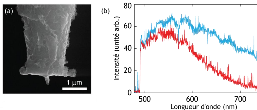
Figure 5.11 : (a) Image MEB d'une pointe, après passage au FIB, avant imagerie optique. Une crête a été taillée en bout de pointe. (b) Spectres mesurés à l'apex de la pointe de l'image (a). (rouge) avant la gravure, (bleu) après. La longueur d'onde d'excitation est 457 nm. Le filtrage est assuré par un miroir dichroïque (MD) à 457 nm et un filtre passe-haut (PH) à 488 nm. Les structurations visibles sur le spectre sont dues au miroir dichroïque.
