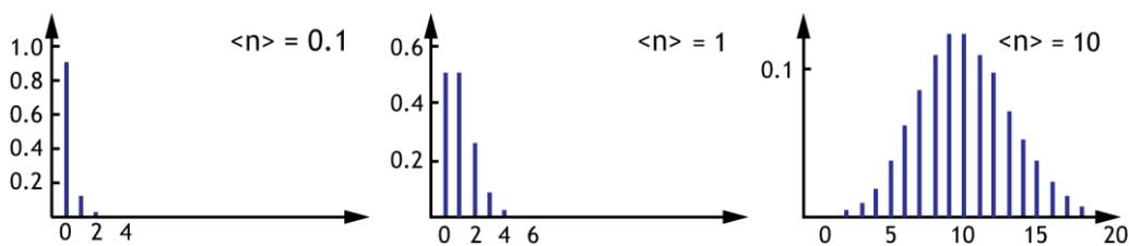
Figure 1.15 : Exemples de distributions poissonniennes pour \langle n \rangle = 0.1, 1 et 10.
