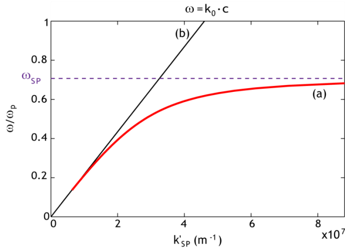
Figure 1.3 : (a) Relation de dispersion pour un plasmon de surface à l'interface air/or. On a aussi représenté l'asymptote horizontale à la courbe de dispersion : \omega = \omega_{SP} qui correspond à la valeur maximale de \omega imposée par le modèle de Drude. (b) Relation de dispersion du photon dans l'air k_0 = \omega/c , aussi appelée ligne de lumière dans l'air.
