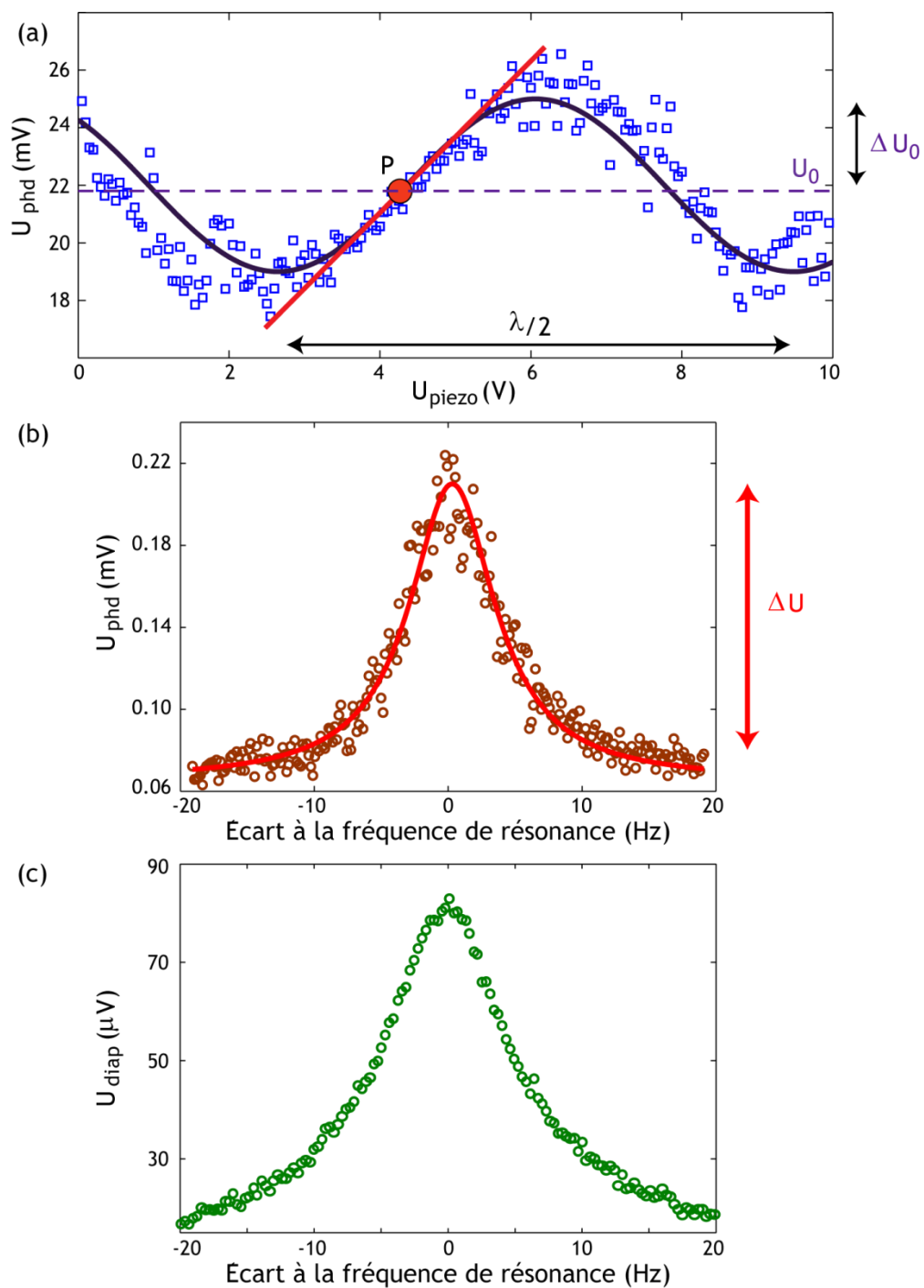
Figure A.20 : (a) Variation de la tension mesurée sur la photodiode U_{\text{phd}} en fonction de la tension U_{\text{piézo}} appliquée sur PZ.
