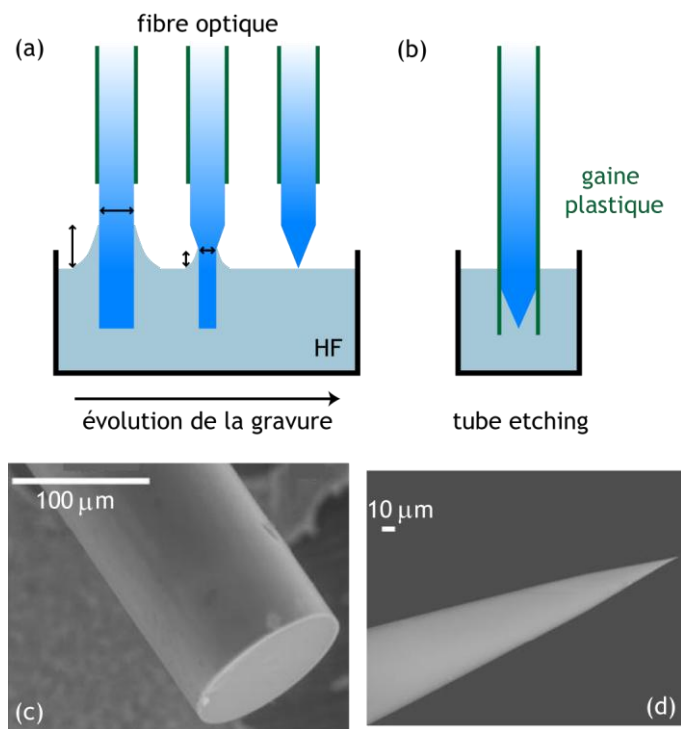
Figure 2.9 : Principe de fabrication des pointes par attaque chimique (a) Technique de gravure à l'acide fluorhydrique (HF) simple. (b) Technique de tube etching . (c,d) Clichés obtenus en microscopie électronique à balayage (MEB) (c) fibre optique avant la gravure, (d) pointe obtenue après gravure simple.
