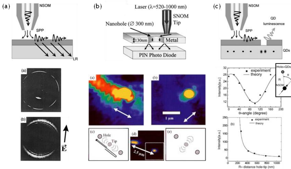
Figure 1.11 : Excitation locale de SP par le champ proche d'une pointe à ouverture. (a) Expérience de B. Hecht et al. : Dispositif expérimental et images obtenues en microscopie de fuites radiatives dans le plan de Fourier sur un film d'argent (en haut) et sur un film d'or (en bas). Tiré de (31). (b) Expérience de Sönnichsen et al. : Dispositif expérimental (film d'argent, \lambda_{exc} = 550 nm) et observation des interférences grâce à la lumière des SP (à 550 nm) diffusée au niveau du trou. Le processus d'interférences est schématisé en (c) et (e) pour une polarisation alignée avec les trous ou orthogonale à cette direction. Tiré de (32). (c) Expérience de Brun et al. : La pointe excite des SP sur le film d'aluminium qui, à leur tour, excitent la fluorescence de boîtes quantiques situées sous le film opaque. La mesure de l'intensité de fluorescence en fonction de la position de la pointe permet de reconstruire la distribution d'intensité des SP. Tiré de (33).
