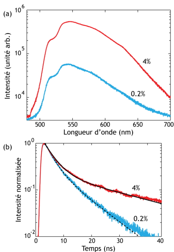
Figure 5.6 : (a) Spectres de photoluminescence obtenus sur une couche épaisse d'agrégats de YAG:Ce dopés à 0.2% et 4%.
