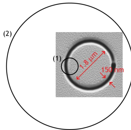
Figure 4.12 : Cliché MEB de la nanostructure étudiée. On a reporté sur l'image les dimensions caractéristiques. (1) et (2) représentent la taille relative des zones confocales de détection au niveau de l'échantillon obtenues pour les FOM de diamètre D_1=50 \mu\text{m} et D_2=365 \mu\text{m} respectivement. Le grossissement du microscope vaut M=60 .
