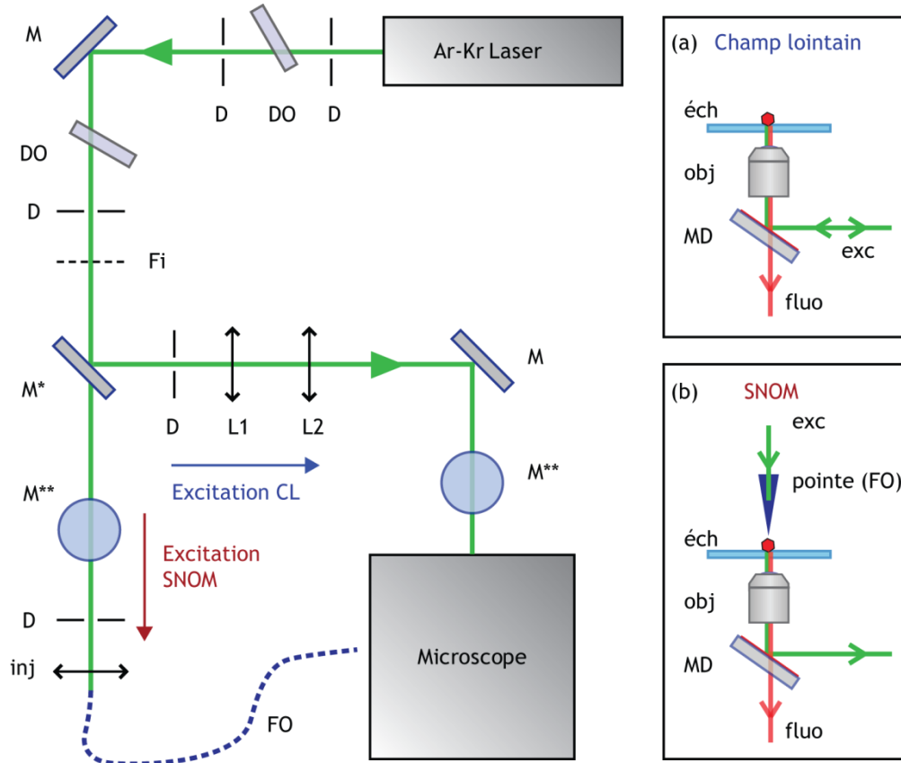
Figure 2.16 : Présentation du montage optique de mise en forme du faisceau. Liste des abréviations utilisées : DO densité optique, M miroir, D diaphragme, Fi filtre interférentiel, L1 et L2 lentilles, inj bloc d'injection dans la fibre optique, FO fibre optique. M* est un miroir amovible qui permet de choisir l'un ou l'autre des bras. M** représente en fait deux miroirs disposés en périscope pour élever le niveau du faisceau par rapport à la table optique. Encarts : Détail de l'intérieur du microscope pour les deux configurations d'excitation : (a) en champ lointain (CL) et (b) en SNOM. Le faisceau d'excitation (exc) est amené au niveau de l'échantillon (éch) soit par l'objectif (obj) soit par la pointe. La fluorescence (fluo) de l'émetteur excité est collectée par l'objectif. MD est un miroir dichroïque adapté à l'excitation.
