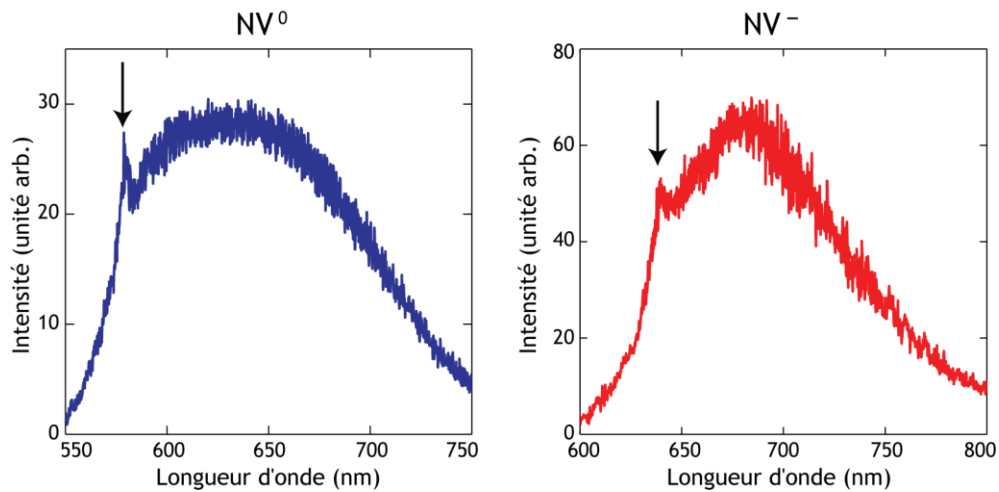
Figure 3.2 : Spectre d'émission des centres NV^0 et NV^- . Les flèches indiquent la ZPL de chaque spectre.
