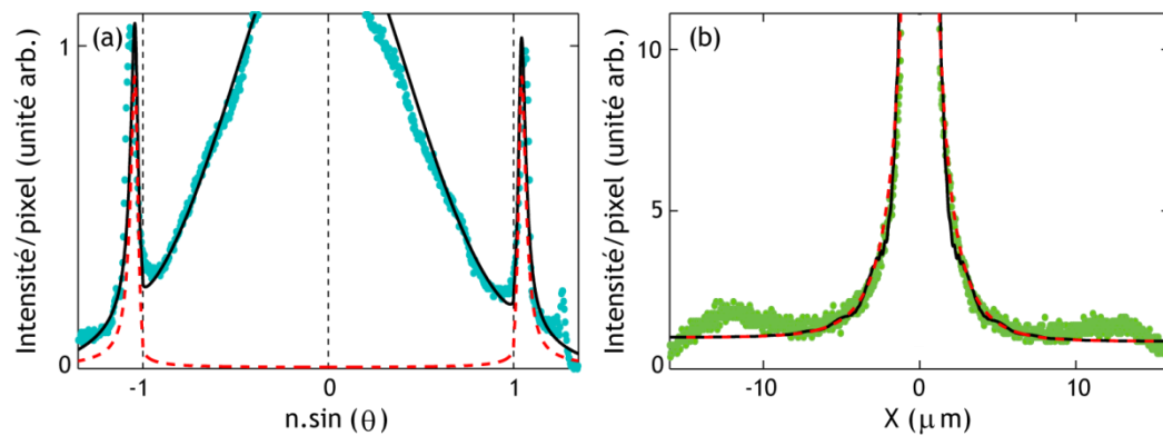
Figure 4.10 : (a) Coupe de l'intensité collectée dans le plan de Fourier le long de la ligne blanche pointillée Figure 4.9 (b). La courbe rouge représente le profil d'intensité théorique des plasmons de surface pour un dipôle perpendiculaire au film métallique. La distribution d'intensité totale incluant le signal autorisé non plasmonique est modélisée par la courbe noire. La coupure à droite correspond à l'ouverture numérique \text{NA}_{\text{eff}} = 1.35 . (b) Coupe de l'intensité collectée dans le plan direct selon la ligne blanche pointillée Figure 4.9 (a). La courbe rouge illustre le profil d'intensité théorique des plasmons de surface alors que la courbe noire tient compte aussi de la lumière non plasmonique. Les sortes d'épaules visibles près des bords sont attribuées au champ de vision fini du microscope.
