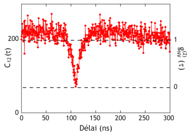
Figure 3.4 : Courbe d'autocorrélation d'un centre NV unique dans un nano-diamant (objet A Figure 3.3). Axe de gauche : valeurs pour l'histogramme brut. Axe de droite : valeurs pour l'histogramme corrigé (voir texte), c'est-à-dire la fonction d'autocorrélation réelle du centre.
