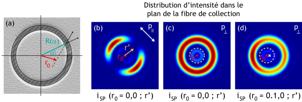
Figure 4.15 : (a) Détail des coordonnées utilisées pour la suite. (b–d) Distributions d'intensité i_{SP}(\vec{r}_0, \vec{r}') (4.15) dans le plan-image du microscope où est située la FOM de collection, pour un dipôle horizontal orientée selon la double flèche (b) et pour un dipôle vertical (c) (d) et pour différentes positions r_0 de la pointe (marquée par une croix rouge). Le cercle pointillé apparaissant sur les images (c) et (d) indique la position de la FOM 1, à tout instant alignée avec la pointe. La FOM 2 englobe quant à elle la totalité de l'image. La configuration expérimentale peut être retrouvée sur la Figure 4.14 (b).
