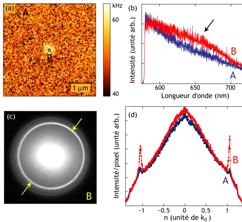
Figure 4.5 : (a) Cartographie du signal optique mesurée en confocal en fluorescence (passe-haut 578 nm) sur des nano-diamants dispersés sur un film d'or de 50 nm. Excitation à 515 nm avec une puissance de 1 mW. I(A) \approx 47 \text{ kHz} , I(B) \approx 64 \text{ kHz} . (b) Spectres mesurés en A (courbe bleue, film d'or seul) et en B (courbe rouge, film d'or+objet lumineux). (c) Distribution de l'intensité LRM dans le plan de Fourier en B lorsque le filtre passe-haut à 578 nm est ajouté dans le faisceau. (d) Comparaison des coupes effectuées sur des images non saturées équivalentes aux images (c) ci-contre (en rouge) et (b) de la Figure 4.4 (en bleu).
