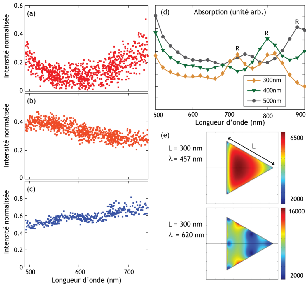
Figure 5.18 : (a–c) Spectres d’extinction (voir équation (2.1)) de nano-prismes uniques. Spectres (a) et (b) mesurés en champ proche sur deux prismes différents avec une même pointe. Le spectre (b) est celui du prisme de la Figure 5.17. Spectre (c) pris sur un troisième prisme avec une autre pointe maintenue à un micron de la surface. (d) Spectres d’absorption calculés pour des prismes en or de différentes tailles. (e) Cartes simulées de l’intensité diffusée au niveau du prisme, pour un prisme de 300 nm de côté, à 457 nm (excitation du YAG:Ce, dans l’interbande de l’or) et à 620 nm (résonance du prisme de 300 nm). Noter l’échelle différente sur les deux images.
