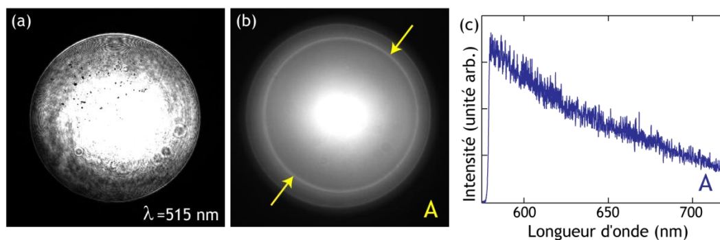
Figure 4.4 : Étude des propriétés optiques du film d'or de 60 nm d'épaisseur sous excitation à 515 nm. (a) Distribution de l'intensité LRM dans le plan de Fourier à la longueur d'onde du laser. (b) Distribution de l'intensité LRM dans le plan de Fourier lorsque le filtre passe-haut à 578 nm est ajouté dans le faisceau. (c) Spectre caractéristique de la luminescence de l'or, mesuré en configuration confocale sous excitation à 515 nm. (A) fait référence à la position du faisceau lors de l'acquisition des images (voir Figure 4.5 (a)).
