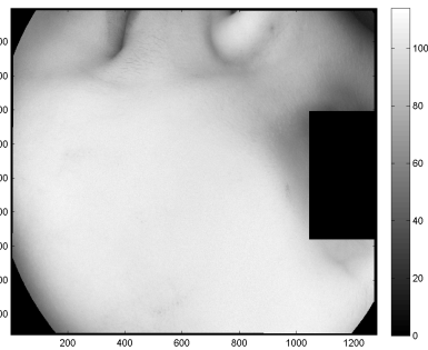
(d) 870 nm
