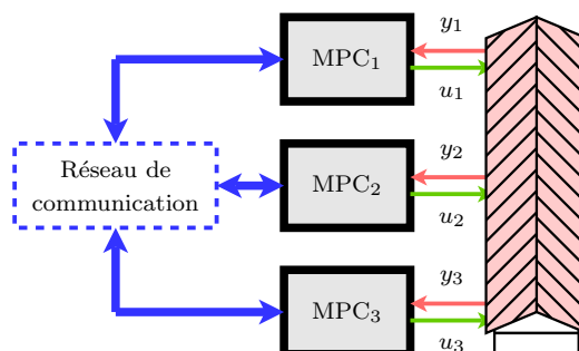
FIGURE 2.8 – Schéma de contrôle distribué
