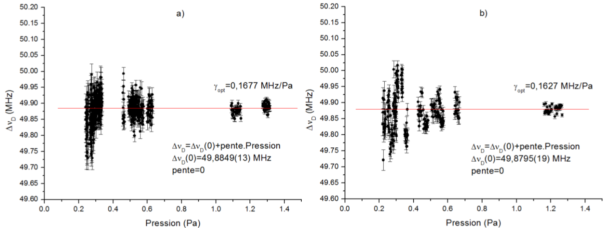
Figure V-15 : Evolution de la demi-largeur Doppler à 1/e en fonction de la pression et moyenne pondérée \Delta v_D(0) correspondante, pour une puissance laser incidente dans la cellule d'absorption a) P_{Laser}^A \sim 0,45 W et b) P_{Laser}^B \sim 0,9 W .
