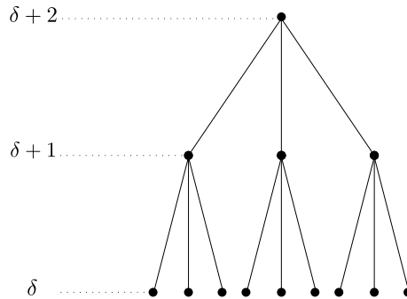
FIGURE 3.1 – L'arbre de B/KZ
