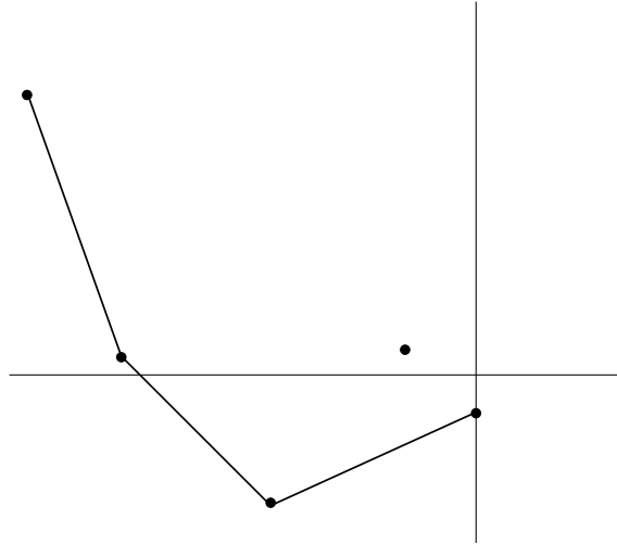
FIGURE 2.1 – Polygone de Newton d'un polynôme à cinq monômes
