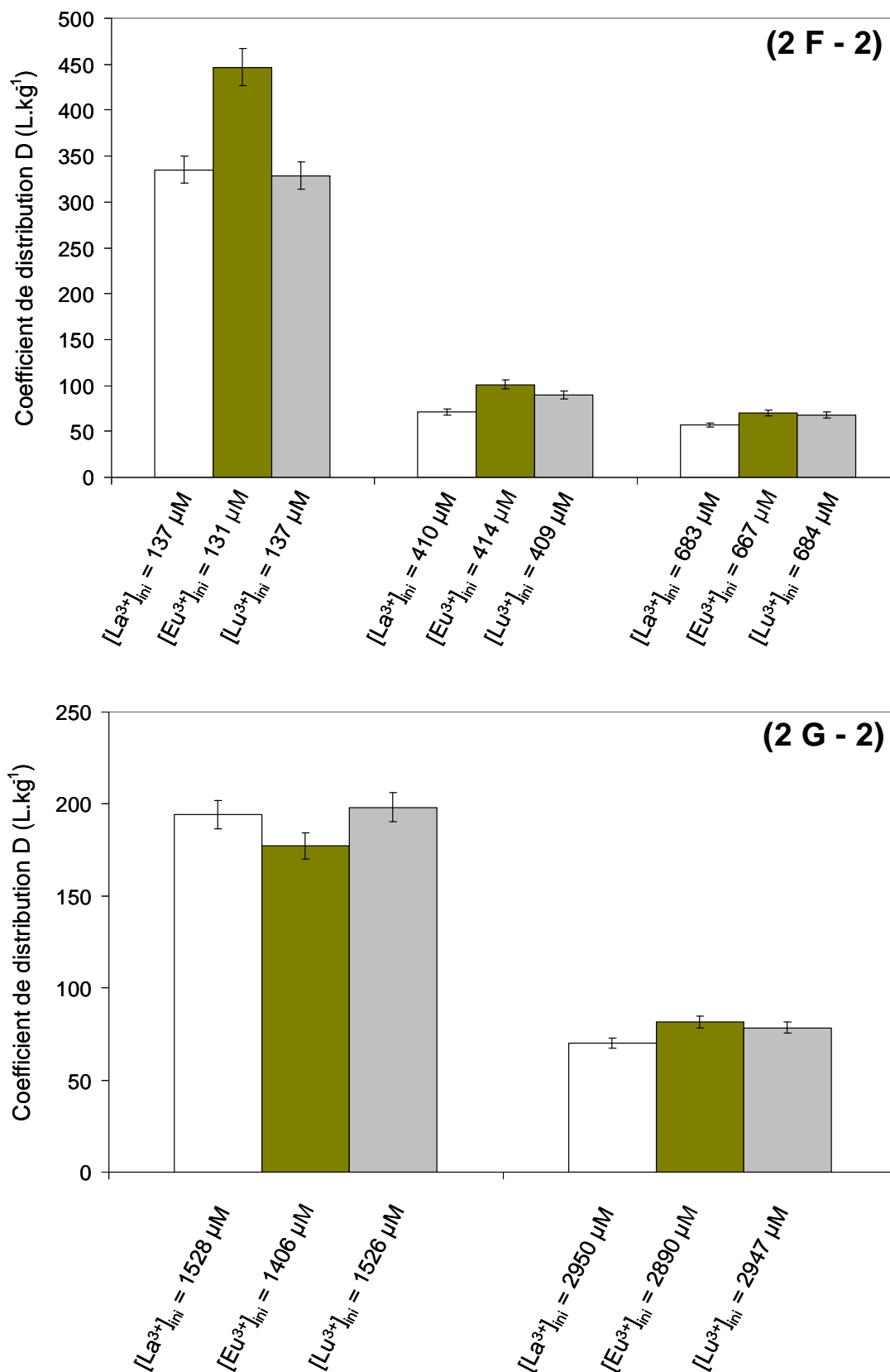
Figure III.13 : Coefficient de distribution du \text{La}^{3+} , de l' \text{Eu}^{3+} et du \text{Lu}^{3+} pour les polymères 2 F - 2 et 2 G - 2 et pour différentes concentrations initiales en lanthanide.
