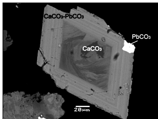
Figure III.11 : Grain de calcite en section polie observé au MEB en mode rétrodiffusé Rhombôdre de calcite en section, la zone plombifère montre une alternance de couches plus ou moins claires selon les teneurs en Pb.
