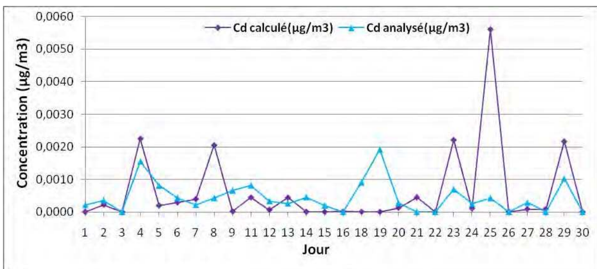
Figure VI.24 : Variation journalière des concentrations calculés et analysées de métaux dans les PM10 au point de prélèvement situé sur la terrasse de la maison en face du terrier DIII
