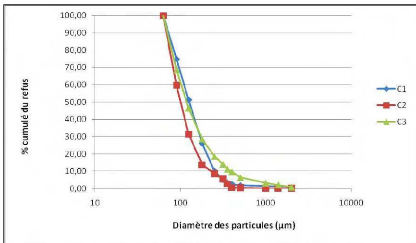
Figure III.2 : Distribution granulométrique de la fraction supérieure à 63 µm dans les carottes.
