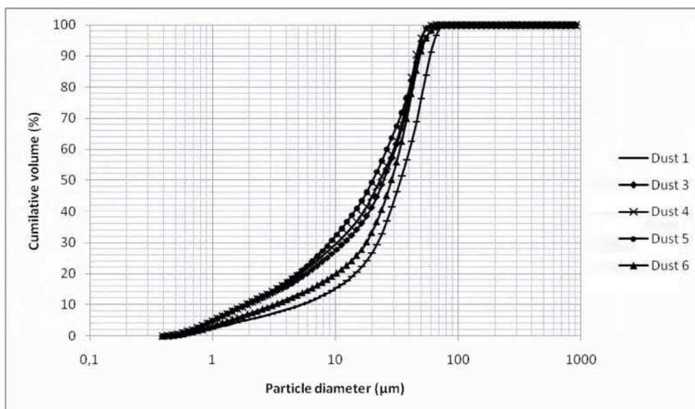
Figure VII.3 : Courbes granulométriques des échantillons de poussières
