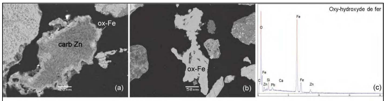
Figure III.15 : grains d'oxy-hydroxyde de fer observés au MEB-EDS en mode rétrodiffusé et exemple de spectre EDS.
