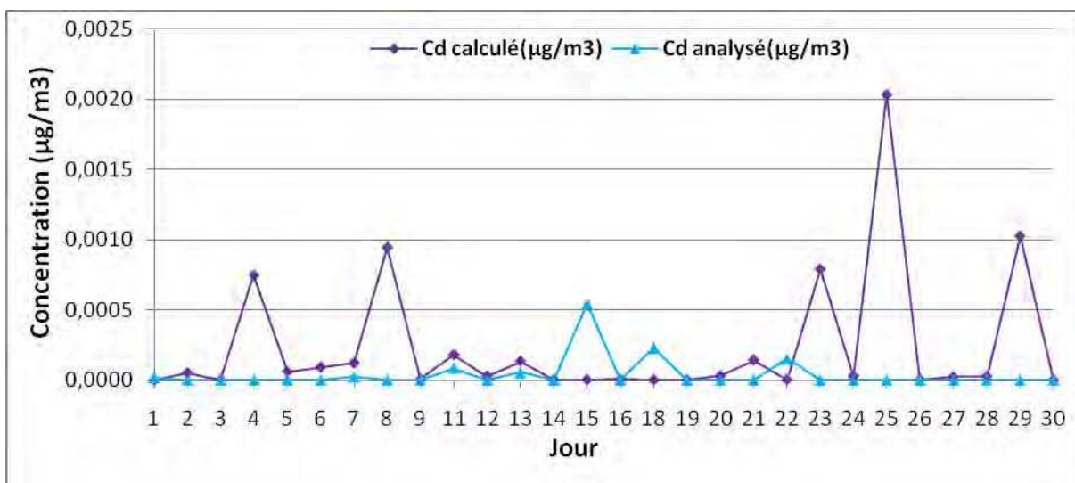
Figure VI.27 : Variation journalière des concentrations calculées et analysées de métaux dans les PM 2,5 au point de prélèvement situé sur la terrasse de la maison en face du terril DIII
