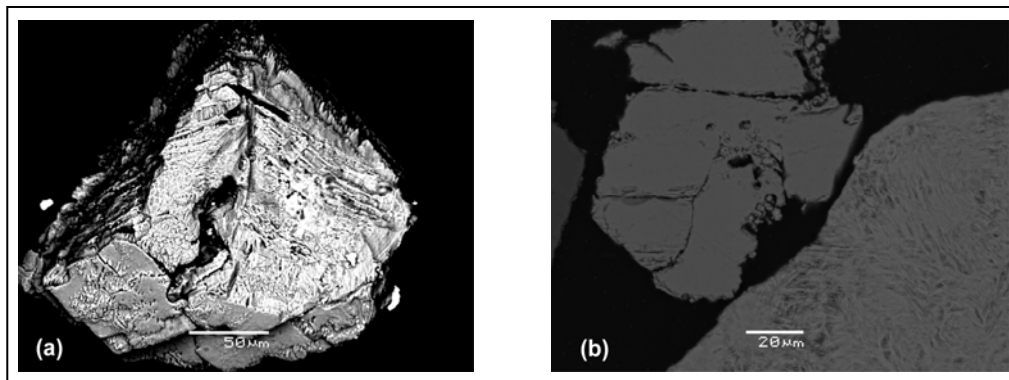
Figure III.7 : Carbonates de Zn observés au MEB en mode rétrodiffusé (a) grain isolé de carbonate de Zn d'aspect feuilleté mais compact avec un dépôt finement fibreux et probablement secondaire de carbonate de Zn. Photo (b) : deux grains de carbonates de Zn en section polie
