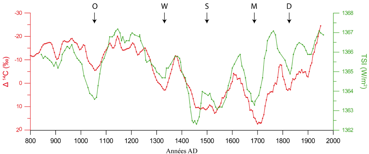
Fig. 1.3. Comparaison de deux reconstitutions indépendantes de l'activité solaire depuis 800 AD basées sur des proxys différents : le 14 C résiduel de la courbe de calibration INTCAL09 mesuré dans les cernes d'arbres (en rouge) (Reimer et al, 2009), et l'irradiance totale (TSI) déduite de la mesure du 10 Be dans une carotte de glace antarctique (en vert) (Bard et al, 2000 ; 2007). Noter la concordance entre les deux séries, ainsi que l'occurrence de grand minima solaires sur cette période (O : Oort, W : Wölf, S : Spörer, M : Maunder, D : Dalton). La courbe INTCAL a été inversée afin que les minima soient vers le bas.
