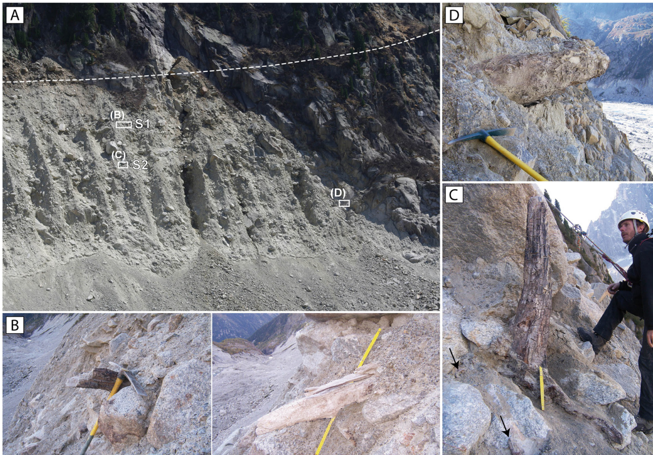
Fig. 3.17. Secteur 5. Site #11 et #12. (A) Vue E du Secteur 5 depuis le glacier. Les tiretés représentent l'extension maximale PAG ; (B) Strate S1, Site #11. Echantillons MDG5-03 (g.) et MDG5-02 (dr., échelle :1m) ; (C) Strate S2, Site #11. Tronc in situ MDG5-04. Les flèches pointent des fragments de racine en place, désolidarisés du tronc ; (D) Site #12. Echantillon MDG5-01.
