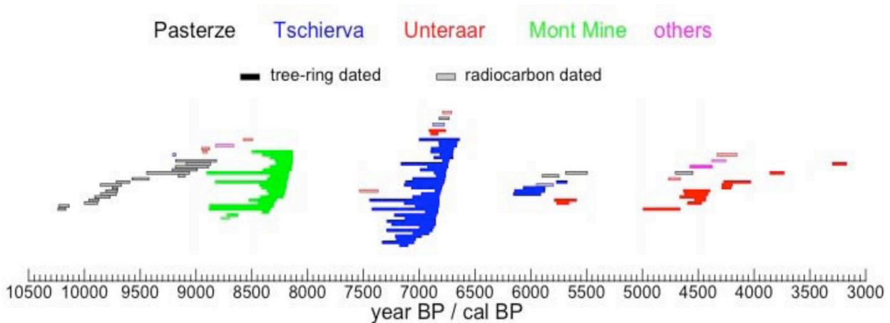
Fig. 2.32. Compilation des dates dendrochronologiques et radiocarbone obtenues sur bois subfossiles dans 4 marges proglaciaires des Alpes suisse et autrichienne, interprétées comme marquant des périodes de retrait glaciaire plus important que l'actuel pendant l'Holocène. Noter la proximité des dates de mort des arbres, et la quasi-absence de dates après 4.0 ka (glacier de l'Unteraar excepté). (Nicolussi et Schlüchter, http://quest.bris.ac.uk/workshops/ASM_08/talks/schluchter.pdf )
