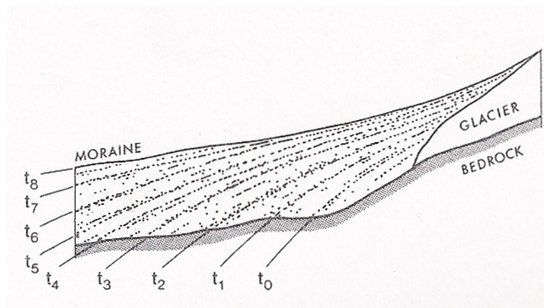
Fig. 2.24. Profil en long schématique de la stratification dans une moraine latérale. Les strates à blocs sont représentés par des isochrones ( t_0 - t_8 ), de plus en plus récentes vers la crête de la moraine (Humlum, 1978).
