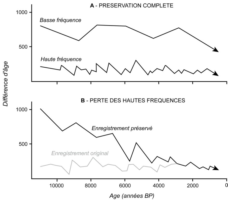
Fig. 2.36. Cadre conceptuel (diagramme « différence d'âge ») permettant d'évaluer les chronologies glaciaires et d'identifier l' « autocensure » du système. (A) Pas de perte de l'enregistrement glaciaire par érosion. Des enregistrements complets produits par des glaciers aux temps de réponse différents, en réponse à des cycles climatiques réguliers, correspondraient à cet exemple ; (B) Un enregistrement incomplet : la différence d'âge entre les formes successives diminue vers le présent. Un tel exemple peut s'expliquer par une préservation sélective due à l'érosion. La fréquence originelle des évènements ne peut plus être déduite des formes les plus anciennes (Kirkbride et Brazier, 1998).
