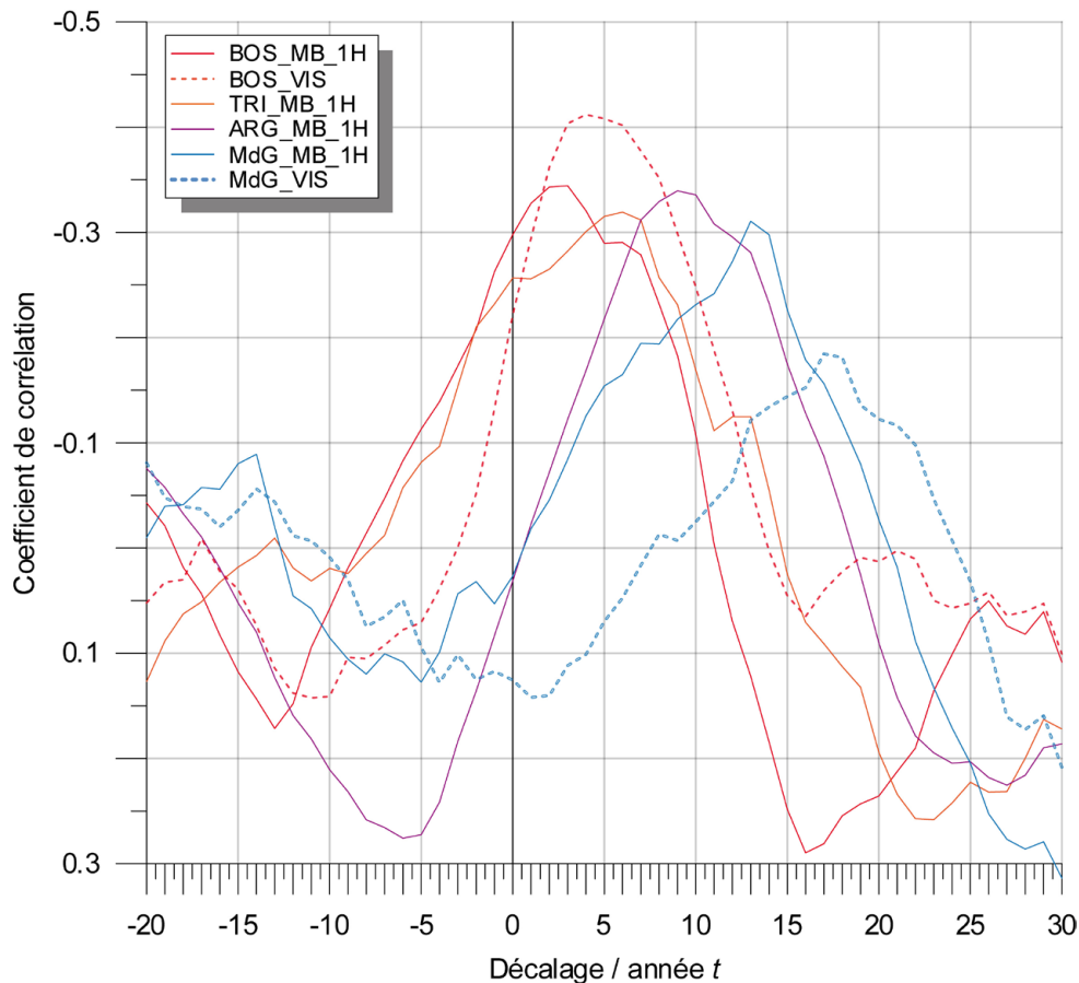
Fig. 4.20. Cross-corrélations entre les variations de longueur des glaciers du versant nord du MMB, et les indices de largeur de cerne pour Bossons (1870-2008), Trient (1879-2008), Argentière et Mer de Glace (1878-2008) (trait plein : chrono MB_1H, tiretés : chrono VIS)
