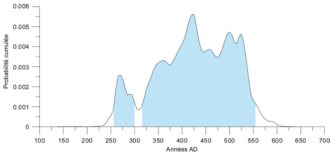
Fig. 3.34. Probabilité cumulée des dates 14 C (2 σ) représentatives de la mort des arbres de la strate S2 du glacier des Bossons.
