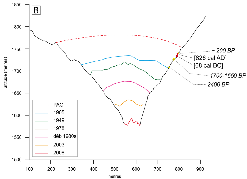
Fig. 3.33. Comparaison de l'altitude des bois datés dans la moraine latérale droite du glacier d'Argentière avec l'altitude de la langue à différentes périodes du 20 e s selon deux profils (localisation : Fig. 3.18). La position des bois datés par Bless (1984) sur le même secteur est donnée à titre indicatif (dates en italiques) d'après les altitudes rapportées par cet auteur. (Exagération verticale x 2).
