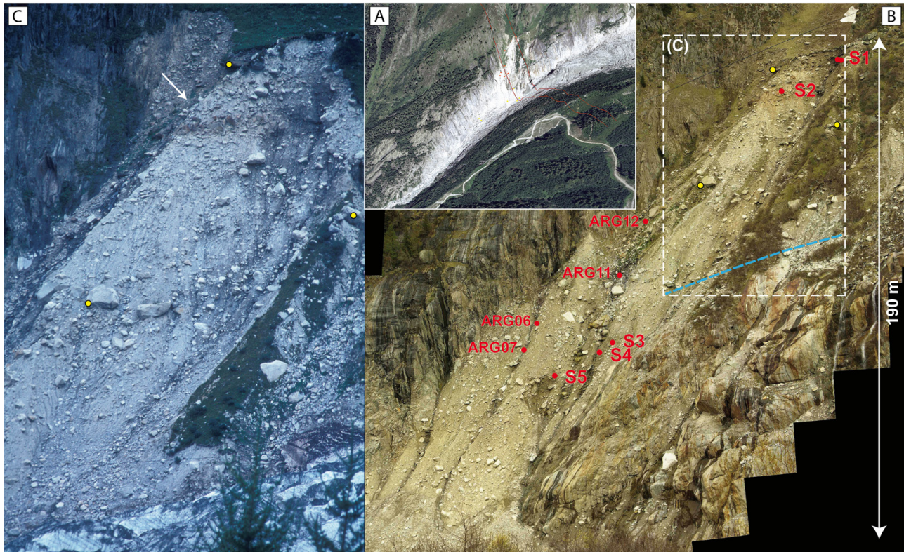
Fig. 3.19. Moraine latérale droite du glacier d'Argentière. (A) Vue ESE avec la position des bois détritiques et des bois en place (Orthophoto 2008 drapée sur MNT Lidar) ; (B) Vue E rapprochée, et position des strates de bois en place (Sxx) et des bois remaniés. La zone en tirets correspond à la même portion sur (C) prise en 09/1978 (photo R. Bless). La partie supérieure du secteur échantillonné par R. Bless est indiquée par la flèche (en face nord, non visible ; Les points jaunes sont des repères communs aux deux photographies). Noter la présence de la marge glaciaire à l'aval du profil en (C), reportée en (B).
