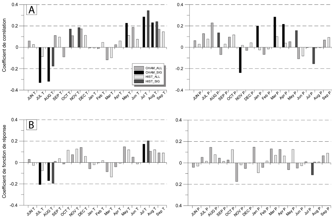
Fig. 4.12. Coefficients de corrélation (A), et fonctions de réponse (B), calculés entre la chronologie de Pinus cembra , et les températures (g) et précipitations (dr.) moyennes, pour le MMB (chrono CHAM / station Chamonix : 1935-2008 ; chrono MB_1H / Histalp_Low : 1826-2008). Les coefficients significatifs au seuil de 95% (SIG) correspondent aux aplats les plus sombres. Les mois de l'année t-1 sont indiqués en majuscule.
