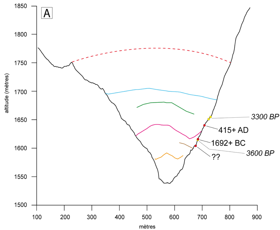
Fig. 3.33. Comparaison de l'altitude des bois datés dans la moraine latérale droite du glacier d'Argentière avec l'altitude de la langue à différentes périodes du 20 e s selon deux profils (localisation : Fig. 3.18). La position des bois datés par Bless (1984) sur le même secteur est donnée à titre indicatif (dates en italiques) d'après les altitudes rapportées par cet auteur. (Exagération verticale x 2).
