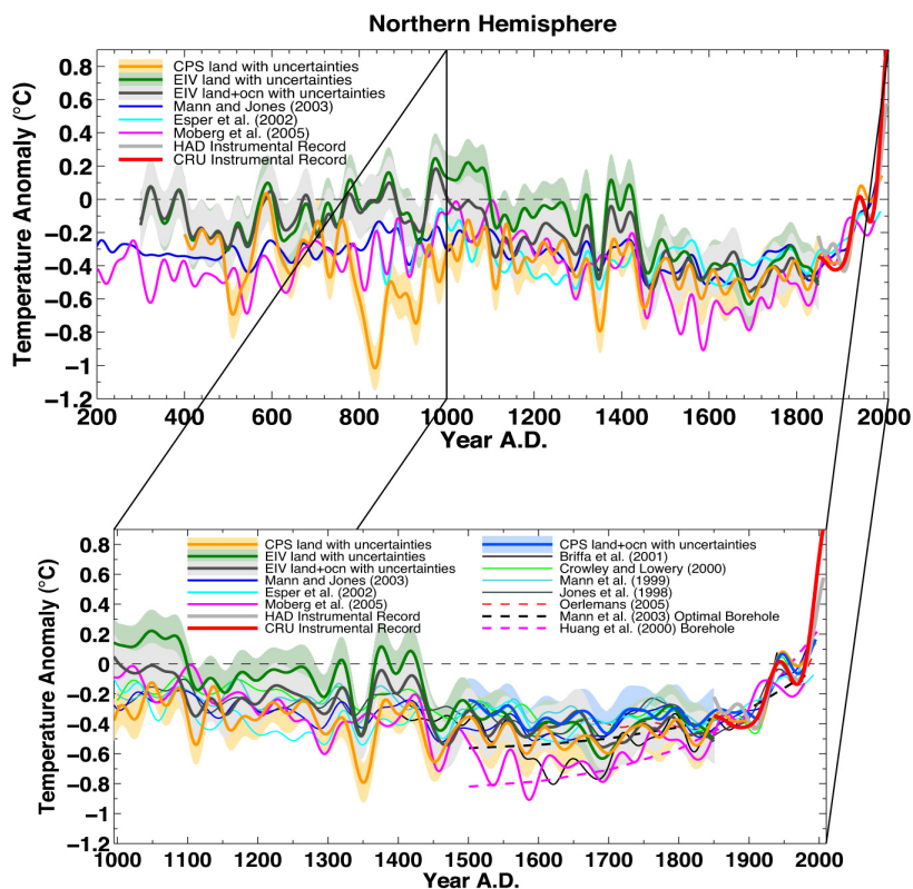
Fig. I-3. Reconstitution des températures de l'hémisphère nord sur les deux derniers millénaires d'après la combinaison de différents proxies par Mann et al (2008), et comparaison avec les reconstitutions existantes. Noter l'ampleur remarquable du réchauffement intervenu au 20 e s (températures instrumentales en rouge), sans équivalent sur la période considérée.
