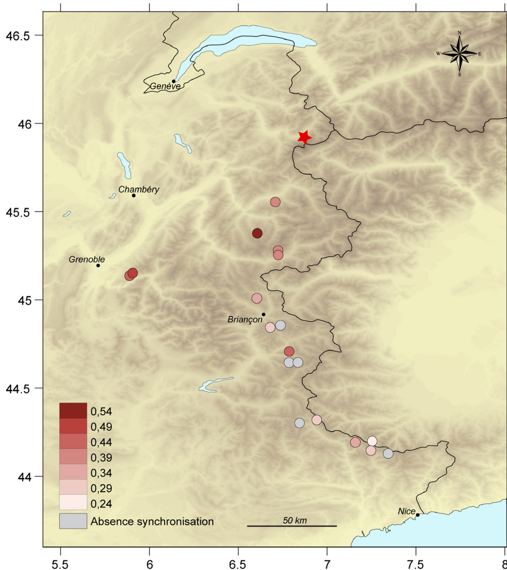
Fig. 4.15. Corrélations entre la chronologie MB_1H et les chronologies de Pinus cembra des Alpes occidentales (données : F. Meijer/ITRDB ; Petitcolas et Rolland, 1998 ; Edouard et al, 2002 ; Edouard non publié ; Saulnier et al, 2011). Calculs effectués avec le Logiciel DENDRON (Lambert, 2006) après standardisation des données avec la méthode de Besançon (Lambert, 2006) Les coefficients présentés correspondent à la position de synchronisation juste (les valeurs du t de Student correspondantes sont comprises entre 3,7 et 9,7). Les chronologies dont les meilleurs résultats indiquent des positions de synchronisation erronées sont représentées en gris ( r \leq 0,33 ).
