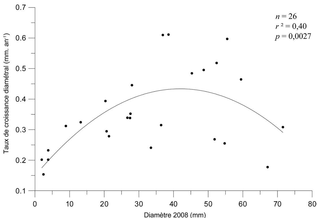
Fig. 6.9. Taux de croissance diamétral en fonction du diamètre initial (année 2008) déterminé d'après le suivi direct.
