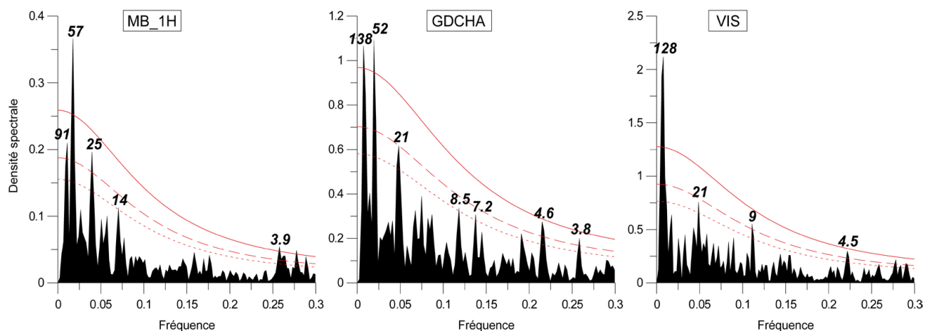
Fig. 4.11. Analyse spectrale des chronologies STD (méthode REDFIT, nombre de segments=3). Les lignes représentent les seuils de signification p < 0,01 , p < 0,05 et p < 0,1 . Les périodes (en années / cycle), correspondant aux fréquences significatives, sont indiquées. Noter l'échelle différente de l'axe des ordonnées.
