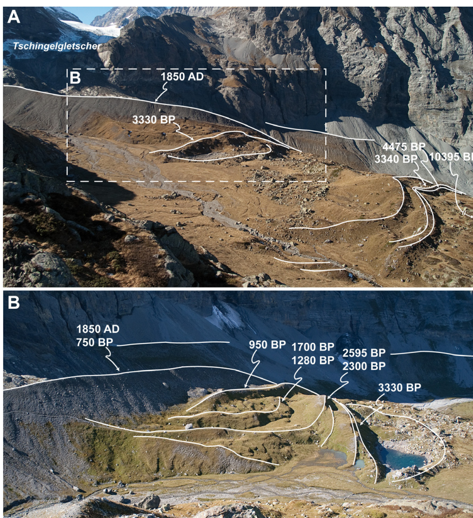
Fig. 2.33. Les cordons morainiques néoglaciatres du glacier de Tschingel (Oberland) dans le secteur de l'Oberhornsee. Les datations reportées sont les âges ^{14}\text{C} conventionnels de sols recouverts par du matériel morainique. Les flèches indiquent les moraines datées (Wipf, 2001). Noter l'extension latérale du glacier au début du Néoglaciatre (~700 m / 1850 AD) et la conservation d'une séquence morainique remarquable du fait d'une tendance récessionnaire et de la prévalence de l'accrétion proximale dans la construction de l'amphithéâtre morainique (photo A. Wipf ; (A) 28/10/05, (B) 21/09/06).
