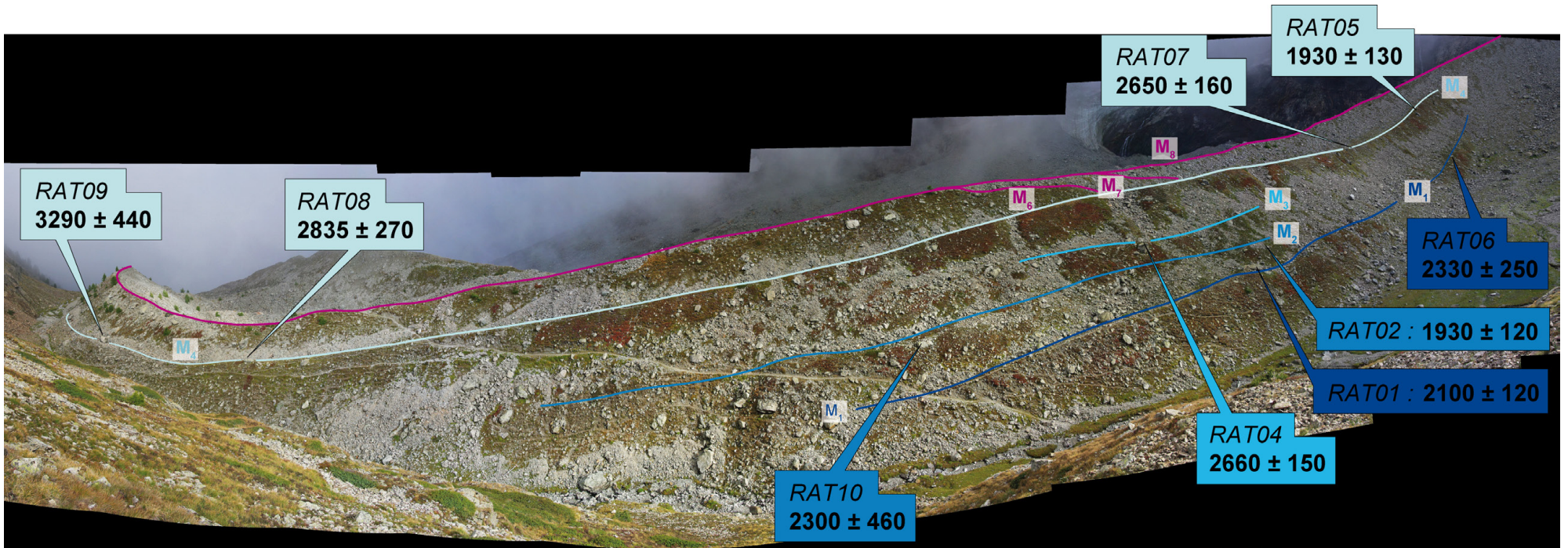
Fig. 5.10. Datations ^{10}\text{Be} sur le lobe latéral gauche du glacier du Rateau. Les âges sont accompagnés des seules incertitudes analytiques. Les cordons M5 (non visible) à M8 n'ont pas été échantillonnés.
