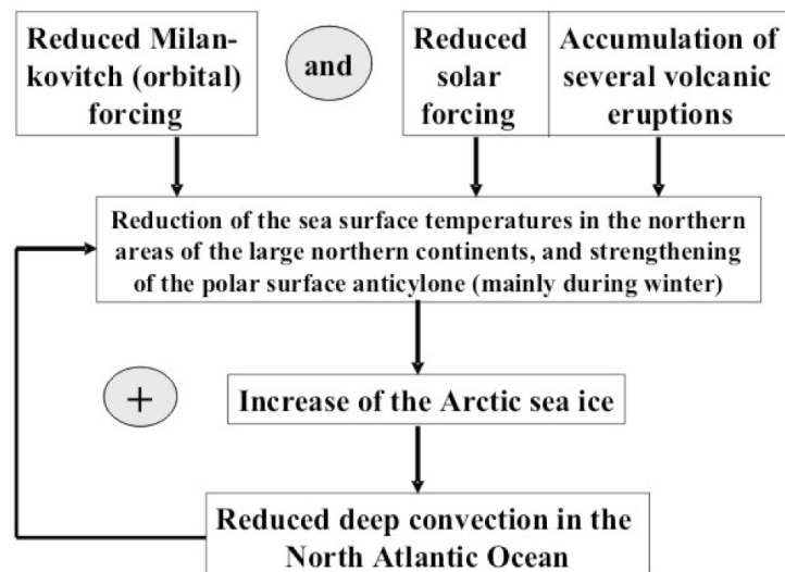
Fig. 1.9. Principaux forçages à l'origine des événements froids de la fin de l'Holocène, et rétroactions positives impliquant l'océan dans le maintien de ces conditions (Wanner et Büttikofer, 2008)
