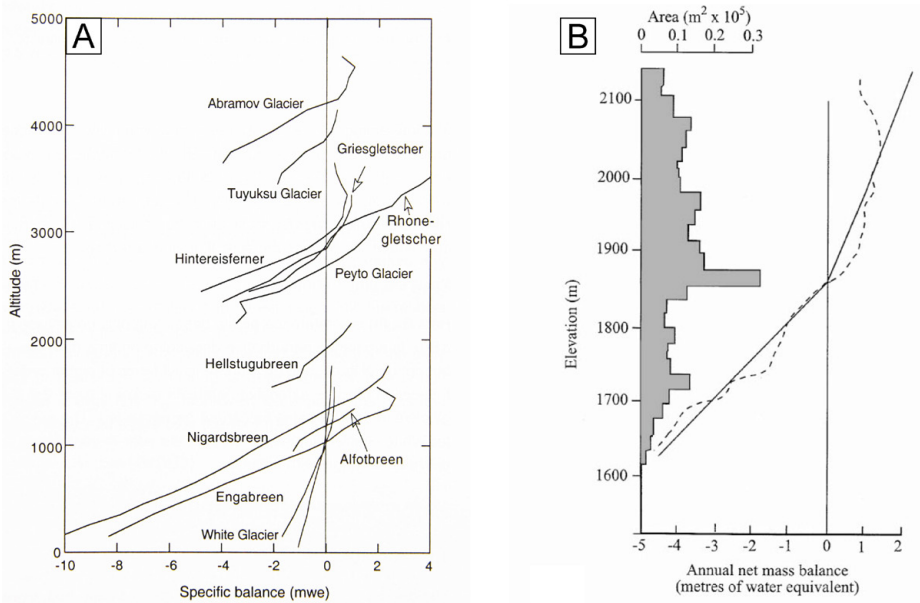
Fig. 2.2. (A) Gradients de bilans de masse de glaciers appartenant à différentes régions climatiques. Les gradients les plus forts sont ceux des glaciers maritimes. Noter les différences d'altitude des LEG (Oerlemans, 2001) ; (B) Gradient de bilan de masse moyen et son approximation avec un gradient linéaire, pour le South Cascade glacier (Chaîne des Cascades, USA). Le gradient est plus important dans la zone d'ablation (Meier et Tangborn, 1965). Dans les deux cas les données de bilans de masse sont des moyennes sur plusieurs années.
