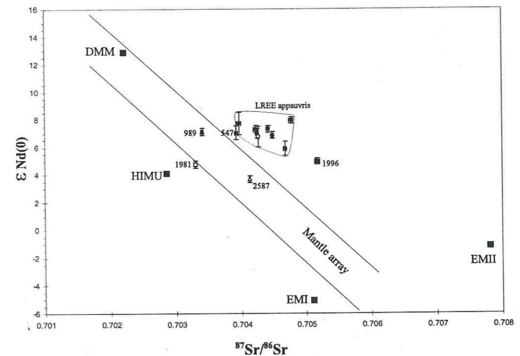
Figure 3-15 : Signature isotopique \epsilon Nd(0) versus 87 Sr/ 86 Sr de tous les niveaux pyroclastiques analysés en éléments traces. (pour la définition des réservoirs, se référer à la note n°19, valeurs Hart et al., 1992).
