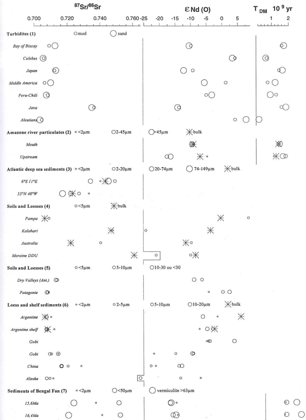
Figure 4-21 : Compositions ^{87}\text{Sr}/^{86}\text{Sr} , \epsilon \text{Nd} (0) et âge modèle ( T_{\text{DM}} ) en fonction de la granulométrie dans différents environnements détritiques. (1) McLennan et al., 1989, 1990 ; (2) Goldstein et al., 1984 ; (3) Dasch, 1969 ; (4) Grousset et al., 1992 ; (5) Grousset, communication personnelle ; (6) Revel et al., en préparation ; (7) Derry et France Lanord, 1996.
