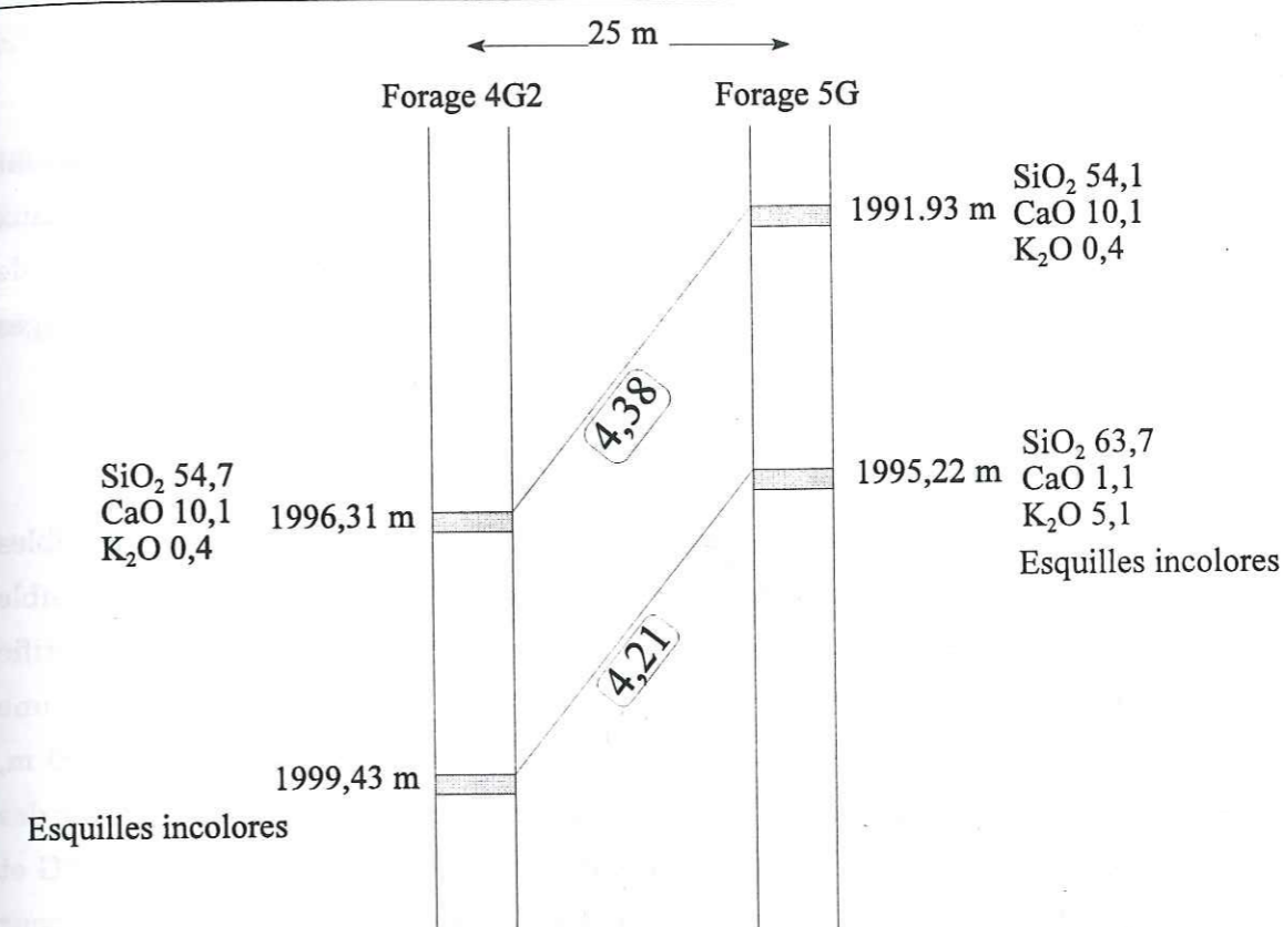
Figure 3-33 : Schématisation du décalage des profondeurs des couches de cendres (en grisé) entre les forages 4G2 et 5G (espacés de 25 m), entre 1990 et 2000 m. Les compositions des couches Si, Ca et K sont données en % poids d'oxyde. Le décalage entre les deux forages est de 4,38 m pour la couche supérieure et 4,21 m pour la couche inférieure.
