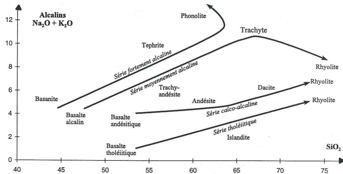
Figure 3-2 : Exemple de classification chimique des laves montrant les évolutions des différentes lignées magmatiques et le nom des laves qu'elles produisent (reproduit d'après Briot, 1995).
