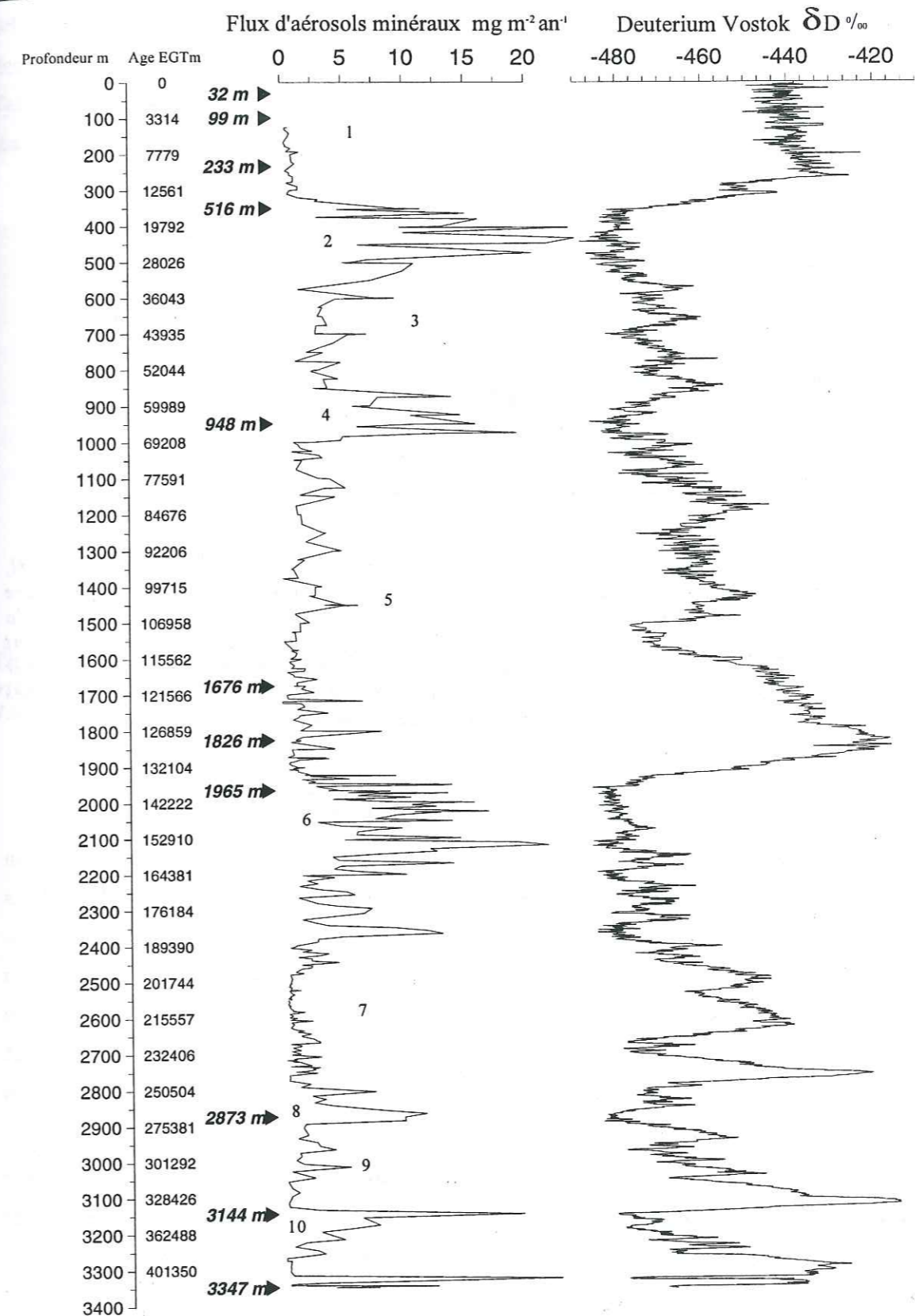
Figure 4-14 : Profils de composition en Deutérium et flux de poussières jusqu'à 3347 m de profondeur (non publiés). Les pointes de flèche indiquent les profondeurs d'échantillonnage. 516 m a été prélevé à Dôme C : il est replacé sur la courbe de Vostok à un âge équivalent. Les flux sont calculés à partir de la concentration en poussières (mesurée au coultre), d'une densité d=2,65 et de l'accumulation utilisée dans EGTm.
