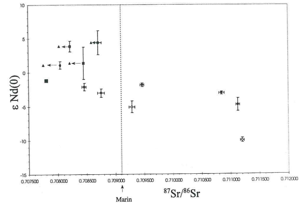
Figure 4-18 : Représentation graphique de la correction consecutive à la contamination par \text{Sr}_{\text{marin}} pour les échantillons mesurés à Toulouse. Triangles noirs : valeurs corrigées ; pour les autres symboles, se référer à la Figure 4-16.
