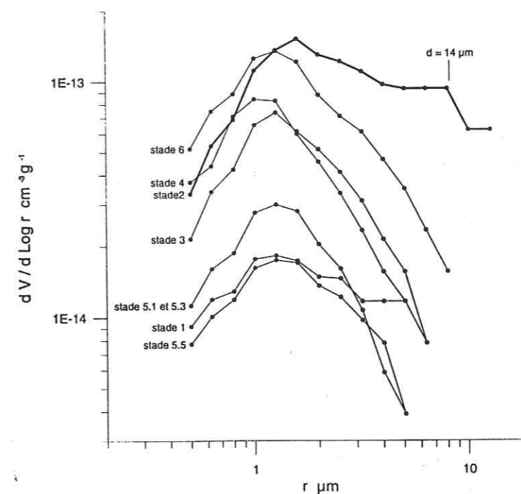
Figure 4-6 : Moyenne par stade de la distribution en volume des aérosols minéraux déposés à Vostok. Les stades 2, 4, et 6 représentent les périodes glaciaires, les stades 1, 3 et 5 les périodes interglaciaires. (données : Mounier, 1988).
