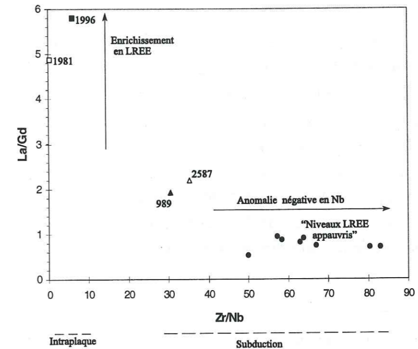
Figure 3-14 : La/Gd versus Zr/Nb de tous les niveaux pyroclastiques analysés en éléments traces. (547 m n'est pas représenté car Nb non mesuré).
