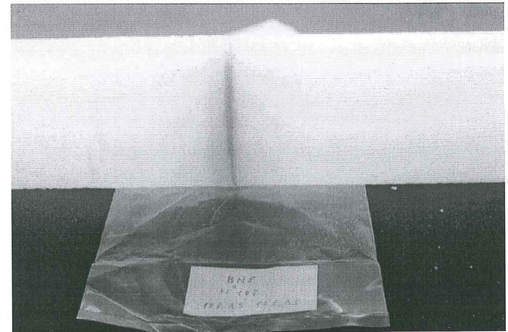
Figure 3-3 : Photographie de la couche de cendres volcaniques située à 102,70 m dans le forage BH. Le diamètre de la carotte est de 10 cm. La couche la plus concentrée (à droite) est située vers le bas. (Photographie E. Lefèvre).
