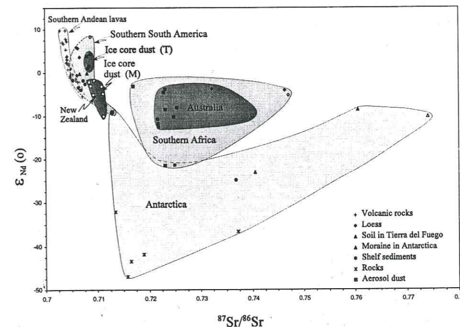
Figure 4-15 : \epsilon \text{ Nd} (0) versus ^{87}\text{Sr}/^{86}\text{Sr} de l'ensemble des poussières et des PSAs mesurés. (identique à la Figure 4-11 avec les nouveaux points mesurés). (T) :Toulouse, (M) : Mayence.
