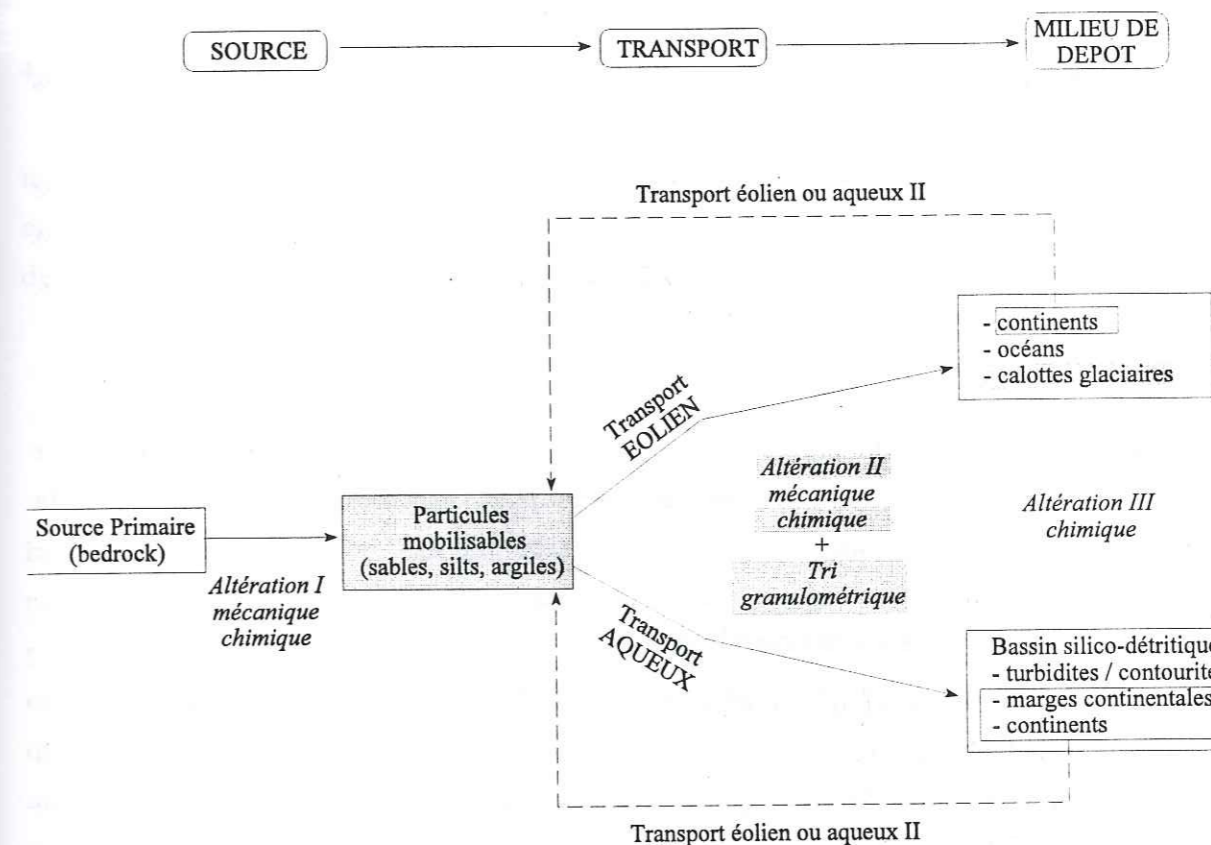
Figure 4-20 : Schéma du cycle formation / transport / sédimentation du matériel déritique issu de l'érosion des continents. Altération I : primaire ; II : secondaire ; III : tertiaire. Les étapes en grisé représentent les problématiques directes de notre étude.
