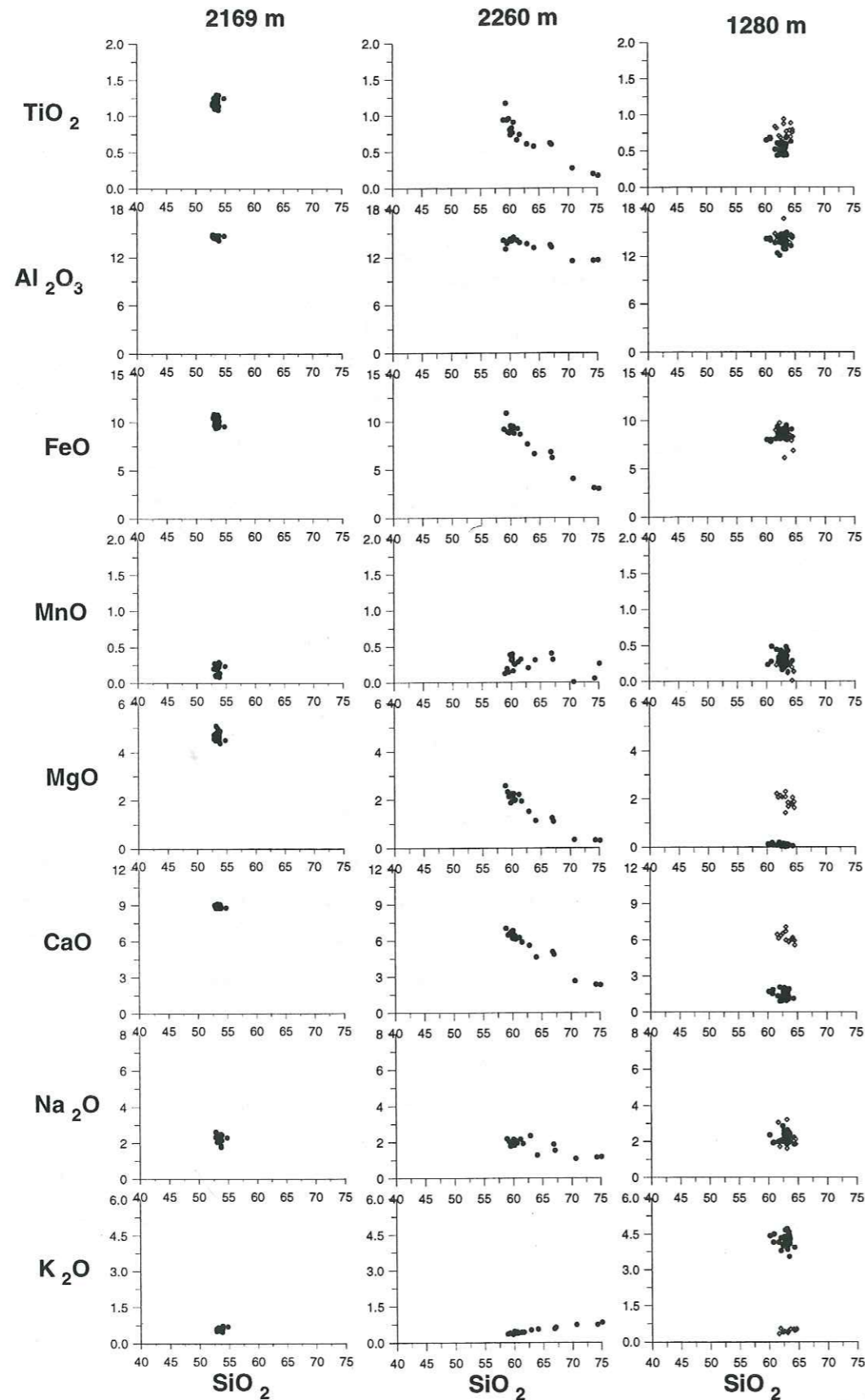
Figure 3-8 : Diagrammes de Harker pour l'horizon à 2169 m (20 verres analysés), l'horizon à 2260 m (20 verres analysés), et l'horizon à 1280 m (47 compositions de verres analysés). Cercles pleins : trachyte ; losanges ouverts : dacite andésitique.
