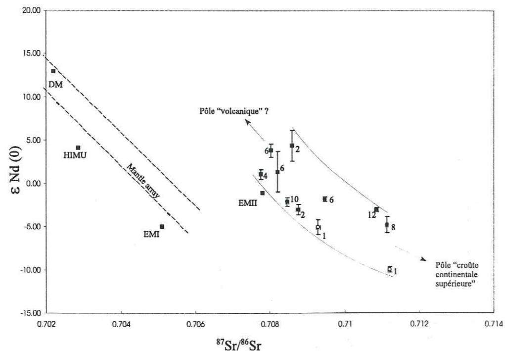
Figure 4-19 : \epsilon Nd(0) versus ^{87}Sr/^{86}Sr de l'ensemble des poussières analysées. Modélisation par une hyperbole de mélange entre un pôle « volcanique » et un pôle « croûte continentale supérieure ». Les valeurs en Sr des poussières mesurées à Toulouse sont corrigées de la contribution en Sr marin. L'incertitude en ^{87}Sr/^{86}Sr pour ces 4 points n'est pas reportée. On se reportera à la note de bas de page N°19, pour la définition des réservoirs théoriques.
