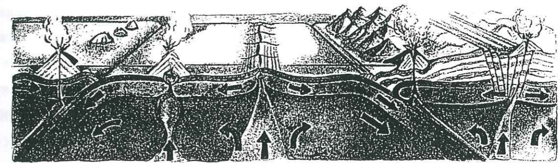
Zone de subduction océan/océan : volcanisme d'arc insulaire (Antilles) Point chaud : volcanisme intraplaque océanique (Hawaii, La Réunion) Zone d'expansion : volcanisme des dorsales océaniques Zone de subduction continent/océan : volcanisme de cordillère (Amérique du Sud) Volcanisme associé à un rift intracontinental (Afrique orientale). Cette situation est celle du Massif Central français.
