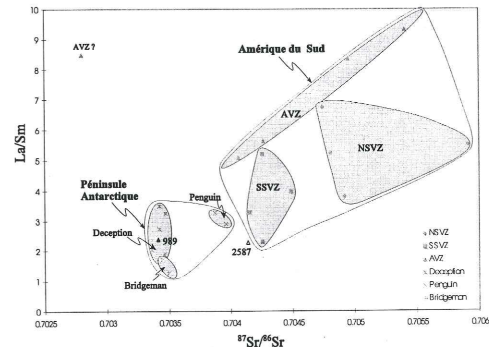
Figure 3-28 : La/Sm versus ^{87}\text{Sr}/^{86}\text{Sr} pour les PSVs de la péninsule Antarctique et de l'Amérique du Sud. (Amérique du Sud, Futa et Stern, 1988 ; Péninsule Antarctique, Weaver et al., 1979). Le point noté AVZ ? a été reporté mais il est isolé de la tendance définie par les autres volcans de la SVZ 17 .
