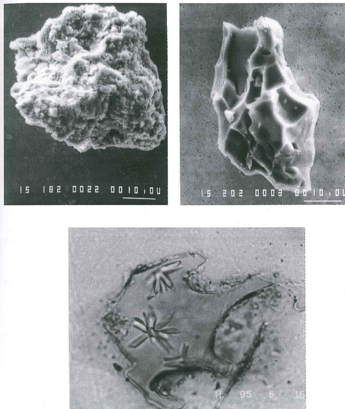
Figure 3-4 : Photographies de tephra a) matériel lithique, b) esquille de verre (microscope électronique à balayage) c) microlithes (microscope optique, lumière transmise, surface polie).
