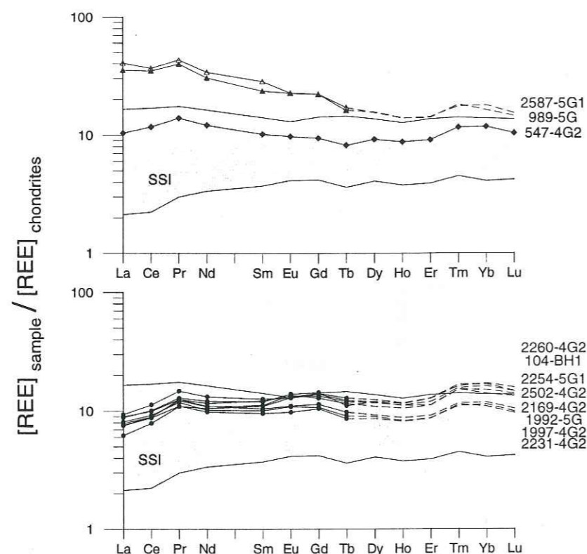
Figure 3-26 : Profils en REE pour les SSI (Pearce et al., 1995), et pour les niveaux 104, 1992, 1997, 2169, 2231, 2254, 2260 et 2502 m (« LREE appauvris »), 547, 989 et 2587 m.
