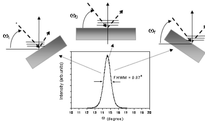
Figure II-5 : Représentation schématique du principe de mesure de la "rocking curve". Les cristaux sont successivement éclairés en fonction de leur désorientation par rapport à la normale à la surface de l'échantillon
