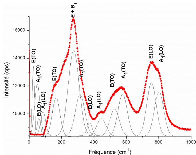
Figure II-13. Le spectre Raman de la cible PMN-PT 65/35 dopé 10%M. PbO après frittage (Les modes à haute fréquence sont simulés par le logiciel Wire 3.0. Les 4 modes à basse fréquence sont ajoutés suivant la définition des modes par A. Kania en 2006).
