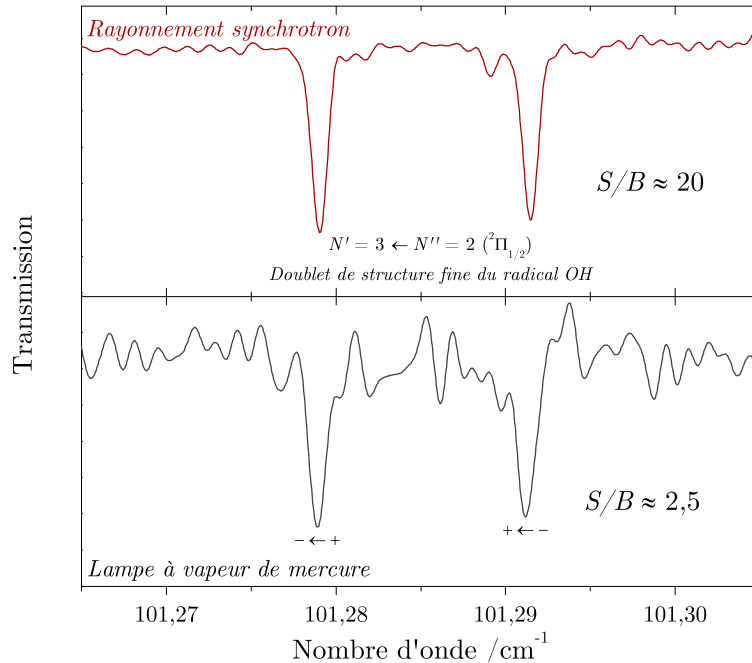
FIGURE 3.6 – Comparaison entre les spectres d’absorption du radical OH obtenus en post-décharge avec le rayonnement synchrotron (en haut) et une source classique (en bas). Les deux spectres ont été enregistrés dans les mêmes conditions expérimentales ( 2h30 d’acquisition / R=0,001\text{ cm}^{-1} ).
