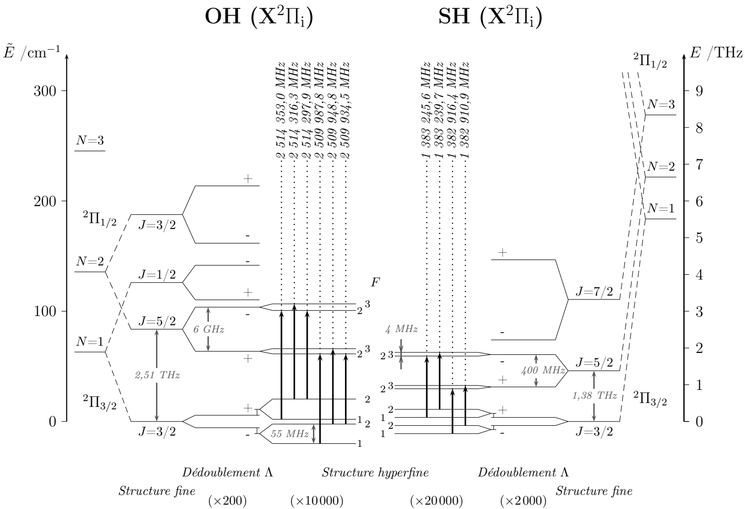
FIGURE 3.7 – Diagramme comparatif des niveaux d'énergie des radicaux OH et SH. Les transitions dans l'état ^2\Pi_{3/2} enregistrées au cours de ce travail par technique cw-THz sont représentées.
