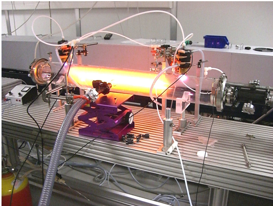
FIGURE 3.11 – Représentation schématique de la cellule à colonne positive et photographie du plasma créé (ici décharge dans N_2 ). La zone orangée est la colonne positive du plasma qui est sondée dans cette expérience. On distingue également sur cette photo la lueur négative de ce plasma (halo rose sous la cathode).
