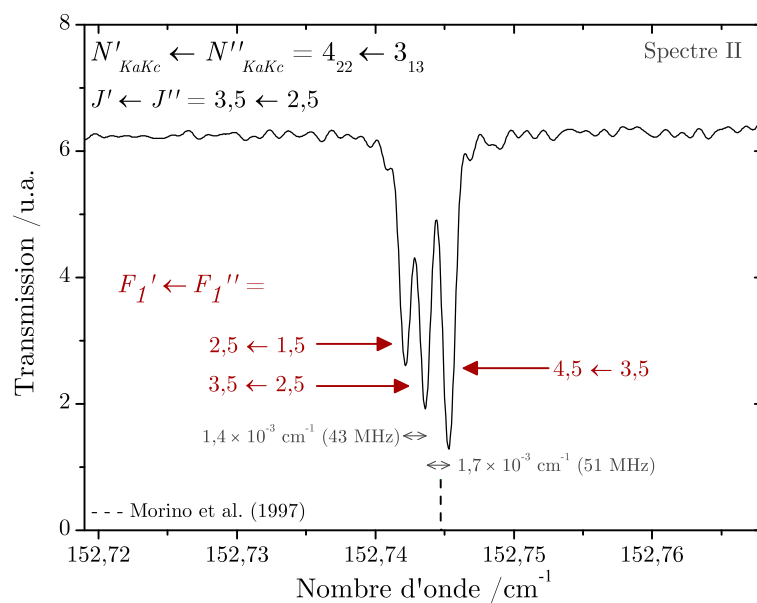
FIGURE 3.20 – Observation de la structure hyperfine due au spin nucléaire de l'atome d'azote dans l'état vibrationnel fondamental de ^{14}\text{NH}_2 (nombre d'onde précédemment reporté dans la littérature indiqué par des tirets).
