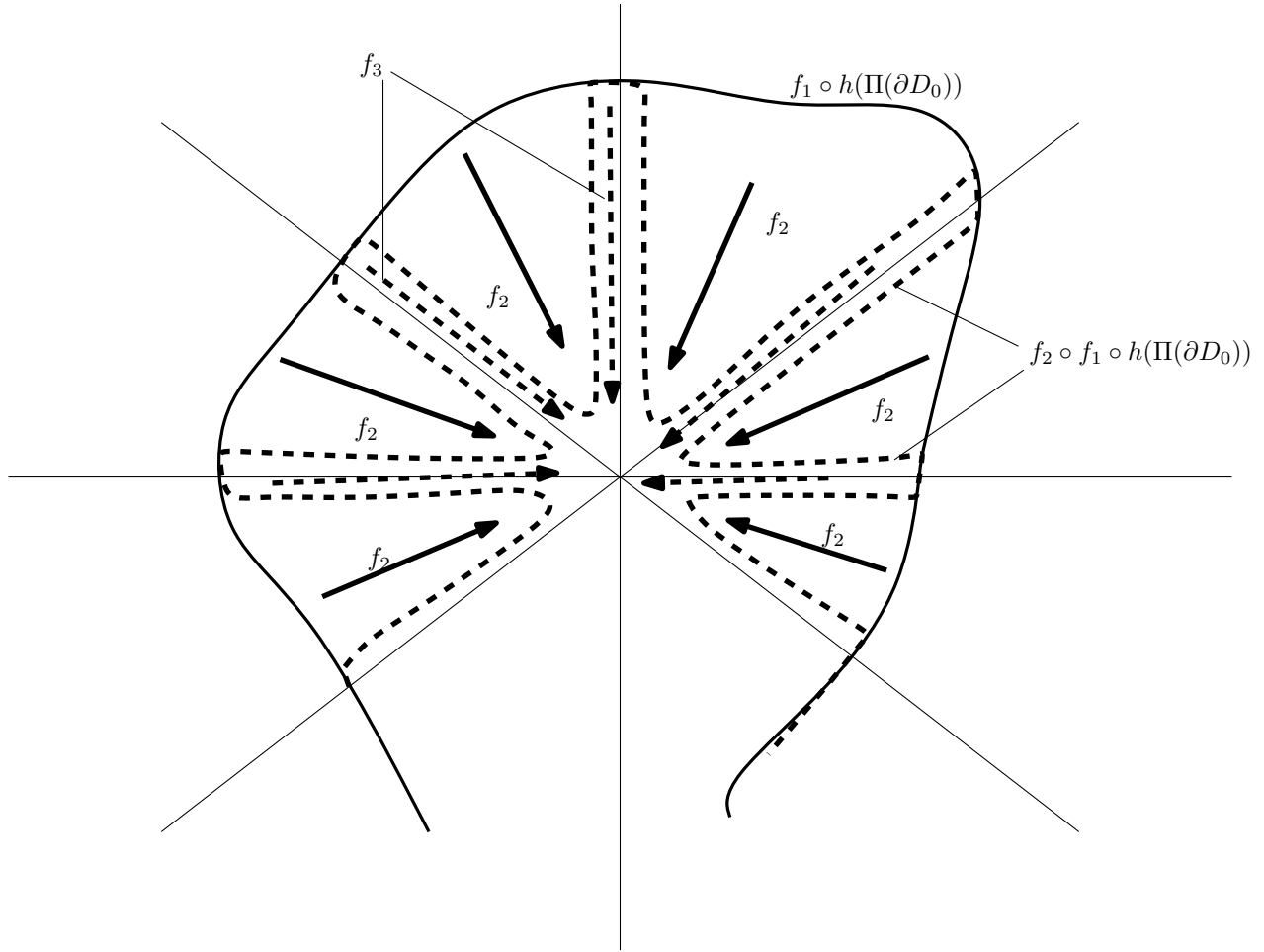
FIGURE 6.12 – Illustration de la preuve du lemme 6.38
