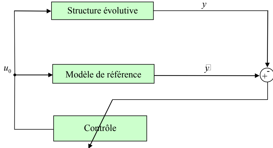
Figure 1.11 Asservissement des paramètres de contrôle à partir de la différence « réponse de la structure contrôlée y / réponse du modèle contrôlé \bar{y} »
