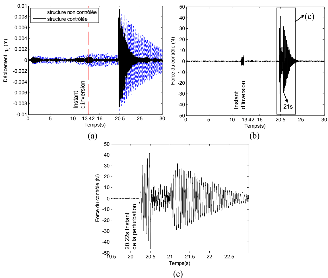
Figure 4.17 Contrôle avec identification systématique avec perturbation et bruit environnemental \nu , RSB=63dB (Vitesse de la masse mobile fixée à 3.6 mm/s)
