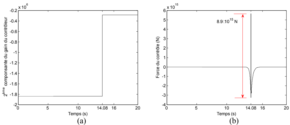
Figure 2.19 Effet d'un changement brutal du contrôle 2^{\text{ème}} composante du gain du contrôleur, (b) force du contrôle
