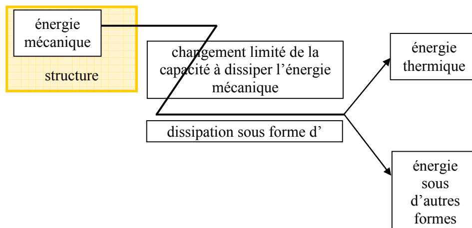
Figure 1.5 Conversion d'énergie du contrôle semi-actif par la modification de l'amortissement
