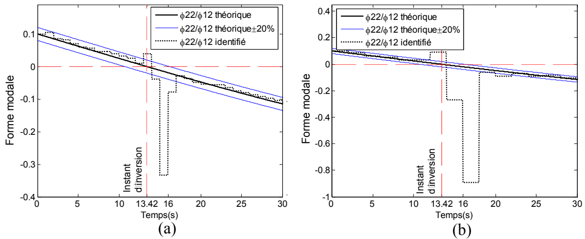
Figure 4.8 Caractéristiques modales identifiées avec deux longueurs de fenêtre d'identification : (a) fenêtre de 1s et (b) fenêtre de 2s (Pas de perturbation ni bruit environnemental \nu )
