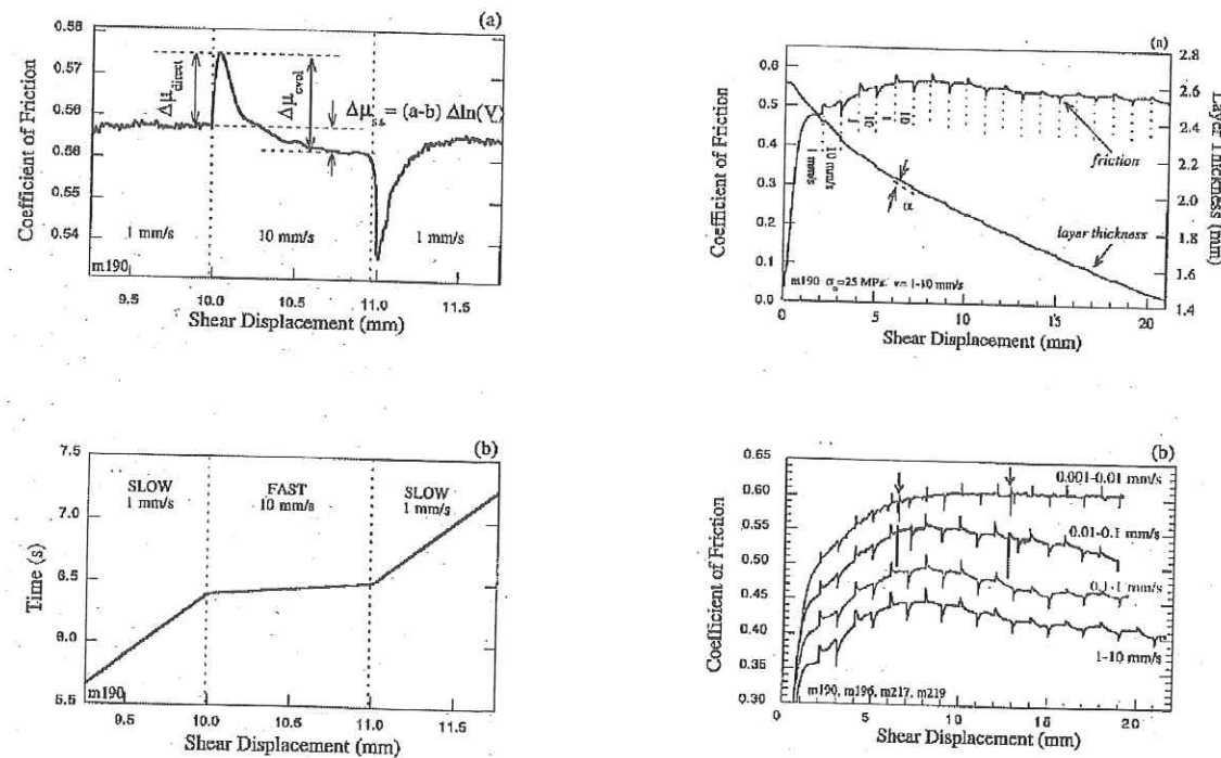
FIG. 1.2 – Le comportement d'une gouge artificielle sollicitée par une vitesse de glissement constante par palier, d'après Mair & Marone (1999). A gauche: le détail du comportement pour une petite sollicitation. A droite: l'évolution globale après une série de petites sollicitations.
