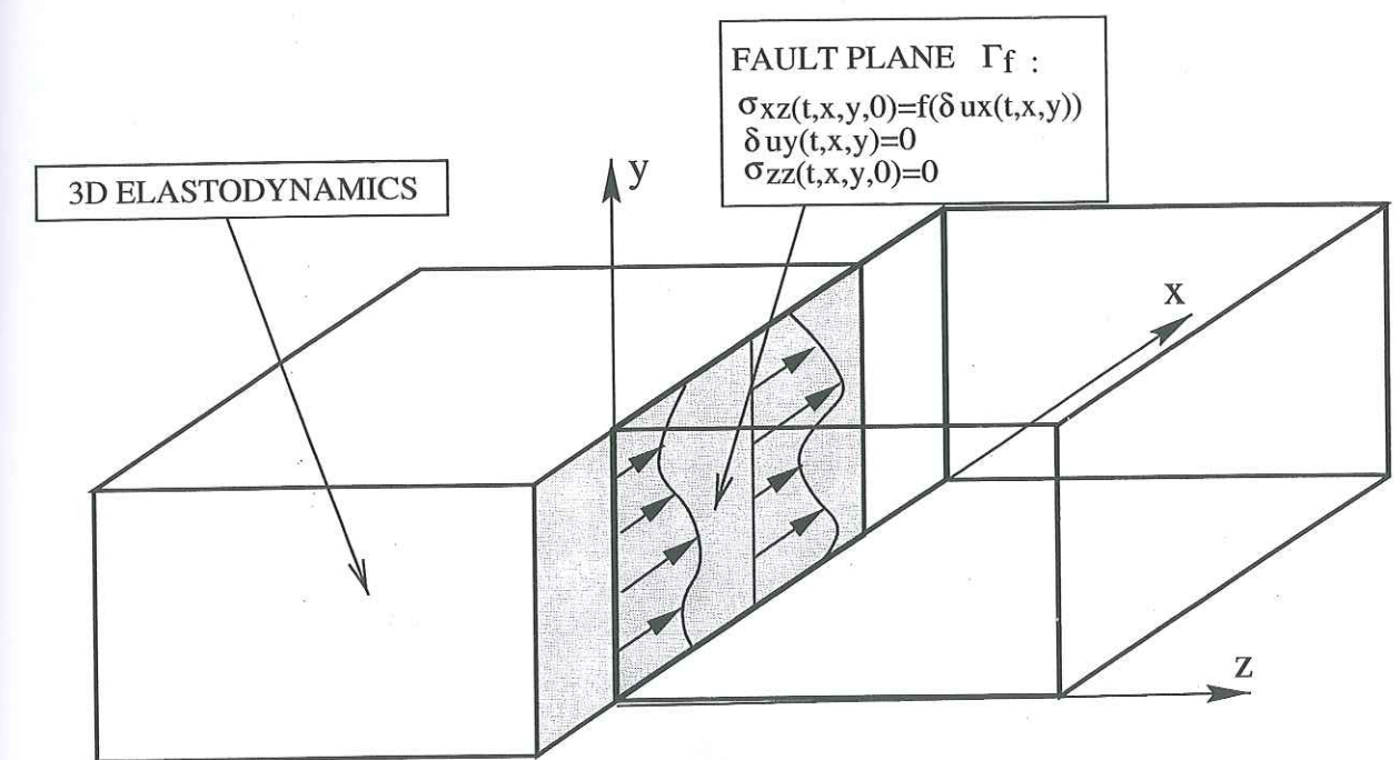
FIG. 3.15 – La géométrie du strike-slip vertical.
