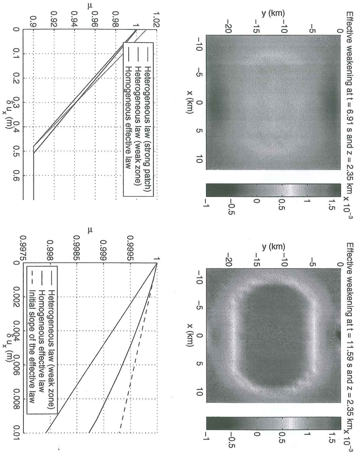
FIG. 4.12 - Le taux d'affaiblissement dans le milieu élastique et la loi de frottement effective.
