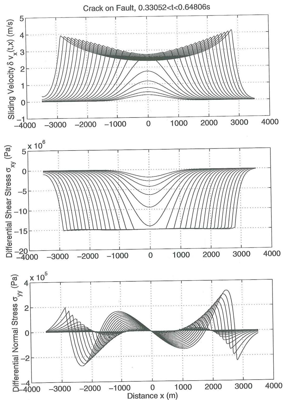
FIG. 2.36 – Crack sur la faille dans le cas homogène. En haut: la vitesse de glissement \delta v_x(t, x, 0) . Au milieu: la contrainte de cisaillement \sigma_{xy}(t, x, 0) - \sigma_{xy}(0, x, 0) différentielle par rapport au temps initial. En bas: la contrainte normale \sigma_{yy}(t, x, 0) - \sigma_{yy}(0, x, 0) différentielle par rapport au temps initial. La perte de symétrie en x est très peu visible dans ce cas homogène.
