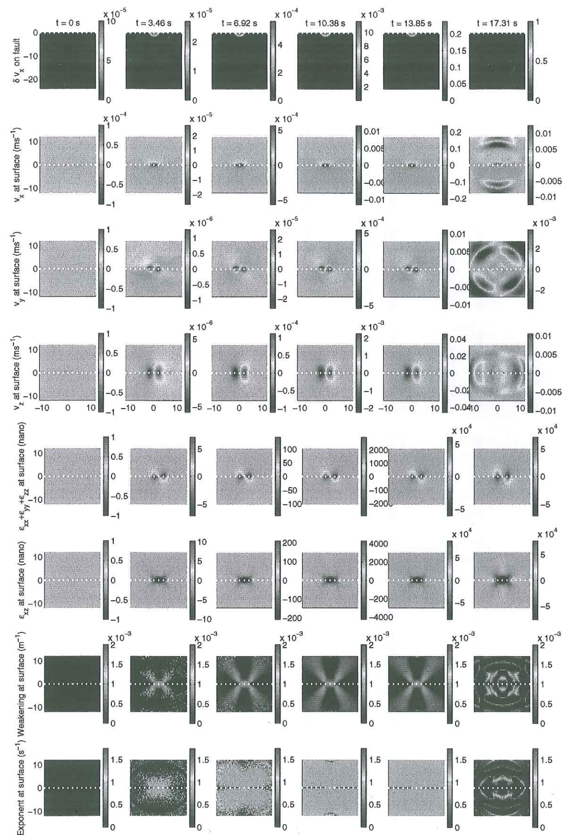
FIG. 3.17 – Cinématique en surface pour le patch lent à 0 km de profondeur. Première ligne: la demi-vitesse de glissement sur la faille. Puis de haut en bas la cinématique en surface: les trois composantes de la vitesse, les déformations volumique et cisailante et enfin l'affaiblissement effectif et l'exposant effectif.
