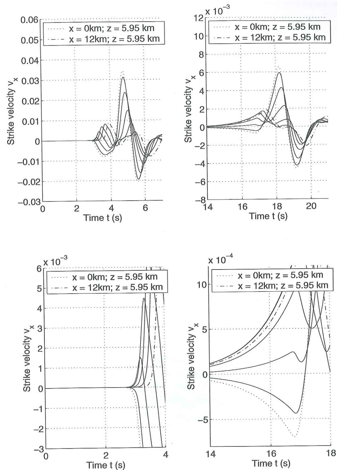
FIG. 3.28 – Quelques phases d'initiation typiques. A gauche: le patch rapide. A droite le patch lent. En haut: en pleine échelle. En bas: le zoom sur l'initiation. Dans les deux cas (rapide et lent), on observe que le processus d'initiation régularise la montée du signal. Dans les cas où x est grand, l'initiation a lieu avant le pulse des ondes P. Dans les cas où x est proche de 0, on se trouve dans une zone de radiation nulle pour le potentiel P. Dans ce cas c'est le champ proche qui produit la suite du signal.
