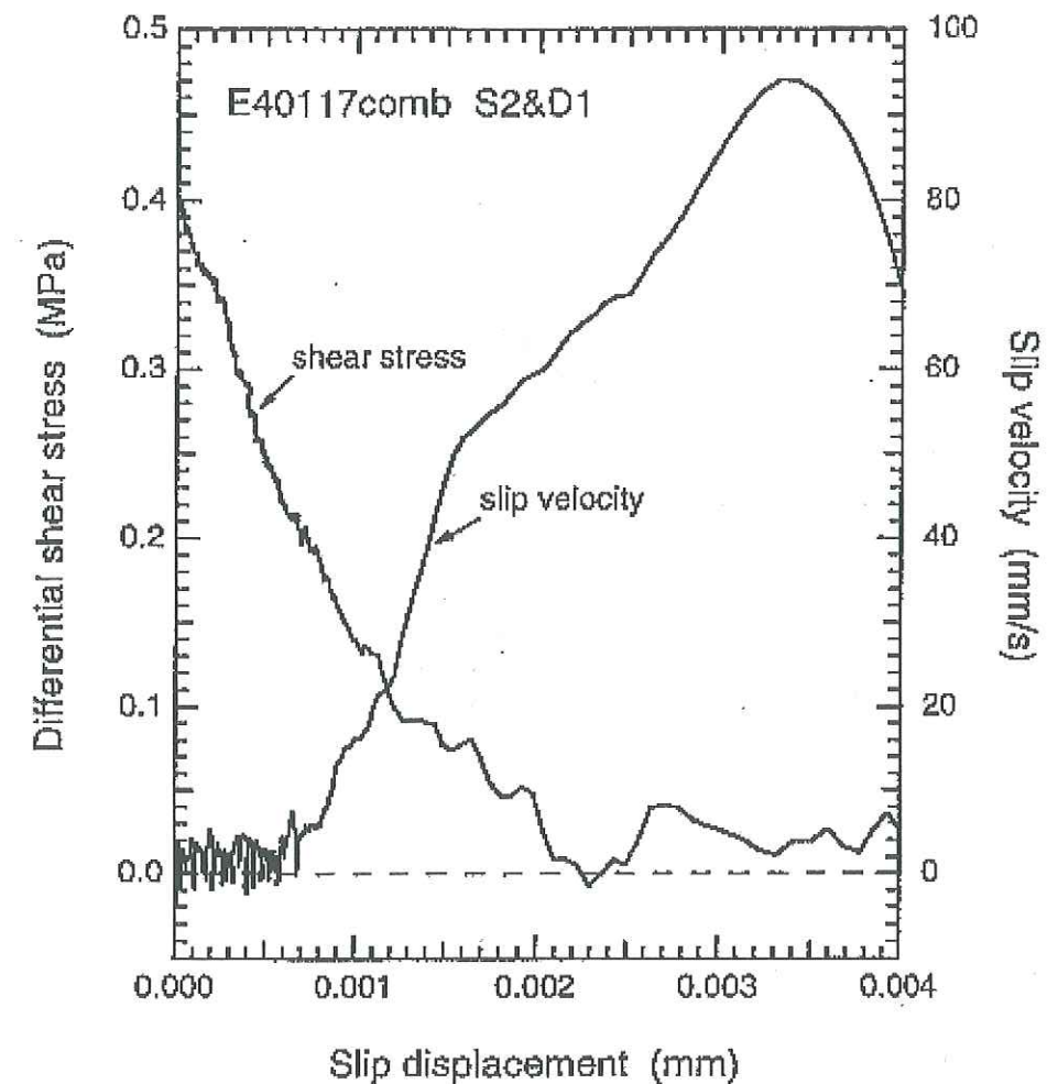
FIG. 1.5 – Le comportement typique obtenu à l'interface dans une expérience de Ohnaka & Shen (1999). Ce dernier se résume à une loi de frottement dépendante du glissement. Les trois principaux paramètres sont la résistance statique, la résistance dynamique et le glissement critique. Ici la chute de résistance est de 0.4MPa et le glissement critique est de 2\mu m .
