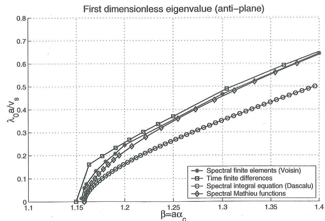
FIG. 2.24 – Problème antiplan. Représentation de la première valeur propre |\lambda_0|a/v_s en fonction de \beta = \alpha\alpha_c calculée par différentes méthodes: Spectre en éléments finis par Voisin et al. (2000), spectre extrait des différences finies en temps, spectre de l'équation intégrale par Dascalu et al. (2000) et spectre en coordonnées elliptiques et fonctions de Mathieu. En bas: zoom près du point critique.
