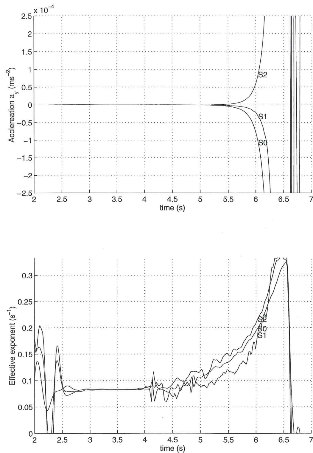
FIG. 3.33 – Les caractéristiques du signal en champ proche à la surface. En haut: l'accélération verticale sur trois récepteurs. On observe quelques irrégularités du signal (brises de pente et ressauts). En bas: l'exposant effectif, la seule quantité capable de mesurer l'évolution du taux d'instabilité du processus d'initiation hétérogène.
