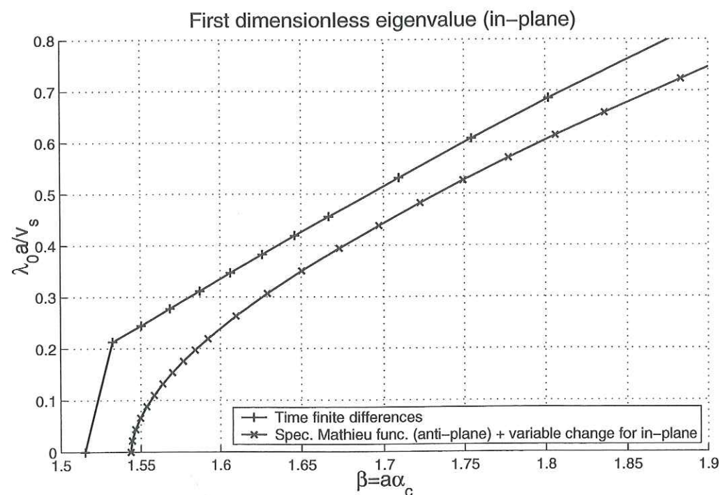
FIG. 2.27 — Problème plan. Représentation de la première valeur propre |\lambda_0|a/v_s en fonction de \beta = \alpha_c pour v_p/v_s = \sqrt{3} , calculée par deux méthodes: Spectre extrait des différences finies en temps et changement de variables dans le problème antiplan, résolu en coordonnées elliptiques et fonctions de Mathieu (méthode non valable loin du point critique!). En bas: zoom près du point critique.
