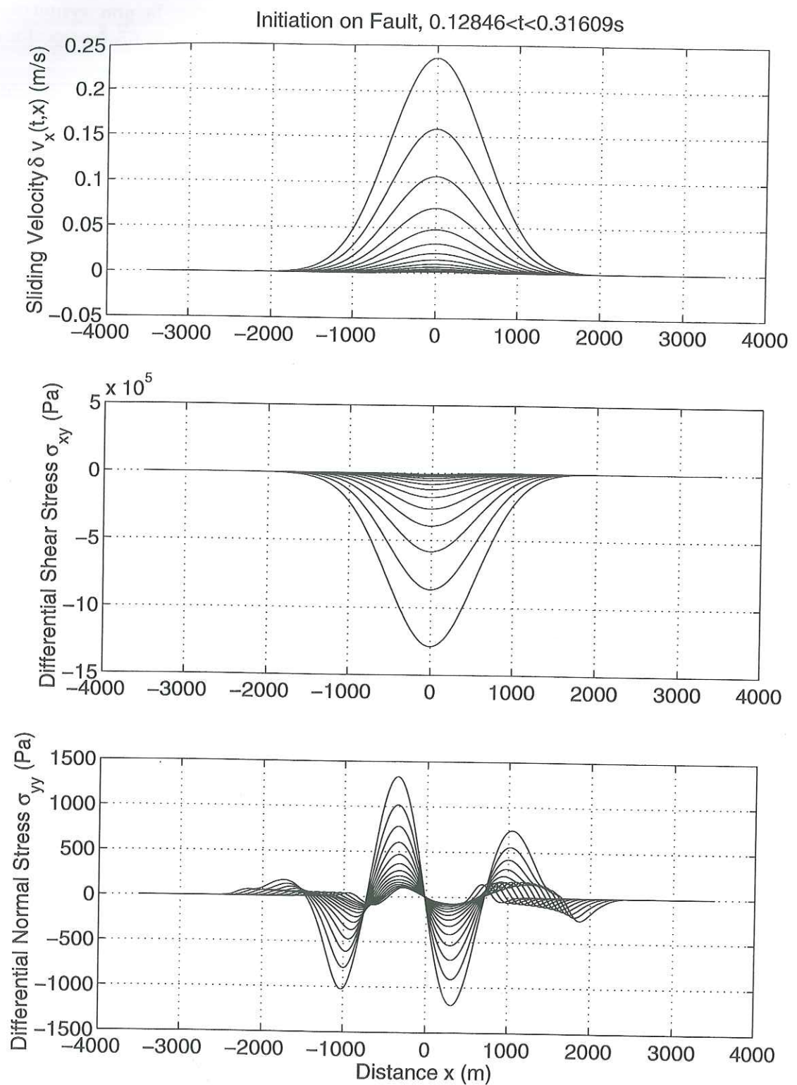
FIG. 2.35 – Initiation sur la faille dans le cas homogène. En haut: la vitesse de glissement \delta v_x(t, x, 0) . Au milieu: la contrainte de cisaillement \sigma_{xy}(t, x, 0) - \sigma_{xy}(0, x, 0) différentielle par rapport au temps initial. En bas: la contrainte normale \sigma_{yy}(t, x, 0) - \sigma_{yy}(0, x, 0) différentielle par rapport au temps initial. La perte de symétrie en x est quasiment nulle.
