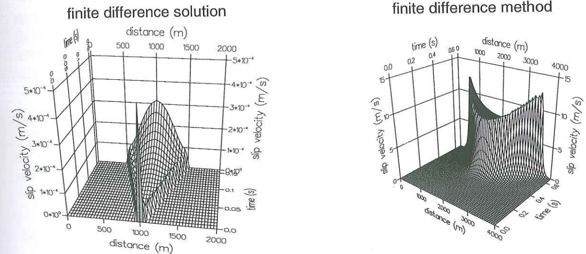
FIG. 2.3 – Le processus instable sur la faille infinie, calculé par une méthode de différences finies d'après Campillo & Ionescu (1997). A gauche: le processus d'initiation. A droite: la fin du processus d'initiation et le début de la phase de crack. Ici les valeurs numériques sont: \rho = 3000 \text{ kg m}^{-3} , v_s = 3000 \text{ m s}^{-1} , L_c = 0.05 \text{ m} et \sigma_s - \sigma_d = 12 \text{ MPa} . La perturbation initiale sur la vitesse a une amplitude maximale de 0.0001 \text{ m s}^{-1} et une extension caractéristique de 100 \text{ m} .
