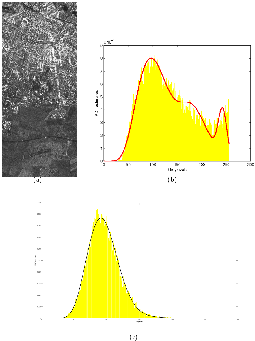
FIG. 3.4 – (a) : Image RSO originale de Amiens (France) (COSMO-SkyMed, ©ASI) ; (b) : Histogramme de niveaux de gris (en jaune) et son approximation par la méthode proposée pour les zones urbaines (en rouge) (c) : Histogramme de niveaux de gris (en jaune) et son approximation par la méthode proposée pour les arbres (en noir).
