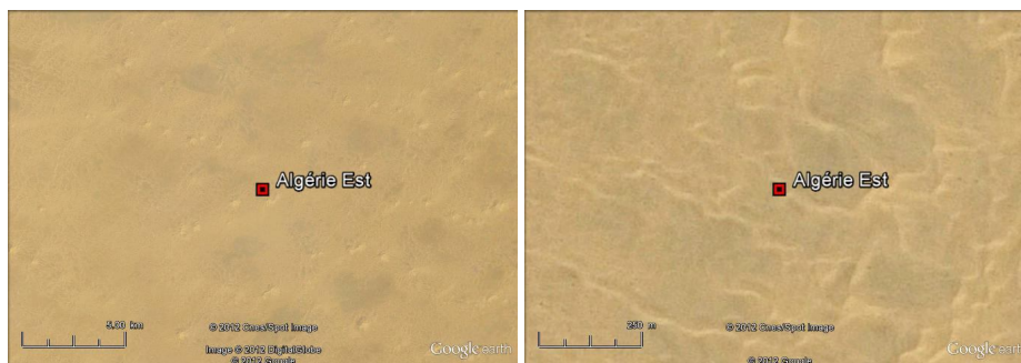
Figure 3.22 Idem figure 3.13 mais pour “Algérie Est”.
