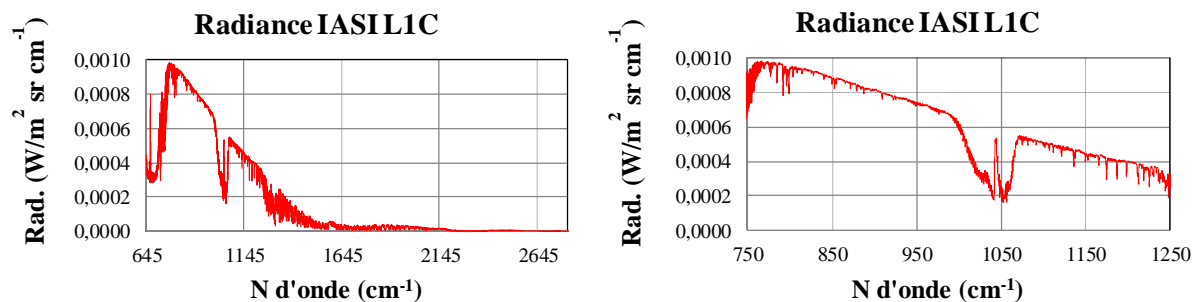
Figure 3.7 Exemple de données radiance IASI. A gauche l'intervalle spectral total de IASI et à droite la représentation comprise entre 750 et 1250 \text{cm}^{-1} .
