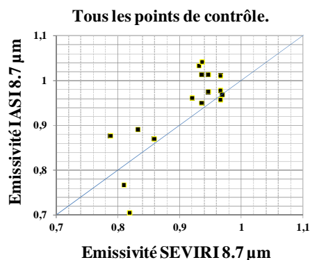
Figure 4.30 Validation émissivités IASI avec SEVIRI bande 7-IR (8.7 \mu\text{m} ).
