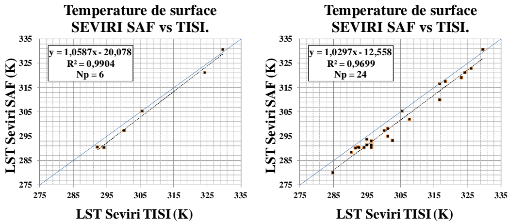
Figure 4.17 A gauche le 3 juillet ; à droite toutes les données TISI disponibles.
