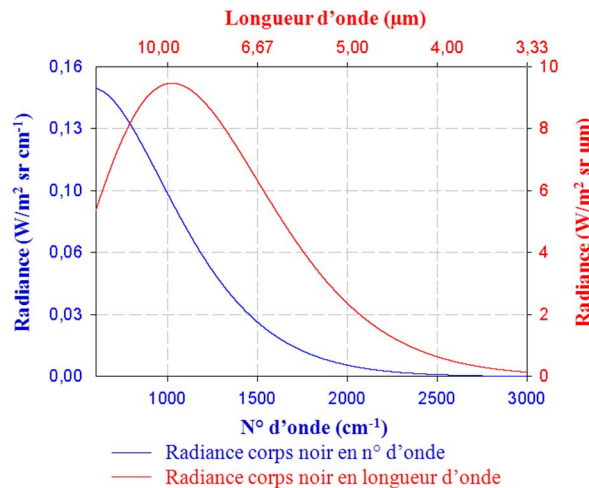
Figure 1.1 Radiance spectrale émise par un corps noir à 297 K ( W/m^2 sr cm^{-1} ).
