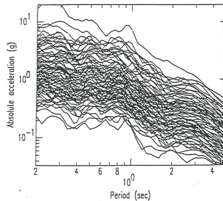
Figure II.29 : Réponse absolue en accélération, pour un amortissement de 5%, pour les 100 scénarios envisagés (Hutchings et al., 1996).
