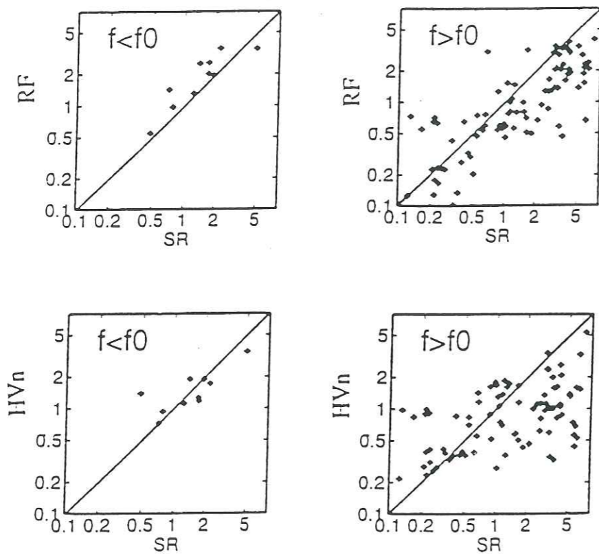
Figure 1.56 : Comparaison de l'amplification moyenne arithmétique à chaque site, pour les fonctions récepteur (RF) et les rapports H/V sur bruit de fond (HVn) avec celle obtenue pour les rapports spectraux classiques (SR), pour les fréquences inférieures ou supérieures à la fréquence de résonance du site.
