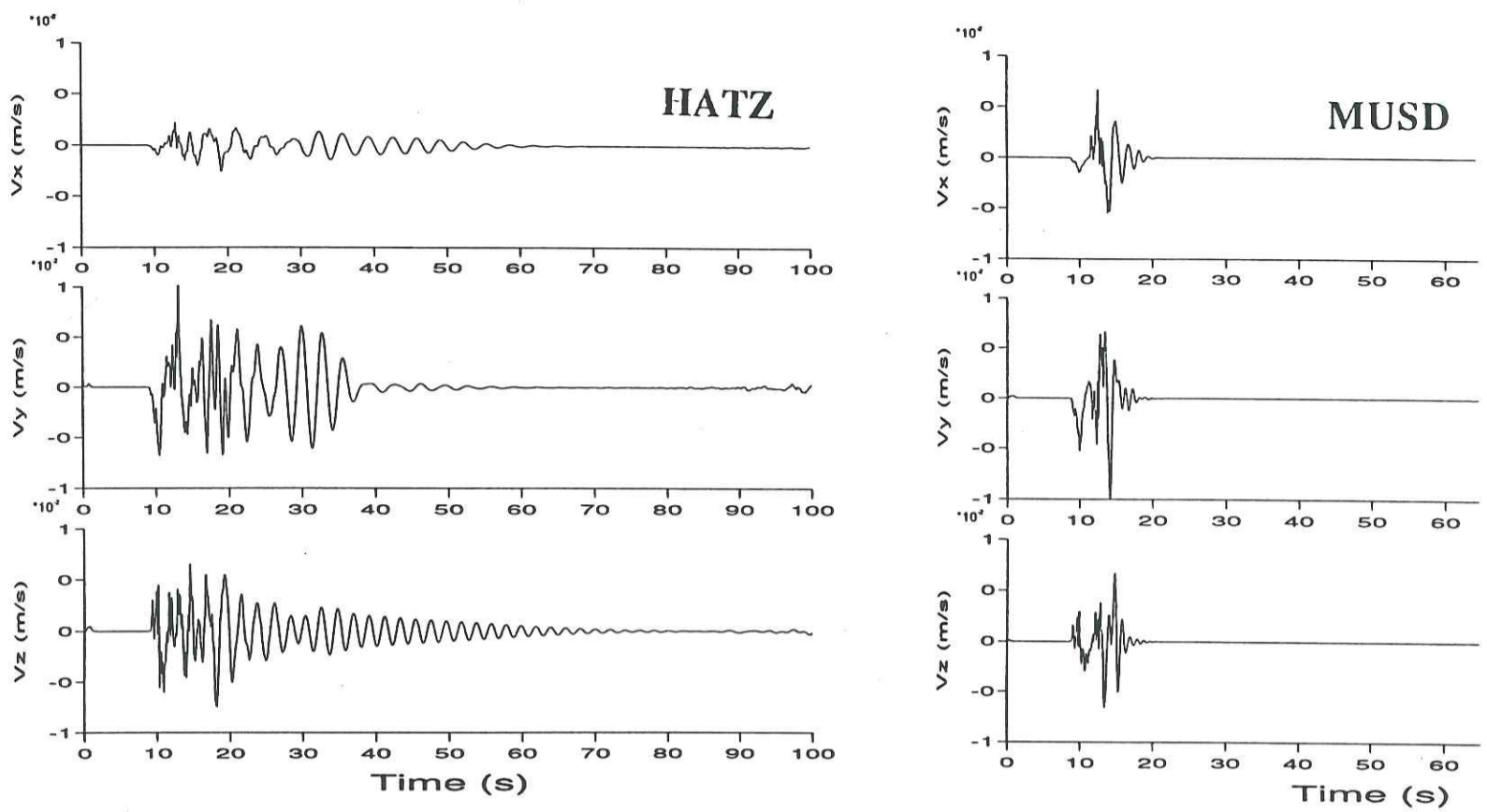
Figure 11.70 : Sismogrammes synthétiques en vitesse, obtenus avec la méthode utilisant une fonction de Green numérique, pour les sites HATZ (à gauche) et MUSD (à droite).
