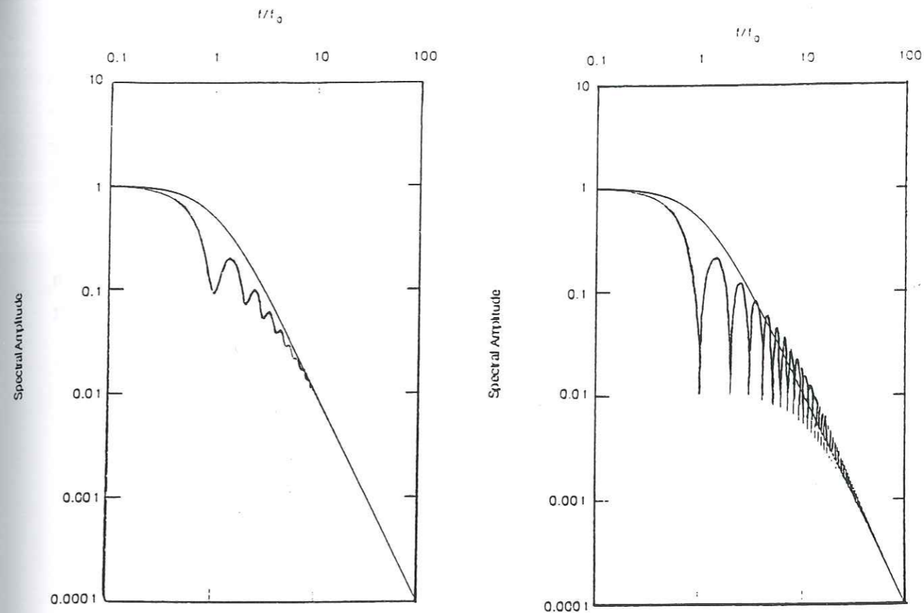
Figure II.28 : Spectre du mouvement simulé pour un rapport de magnitude de moment de une unité entre le séisme simulé et le fonction de Green (à gauche) et de deux unités (à droite). Le trait plus épais correspond dans les deux cas au spectre théorique en \omega^2 (Joyner et Boore, 1986).
