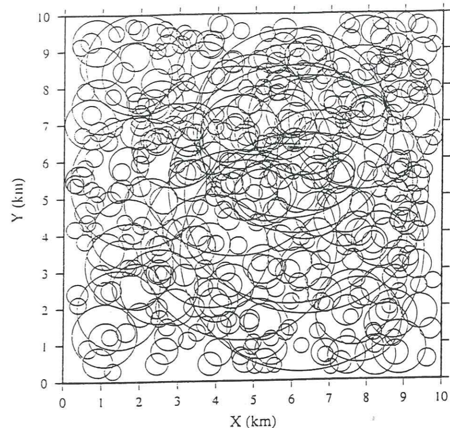
Figure II.31 : Exemple de distribution des sous-événements sur le plan de faille.
