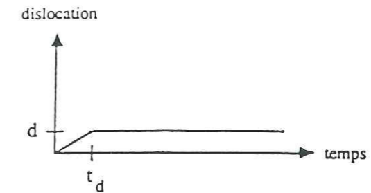
Figure II.5 : Schéma de la dislocation d , obtenue en un temps de montée t_d .
