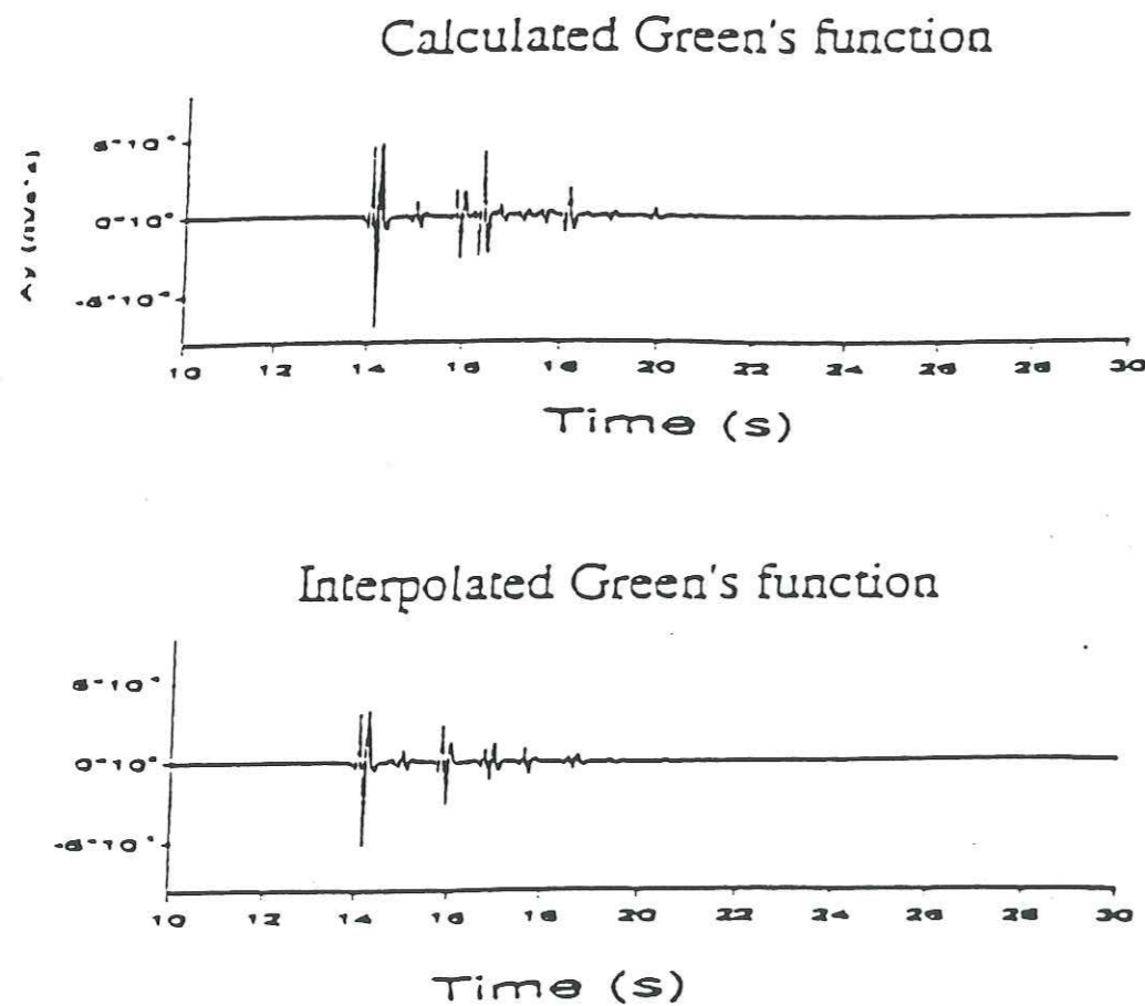
Figure II.35 : Comparaison entre une fonction de Green calculée (en haut) et la fonction de Green interpolée au même point (en bas).
