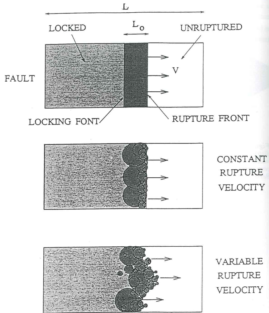
Figure II.21 : Haut : temps de montée et vitesse de rupture constants ; milieu : temps de montée dépendant de la taille des sous-événements et vitesse de rupture constante ; bas : temps de montée dépendant de la taille des sous-événements et vitesse de rupture variable (Bernard et al., 1996).
