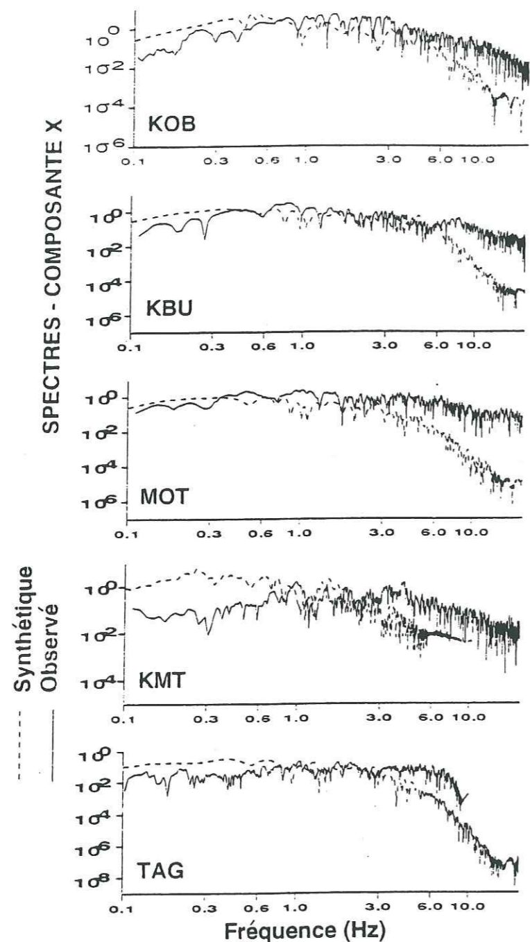
Figure II.57 : Comparaison entre les spectres de l'accélération observés et synthétiques pour les différents sites de Kobe.
