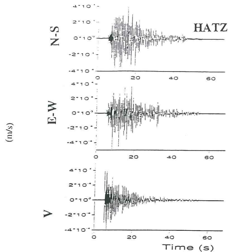
Figure II.60 : Enregistrement du séisme de Lancey, utilisé comme fonction de Green empirique, au site HATZ.
