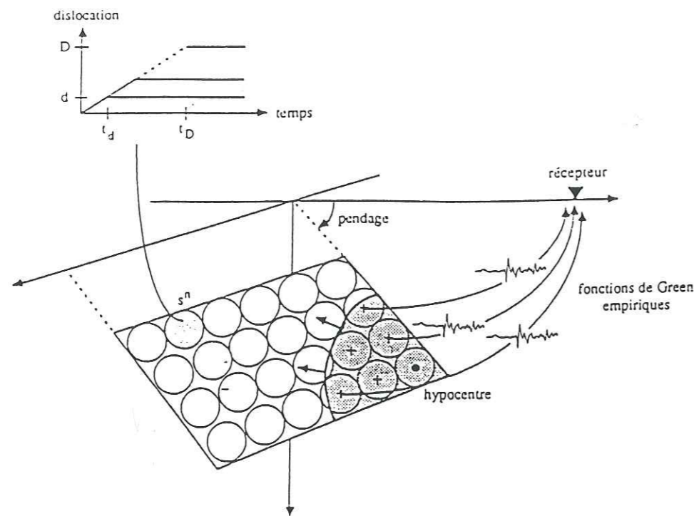
Figure II.1 : Différentes contributions aux décalages temporels entre les fonctions de Green empiriques : la montée de la dislocation, la propagation de la rupture et la propagation des ondes (Bour, 1993).
