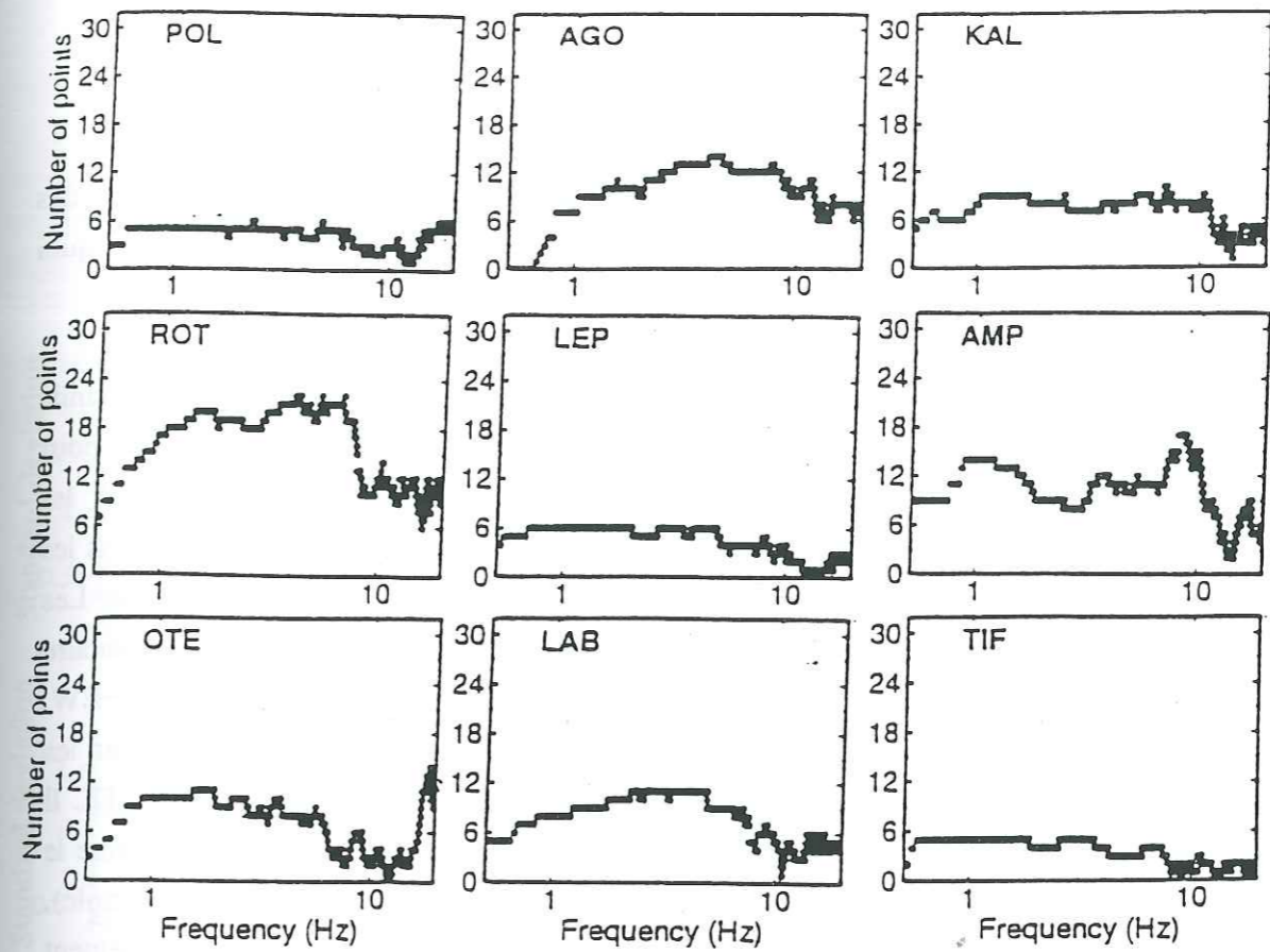
Figure 1.51 : Nombre de valeurs des fonctions récepteur disponibles à chaque fréquence pour chacun des sites.
