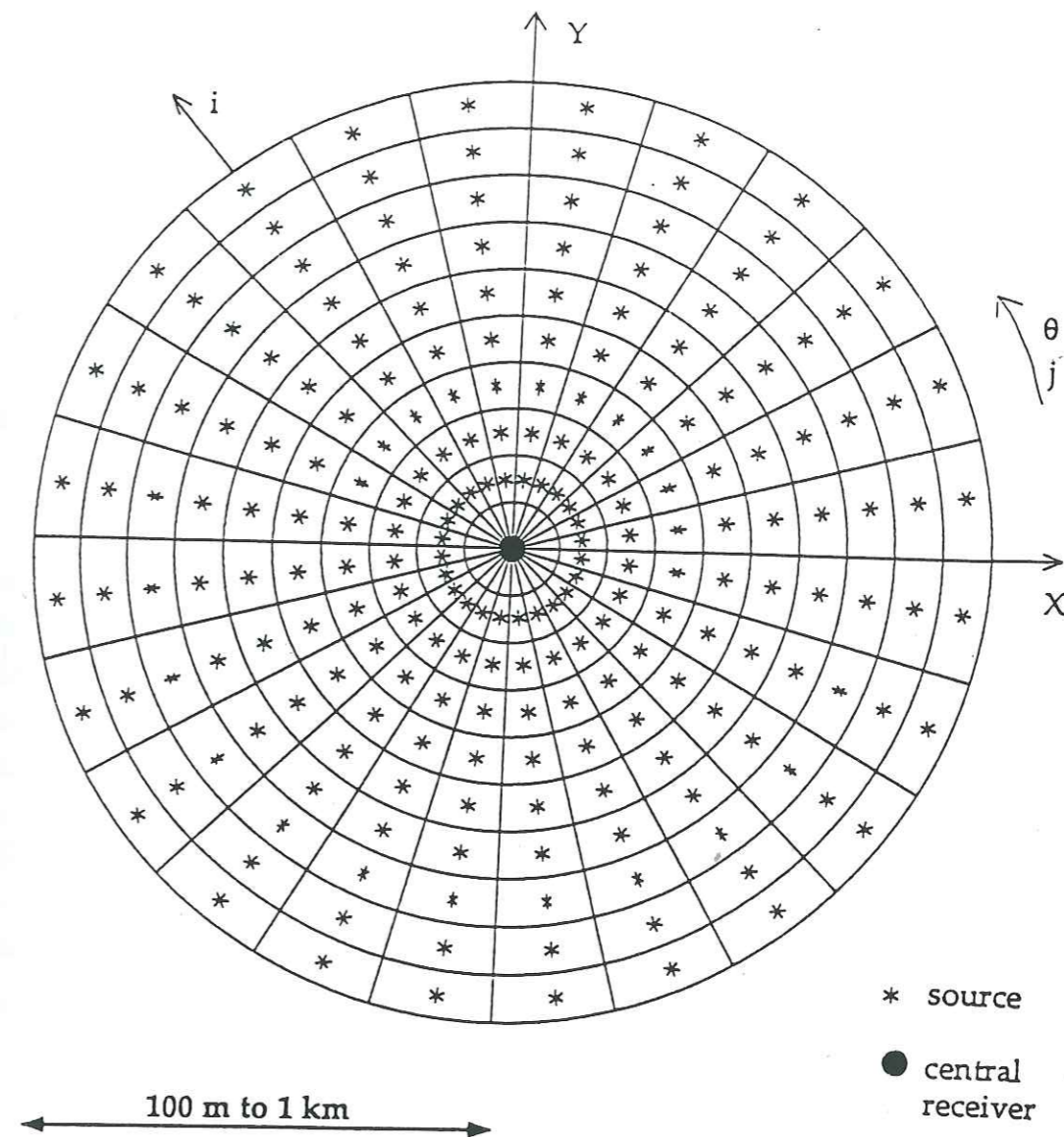
Figure I.22 : Modèle multi-sources utilisé pour les simulations de bruit de fond urbain.
