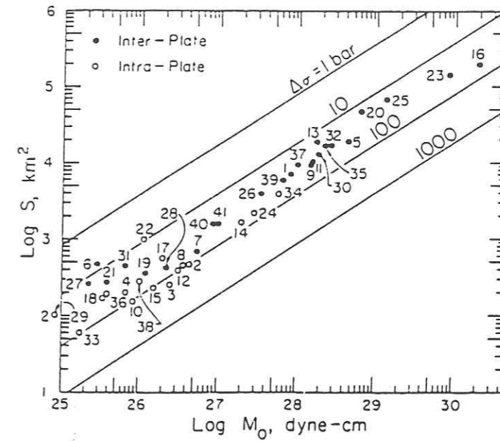
Figure II.3 : Relation entre la surface de faille S et le moment sismique M_0 . Les lignes indiquent la relation pour des failles circulaires avec une chute de contrainte constante ( \Delta\sigma ). Les numéros correspondent aux numéros des séismes utilisés (Kanamori et Anderson, 1975).
