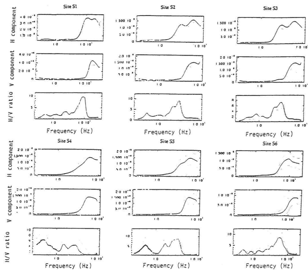
Figure 1.27 : Spectres obtenus pour les six structures théoriques. Lissage sur une échelle logarithmique, de largeur 0.1. Les pointillés indiquent l'écart type, pour 10 simulations de bruit différentes.
