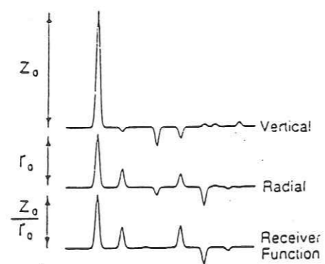
Figure 1.20 : Réponses verticale et radiale, et fonction récepteur correspondante, calculées pour une couche sur un demi-espace (Ammon, 1991).
