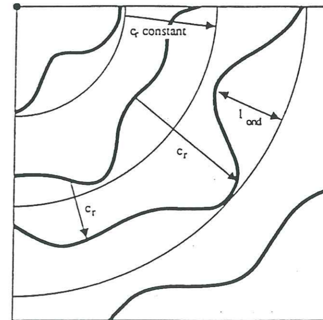
Figure II.4 : Plan de faille avec un front ondulant décrivant la propagation de la rupture (Bour, 1993).
