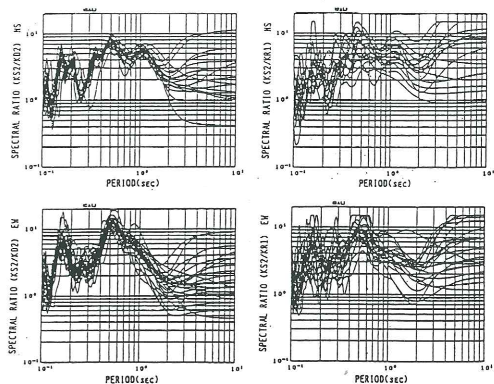
Figure I.8 : Rapports spectraux entre un site sédimentaire et un site en forage (à gauche), et un site rocheux de surface (à droite) (Kudo et Wang, 1992).
