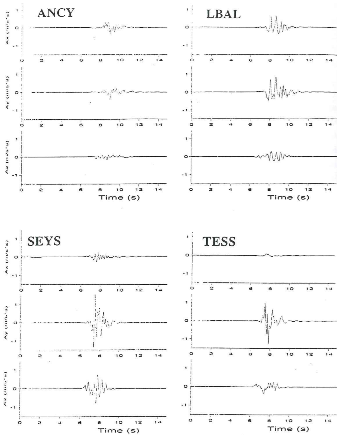
Figure II.78 : Accélérogrammes simulés pour les sites ANCY (en haut à gauche), LBAL (en haut à droite), SEYS (en bas à gauche) et TESS (en bas à droite) ; pour une structure de type "sédimentaire" ; en introduisant une vitesse de rupture variable selon la profondeur sur le plan de faille.
