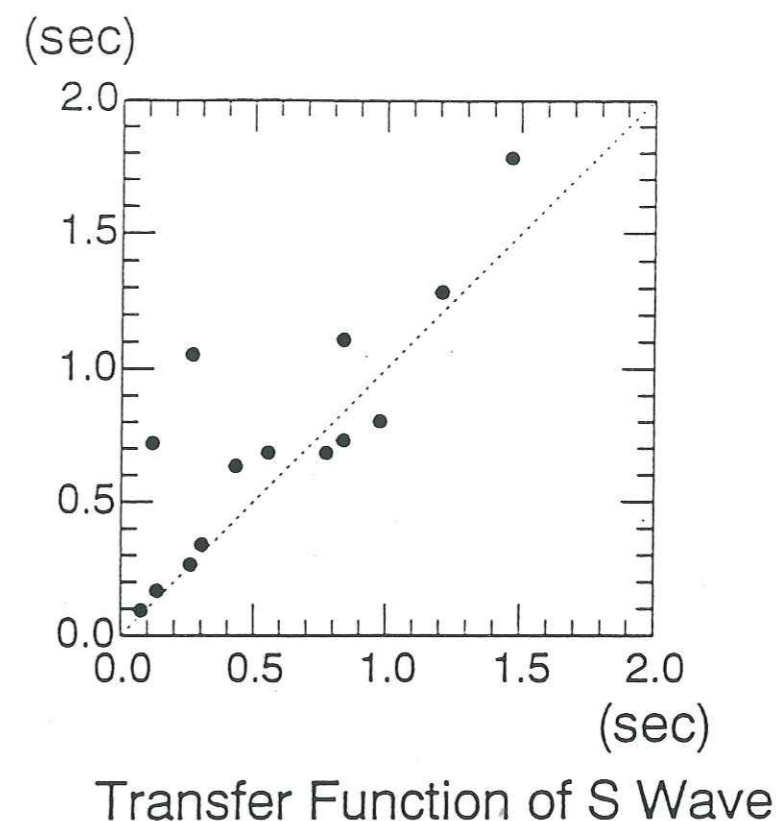
Figure I.17 : Comparaison des périodes prédominantes obtenues avec des rapports H/V sur bruit de fond, et des fonctions de transfert en ondes S (Konno et al., 1994).
