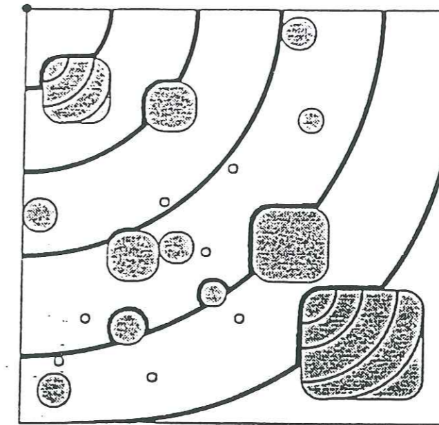
Figure II.8 : Plan de faille avec une distribution de barrières se comportant comme des sources secondaires après le passage du front de rupture (Bour, 1993).
