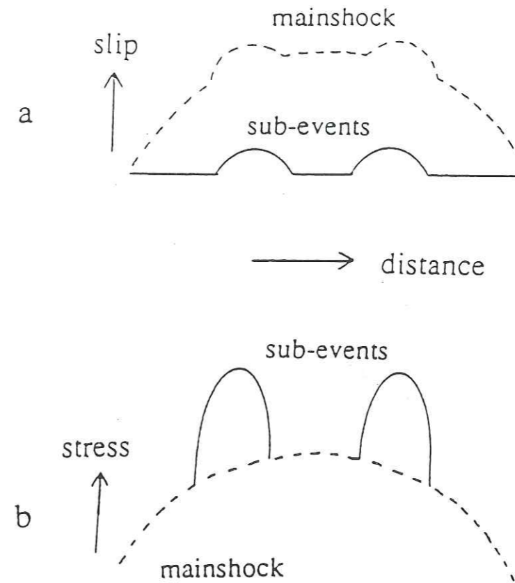
Figure II.15 : Glissement (a) et chute de contrainte (b) sur la faille en fonction de la distance. (a) la ligne pointillée correspond au glissement du choc principal qui contient deux sous-événements de niveau 1. La ligne en trait plein est le glissement pour les deux sous-événements. (b) La ligne en trait plein est la contrainte initiale des sous-événements. La ligne pointillée est le relâchement de contrainte durant le choc principal (Frankel, 1991).
