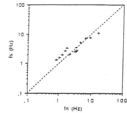
Figure I.30 : Comparaison des fréquences du pic H/V pour chaque site ; f_n : pour les simulations de bruit, f_s : pour des ondes S verticales. La ligne pointillée correspond à f_s = f_n .
