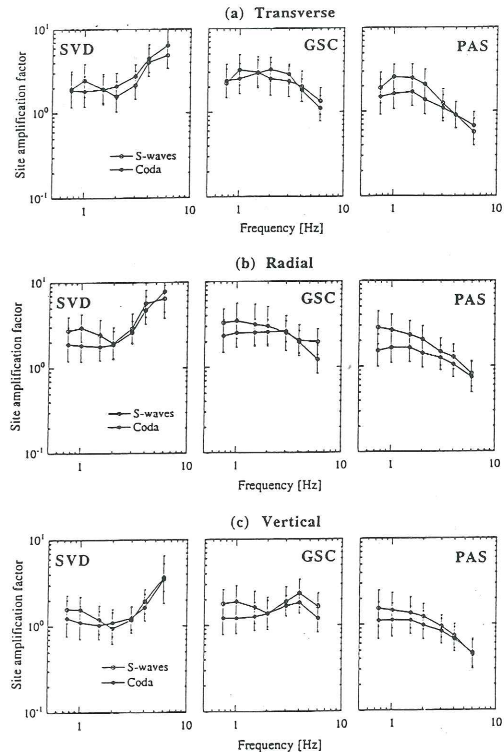
Figure 1.7 : Comparaison des facteurs d'amplification pour les composantes (a) transversale, (b) radiale, et (c) verticale. Les cercles pleins indiquent les facteurs d'amplification pour la coda, les cercles vides, ceux pour les ondes S, et les barres verticales correspondent à +/- un écart type (Kato et al. , 1995).
