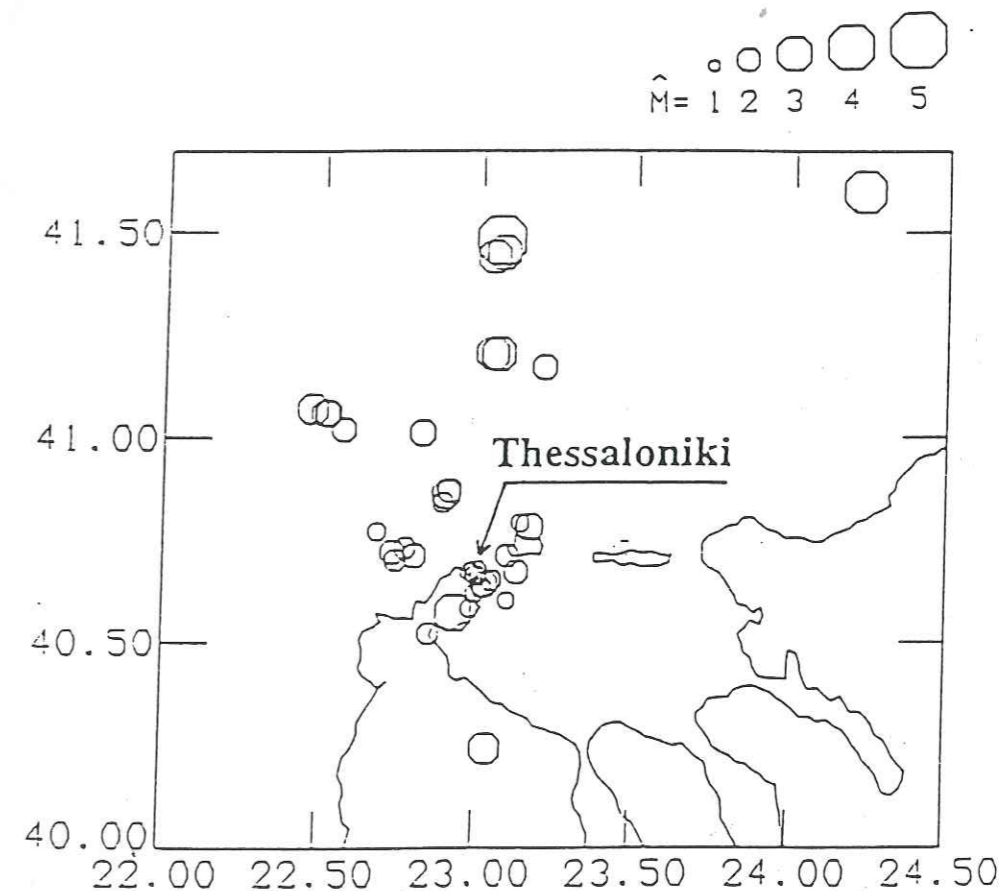
Figure I.41 : Position des épicentres des séismes enregistrés par le réseau temporaire.
