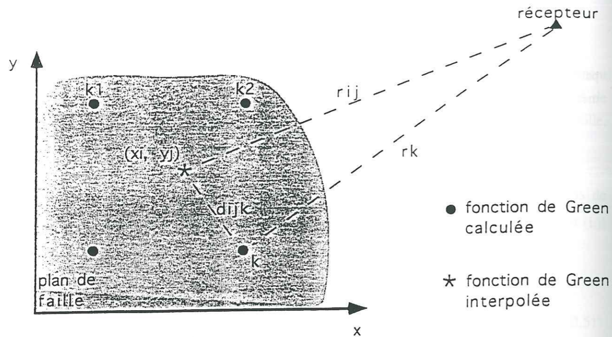
Figure II.34 : Interpolation de la fonction de Green numérique au point (i,j) , en utilisant toutes les fonctions de Green réellement calculées aux points k_i .
