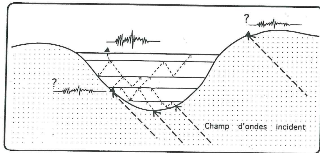
Figure 1.3 : Différence entre les champ d'onde arrivant sur un site sédimentaire, et celui au site rocheux.
