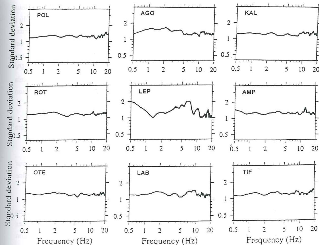
Figure I.53 : Ecart type à chaque fréquence pour les rapports H/V calculés sur les enregistrements de bruit de fond, pour chaque site.
