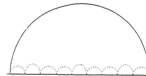
Figure II.17 : Explication schématique du processus de rupture sur la source d'un grand séisme (Irikura et Kamae, 1994).
