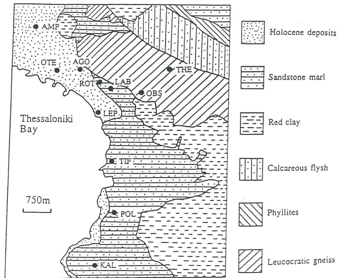
Figure 1.39 : Position des stations du réseau temporaire, sur une carte géologique simplifiée de la ville de Thessalonique.
