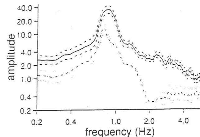
Figure I.18 : Rapports spectraux moyens sur du bruit de fond. Les traits plein et tiré représentent respectivement la moyenne et l'écart type pour des rapports spectraux par rapport à une site de référence. Les lignes tirets-points et pointillés donne l'équivalent pour des rapports H/V (Field et al., 1993).
