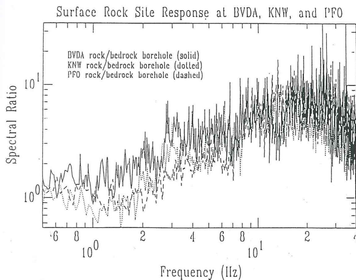
Figure 1.6 : Rapports spectraux entre sites rocheux en surface et substratum en profondeur (Steidl et al. , 1996).
