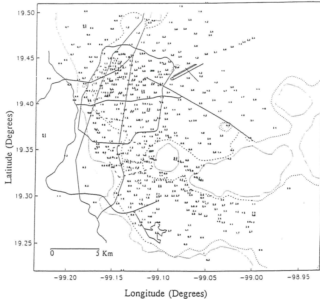
Figure I.10 : Carte des périodes prédominantes (en secondes), obtenues à partir de mesures de bruit de fond, dans la ville de Mexico (Lermo et Chavez-Garcia, 1994).
