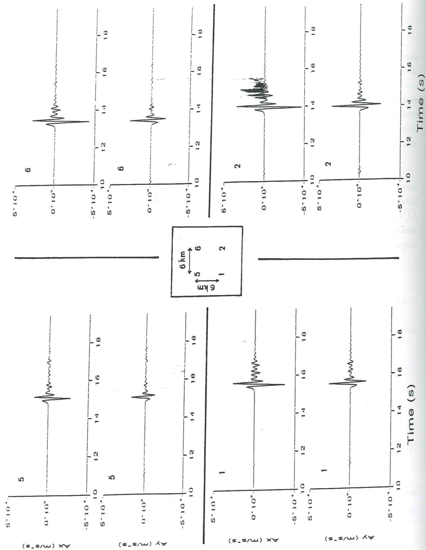
Figure II.33 : Variabilité spatiale d'une fonction de Green numérique calculée en différents points sur le plan de faille.
