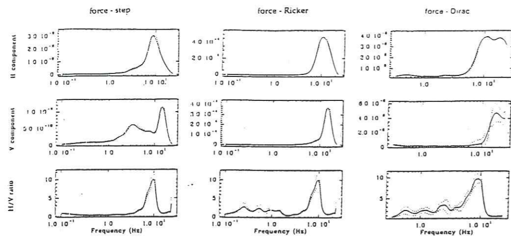
Figure 1.26 : Spectres pour la structure simple S1, avec des sources de type forces unidirectionnelles et des fonctions step, Ricker et Dirac (respectivement de gauche à droite). Lissage sur une échelle logarithmique, de largeur 0.1. Les pointillés indiquent l'écart type, pour 10 simulations de bruit différentes.
