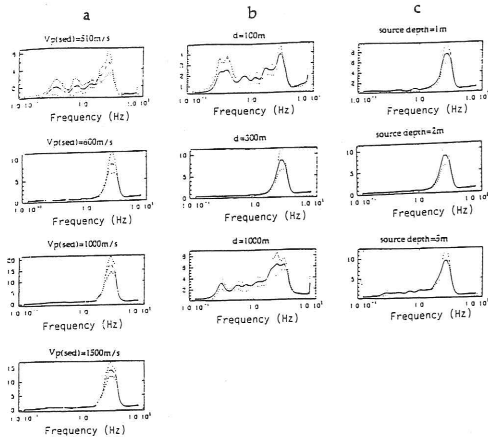
Figure 1.36 : Rapports H/V pour la structure simple S2, avec : (a) un coefficient de Poisson variable dans la couche sédimentaire. La vitesse des ondes S est constante et égale à 300m/s tandis que la vitesse des ondes P ( V_p(\text{sed}) ) est variable. L'amplitude H/V varie alors entre 4.75 et 17.5. (Pour une source à une profondeur constante de 2m, et une distance source-récepteur maximale de 300m). (b) Variations de la distance d , entre les sources les plus éloignées et le récepteur central. L'amplitude du pic H/V varie alors entre 4 et 8.7. (pour une profondeur des sources constante de 2m, et V_p(\text{sed})=600\text{m/s} ). (c) Profondeur des sources variable. L'amplitude du pic H/V reste entre 7.5 et 9.5. (Pour une distance d=300\text{m} et V_p(\text{sed})=600\text{m/s} ). Les pointillés indiquent l'écart type pour dix simulations de bruit différentes.
