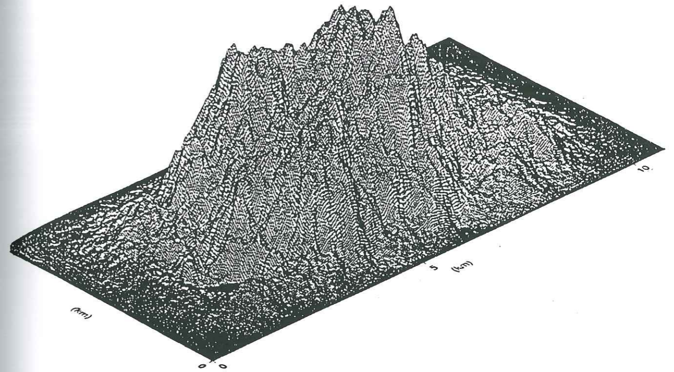
Figure II.19 : Exemple de distribution de glissement satisfaisant le modèle en k^{-2} . La distribution de glissement est apodisée sur les bords de la faille et les valeurs négatives sont mises à zéro. La phase est calculée de manière à concentrer le maximum du glissement au centre de la faille, et pour les grands nombres d'onde, celle-ci est stochastique (Herrero et Bernard, 1994).
