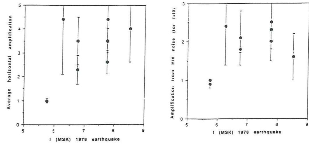
Figure 1.58 : (a) Amplification moyenne arithmétique obtenue avec les rapports spectraux classiques, en fonction de l'intensité mesurée pour le séisme de 1978, en chaque site. (b) Amplification moyenne arithmétique obtenue avec les rapports H/V sur bruit de fond, en fonction de l'intensité mesurée pour le séisme de 1978, en chaque site.
