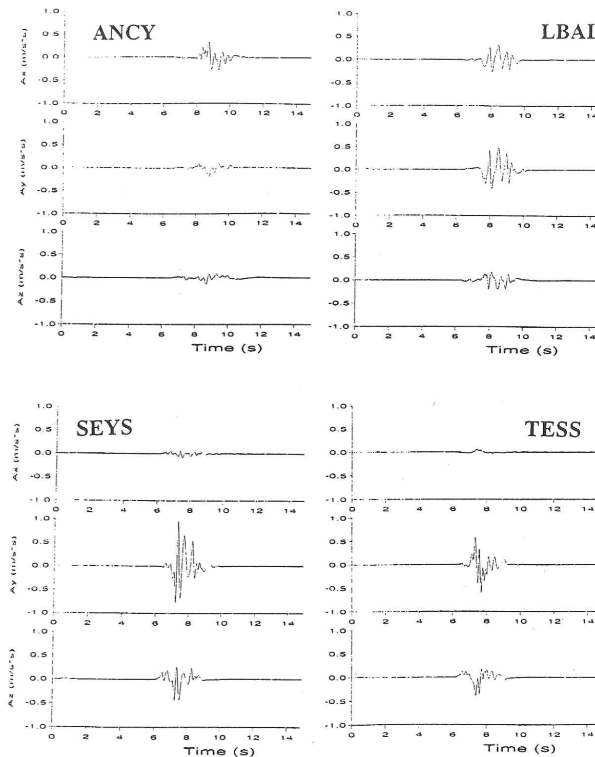
Figure II.77 : Accélérogrammes simulés pour les sites ANCY (en haut à gauche), LBAL (en haut à droite), SEYS (en bas à gauche) et TESS (en bas à droite) ; pour une structure de type "rocher" ; en introduisant une vitesse de rupture variable selon la profondeur sur le plan de faille.
