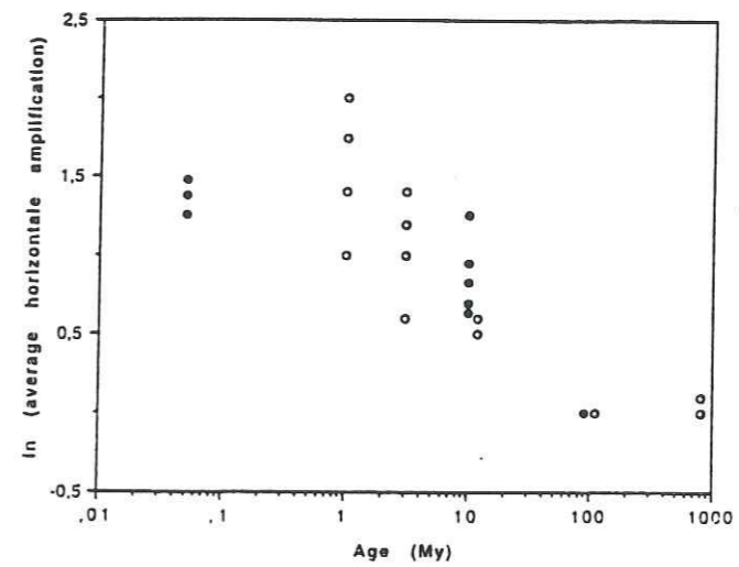
Figure 1.59 : Amplification moyenne arithmétique en fonction de l'âge de la formation géologique de surface, pour chaque site. Les cercles pleins sont les données de l'expérience de Thessalonique, les cercles vides correspondent à des données de Californie de Su et Aki (1995).
