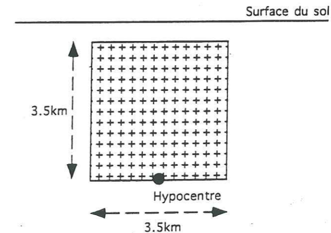
Figure II.73 : Schéma du plan de faille utilisé pour les simulations du séisme de Annecy (magnitude 5.3).
