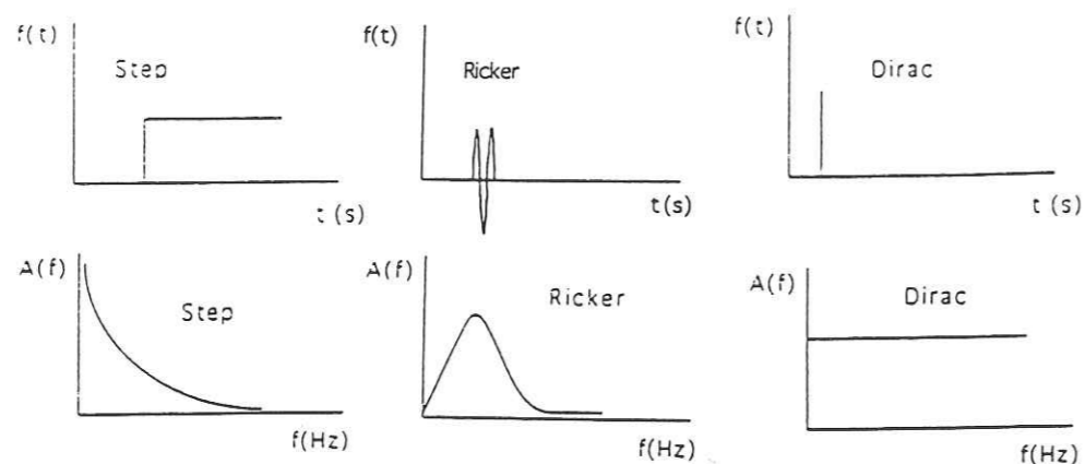
Figure 1.24 : Forme en temps et en fréquence des fonctions source utilisées.
