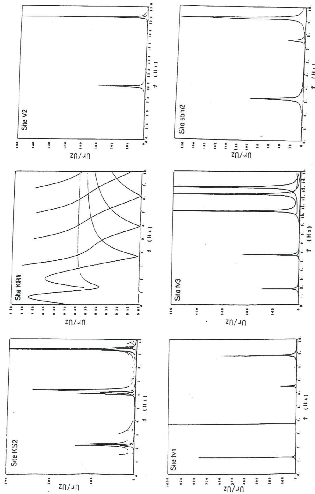
Figure I.32 : Courbes de polarisation des ondes de Rayleigh pour les sites à Ashigara Valley, Turkey Flat et SE de la France. L'axe vertical correspond au rapport entre la composante radiale et la composante verticale ( U_x/U_z ).
