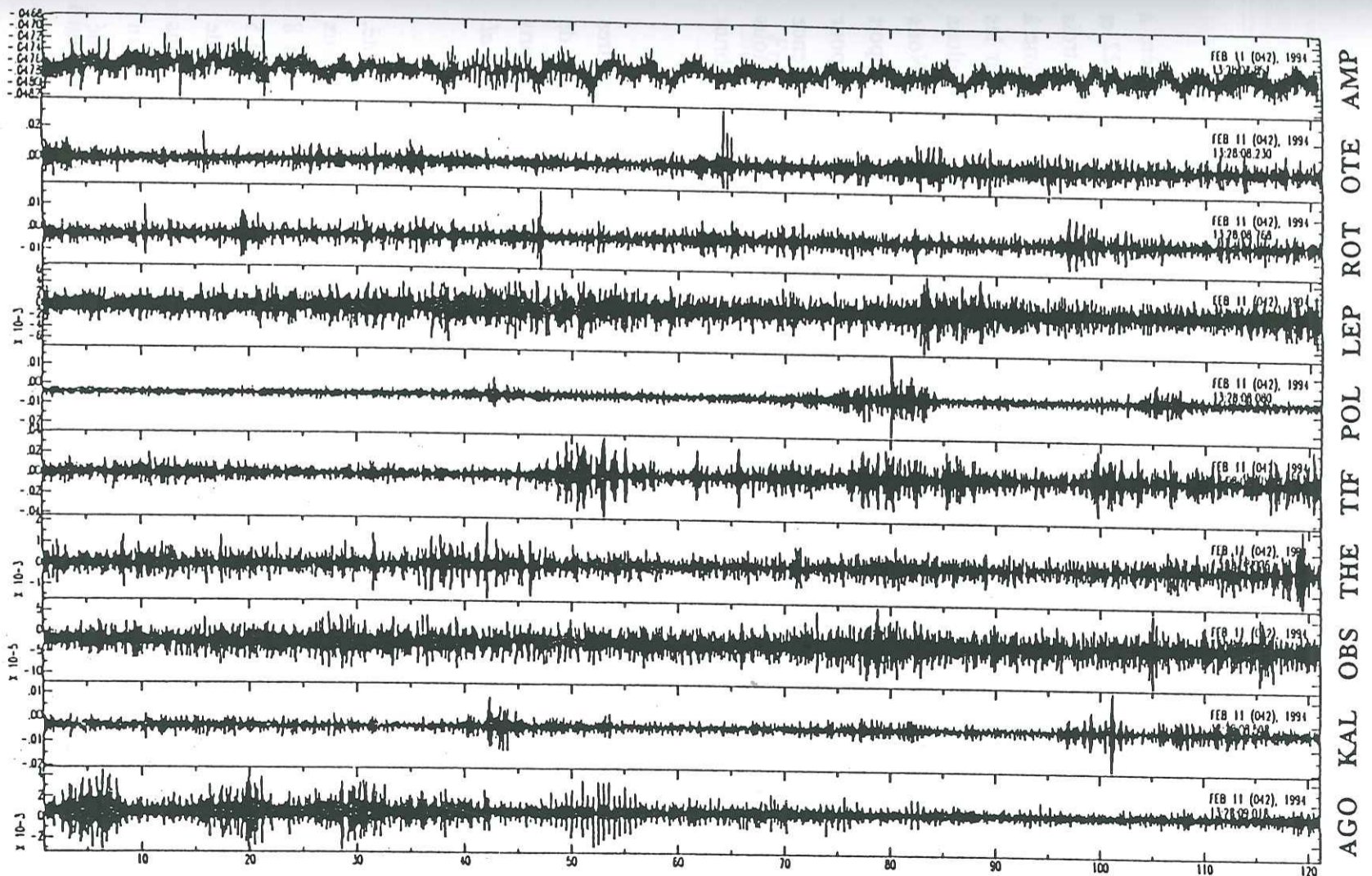
Figure 1.43 : Exemple d'un enregistrement de bruit de fond ambiant. Composante EW.
