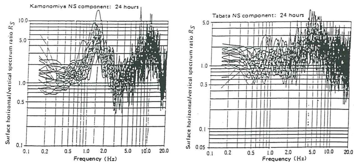
Figure 1.12 : Variations temporelles des rapports H/V pour deux sites sur des enregistrements de bruit de fond étalés sur 24 heures (Nakamura, 1989).
