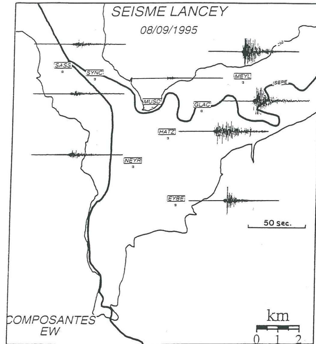
Figure II.59 : Enregistrement du séisme de la Combe de Lancey (08/09/95) par différentes stations installées dans la ville de Grenoble (Le Brun et Hatzfeld, 1996).
