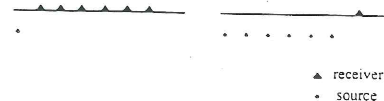
Figure I.23 : Dispositif source-récepteur. Etant donné que ces deux schémas sont équivalents, nous pouvons utiliser directement les résultats fournis par le programme Axitra (pour une source et plusieurs récepteurs), pour calculer les sismogrammes synthétiques correspondant au modèle multi-sources.
