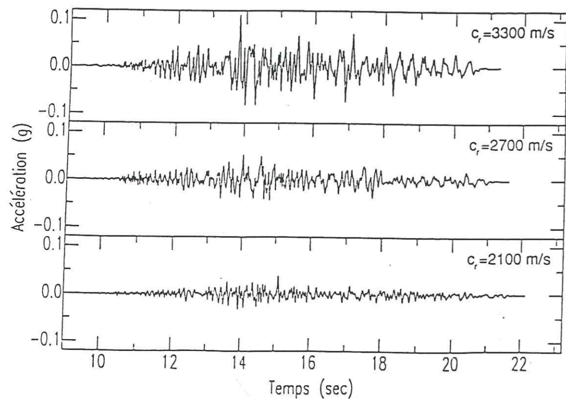
Figure II.27 : Haut : Variation de l'accélération simulée avec le sens de propagation de la rupture sur la faille. Bas : Variation de l'accélération simulée avec le vitesse de propagation de la rupture (Bour, 1993).
