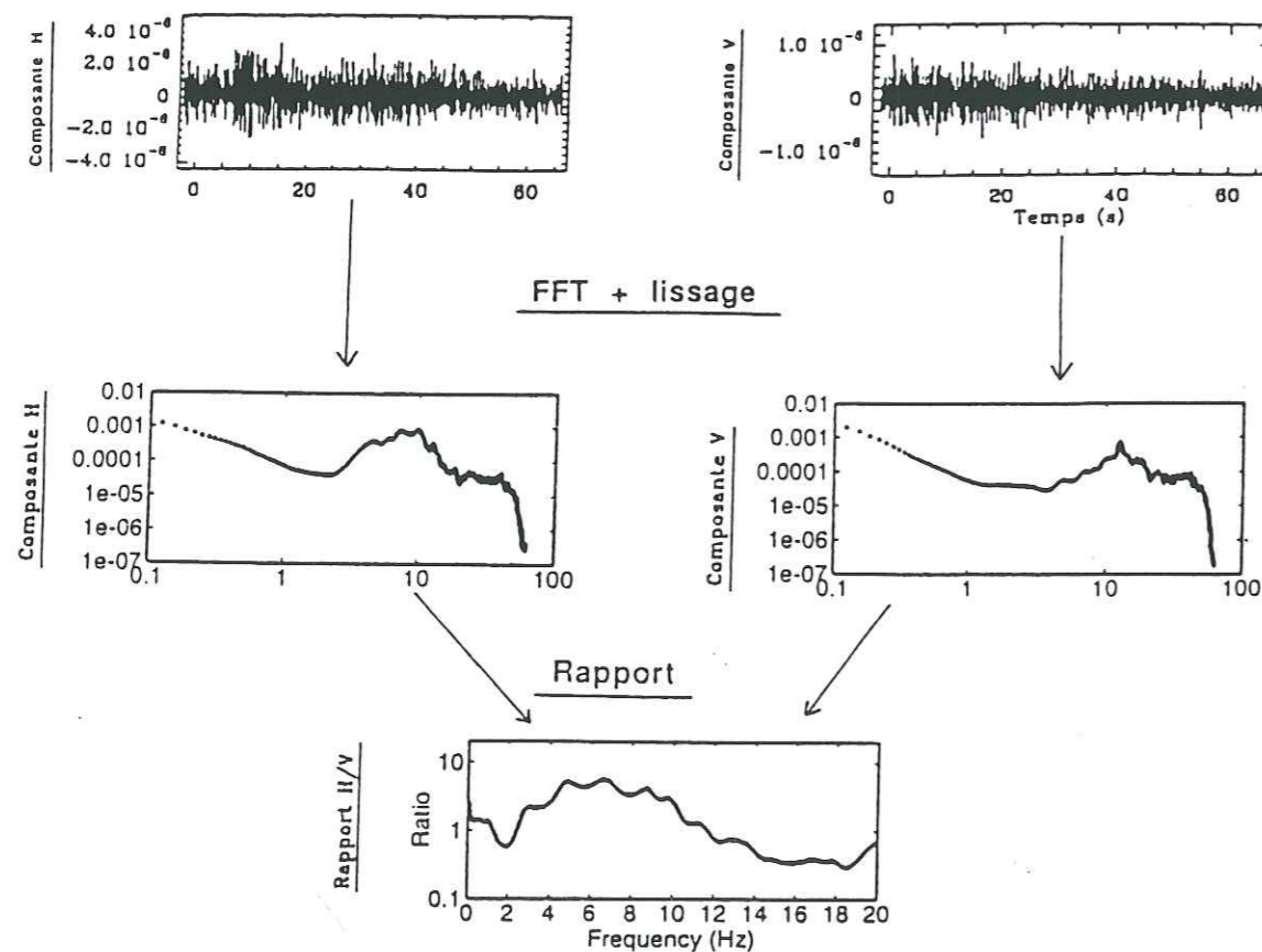
Figure 1.13 : Schéma descriptif de la méthode du rapport H/V.
