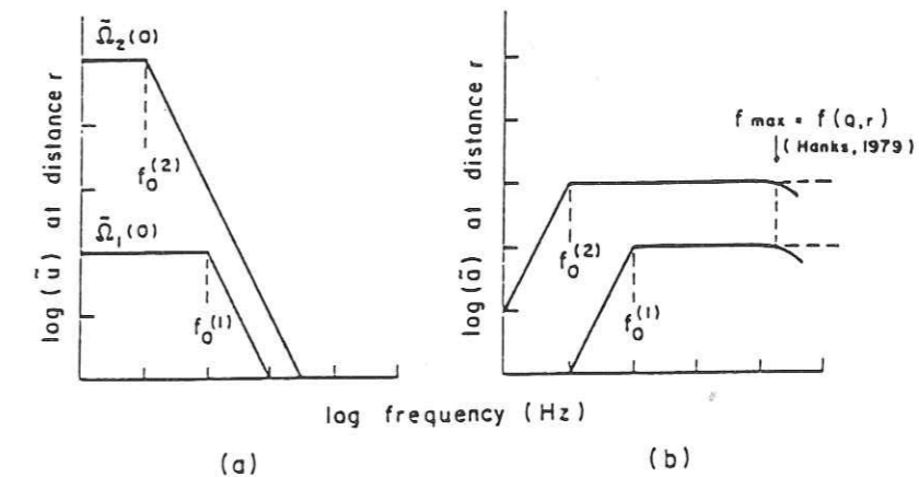
Figure II.6 : Spectres de (a) déplacement et (b) accélération pour le modèle de source en \omega^2 , pour deux séismes avec une chute de contrainte constante, observés à la même distance, dans un milieu infini, homogène, isotrope et élastique (Papageorgiou et Aki, 1983).
