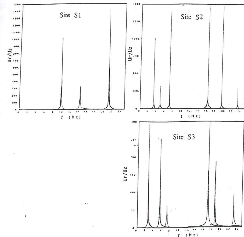
Figure I.31 : Courbes de polarisation des ondes de Rayleigh pour les structures à une couche. L'axe vertical correspond au rapport entre la composante radiale et la composante verticale ( U_r/U_z ).
