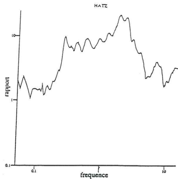
Figure II.62 : Rapport spectral entre les sites HATZ (sédiments) et MUSD (rocher), calculé sur plusieurs séismes enregistrés par ces stations (Le Brun et Hatzfeld, 1996).
