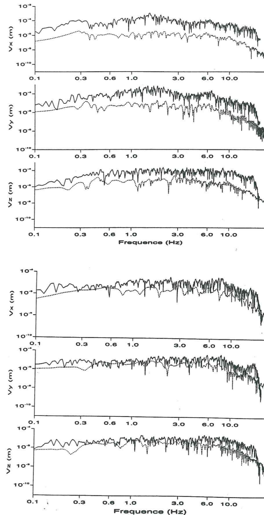
Figure II.69 : Comparaison des spectres en vitesse des fonctions de Green empirique (trait plein) et numérique (trait pointillés) pour les sites HATZ (en haut) et MUSD (en bas).
