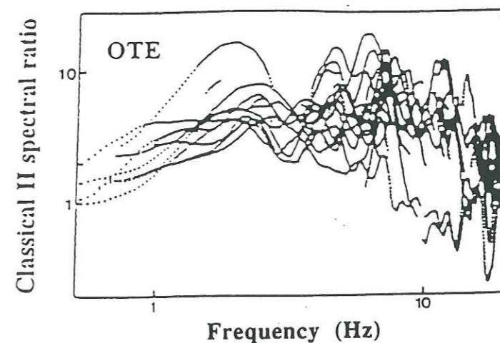
Figure I.45 : Rapports spectraux classiques obtenus pour tous les séismes au site OTE.
