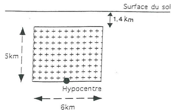
Figure II.64 : Schéma du plan de faille utilisé pour les simulations d'un séisme de magnitude 5.5 sous la Combe de Lancey. Plan de faille : orientation : 39^\circ N , pendage : 80^\circ , direction du glissement : -5^\circ .
