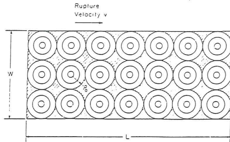
Figure II.10 : Distribution de failles circulaires sur le plan de faille, pour le modèle spécifique de barrières (agrégat de failles circulaires) (Papageorgiou et Aki, 1983).
