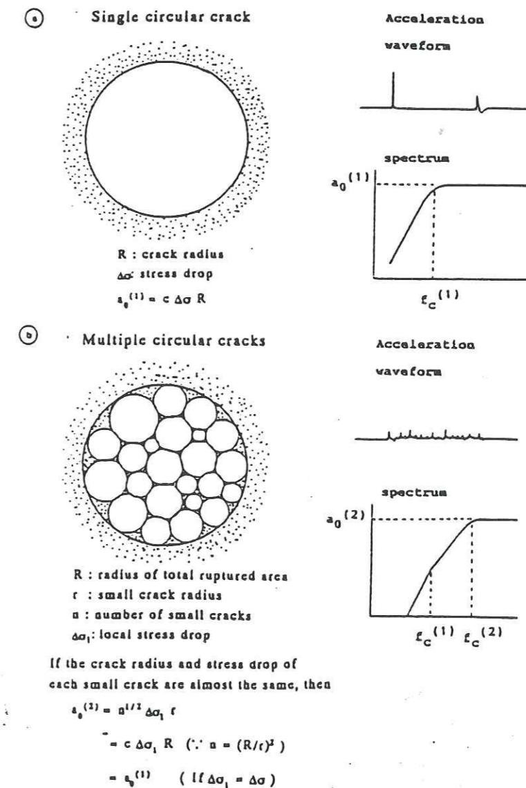
Figure II.9 : Illustration des modèles de source pour un séisme provoquant un mouvement du sol en \omega^2 . Modèle de faille circulaire unique (a), et modèle multi-failles (b). Pour chacun des deux modèles, sont données l'accélération et sa forme spectrale correspondante (Irikura et Kamae, 1994).
