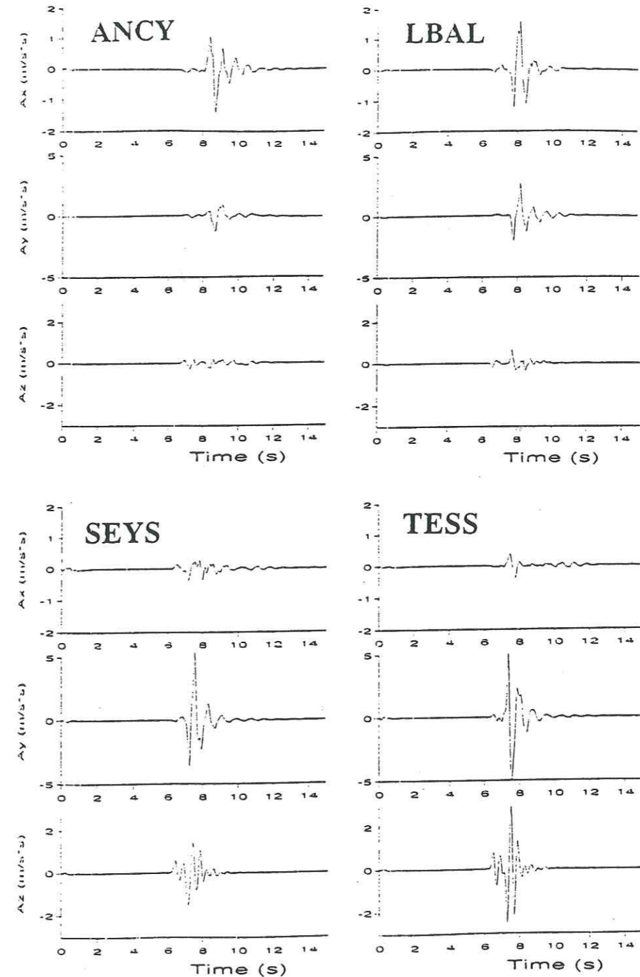
Figure II.76 : Accélérogrammes simulés pour les sites ANCY (en haut à gauche), LBAL (en haut à droite), SEYS (en bas à gauche) et TESS (en bas à droite) ; pour une structure de type "sédimentaire".
