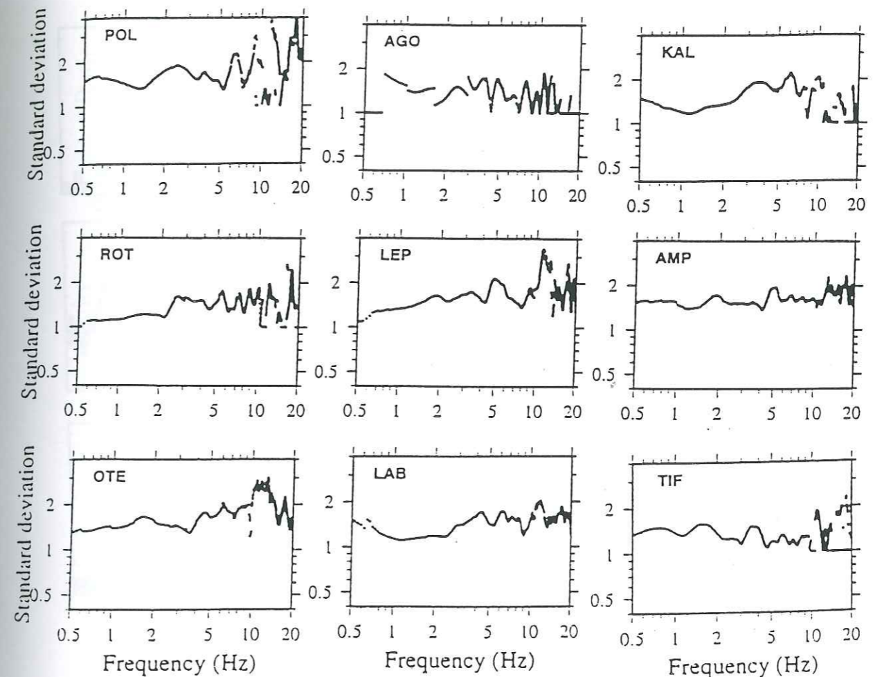
Figure I.46 : Ecart type à chaque fréquence pour les rapports spectraux classiques calculés sur tous les séismes, pour chaque site.
