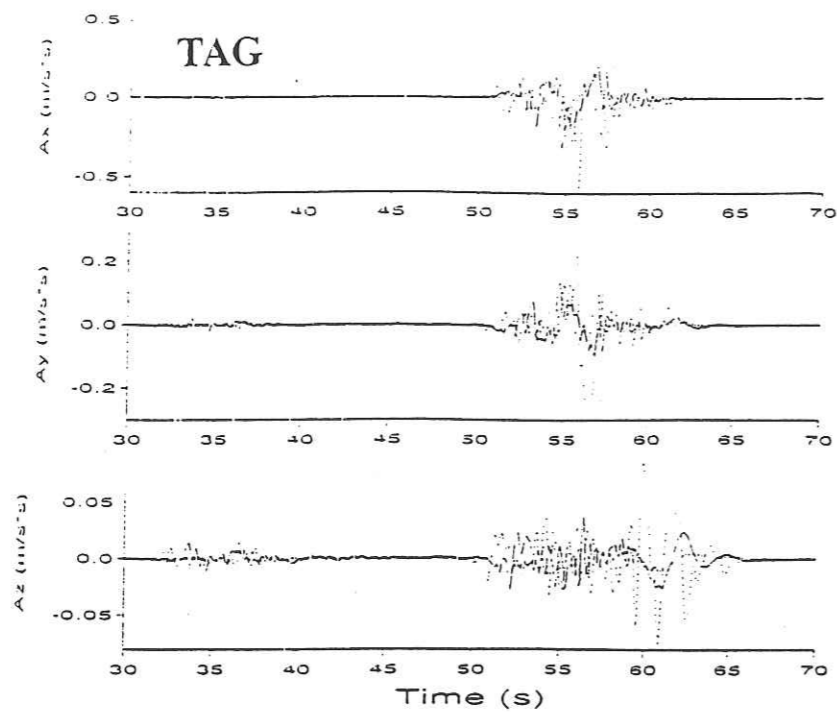
Figure II.51 : Accélérogrammes simulés au site TAG, avec une fonctions de Green unique calculée en bas à gauche du plan de faille (cas 1, trait pointillés serrés), au centre du plan de faille (cas 2, trait plein) et en haut à droite du plan de faille (cas 3, trait pointillés espacés).
