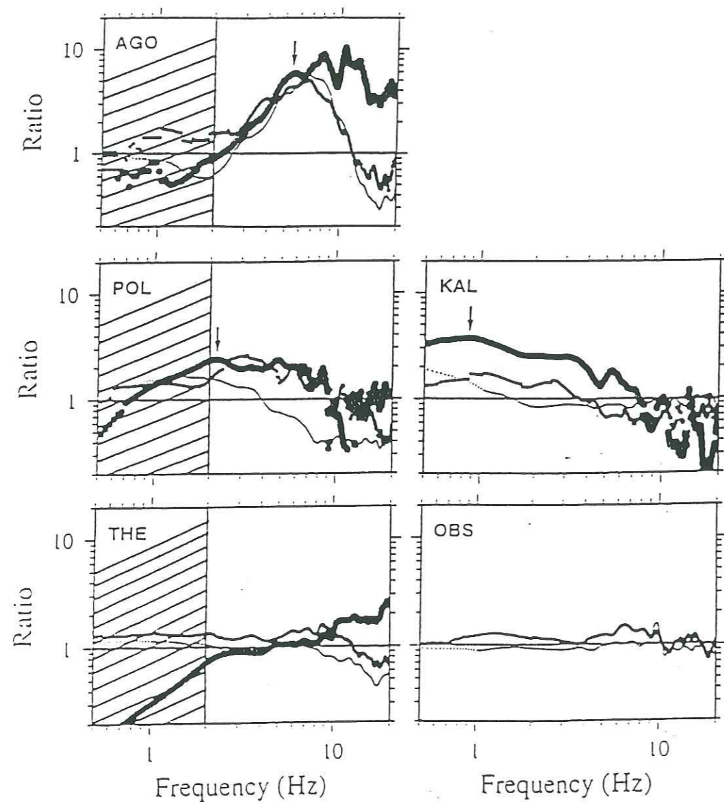
Figure 1.48-b : Rapports spectraux pour chaque site. Trait épais : rapport spectral classique; trait intermédiaire : fonction récepteur ; trait fin : rapport H/V sur bruit de fond. Les flèches indiquent la valeur choisie comme fréquence de résonance ( f_0 ) pour chaque site. Les zones hachurées correspondent à la bande de fréquence inutilisable pour les capteurs L22.
