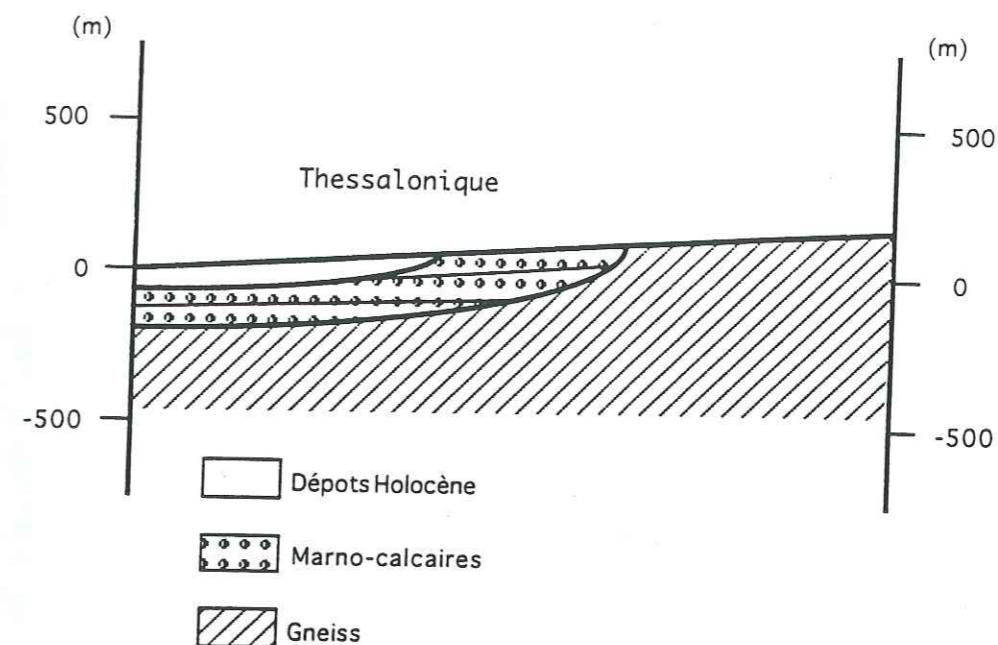
Figure I.40 : Coupe géologique simplifiée à travers le bassin de Thessalonique.
