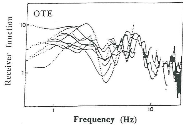
Figure 1.49 : Fonctions récepteur obtenues pour tous les séismes au site OTE.
