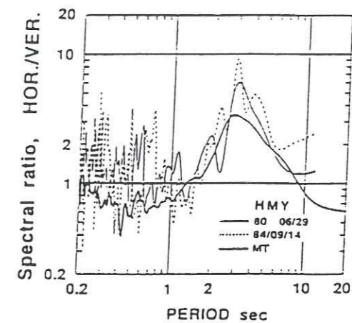
Figure 1.21 : Comparaison entre le rapport H/V sur du bruit de fond (trait épais) et les fonctions récepteur calculées sur des séismes (trait fin et pointillé) (Yamanaka et al., 1994).
