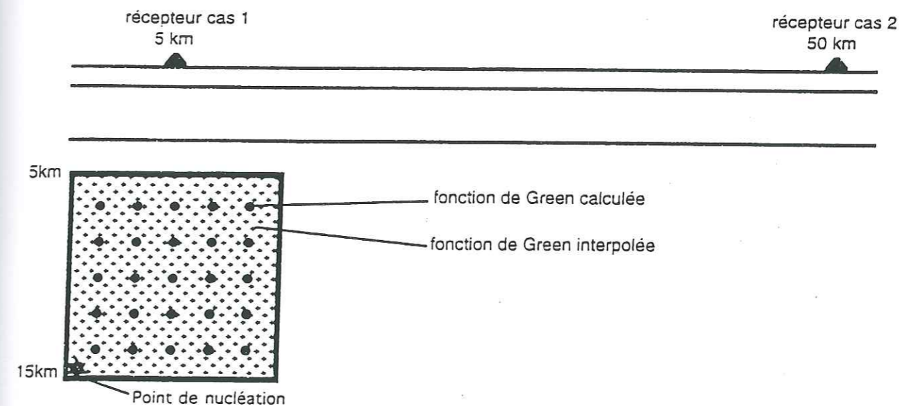
Figure II.30 : Schéma du dispositif source-stations utilisé, et de la discrétisation du plan de faille.
