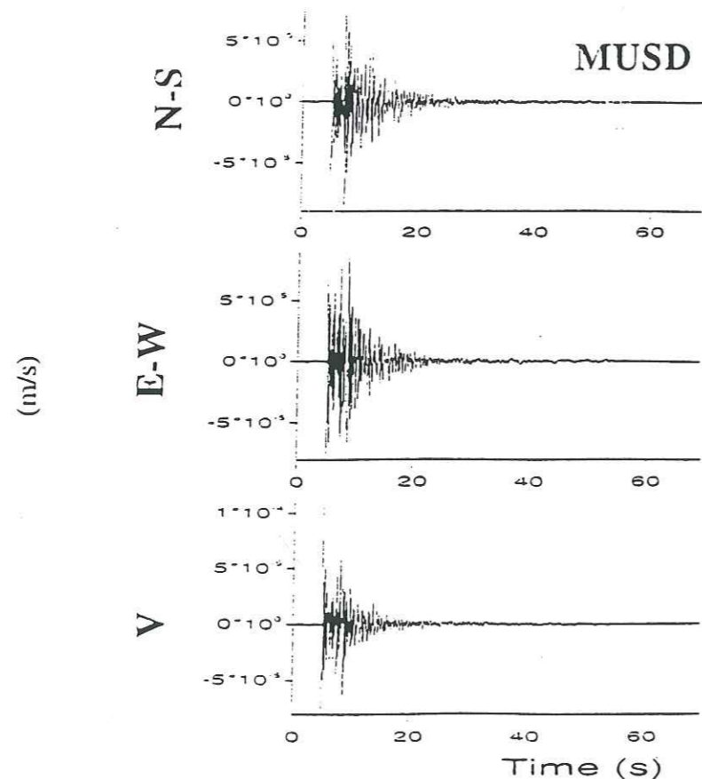
Figure II.61 : Enregistrement du séisme de Lancey, utilisé comme fonction de Green empirique, au site MUSD.
