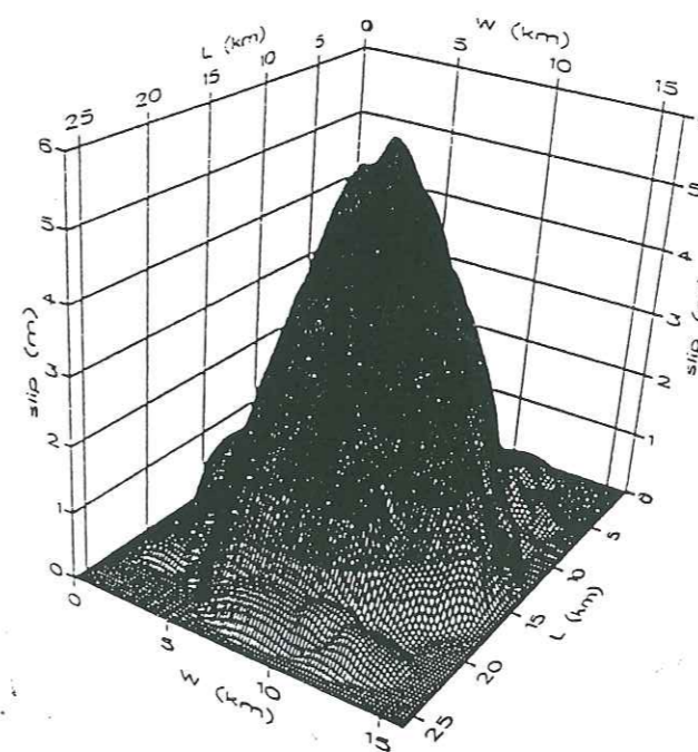
Figure II.44 : Distribution du glissement sur le plan de faille.
