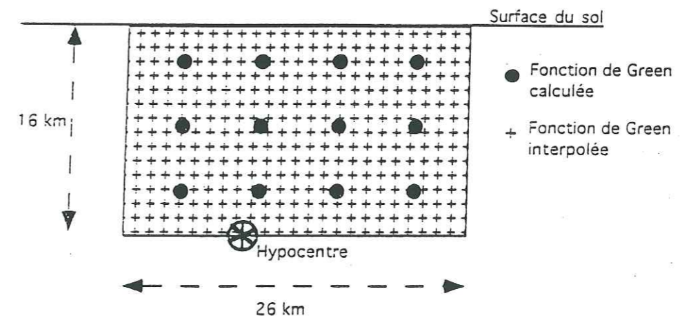
Figure II.42 : Schéma du plan de faille utilisé pour les simulations du séisme de Kobe.
