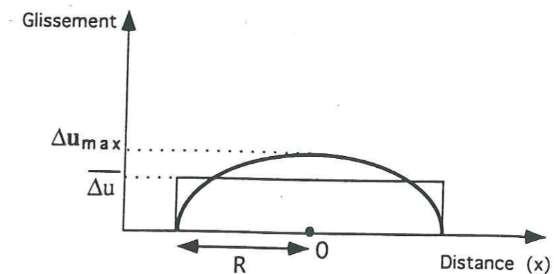
Figure II.7 : Forme du glissement en chaque point et du glissement moyen pour une faille circulaire.
