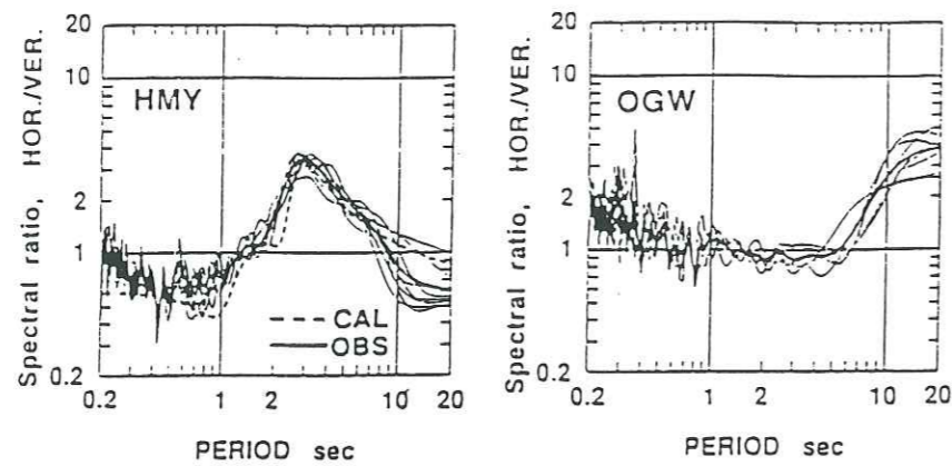
Figure 1.14 : Rapports H/V sur du bruit de fond pour deux sites. Les traits fins donnent les courbes obtenues à chaque période d'observation, les traits épais donnent la moyenne, et les pointillés sont les rapports H/V théoriques pour des ondes de Rayleigh fondamentales (Yamanaka et al., 1994).
