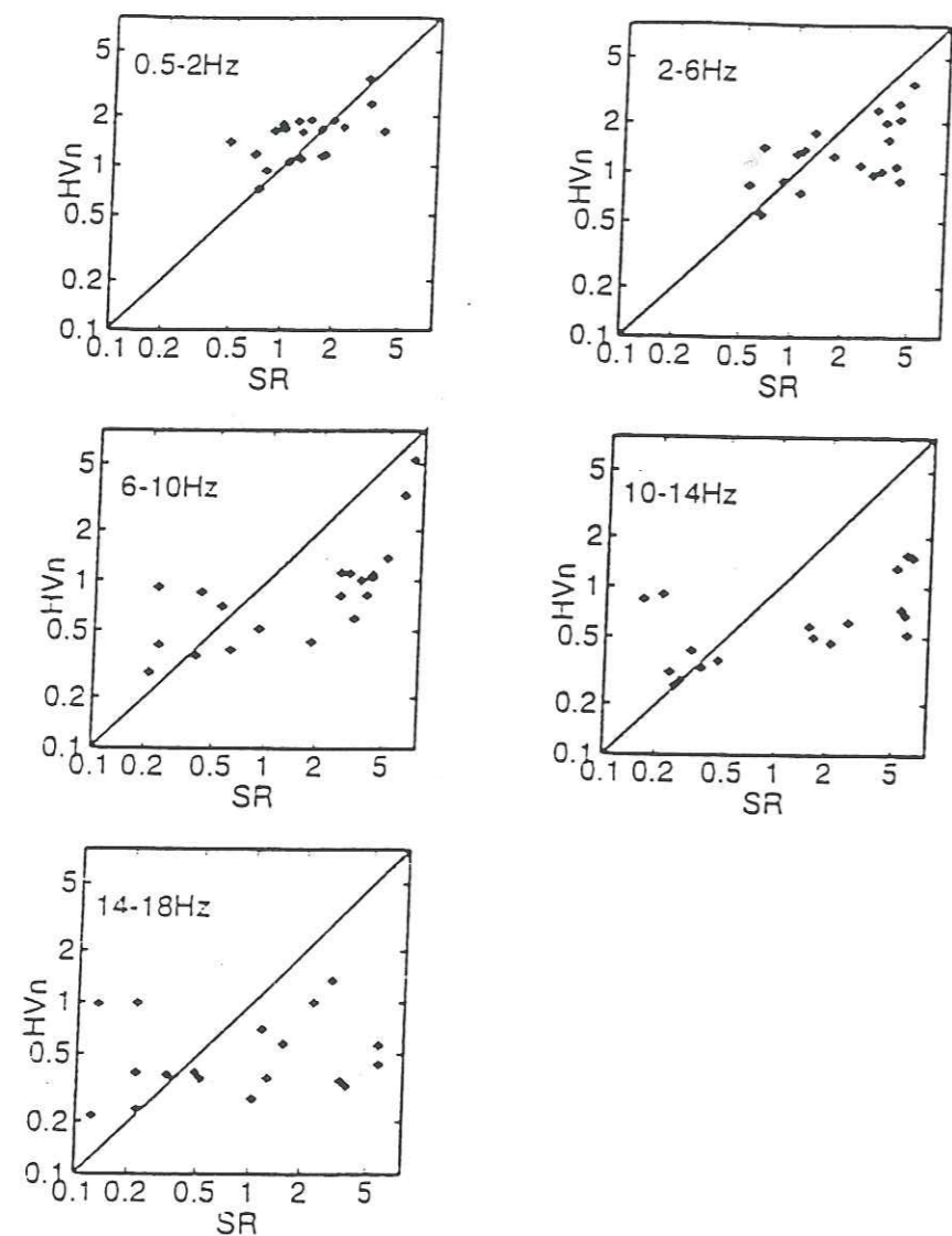
Figure 1.55 : Comparaison de l'amplification moyenne arithmétique à chaque site, pour les rapports H/V sur bruit de fond (HVn) et les rapports spectraux classiques (SR) pour différentes bandes de fréquence. L'accord entre les deux, se dégrade vers les hautes fréquences.
