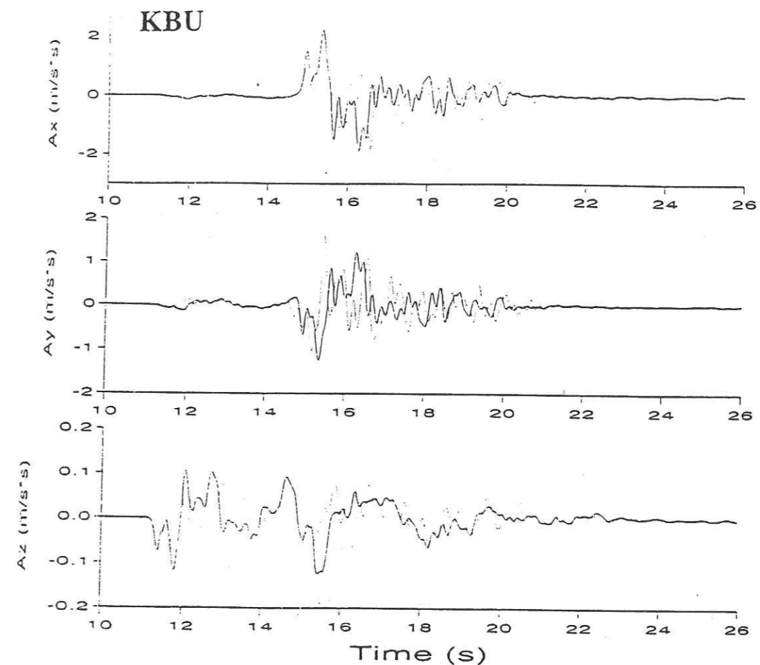
Figure II.45 : Accélération simulée au site KBU pour deux valeurs différentes de la taille minimale des sous-événements : r_{min}=1570m (trait plein) et r_{min}=570m (trait pointillé).
