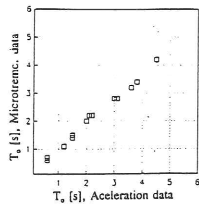
Figure I.11 : Comparaison entre les périodes prédominantes obtenues d'après la fonction de transfert empirique moyenne sur des données accélérométriques et celles obtenues avec des mesures de bruit de fond (Lermo et Chavez-Garcia, 1994).
