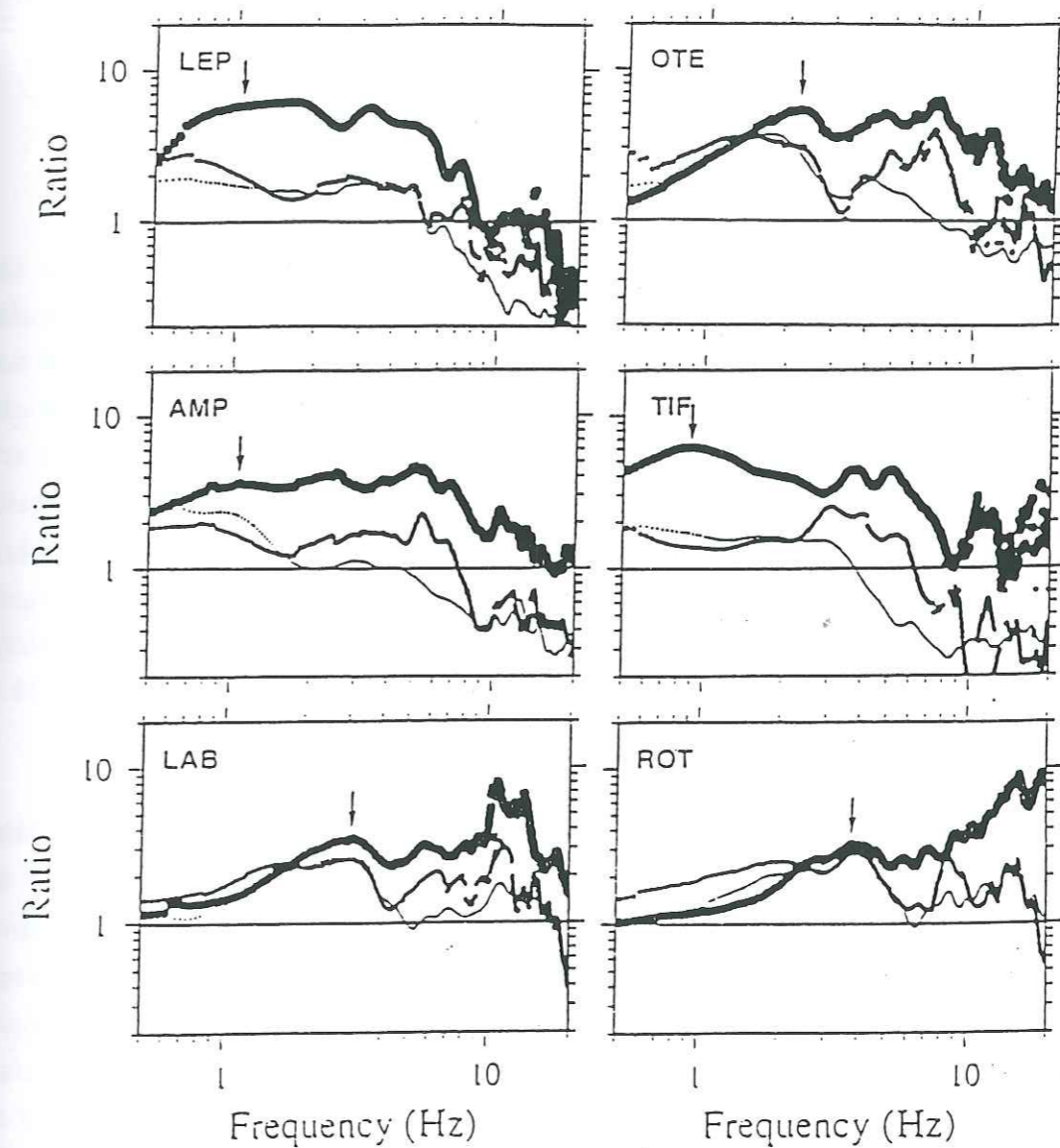
Figure 1.48-a : Rapports spectraux pour chaque site. Trait épais : rapport spectral classique ; trait intermédiaire : fonction récepteur ; trait fin : rapport H/V sur bruit de fond. Les flèches indiquent la valeur choisie comme fréquence de résonance ( f_0 ) pour chaque site.
