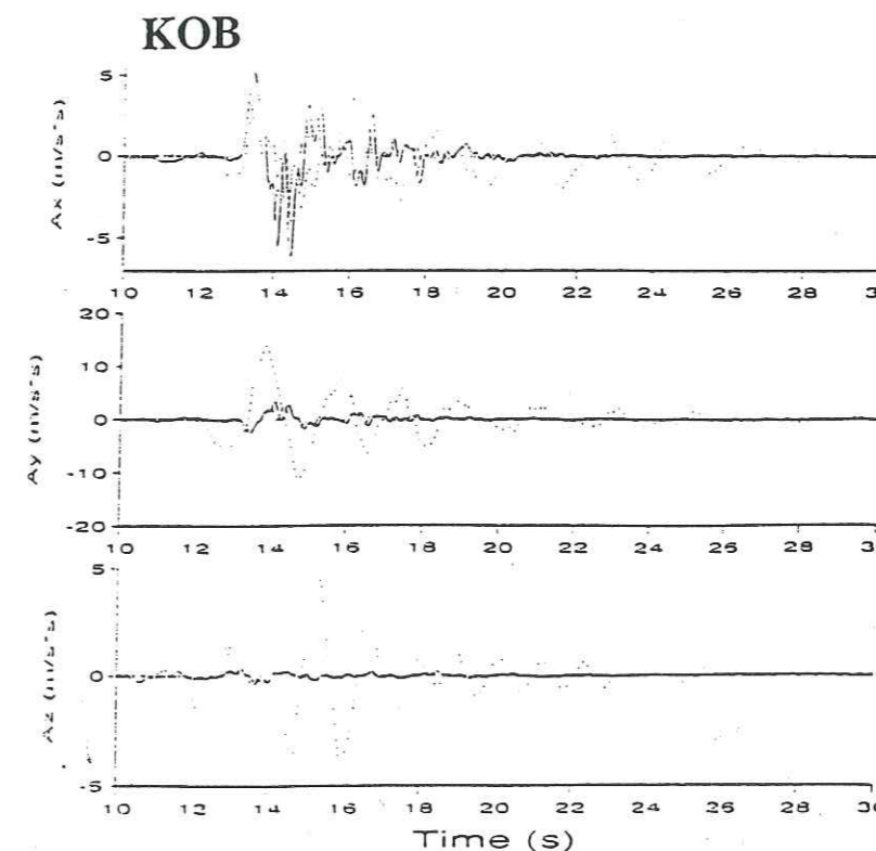
Figure II.50 : Accélérogrammes simulés au site KOB, avec une fonctions de Green unique calculée en bas à gauche du plan de faille (cas 1, trait pointillés serrés), au centre du plan de faille (cas 2, trait plein) et en haut à droite du plan de faille (cas 3, trait pointillés espacés).
