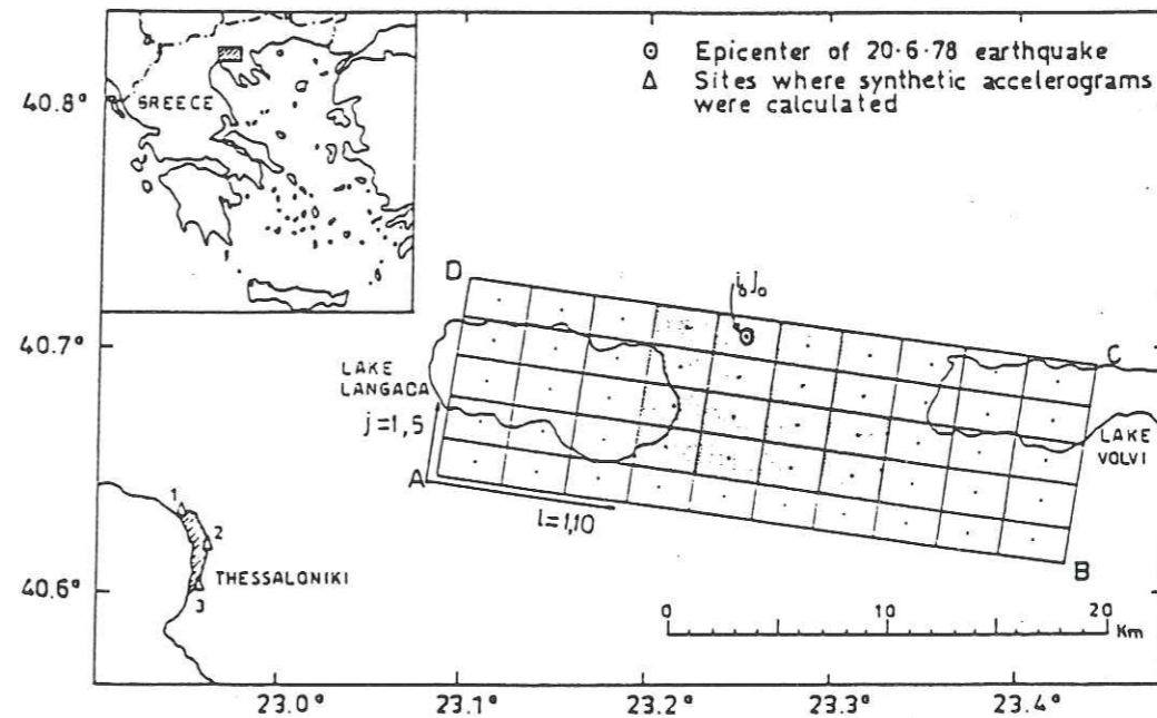
Figure II.25 : Projection du plan de faille en surface, pour le séisme de Thessalonique de 1978, et sa subdivision en 50 sous-failles. Le moment est distribué préférentiellement au centre de la faille (zone ombrée), avec un glissement uniforme (Theodulidis et Bard, 1995).
