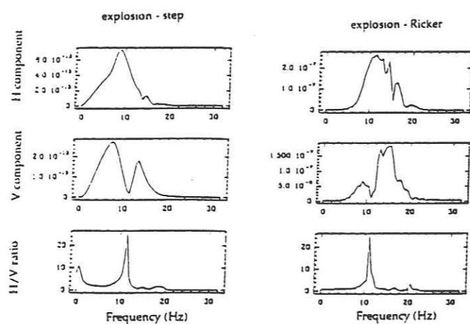
Figure 1.25 : Spectres pour la structures simple S1, avec une source de type explosion et une fonction step (à gauche) et Ricker (à droite). Largeur de la fenêtre de lissage : 1 Hz.
