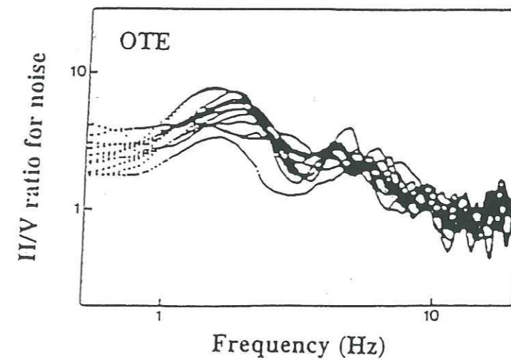
Figure 1.52 : Rapports H/V calculés sur les enregistrements de bruit de fond, au site OTE.
