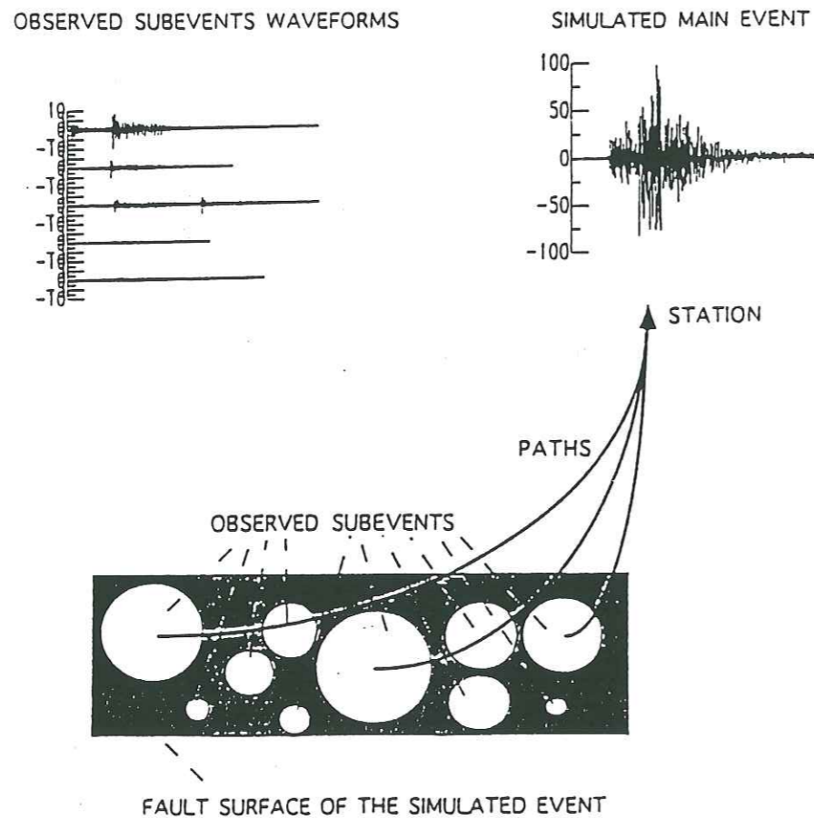
Figure II.23 : Diagramme schématique d'une simulation de mouvement fort utilisant plusieurs fonctions de Green empiriques. Composantes NS du mouvement observé pour 5 répliques (en haut à gauche) et pour le choc principal (en haut à droite) (Tumarkin et Archuleta, 1994).
