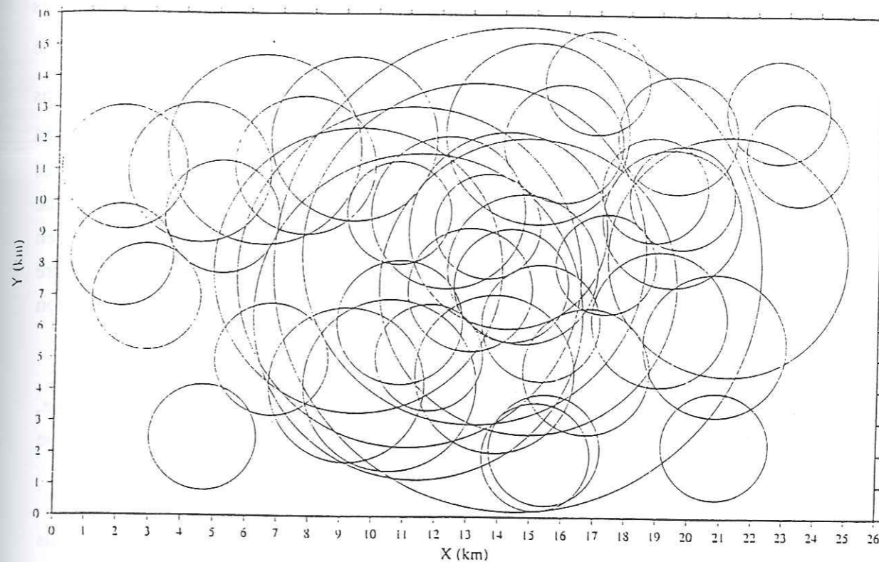
Figure II.43 : Distribution des sous-événements sur le plan de faille.
