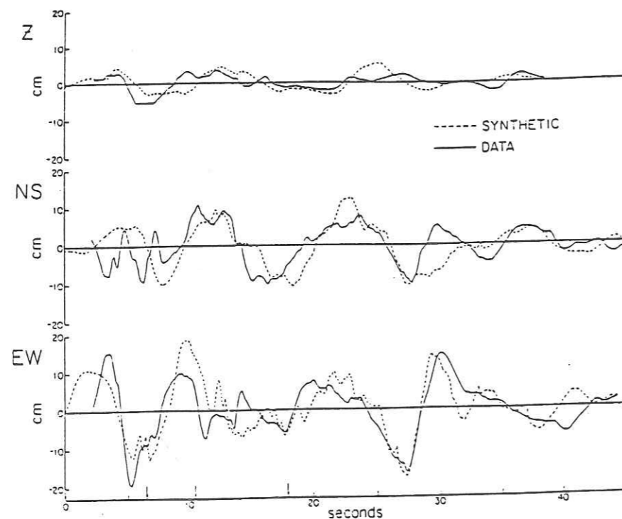
Figure II.2 : Comparaison entre les synthétiques obtenus par sommation de trois répliques et le déplacement enregistré à El Centro, du séisme d'Imperial Valley, 1940. Le temps d'initiation de chaque réplique utilisée est indiqué par une flèche (Hartzell, 1978).
