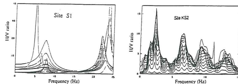
Figure 1.34 : Rapports H/V obtenus avec des ondes SV à incidence variable, pour une structure simple (à gauche) et un site à Ashigara Valley (à droite).
