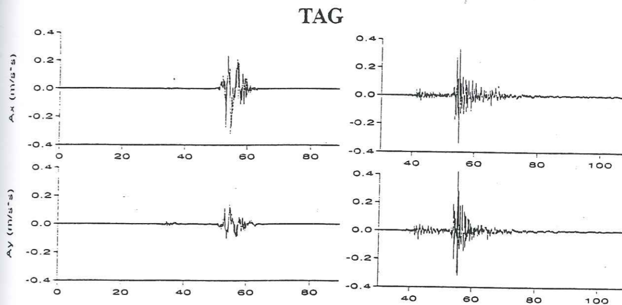
Figure II.56 : Comparaison entre accélérogrammes simulés avec une seule fonction de Green (trait pointillé) et l'interpolation des fonctions de Green en chaque point (trait plein), à gauche; et accélérogramme observé (à droite) ; pour le site TAG.
