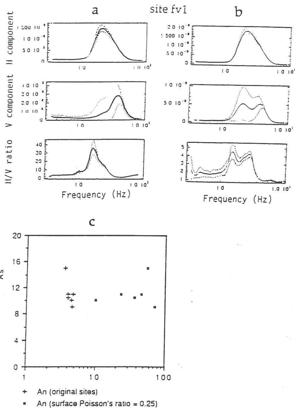
Figure 1.37 : Spectres pour le site fv1 (SE de la France) ; (a) Structure géologique de départ pour ce site. (b) Introduction d'une couche de surface de 4m d'épaisseur, avec un coefficient de Poisson de 0.25. L'amplitude du rapport H/V chute de 35 à 4.5. Les pointillés indiquent l'écart type pour dix simulations de bruit différentes. (c) Comparaison des amplitudes du pic H/V pour les simulations de bruit, A_n , (pour les sites KS2, fv1, sbm1, sbm2, larv1, larv2) pour les structures géologiques de départ, puis avec un coefficient de Poisson de 0.25 en surface ; en fonction des amplitudes, A_s , pour des ondes S verticales.
