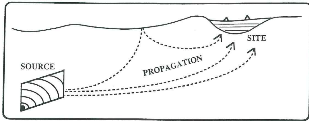
Figure 1.1 : Effets de source, propagation et site, mis en jeu au cours d'un séisme.
