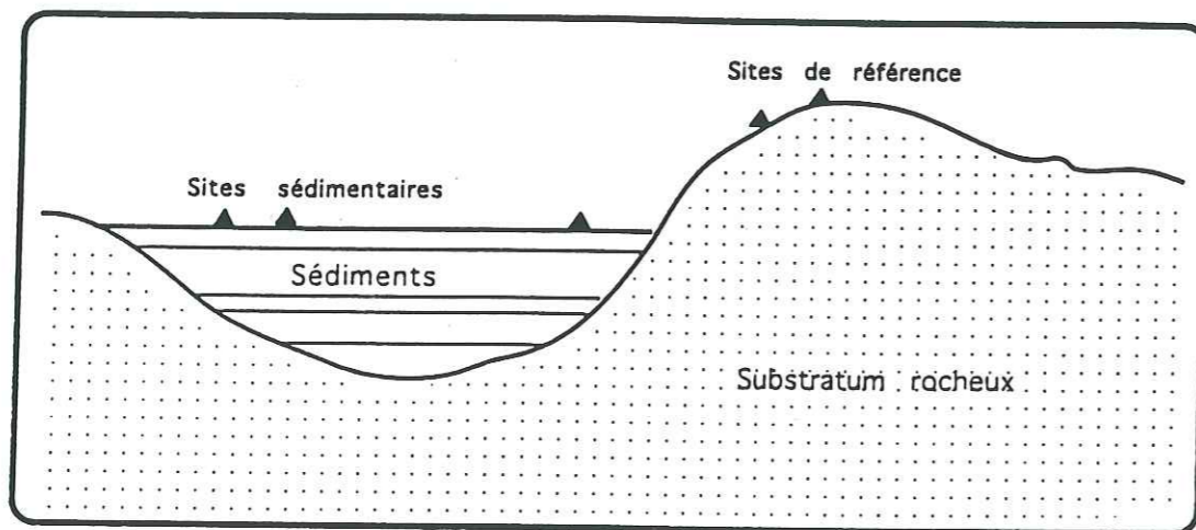
Figure 1.2 : Etude des effets de site à l'aide de stations sur les sédiments, et sur le substratum rocheux.
