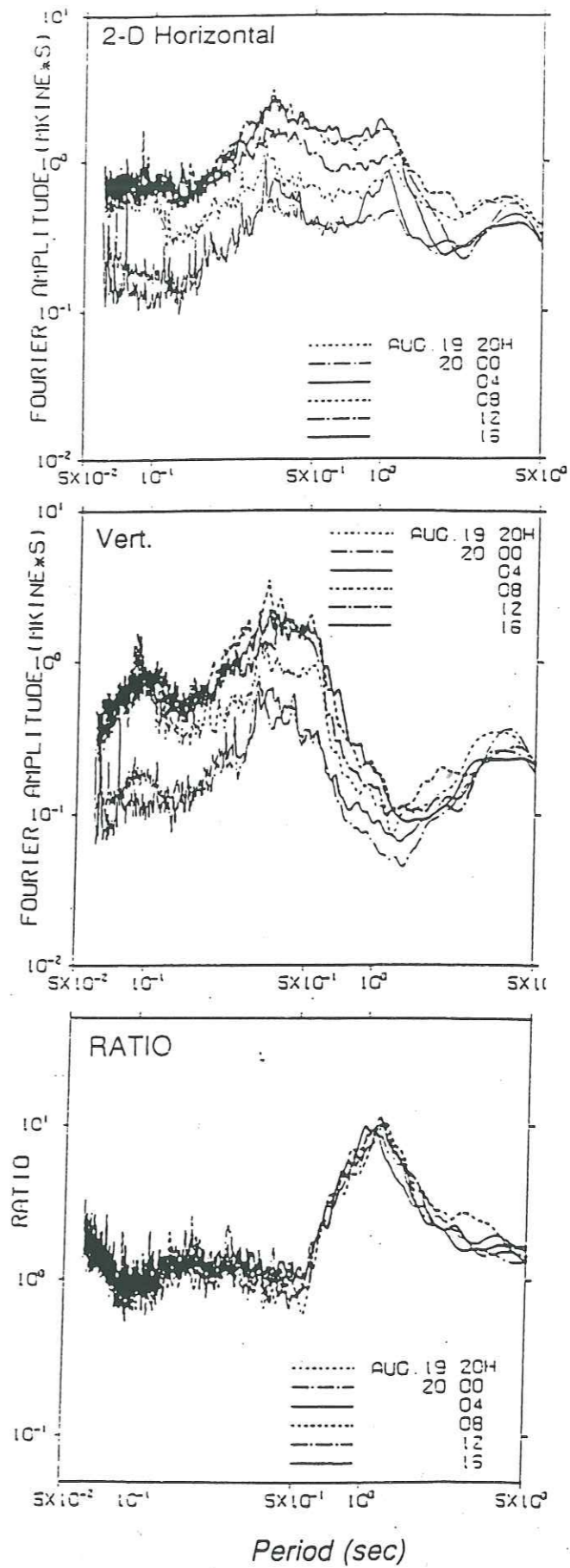
Figure 1.16 : Spectres (lissage avec une fenêtre Parzen de 0.1 Hz) et le rapport spectral H/V correspondant, sur des enregistrements de bruit de fond (Xian-Sheng et al., 1994).
