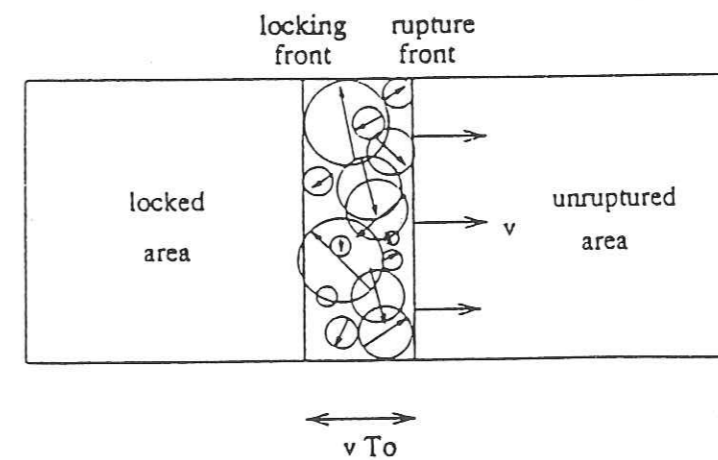
Figure II.20 : Dépendance en fréquence de la directivité. Introduction d'un caractère aléatoire dans la direction de rupture des sous-événements dans la bande de glissement (Bernard et Herrero, 1994).
