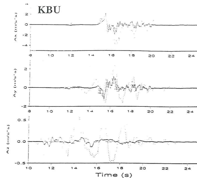
Figure II.49 : Accélérogrammes simulés au site KBU, avec une fonctions de Green unique calculée en bas à gauche du plan de faille (cas 1, trait pointillés serrés), au centre du plan de faille (cas 2, trait plein) et en haut à droite du plan de faille (cas 3, trait pointillés espacés).
