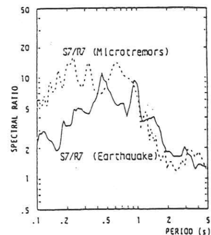
Figure I.9 : Rapports spectraux entre sédiment et rocher pour des séismes et du bruit de fond (Seo et al. , 1989).
