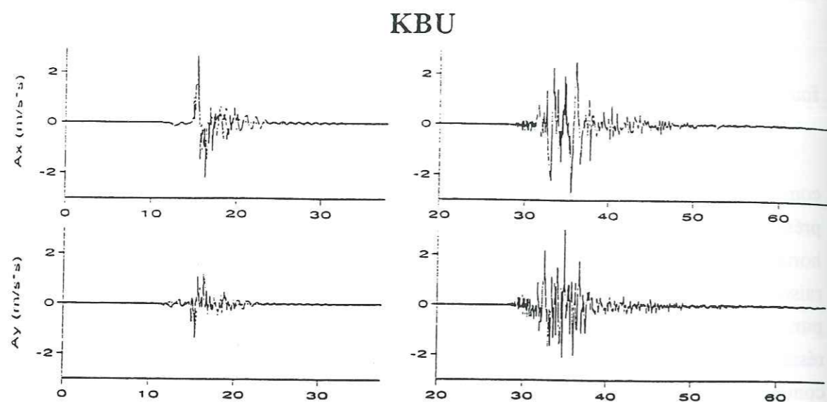
Figure II.53 : Comparaison entre accélérogrammes simulés avec une seule fonction de Green (trait pointillé) et l'interpolation des fonctions de Green en chaque point (trait plein), à gauche; et accélérogramme observé (à droite) ; pour le site KBU.
