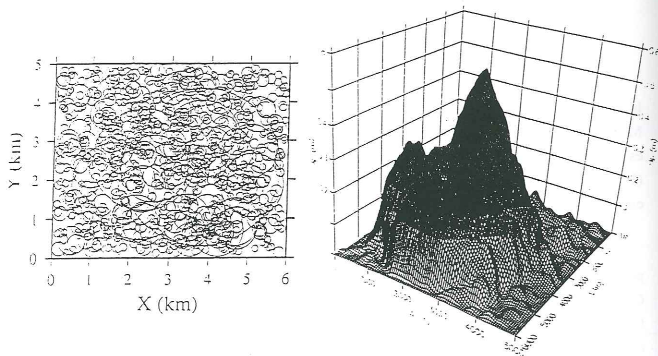
Figure II.65 : Distribution des sous-événements (à gauche) et du glissement (à droite) sur le plan de faille.
