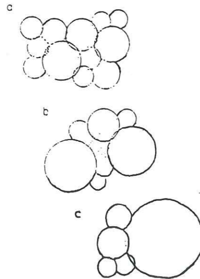
Figure II.12 : Trois distributions de sous-événements réalisées à partir du même modèle. Les sous-événements sont arrangés arbitrairement. Les contours des sous-événements sont indiqués pour montrer les zones d'initiation et d'arrêt de la rupture. Les zones de barrières non cassées à la fin de la rupture sont indiquées par des hachures, pour montrer le relâchement de contrainte pour chaque cas de rupture (Boatwright, 1982).
