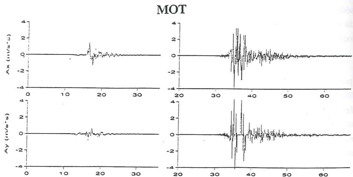
Figure II.54 : Comparaison entre accélérogrammes simulés avec une seule fonction de Green (trait pointillé) et l'interpolation des fonctions de Green en chaque point (trait plein), à gauche; et accélérogramme observé (à droite) ; pour le site MOT. La station qui a enregistré le mouvement en ce site à eu un problème de fonctionnement visible sur l'accélérogramme observé.
