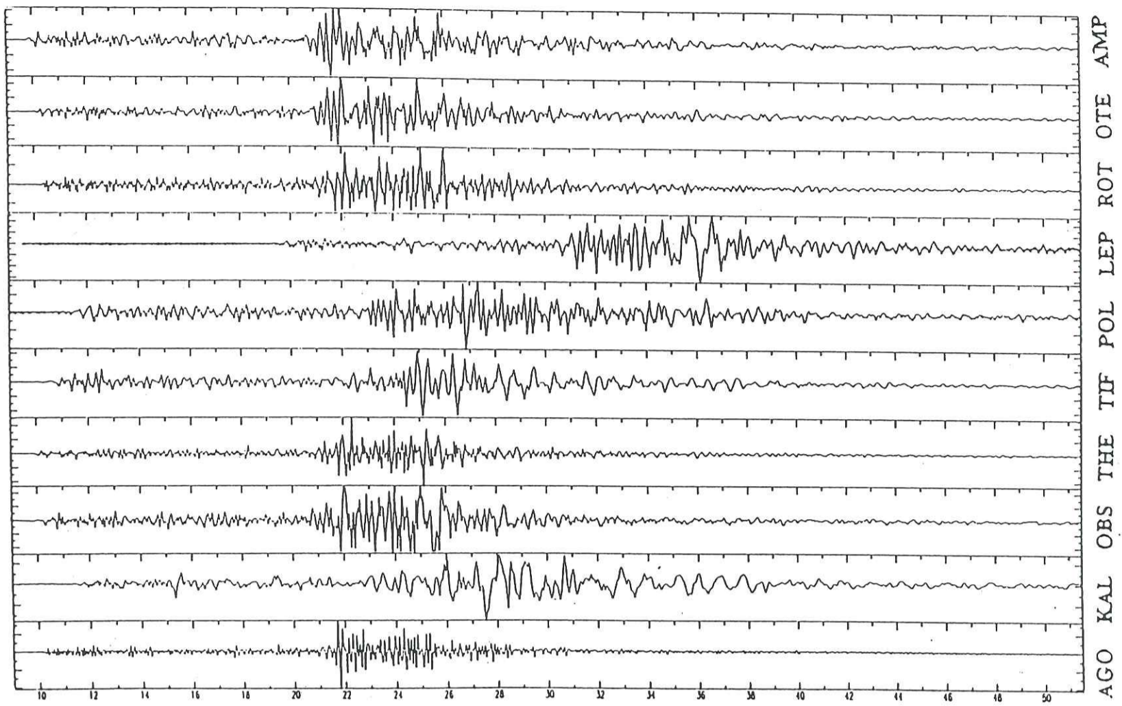
Figure 1.42 : Exemple d'un séisme de magnitude 4.2, à une centaine de km de la ville, enregistré par les stations du réseau temporaire. Composante EW.
