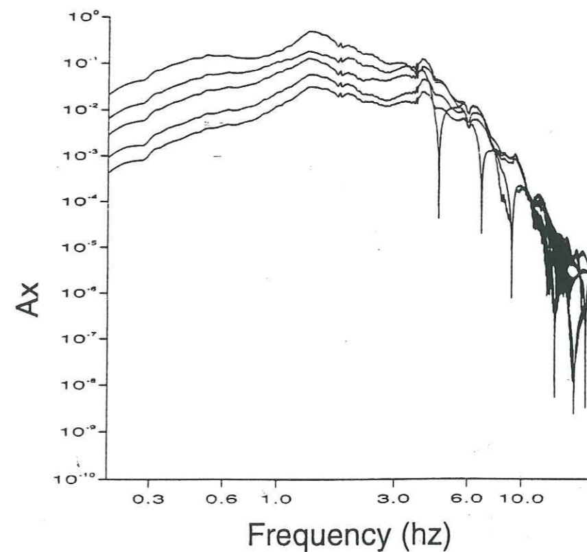
Figure II.32 : Forme du spectre de l'accélération obtenu pour une fissure circulaire unique, pour différents rayons: 1750m, 1166m, 875m, 583m et 437m.
