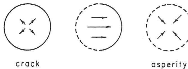
Figure II.11 : Différents comportements de rupture sur un sous-événement. Les contours pointillés et pleins indiquent les zones d'initiation et d'arrêt de la rupture, respectivement ; les flèches montrent la direction de propagation de la rupture. Le premier sous-événement correspond à une faille circulaire, le troisième à une aspérité, et le second à un mélange des deux (Boatwright, 1982).
