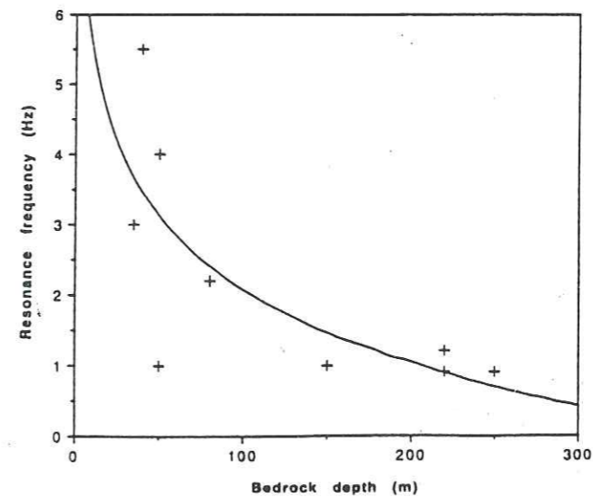
Figure 1.60 : Fréquence de résonance en fonction de la profondeur du substratum, pour chaque site.
