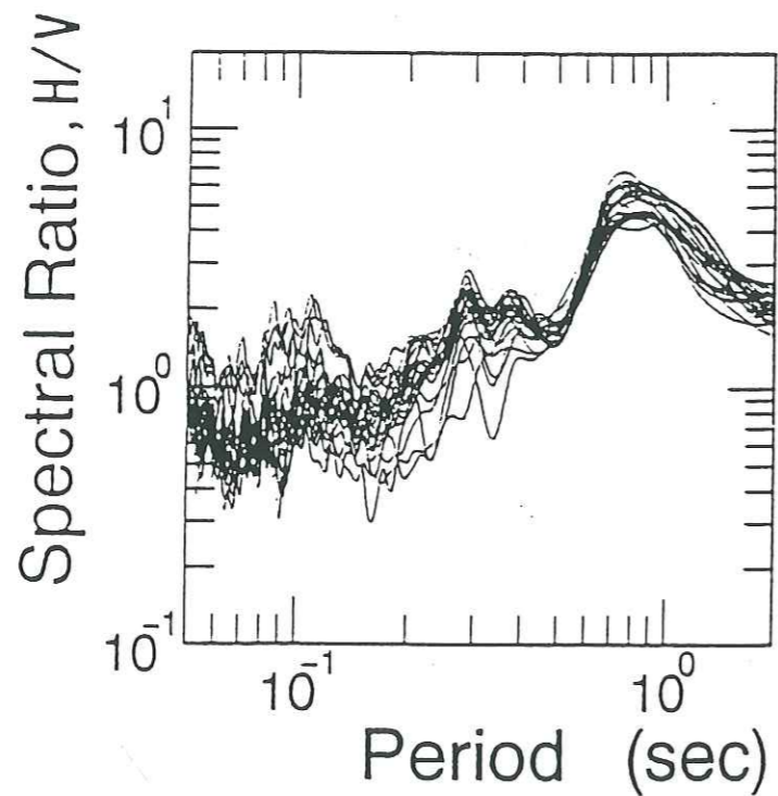
Figure 1.15 : Rapports H/V sur du bruit de fond mesurés chaque heure pendant un jour, à Tokyo (Konno et al., 1994).
