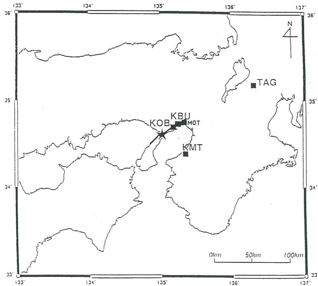
Figure II.41 : Carte des sites étudiés dans la région de Kobe, et trace de la faille en surface.
