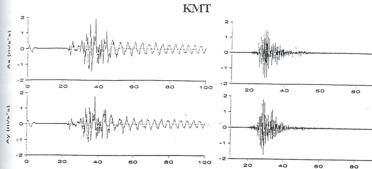
Figure II.55 : Comparaison entre accélérogrammes simulés avec une seule fonction de Green (trait pointillé) et l'interpolation des fonctions de Green en chaque point (trait plein), à gauche; et accélérogramme observé (à droite) ; pour le site KMT.
