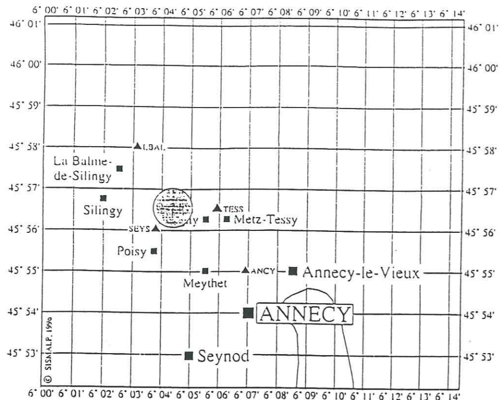
Figure II.74 : Carte indiquant l'épicentre du séisme de Annecy, ainsi que les sites étudiés : LBAL, ANCY, TESS, SEYS.
