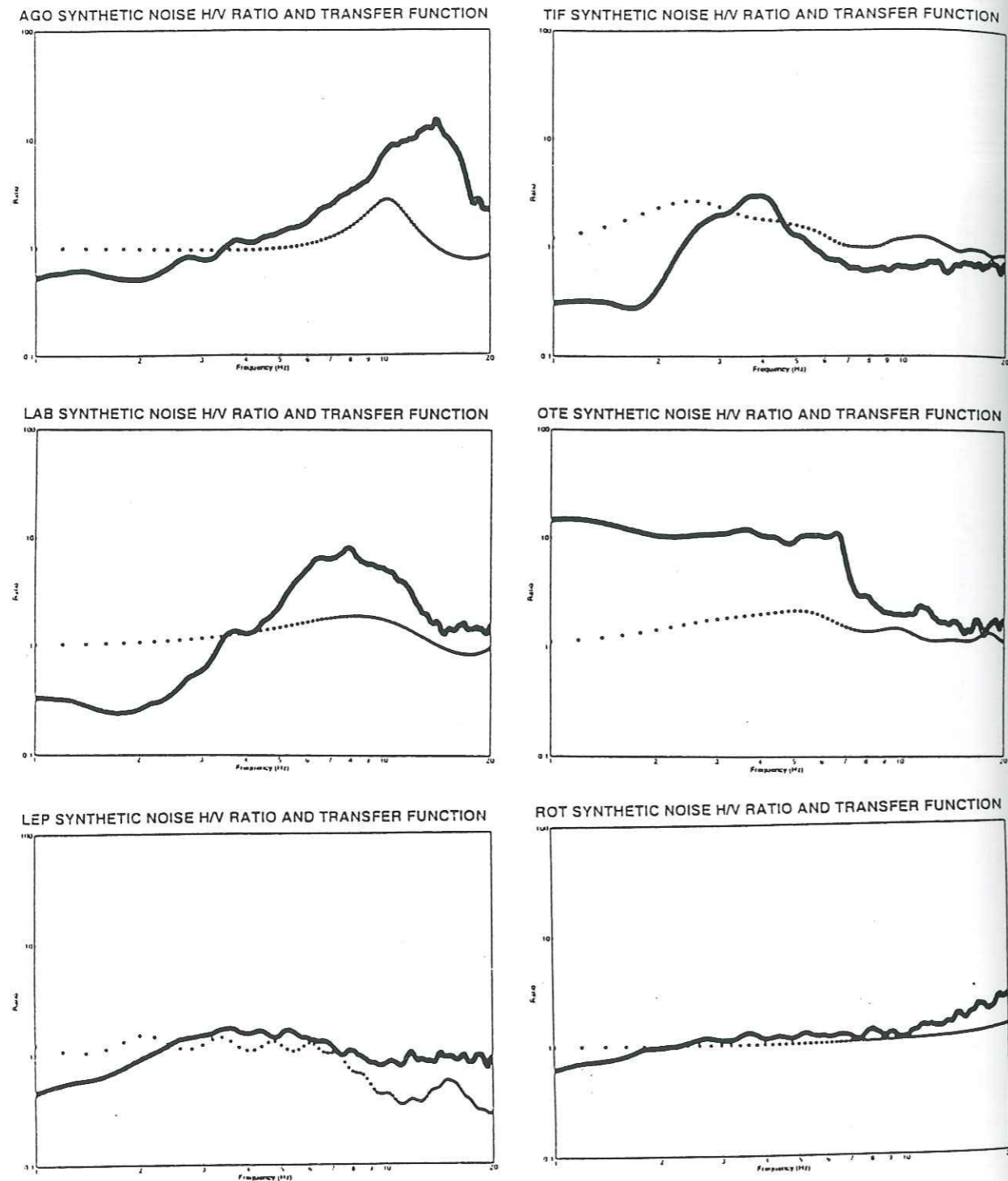
Figure 1.61 : Rapports H/V calculés sur des simulations de bruit ambiant (trait épais) et fonction de transfert en ondes S (trait fin) pour différents sites.
