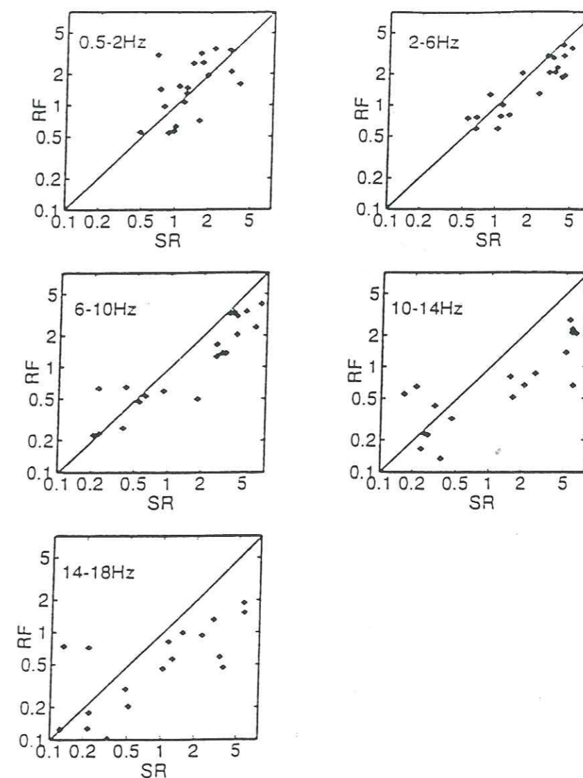
Figure I.54 : Comparaison de l'amplification moyenne arithmétique à chaque site, pour les fonctions récepteur (RF) et les rapports spectraux classiques (SR) pour différentes bandes de fréquence. L'accord entre les deux, se dégrade vers les hautes fréquences.
