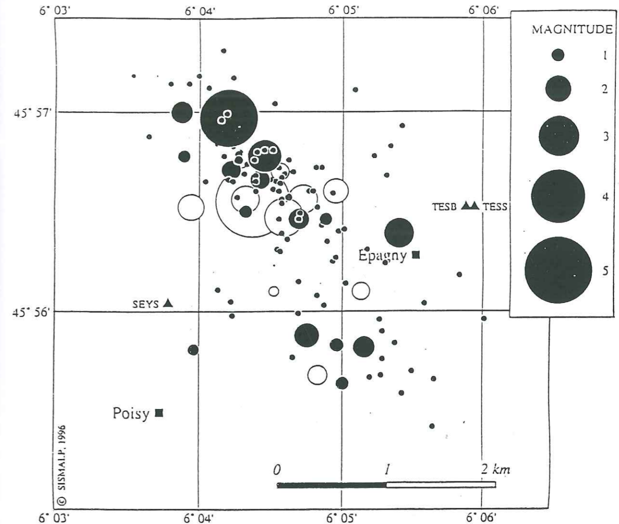
Figure II.72 : Localisation de l'épicentre (cercle de plus grand diamètre) et des répliques du séisme de Annecy (15/07/96).
