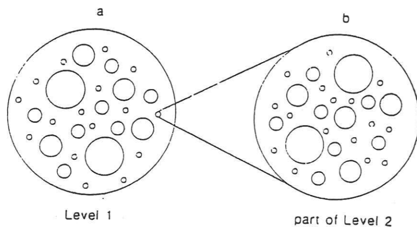
Figure II.14 : (a) Une exemple simplifié d'un modèle de rupture avec une distribution de sous-événements continue self-similaire. Les zones de rupture des sous-événements sont montrées par des cercles de tailles différentes. Le cercle le plus extérieur représente la surface de rupture du choc principal. Les zones de rupture montrées sur la Figure (a) sont les sous-événements de niveau 1. Un agrandissement de l'un des sous-événements (b) montre qu'il contient sa propre distribution self-similaire de sous-événements (niveau 2) (Frankel, 1991).
