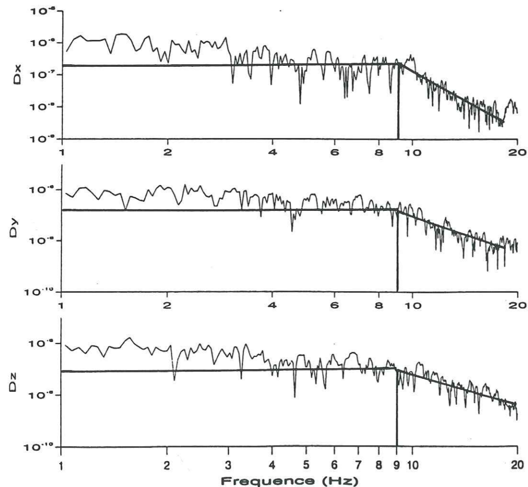
Figure II.63 : Spectres en déplacement de l'enregistrement du séisme de Lancey, à la station au rocher, MUSD. Détermination du niveau plat du spectre basse fréquence et de la fréquence coin, pour calculer la surface de la faille et le moment du séisme.
