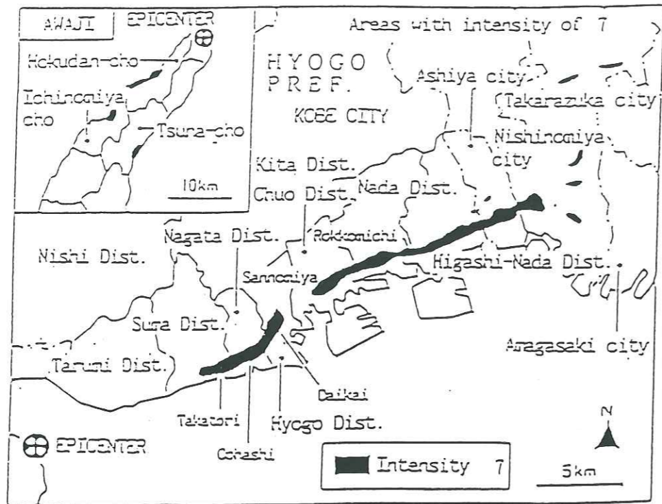
Figure II.40 : Carte montrant les zones de dégâts d'intensité 7 (maximum sur l'échelle japonaise) dans la région de Kobe.
