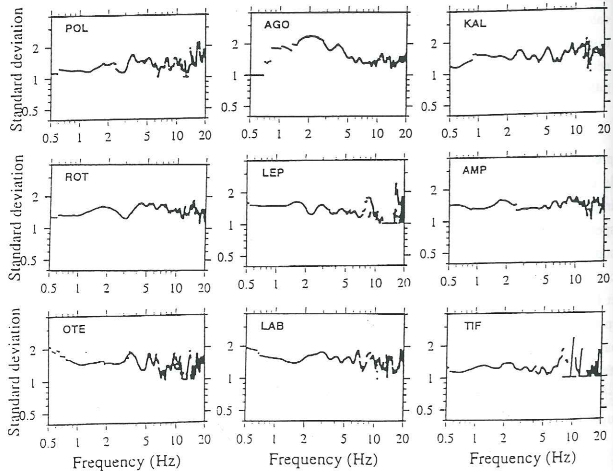
Figure 1.50 : Ecart type à chaque fréquence pour les fonctions récepteur calculées sur tous les séismes, pour chaque site.
