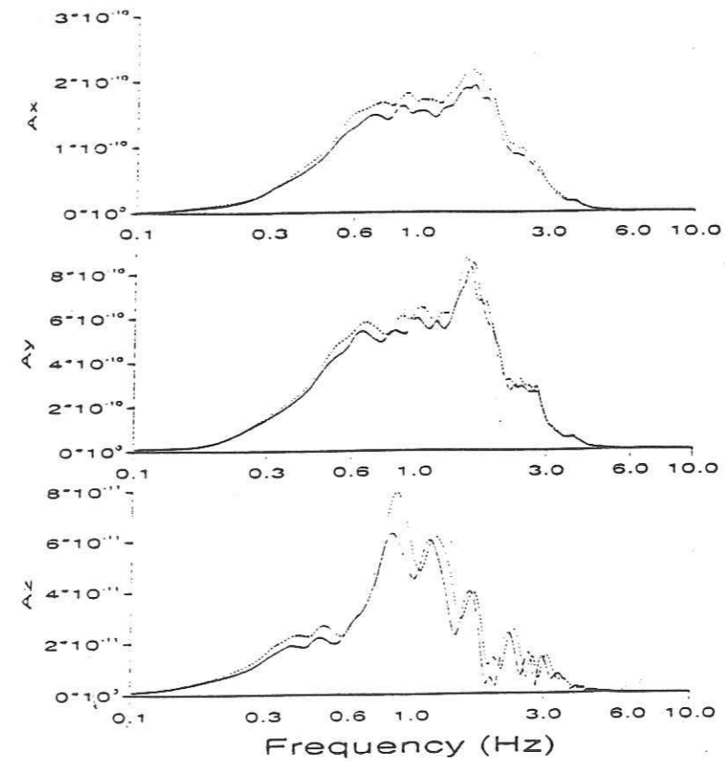
Figure II.37 : Spectres des fonctions de Green calculée (trait plein) et interpolée (trait pointillé) au même point.
