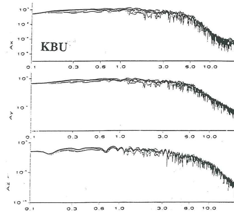
Figure II.48 : Spectres obtenus au site KBU, pour différentes distributions des sous-événements sur la plan de faille.
