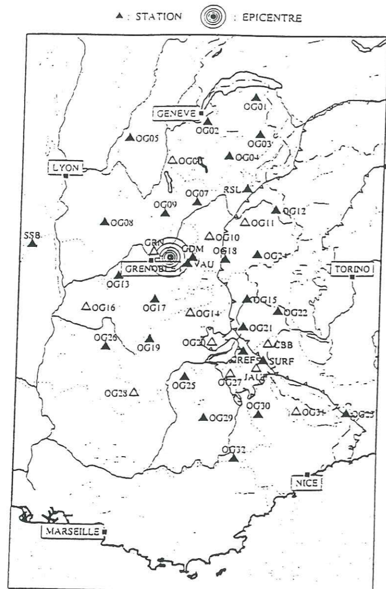
Figure II.58 : Localisation de l'épicentre du séisme de la Combe de Lancey (08/09/95).
