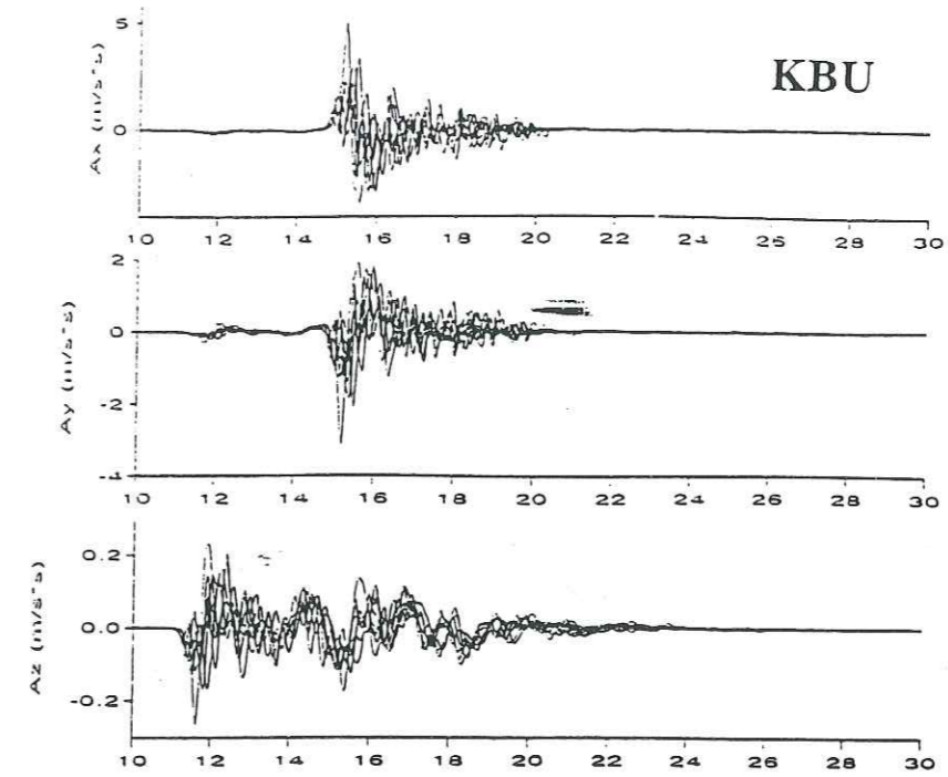
Figure II.47 : Accélérogrammes simulés au site KBU, pour différentes distributions des sous-événements sur la plan de faille.
