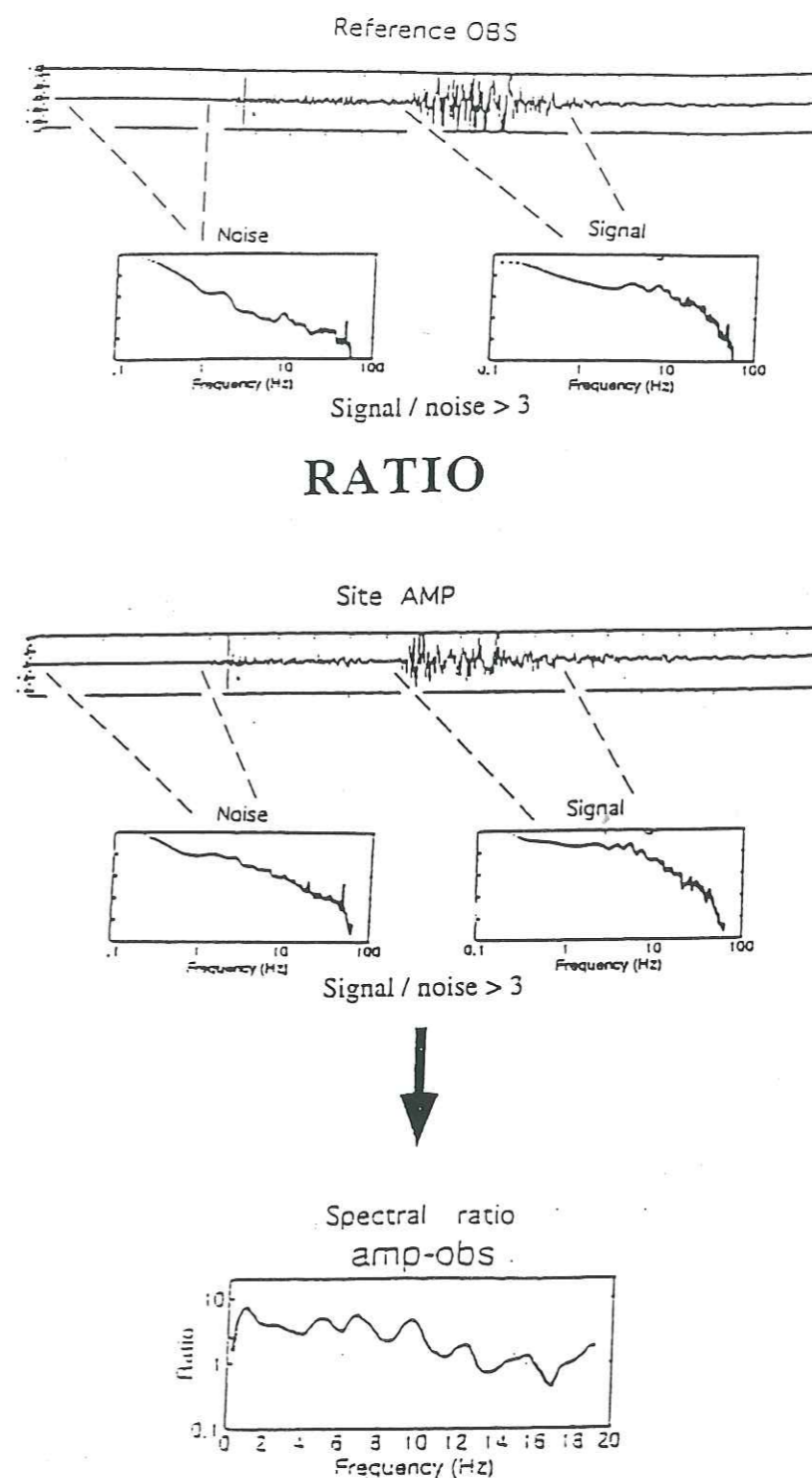
Figure I.4 : Schéma descriptif de la méthode du rapport spectral classique.
