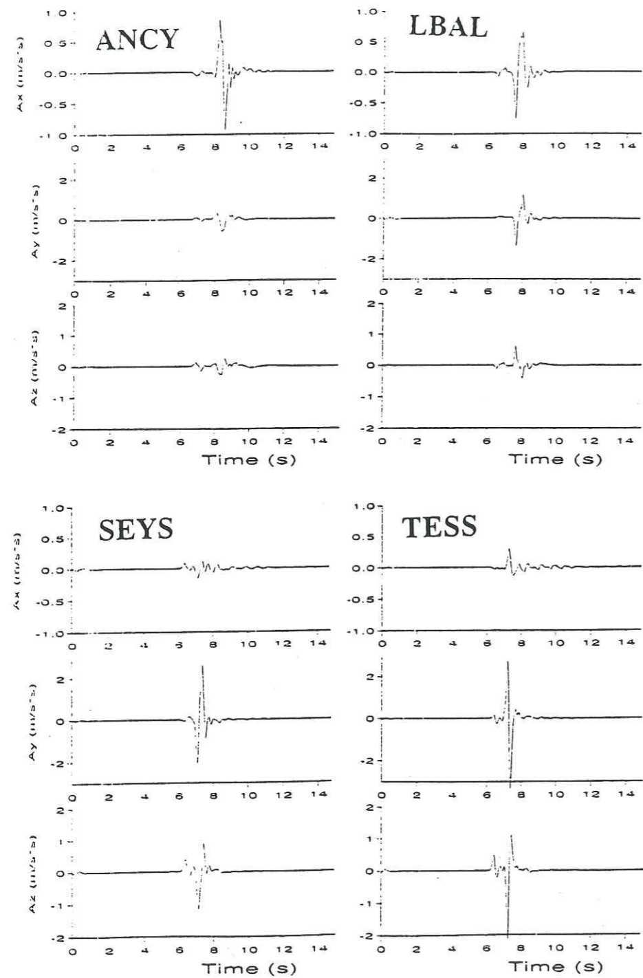
Figure II.75 : Accélérogrammes simulés pour les sites ANCY (en haut à gauche), LBAL (en haut à droite), SEYS (en bas à gauche) et TESS (en bas à droite) ; pour une structure de type "rocher".
