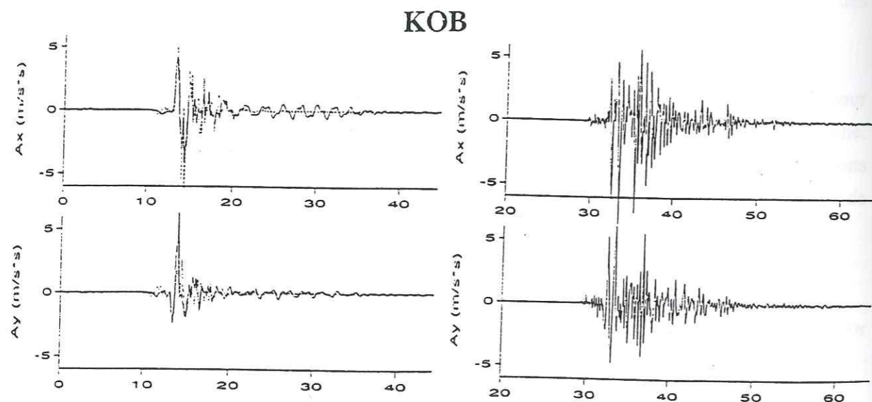
Figure II.52 : Comparaison entre accélérogrammes simulés avec une seule fonction de Green (trait pointillé) et l'interpolation des fonctions de Green en chaque point (trait plein), à gauche; et accélérogramme observé (à droite); pour le site KOB.
