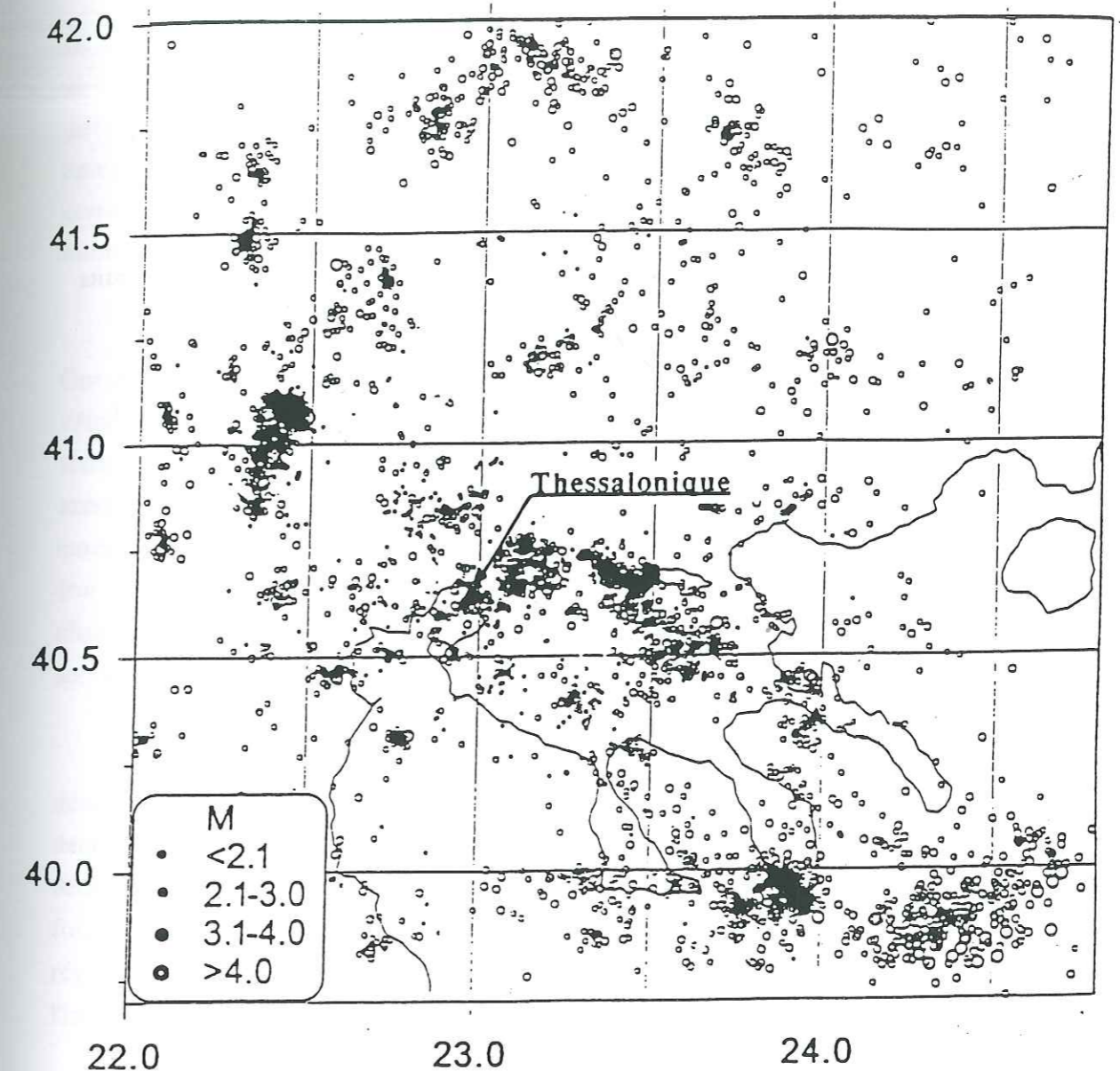
Figure I.38 : Carte de la sismicité enregistrée entre 1981 et 1992 dans la région de Thessalonique (Euro-Seistest, 1994).
