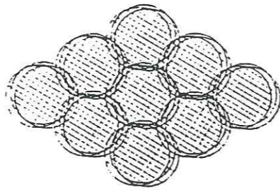
Figure II.13 : Réalisation schématique du modèle à ruptures multiples de Hadley et Helmberger (1980) et Irikura (1983). Chaque point de la surface de faille est supposé casser trois fois (Boatwright, 1988).
