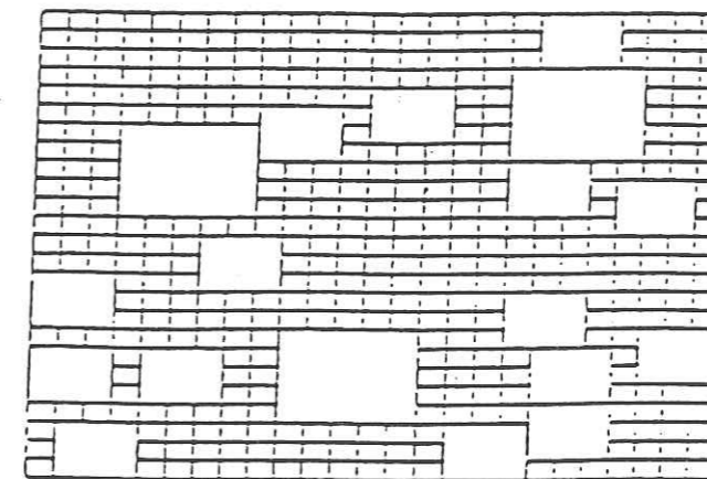
Figure II.16 : Distribution self-similaire de sous-événements, composée de trois différentes tailles de sous-événements (Irikura et Kamae, 1994).
