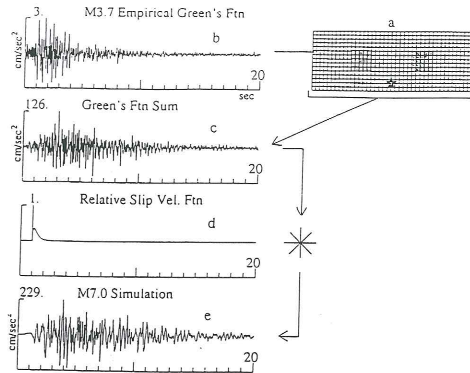
Figure II.24 : Procédure de simulation du choc principal. (a) Modèle de faille utilisé. Les zones ombrées sont des aspérités et l'étoile donne l'hypocentre. (b) Fonction de Green empirique utilisée. (c) Somme des fonctions de Green décalées en temps. (d) Fonction de vitesse de glissement relatif. (e) Simulation de choc principal résultant de la convolution entre la somme des fonctions de Green empiriques et la fonction de vitesse de glissement relatif (Frankel, 1995).
