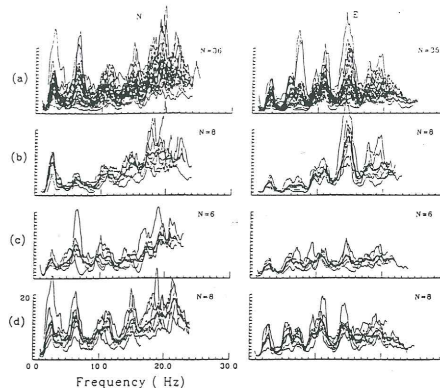
Figure 1.5 : Rapports spectraux (trait fin) et valeur moyenne (trait épais), (a) pour tous les séismes disponibles, (b) pour les événements superficiels au SE, (c) pour les événements superficiels au NE, et (d) pour les événements NE profonds (Gagnepain-Beyneix et al. , 1995).
