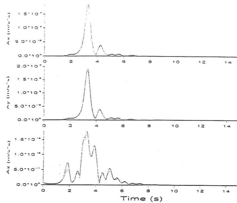
Figure II.36 : Enveloppes des fonctions de Green calculée (trait plein) et interpolée (trait pointillé) au même point.
