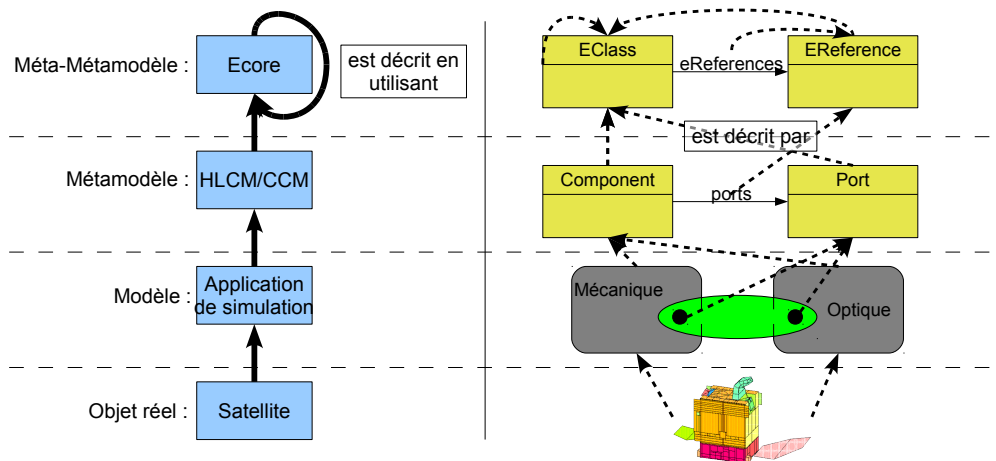
FIGURE 6.1 – Les quatre niveaux de modélisation dans le cadre du projet de modélisation d'ECLIPSE.
