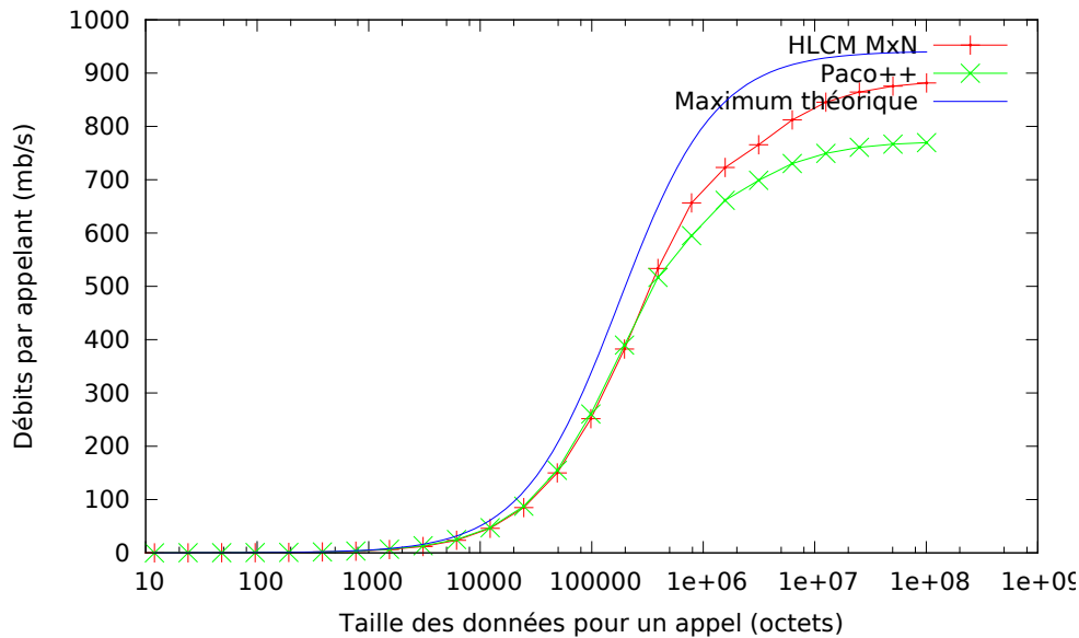
FIGURE 7.28 – Comparaison de la bande passante obtenue sur les appelants lors de l'exécution d'un appel parallèle de méthode M \times N dans le cas où M = 3 et N = 4 . Les résultats obtenus en redistribuant les données sur le fil avec Paco++ et HLCM/CCM sont comparés au maximum théorique. L'axe des ordonnées présente la taille du vecteur distribué utilisé comme paramètre de l'appel selon une échelle logarithmique. L'axe des abscisses présente la bande passante obtenue divisée par trois pour la ramener à chaque processus appelant.
