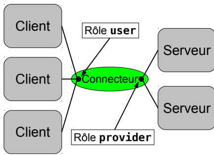
FIGURE 5.1 – Utilisation d'un connecteur pour décrire une interaction par appel de méthode parallèle. Le connecteur représenté par une ellipse possède deux rôles représentés par des cercles pleins : le rôle user et le rôle provider. Chacun de ces rôles est rempli les ports de plusieurs instances de composant pour gérer le cas de l'appel de méthode M \times N dans le cas représenté de deux codes parallèles de degré 3 et 2.
