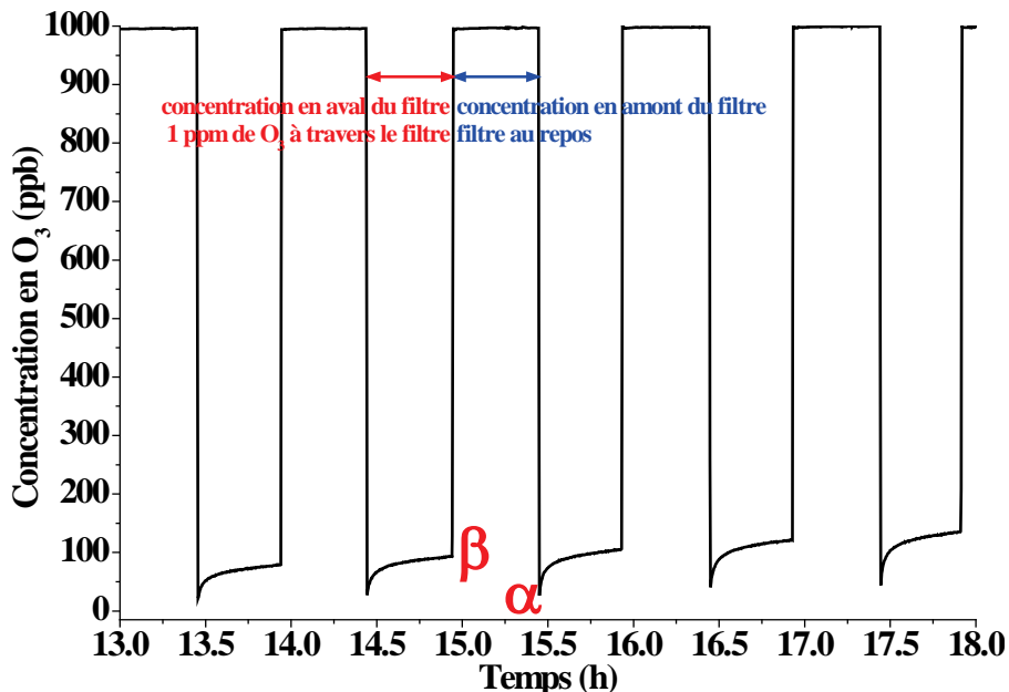
Figure 4-33: Paliers d'exposition relatifs à la phase B montrant la diminution des propriétés de filtration lors du test de durabilité réalisé à une concentration d'ozone proche de 1 ppm.
