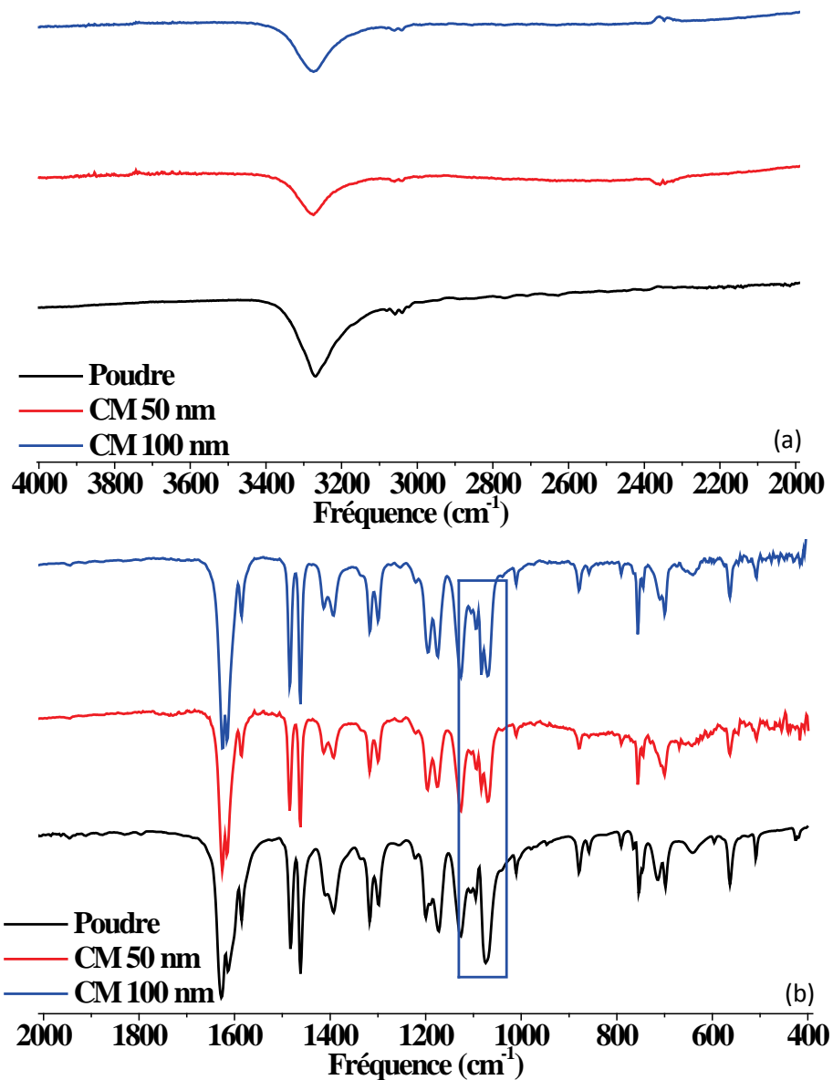
Figure 3-45: Spectre FT-IR de la poudre d'indigo et de deux couches minces de 50 et 100 nm d'épaisseur entre 4000 et 2000 cm⁻¹ (a) et entre 2000-400 cm⁻¹ (b).
