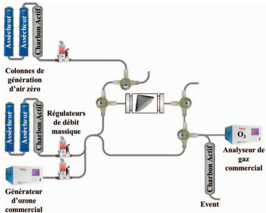
Figure 5-6: Synoptique du banc de mesure développé pour expérimenter le nettoyage sous air zéro du filtre nanocarboné.
