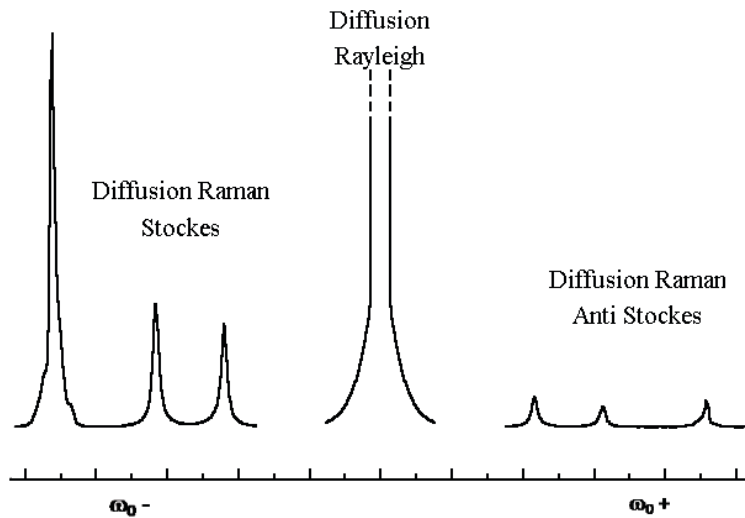
Figure 2-14: Représentation schématique d'un spectre Raman avec les contributions élastique (Rayleigh) et inélastiques (Stokes et anti-Stokes) [6].
