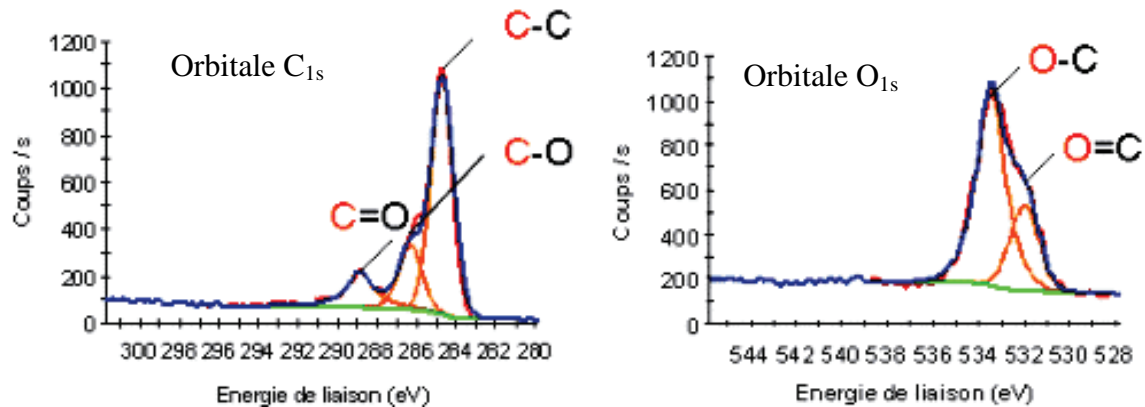
Figure 2-34: Déconvolutions des contributions pour les orbitales C_{1s} et O_{1s} dans le cas d'une liaison C-O [18].
