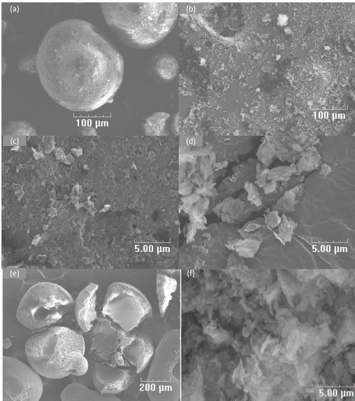
Figure 3-14: Images MEB indigo Ac (a, c, e et f) et indigo K (b et d) ; grossissement x 100 (e), x 250 (a et b) et x 5000 (c, d et f)
