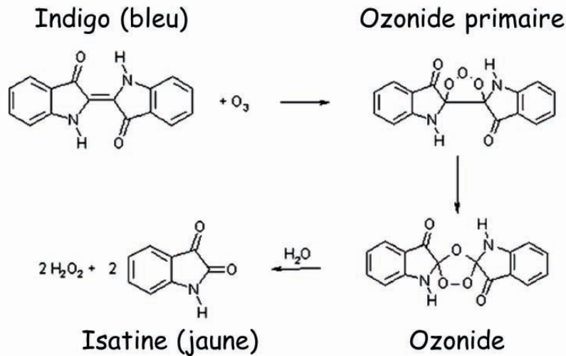
Figure 3-27: Réaction d'ozonolyse de la molécule d'indigo.
