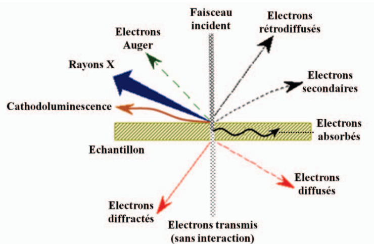
Figure 2-31: Schéma des interactions entre le faisceau électronique incident et l'échantillon.
