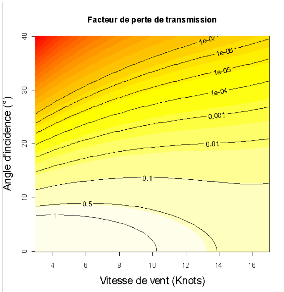
Fig. 2. Facteur de perte de transmission à travers la surface (Réflectance) en fonction de l'angle d'incidence et de la vitesse du vent (en nœuds marins) pour une direction orthogonale du vent.
