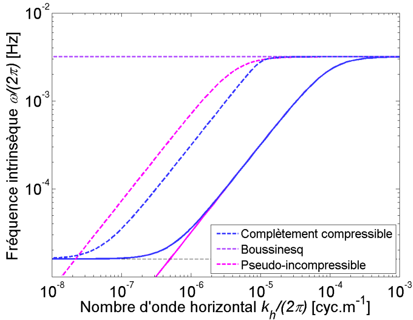
FIGURE A.2 – Comparaison entre les solutions des équations de dispersion (2.40) (bleu), (2.45) (violet) et (2.46) (rose) dans le domaine (\hat{\omega}, k_h) pour m = 10^{-4} cyc.m ^{-1} (solide) et m = 0 (pointillés).
