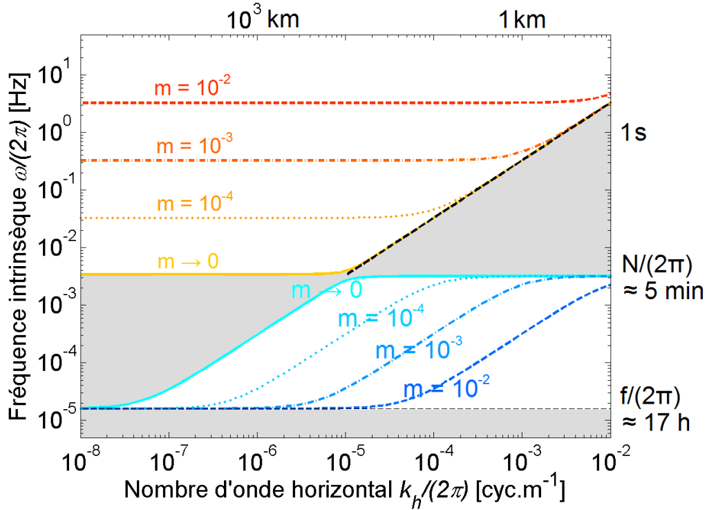
FIGURE 2.2 – Solutions de l'équation de dispersion (2.38) dans le domaine (\hat{\omega}, k_h) pour différentes valeurs du nombre d'onde vertical m [ \text{cyc.m}^{-1} ]. Les courbes de couleur rouge/orange correspondent aux solutions acoustiques-gravité, celles de couleur bleu aux solutions inertie-gravité. La droite en noir représente l'équation de dispersion simplifiée des ondes sonores, les zones grisées les domaines où l'équation de dispersion n'admet aucune solution.
