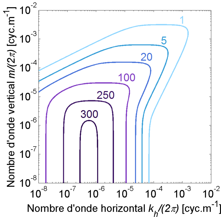
FIGURE 2.6 – Module de la vitesse de groupe des ondes de gravité |c_g| [ \text{m.s}^{-1} ] dans le domaine (k_h, m) .
