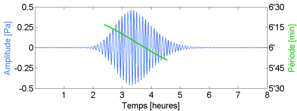
FIGURE 2.16 – Amplitude de la fluctuation de pression [Pa] au niveau du sol à x = 12 km.
