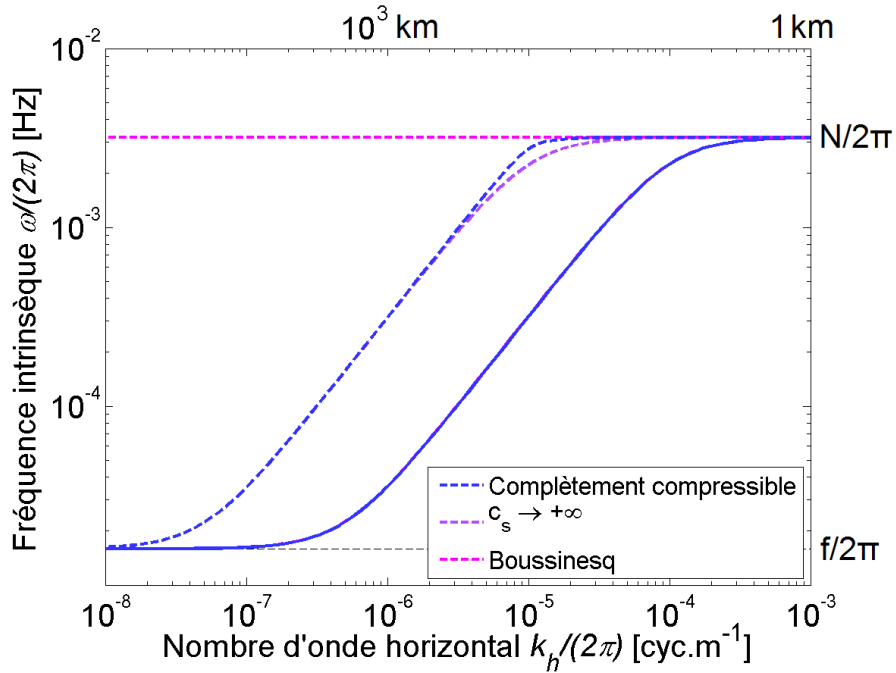
FIGURE 2.4 – Comparaison entre les solutions des équations de dispersion (2.40) (bleu), (2.45) (violet) et (2.46) (rose) dans le domaine (\hat{\omega}, k_h) pour m = 10^{-4} \text{ cyc.m}^{-1} (solide) et m = 0 (pointillés).
