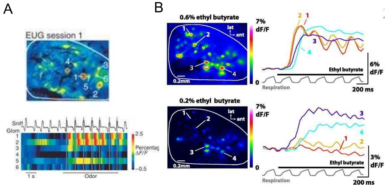
Figure I.7. Dynamique temporelle des cartes d'activation visualisée par imagerie calcique. A. En haut : carte d'activation en réponse à l'eugenol (6 glomérules détectés) chez l'animal éveillé restreint de ses mouvements. En bas : décours temporel de l'activation des différents glomérules : chaque glomérule a son temps de latence et l'intensité de son activation varie pendant la durée de la stimulation odorante. Notez les différences d'activation du glomérule au sein de chaque cycle respiratoire. B. A gauche : cartes d'activations induites par l'ethyl butyrate à 0,2 et 0,6 % chez la souris anesthésiée et trachéotomisée. A droite : les décours temporels d'activation des quatre glomérules. Notons les différences d'intensité d'activation présentée par un même glomérule (1 ou 2) notamment pendant la forte stimulation. A. Figure adaptée de Verhagen et al., 2007. B. Adaptée de Spors et al., 2006.
