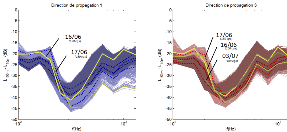
Figure 3.6 : spectres d'atténuation sonore à 150 m de la source relatifs au spectre de référence à 10 m selon les axes de propagation DP1 et DP3 groupés selon la première partie (clair) et la deuxième partie (foncé) de la campagne. En traits pointillés, écarts types des spectres obtenus en conditions homogènes. En jaune, les spectres obtenus pour les trois échantillons retenus.
