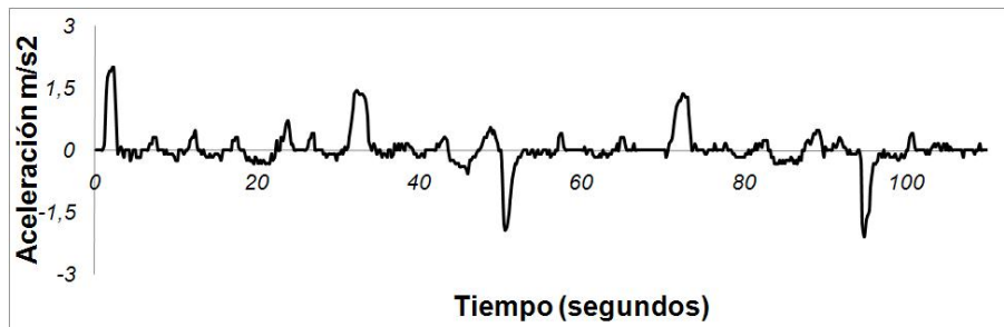
(c) Aceleación del vehículo, experimento 2
