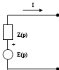
Figure 2.5 : Schéma électrique équivalent simplifié d'une batterie en Laplace
