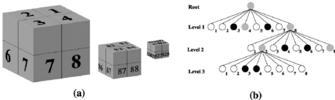
Figure 22 : Définition d'un octree [Ding04]
