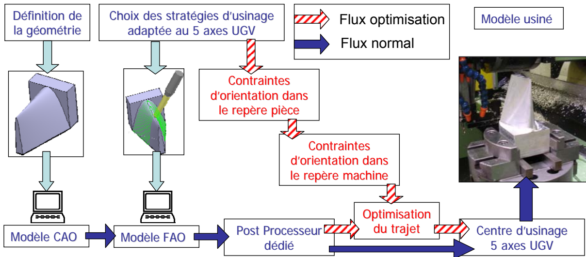
Figure 49 : Flux classique et avec optimisation de la CFAO
