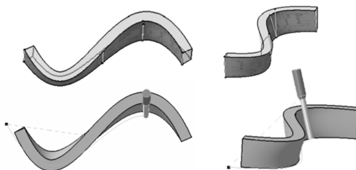
Figure 76 : Géométrie d'une pièce d'essai
