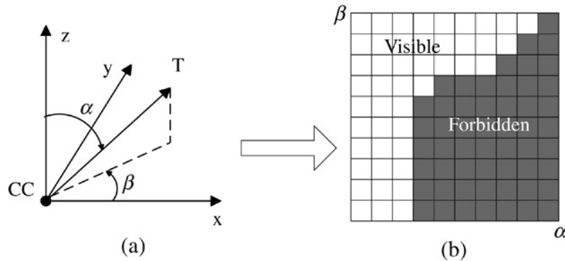
Figure 19 : Définition des zones accessibles pour les deux angles [Wang07]
